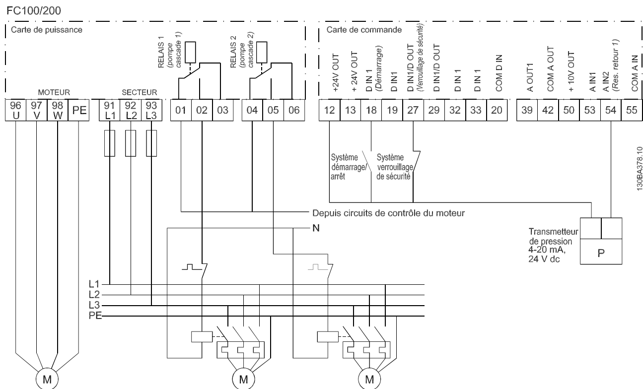
Illustration 12.6 Schéma de câblage du contrôleur de cascade
