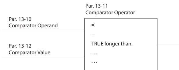
Illustration 5.5 Comparateurs
