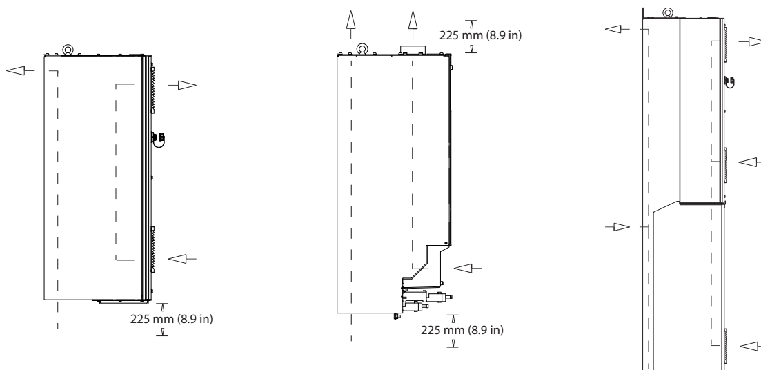
Illustration 5.18 Configuration de circulation d'air en option à l'aide de kits de refroidissement par canal de ventilation arrière pour les boîtiers D1h–D8h.
