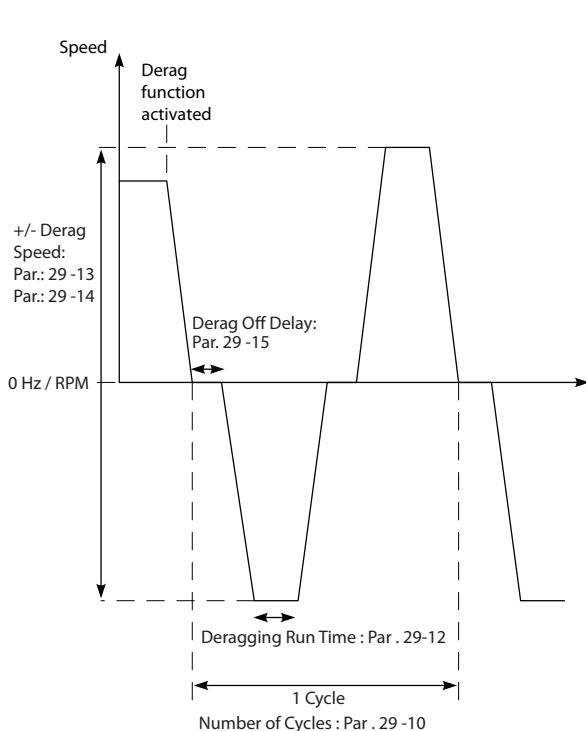
Disegno 5.12 Funzione di pulizia
