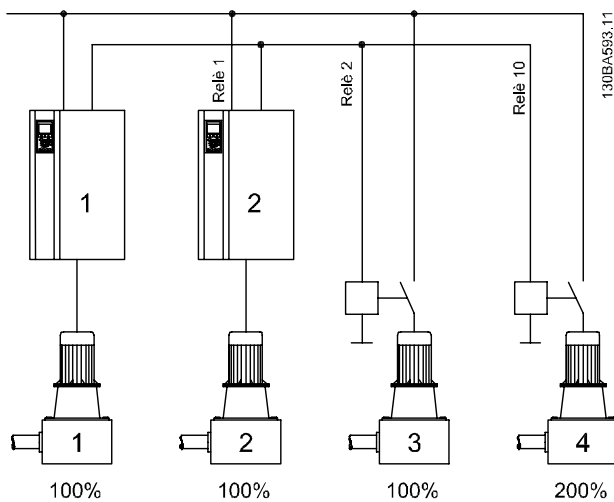
Disegno 5.8 Panoramica delle applicazioni
