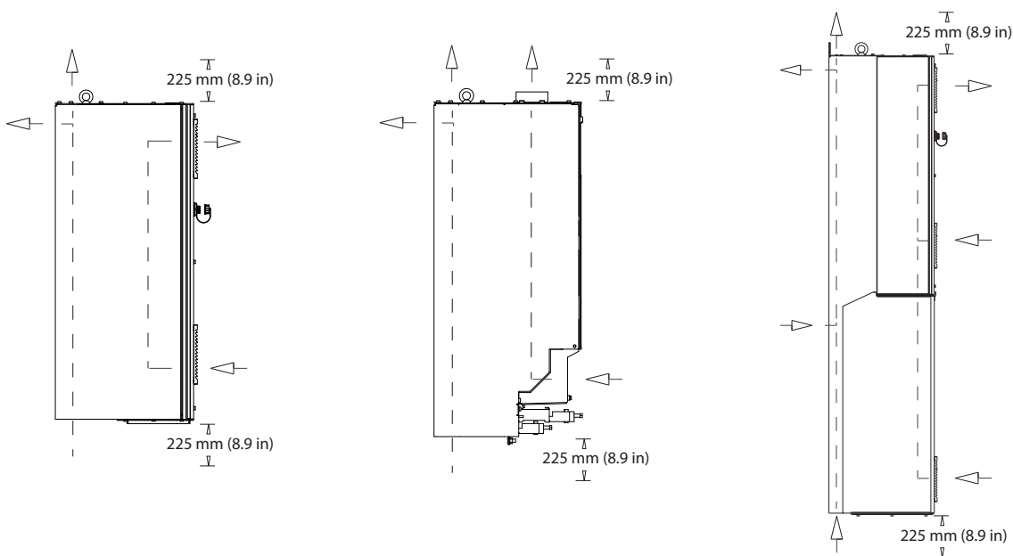
Disegno 5.17 Configurazione di flusso d'aria standard per frame D1h/D2h (sinistra), D3h/D4h (centro) e D5h/D8h (destra).
