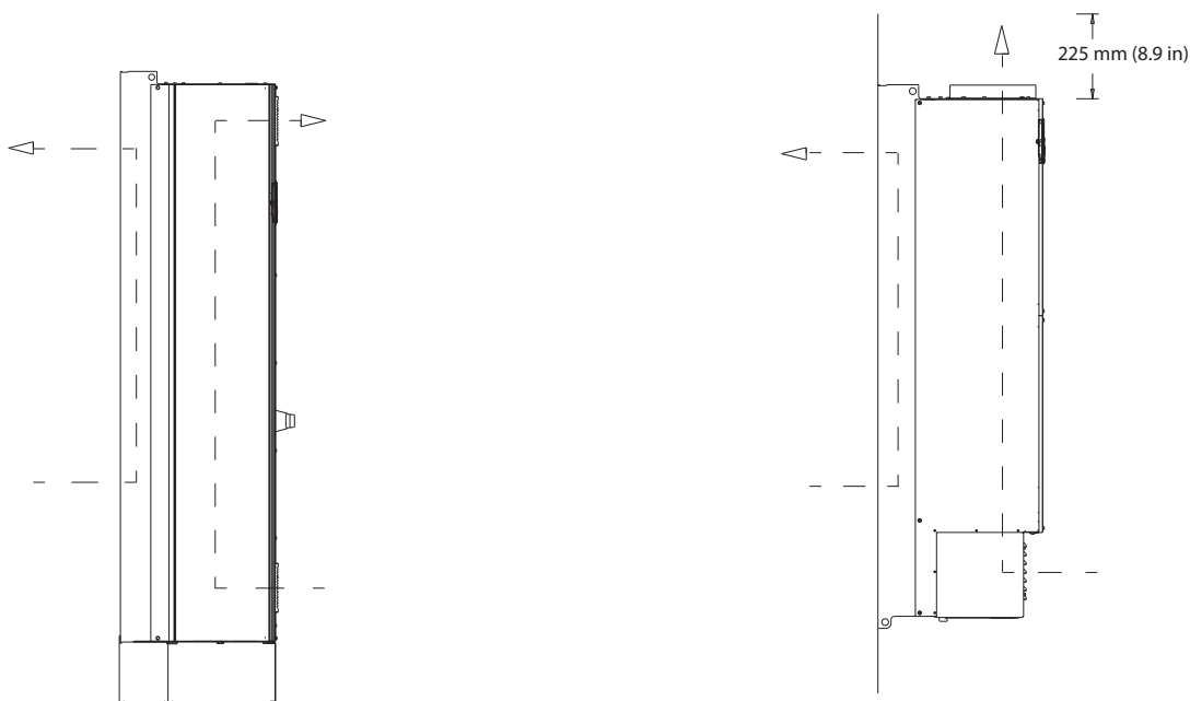
Disegno 5.20 Configurazione opzionale di flusso d'aria attraverso la parete posteriore per E1h/E2h (sinistra) ed E3h/E4h (destra)
