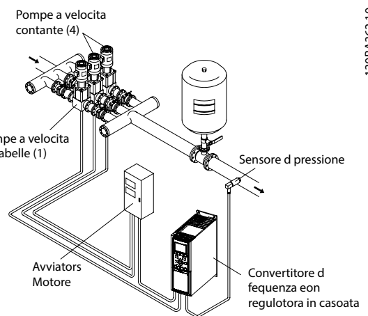
Disegno 5.10 Controllore in cascata di base
