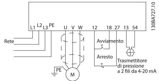
Disegno 12.4 Cablaggio per applicazione a pompa sommersa
