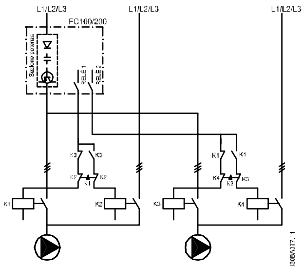
Disegno 12.8 Schema di cablaggio dell'alternanza della pompa primaria.
