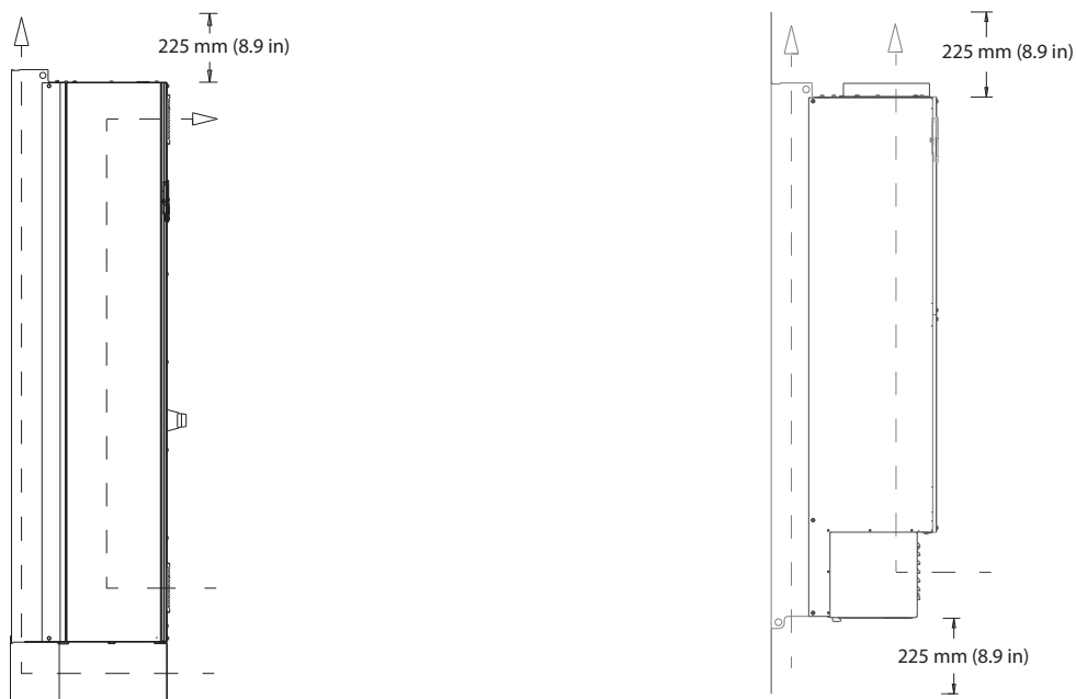
图 5.19 E1h/E2h (左) 和 E3h/E4h (右) 的标准气流配置
