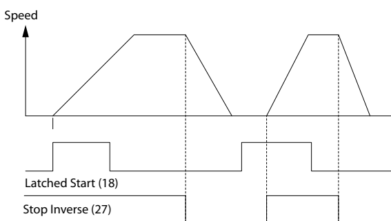
图 12.2 自锁启动/停止反逻辑
