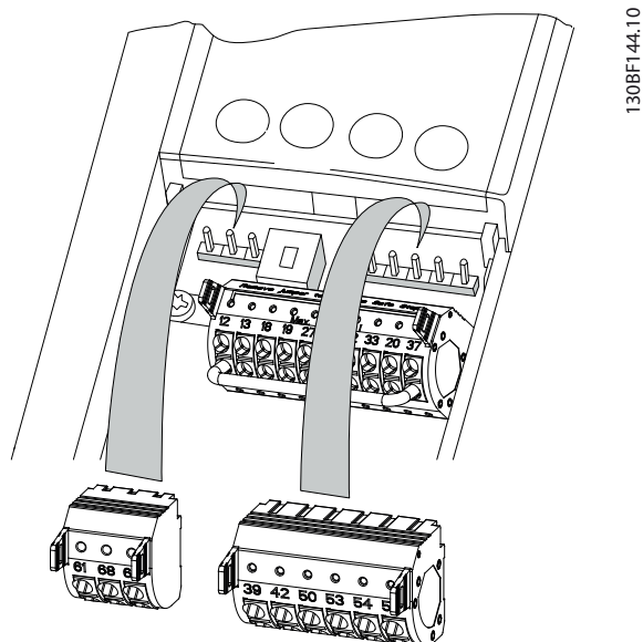
图 10.6 控制端子位置
