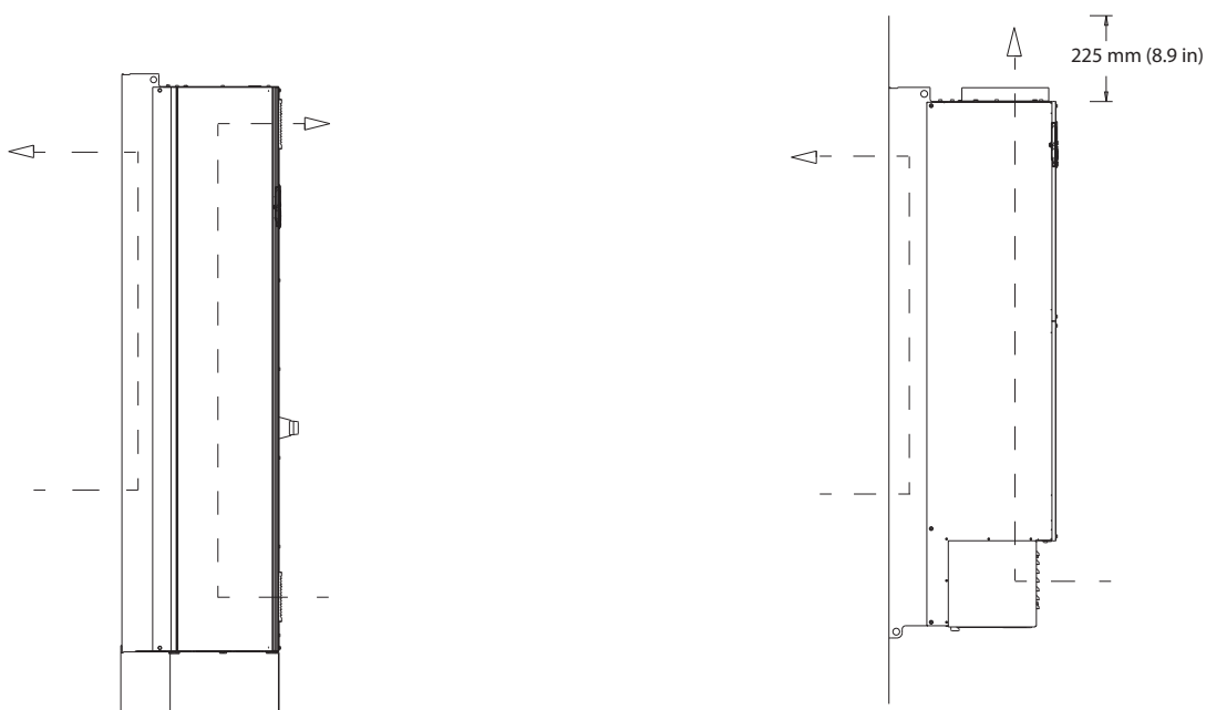
图 5.20 E1h/E2h (左) 和 E3h/E4h (右) 上通过后壁的可选气流配置
