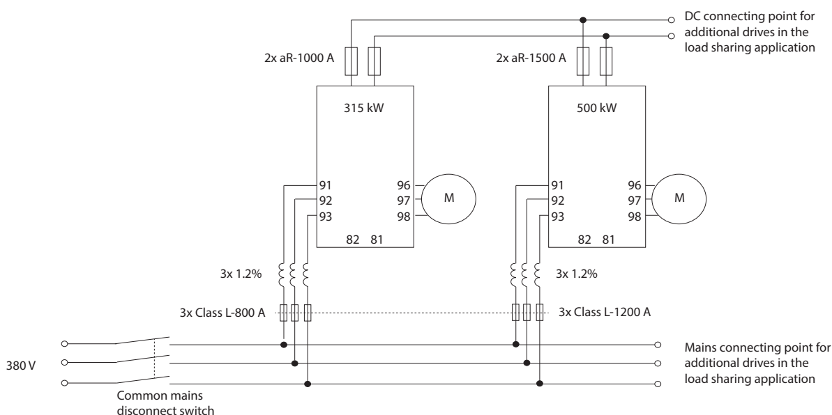
图 5.16 应用最佳做法的负载共享应用的图表
