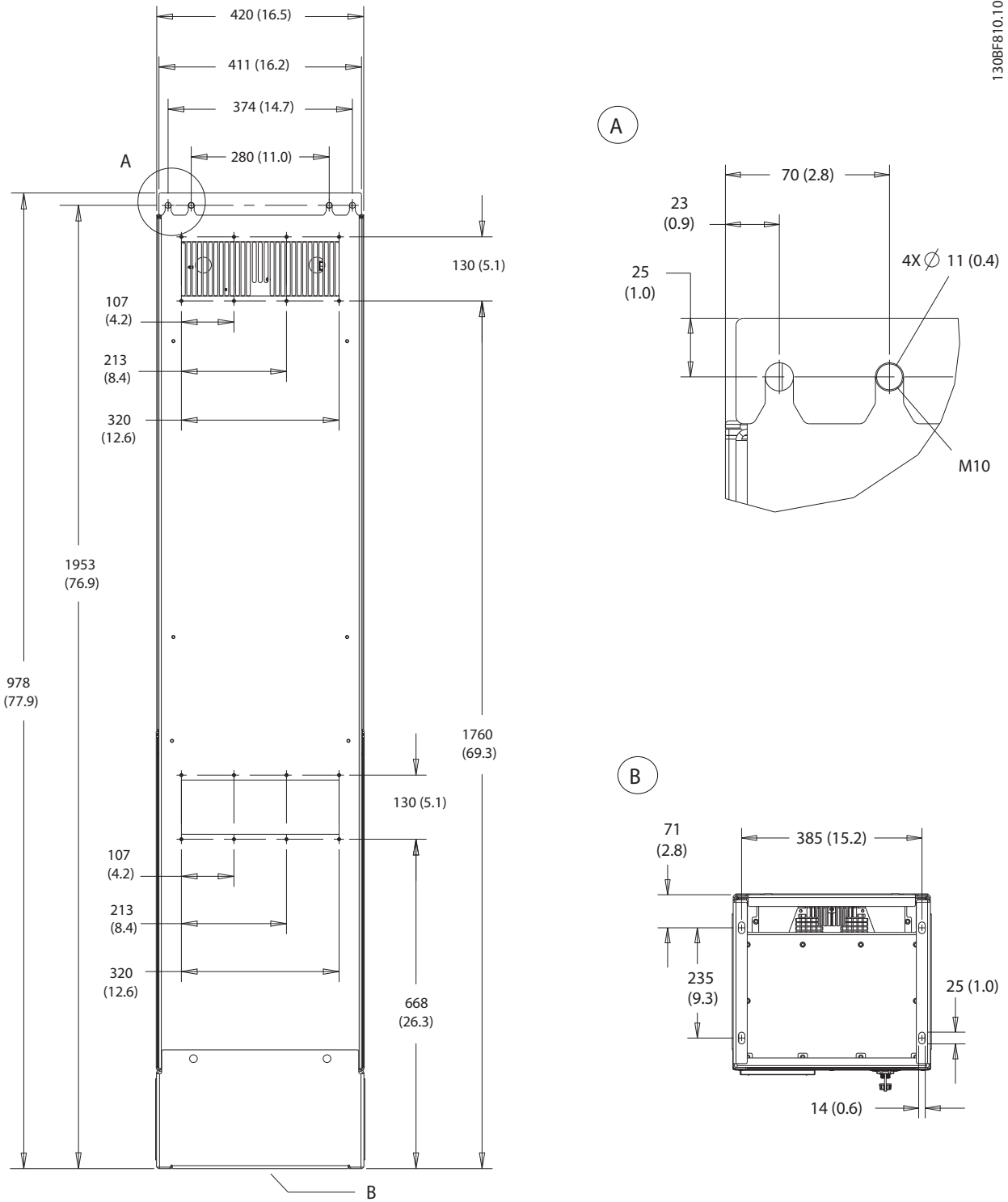
图 8.49 D7h 的后视图
