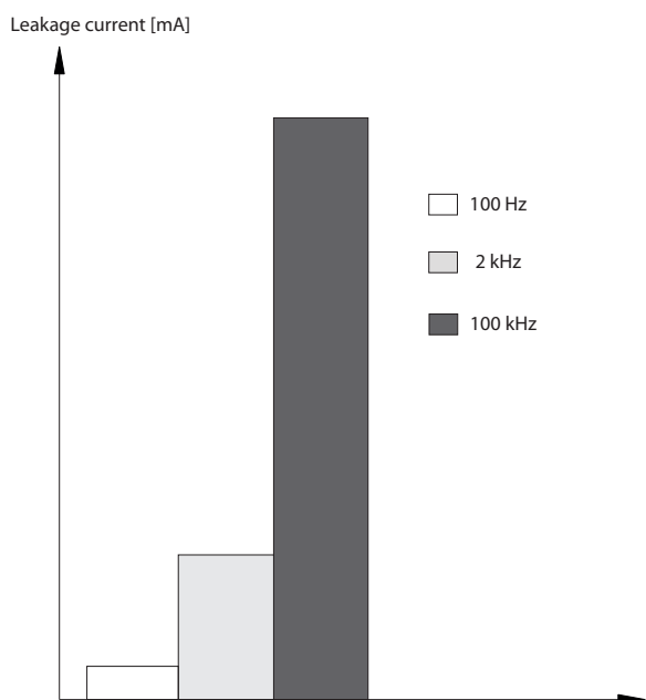
图 10.15 RCD 截止频率对漏电电流的影响
