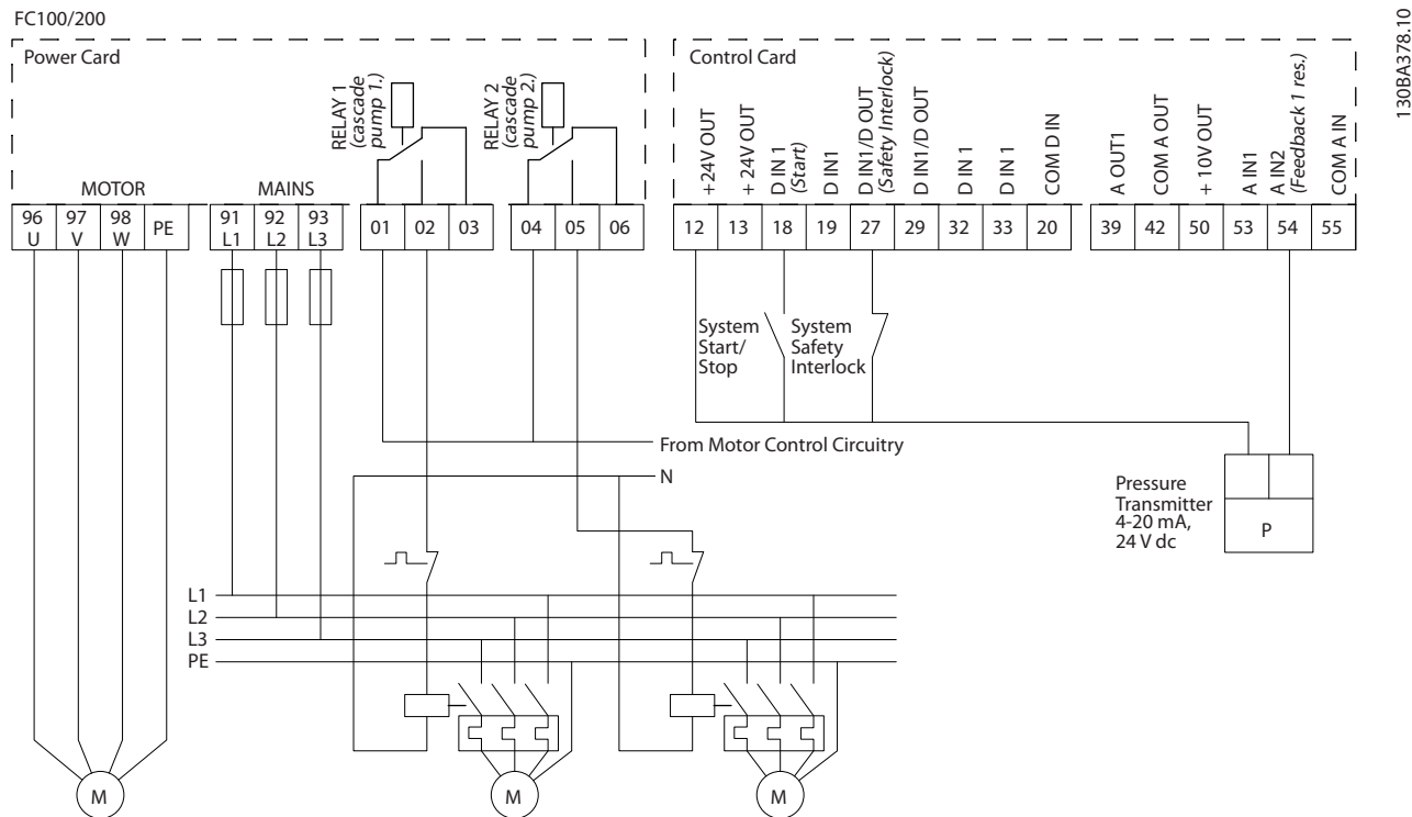
图 12.6 多泵控制器接线图
