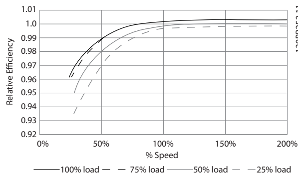
图 10.16 典型效率曲线
