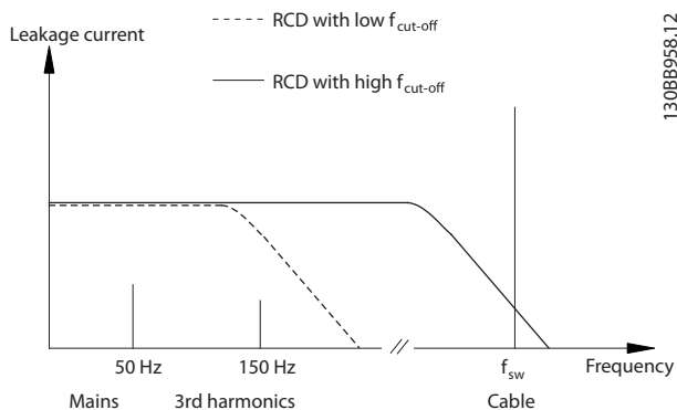
图 10.14 漏电电流的主要成分
