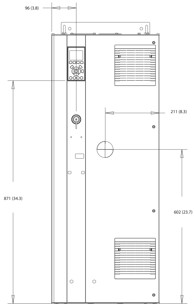
图 8.8 D2h 的正视图
