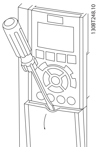
Ilustrația 2.9 Accesul la cablajul de control pentru carcasa A2, A3, B3, B4, C3 și C4
