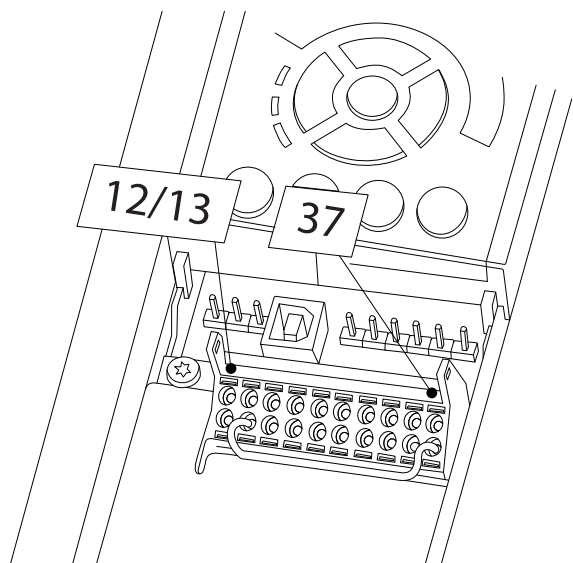
Ilustrația 2.19 Conductor de șuntare între borna 12/13 (24 V) și 37
