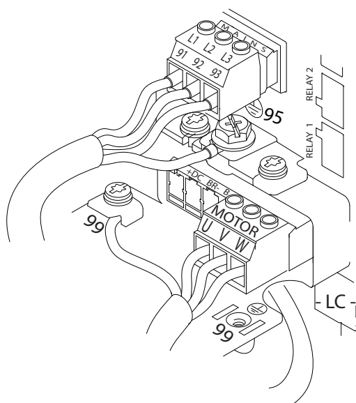
Ilustrația 2.8 Exemplu de cabluri de motor, de rețea de alimentare și de împământare
