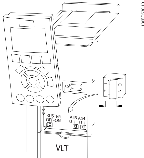
图 4.10 端子 53 和 54 的开关位置
