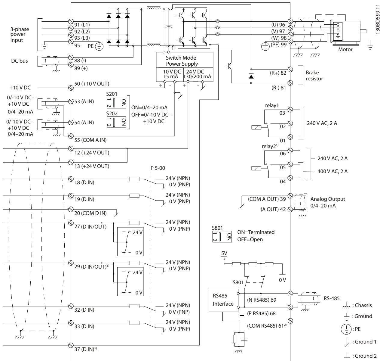
図 4.2 基本配線図
