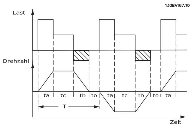
Abbildung 5.8 Typischer Bremszyklus
