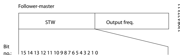
Abbildung 12.17 Zustandswort
