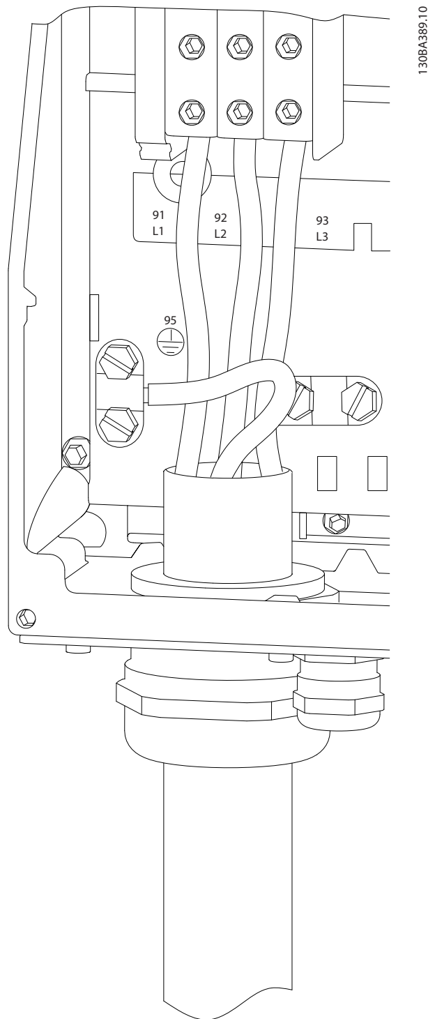
Abbildung 9.26 Netzanschluss Baugrößen C1 und C2 (IP21 und IP55/66).
