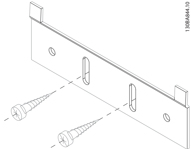
Abbildung 11.30 Untere Halterung
