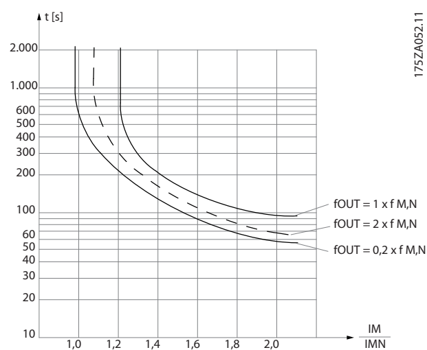
Abbildung 4.1 ETR-Eigenschaften
