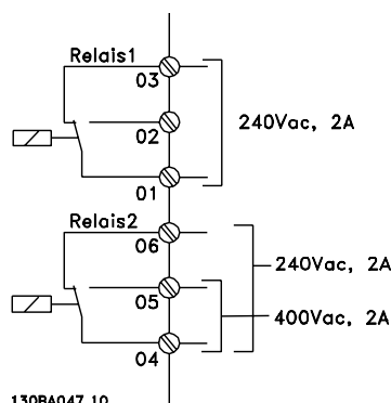
Abbildung 9.41 Relaisausgänge 1 und 2
