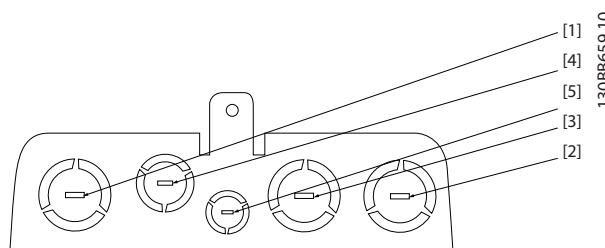
Abbildung 9.6 A5- IP55 Geschraubte Kabeleinführungsöffnungen
