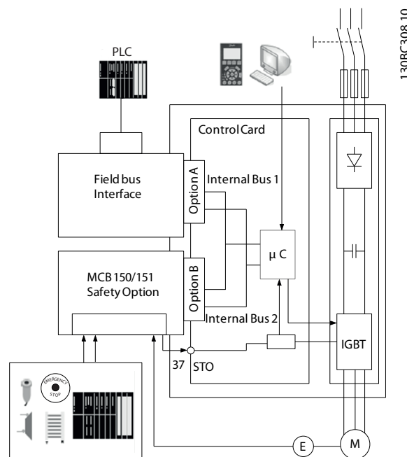
Abbildung 11.19 Sicheres Antriebssystem
