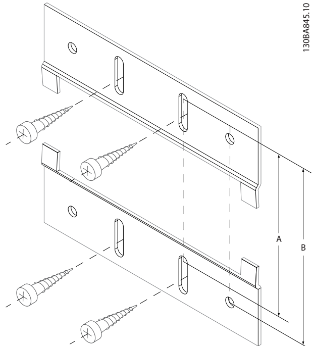
Abbildung 11.31 Obere Halterung
