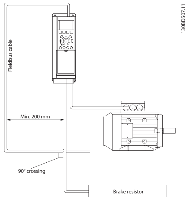
Abbildung 12.4 Kabelführung
