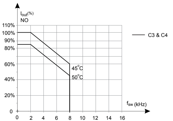
Abbildung 6.27 Leistungsreduzierung von I_{out} für abweichende T_{AMB, MAX} für die Bauformen C3 und C4, mittels SFAVM im Modus „Normale Überlast“ (110 % Übermoment)
