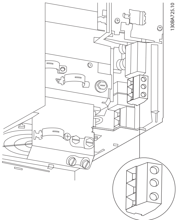
Abbildung 9.24 Netzanschluss Baugröße B3
