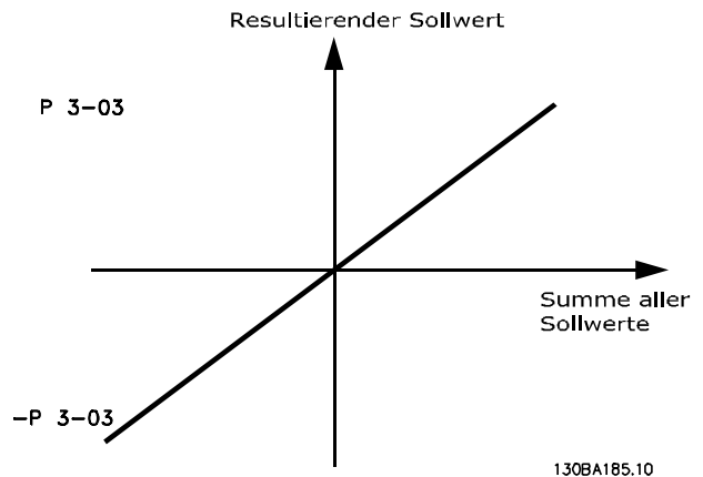
Abbildung 3.15 Resultierender Sollwert
