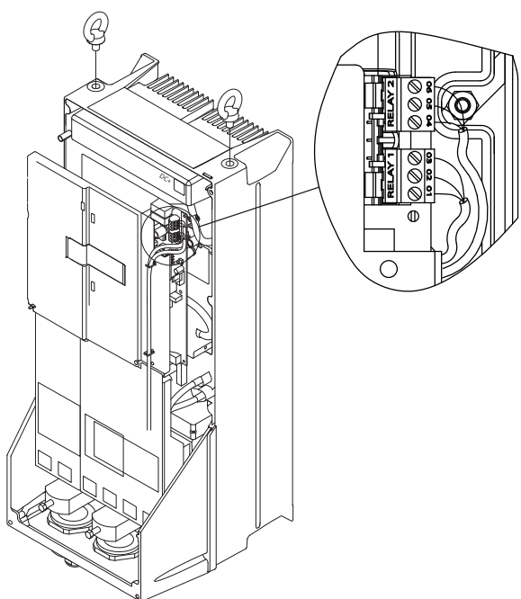
Abbildung 9.43 Klemmen für Relaisanschluss (Baugrößen C1 und C2).
