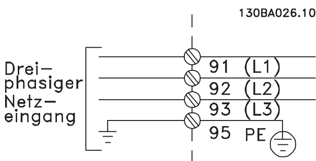
Abbildung 9.16 Netzanschluss
