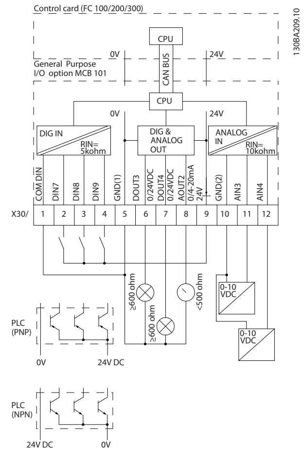
Abbildung 11.2 Prinzipschema
