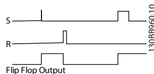
图 3.51 正反器输出
