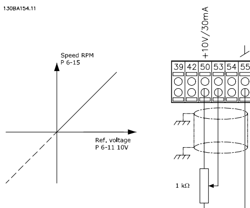
图 1.9 电位计参考值
