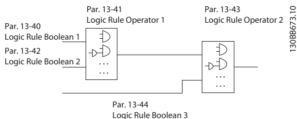
图 3.52 逻辑规则
