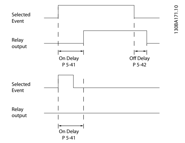
图 3.35 继电器打开延时
