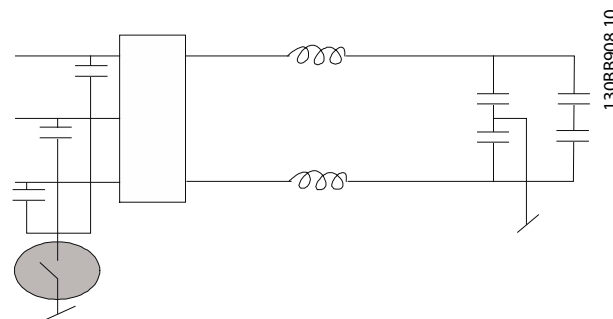
图 3.59 射频干扰滤波器
