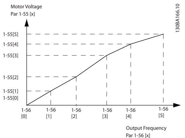
图 3.10 U/f 特性
