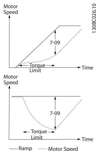
图 3.46 加减速和实际速度之间的速度误差
