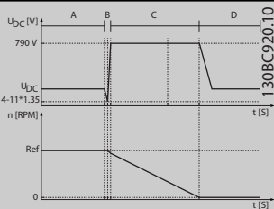
图 3.54 借能运行跳闸
