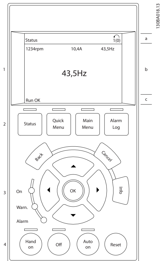
图 2.1 控制面板 (LCP)
