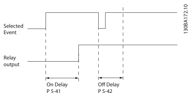
图 3.36 继电器关闭延迟
