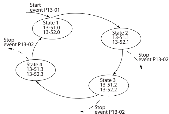
图 3.48 事件和操作
