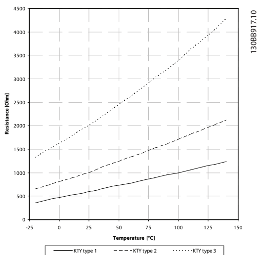
图 3.15 KTY 类型选择
