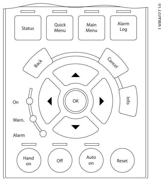
图 2.9 LCP
