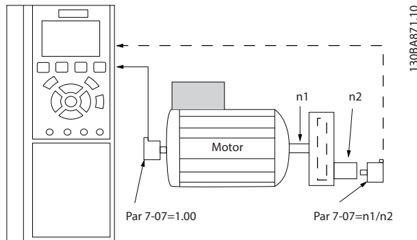
图 3.45 速度 PID 反馈传动比
