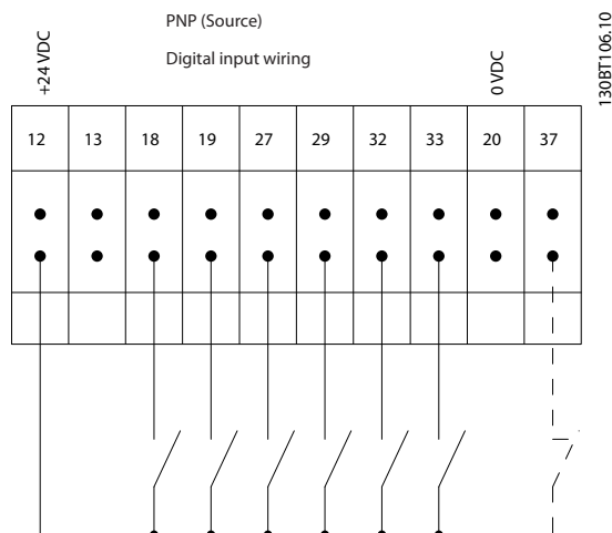
图 1.3 PNP (源型)
