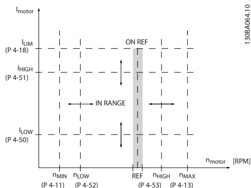
图 3.32 可调整警告
