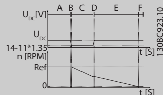
图 3.56 [7] 借能运行, 跳闸并恢复, 跳闸慢斜坡, 当主电源以低于参数 14-15 Kin. Backup Trip Recovery Level 的速度恢复时。在此图中采用了慢斜坡。
