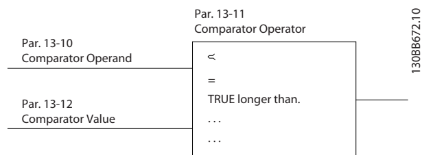
图 3.49 比较器
