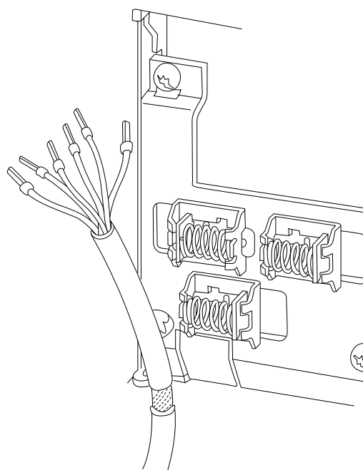
图 1.5 屏蔽/铠装控制电缆的接地
