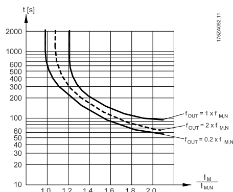
图 3.16 ETR 协议
