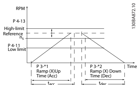
图 3.25 线性加减速时间
