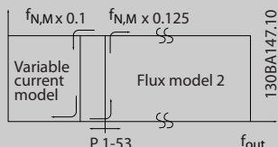
图 3.9 参数 1-00 配置模式 = [0] 开环速度, 参数 1-01 电动控制原理 = [2] 无传感器矢量
