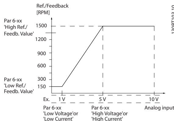
图 3.41 模拟输入 1
