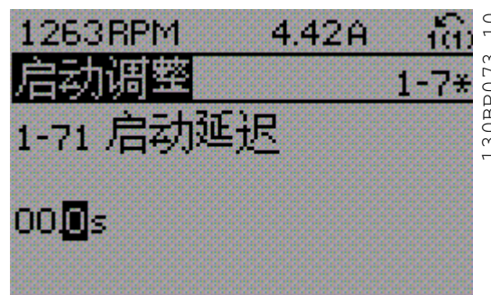
图 2.19 选择数字
