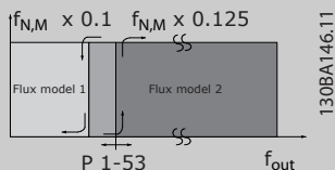
图 3.8 参数 1-00 配置模式 = [1] 闭环速度或 [2] 转矩和 参数 1-01 电动控制原理 = [3] 磁通矢量带电动机反馈
