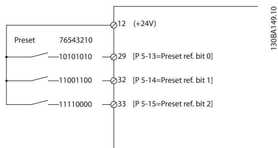
图 3.21 预置参考值
