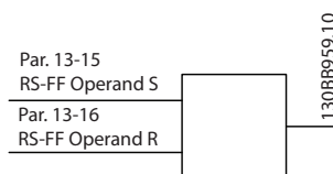
图 3.50 复位/设置触发器
