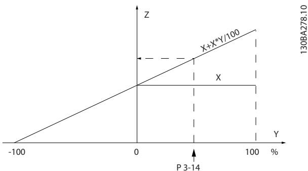
图 3.23 实际参考值
