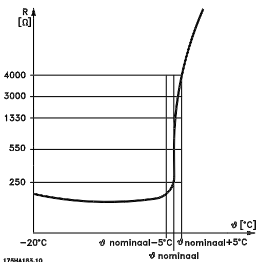
图 3.12 PTC 协议
