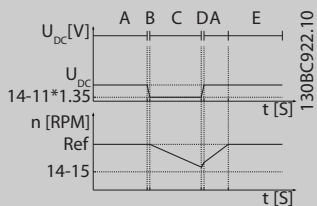
图 3.55 [7] 借能运行, 并在主电源恢复到超过参数 14-15 Kin. Backup Trip Recovery Level 时, 跳闸并恢复。
