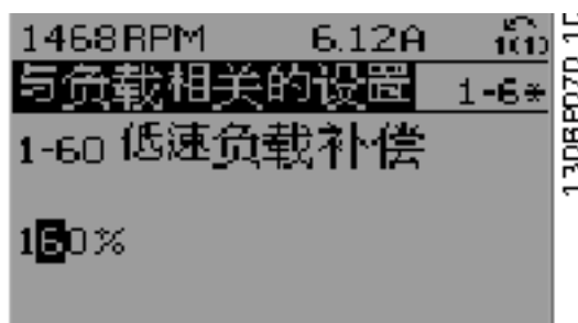
图 2.18 保存数据值
