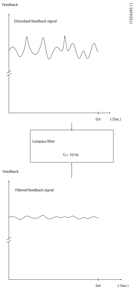
图 3.44 反馈信号
