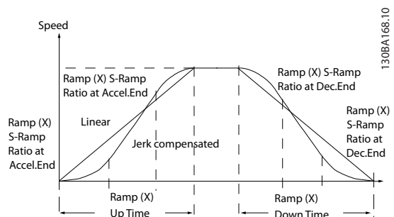
图 3.26 线性加减速时间
