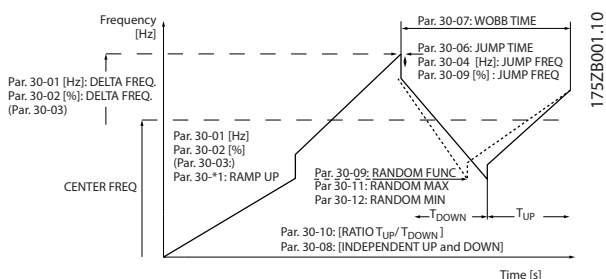
图 3.63 摆频功能
