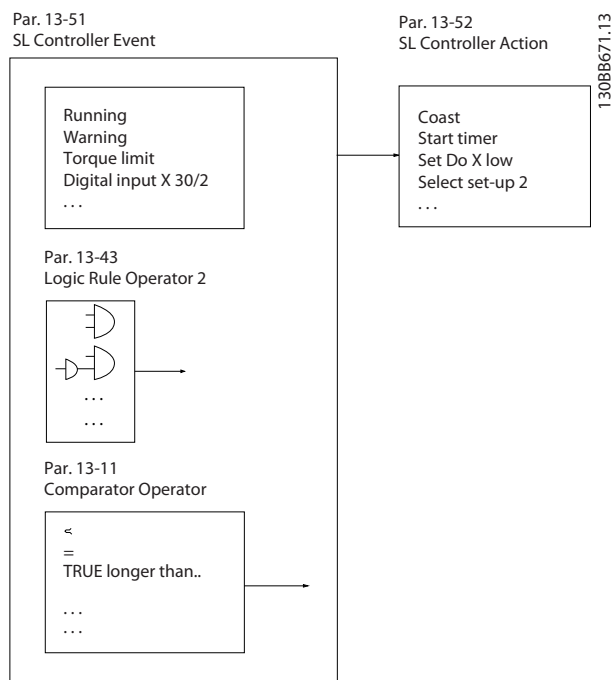
图 3.47 智能逻辑控制 (SLC)
