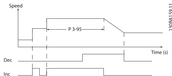
图 3.30 增加/减小实际参考值
