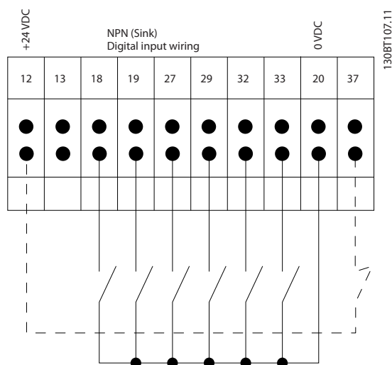
图 1.4 NPN (漏型)
