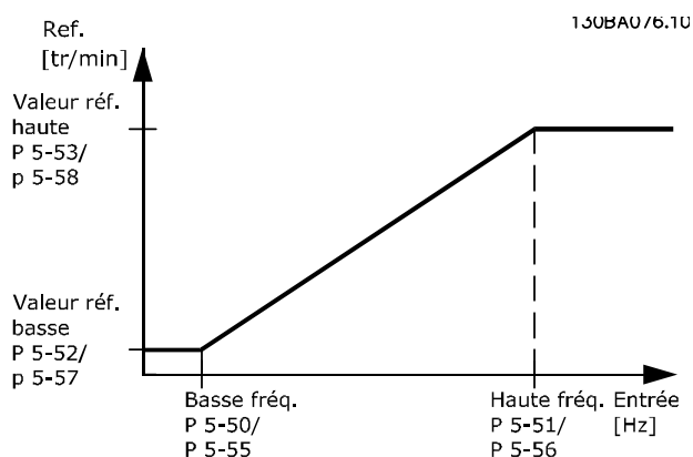
Illustration 3.37 Entrée impulsions
