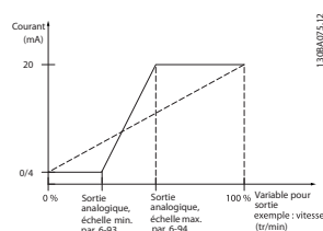
Illustration 3.43 Échelle max. sortie
