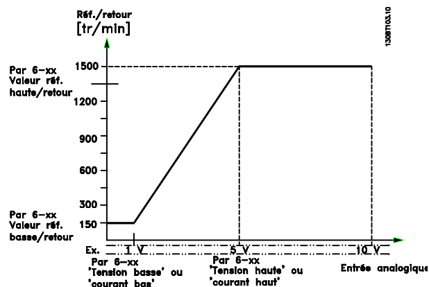
Illustration 3.41 Entrée ANA 1
