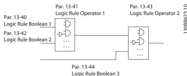
Illustration 3.53 Règles de Logique
