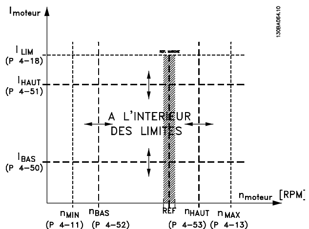
Illustration 3.32 Avertissements réglables
