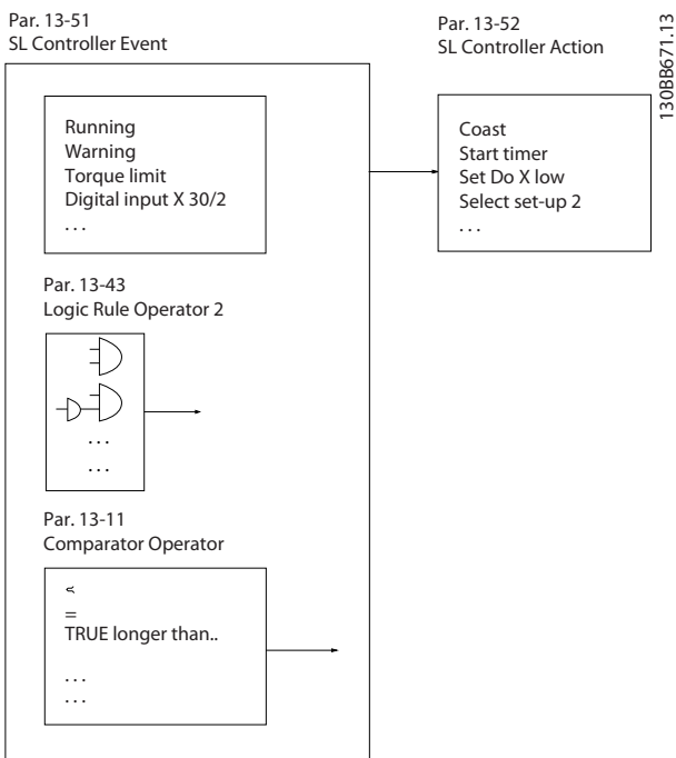
Illustration 3.48 Contrôleur logique avancé (SLC)
