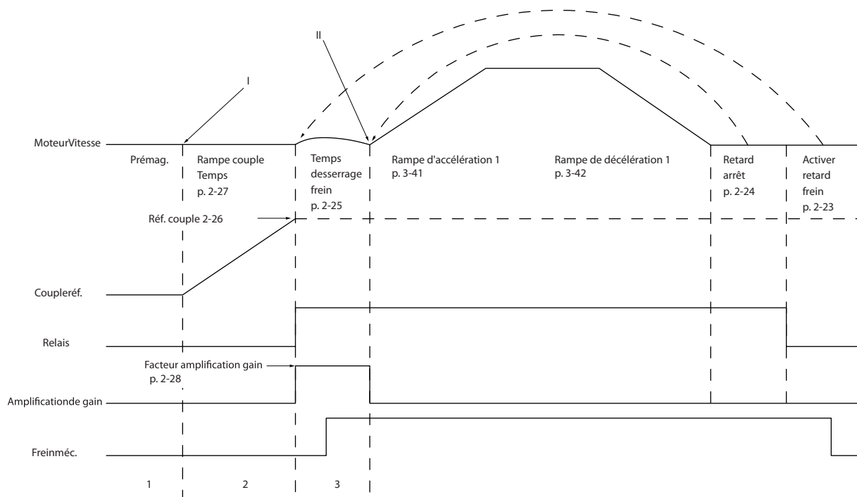
Illustration 3.20 Séquence de déclenchement du frein pour la commande de frein mécanique pour levage. Cette commande de frein est disponible en FLUX avec signal de retour du moteur uniquement, pour les moteurs PM non saillants et asynchrones.
