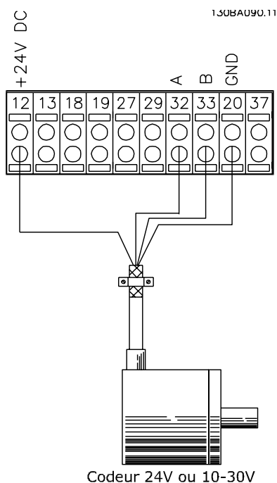
Illustration 3.39 Raccordement du codeur
