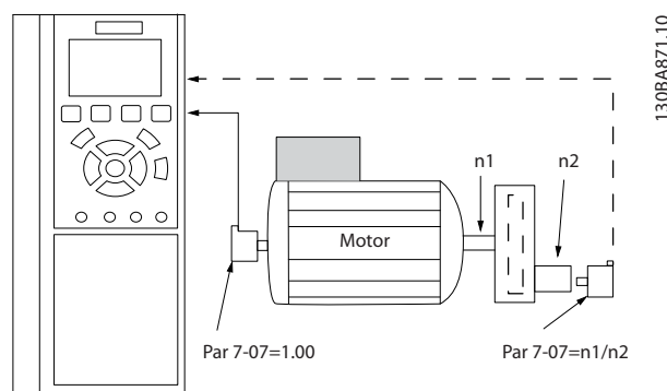
Illustration 3.46 Rapport démultipl. ret.PID vit.
