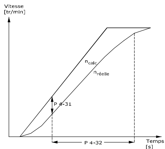
Illustration 3.31 Erreur vitesse signal de retour moteur
