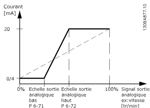
Illustration 3.44 Échelle max. sortie
