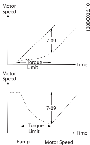
Illustration 3.47 Erreur de vitesse entre la rampe et la vitesse réelle
