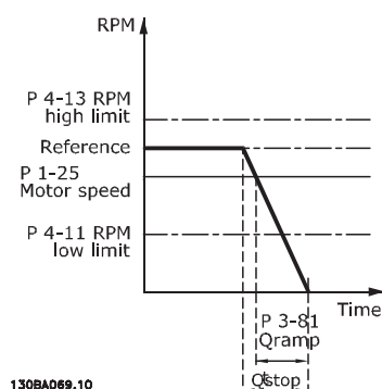
Illustration 3.28 Temps rampe arrêt rapide
