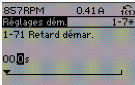
Illustration 2.19 Sélectionner un chiffre
