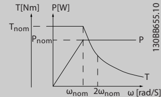
Illustration 3.5 Puissance constante
