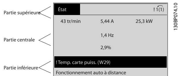
Illustration 2.2 Écran LCD
