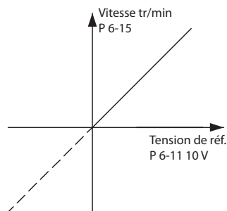
Illustration 1.9 Référence potentiomètre
