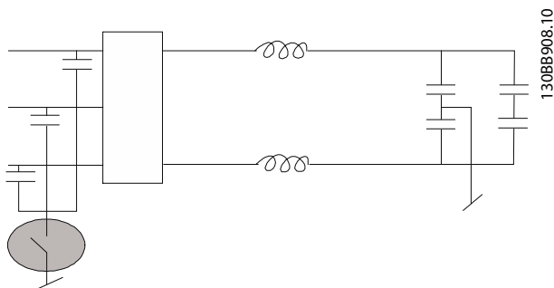
Illustration 3.60 Filtre RFI
