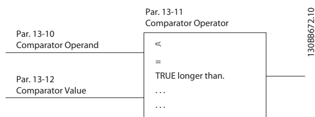
Illustration 3.50 Comparateurs
