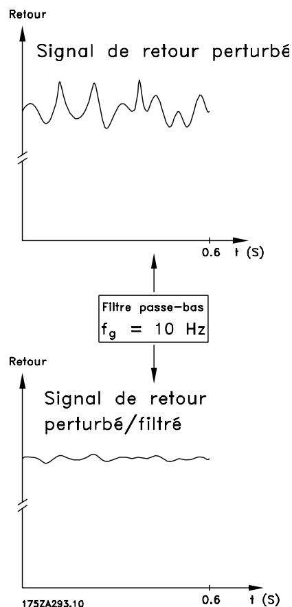
Illustration 3.45 Signal de retour
