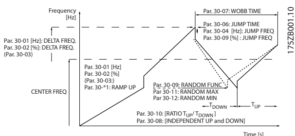
Illustration 3.64 Fonction de modulation (wobble)
