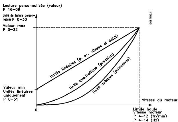
Illustration 3.4 Lect.paramétri.
