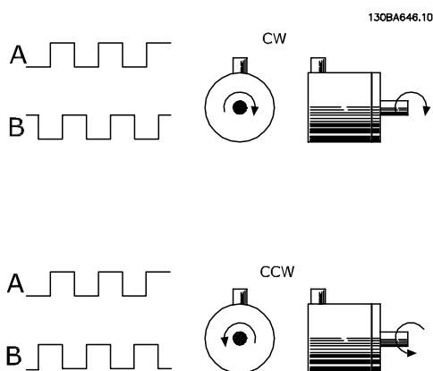
Illustration 3.40 Sens de rotation du codeur
