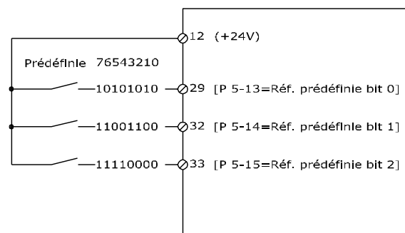
Illustration 3.21 Réf.prédéfinie
