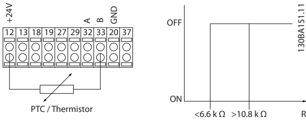
Рисунок 3.19 Подключение термистора
