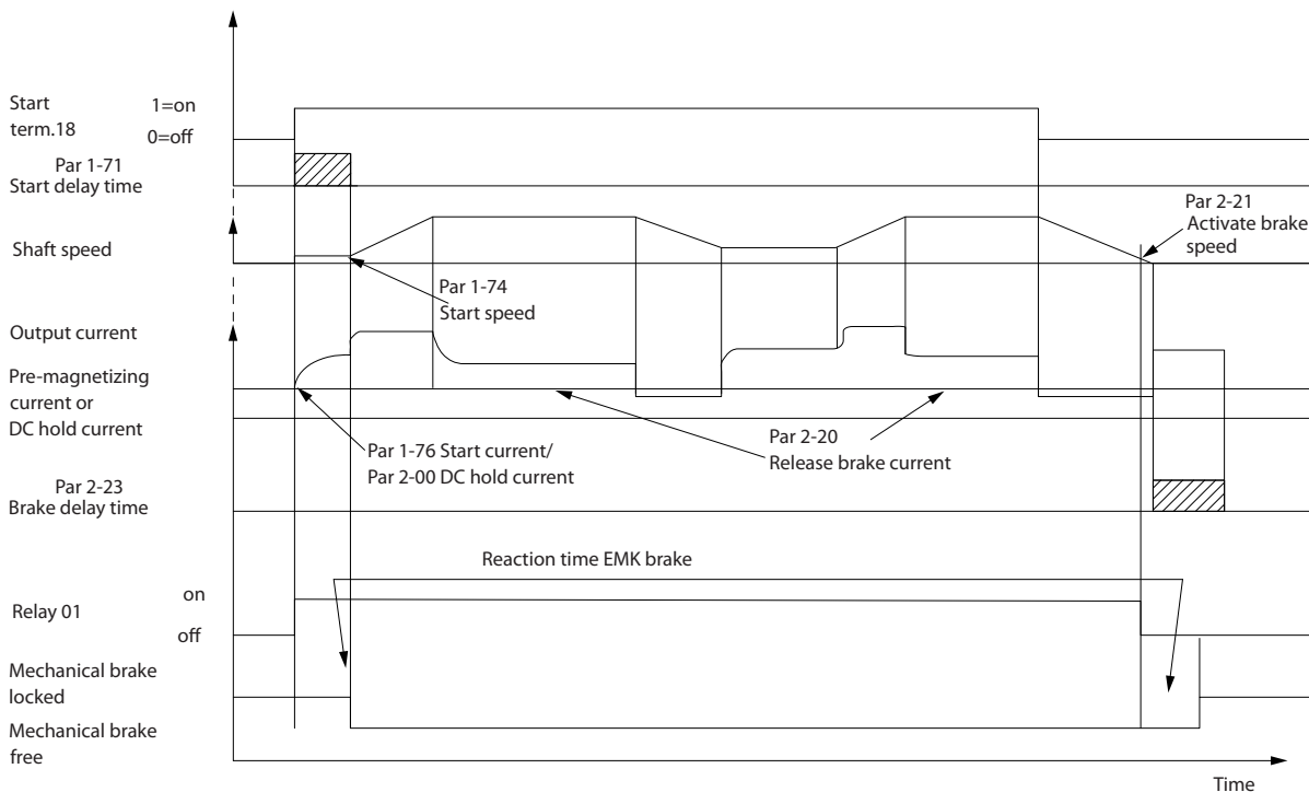
Рисунок 3.21 Механическое торможение
