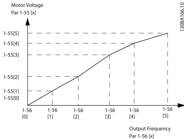
Рисунок 3.12 Характеристика U/f
