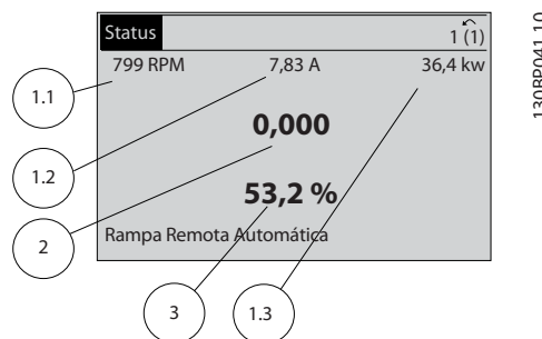
Ilustração 2.10 Visualização do status I
