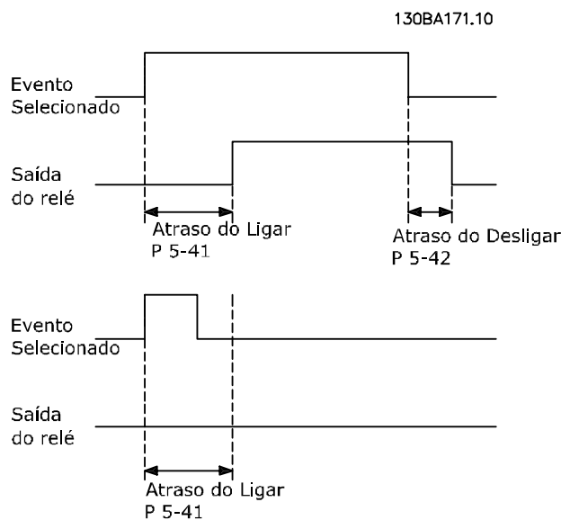
Ilustração 3.36 Atraso de Ativação do Relé
