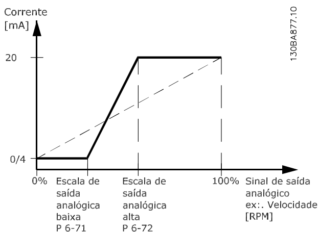
Ilustração 3.45 Escala máxima de saída
