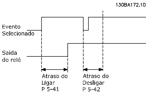
Ilustração 3.37 Atraso de desligamento, relé
