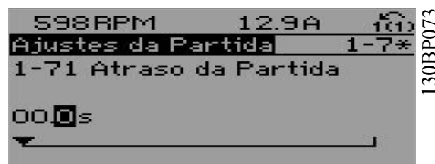
Ilustração 2.19 Selecionando um dígito
