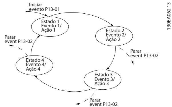
Ilustração 3.52 Eventos e Ações
