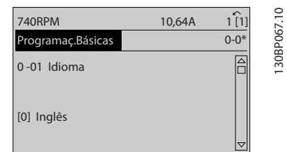
Ilustração 2.15 Seleção de Parâmetro
