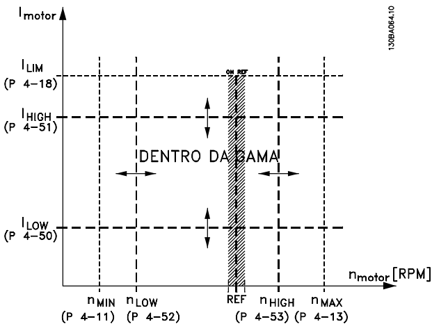
Ilustração 3.33 Advertências Ajustáveis
