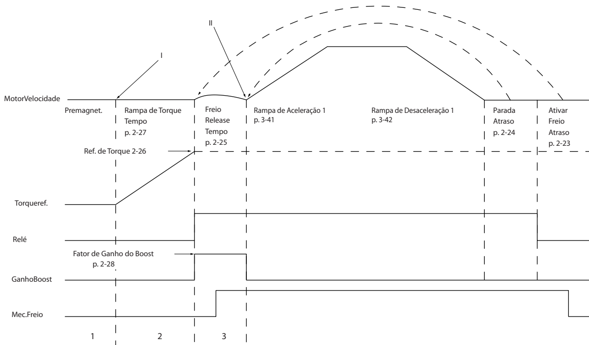
Ilustração 3.20 Sequência de Liberação do Freio para Controle do Freio Mecânico de Içamento
