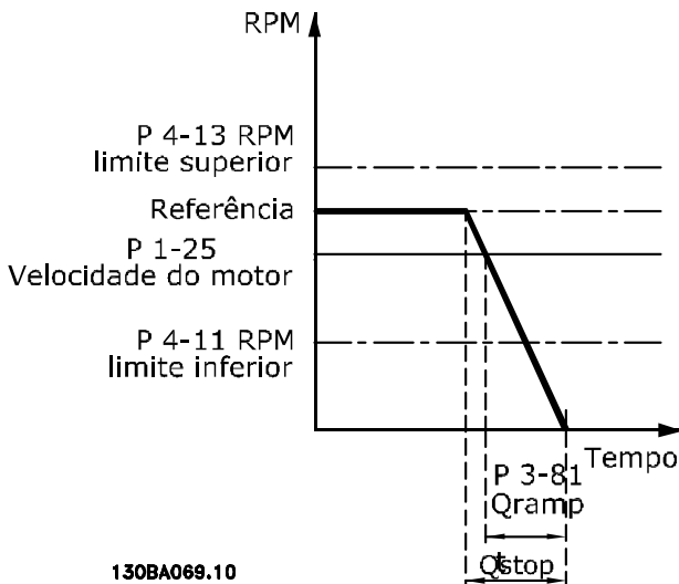
Ilustração 3.28 Tempo de Rampa da Parada Rápida
