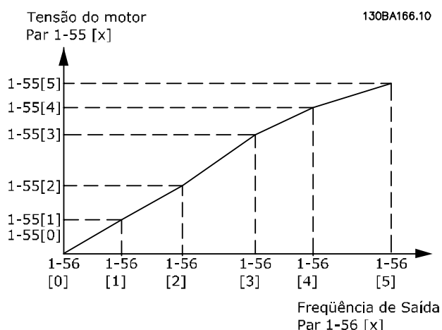
Ilustração 3.10 Característica U/f
