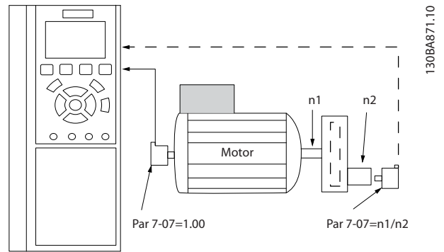
Ilustração 3.49 Relação de Engrenagem do Feedback do PID de Velocidade
