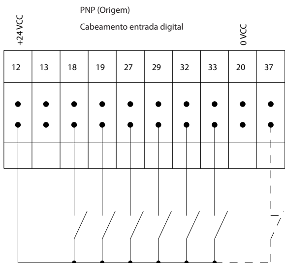
Ilustração 1.3 PNP (Origem)
