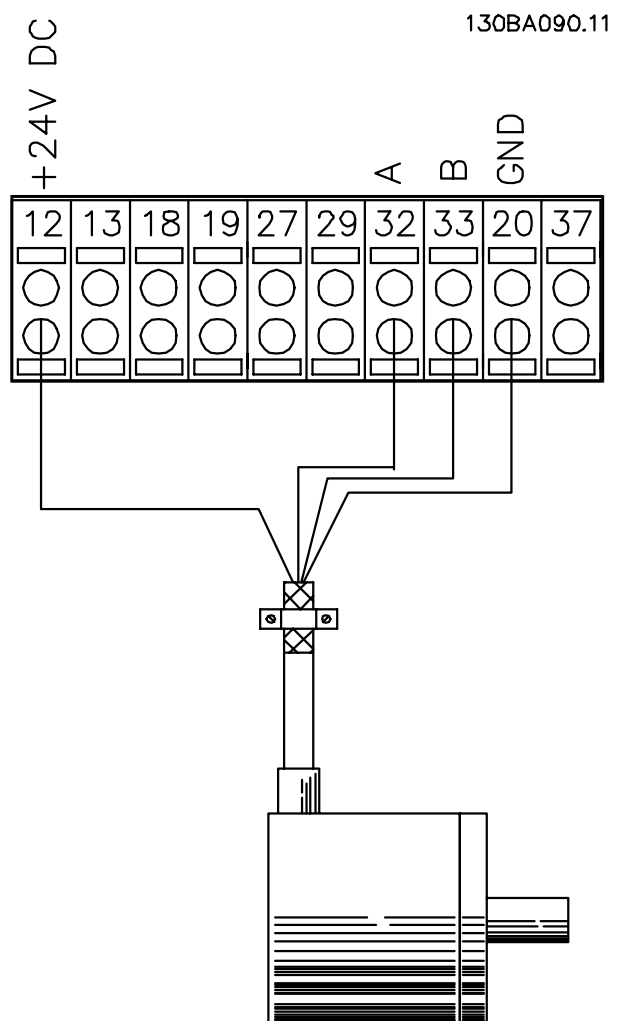
Codificador de 24V ou 10-30V Ilustração 3.40 Conexão do Encoder
