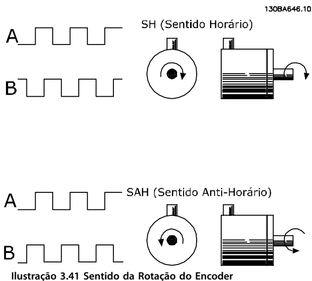
Ilustração 3.41 Sentido da Rotação do Encoder
