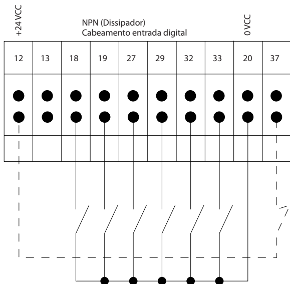
Ilustração 1.4 NPN (Dissipador)
