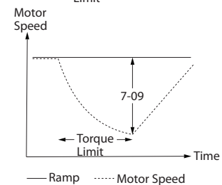
Ilustração 3.50 Erro de Velocidade entre Rampa e Velocidade Real
