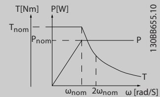
Ilustração 3.5 Potência Constante
