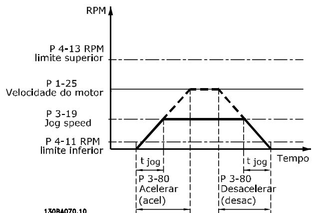
130BA070.10 Ilustração 3.27 Tempo de Rampa do Jog
