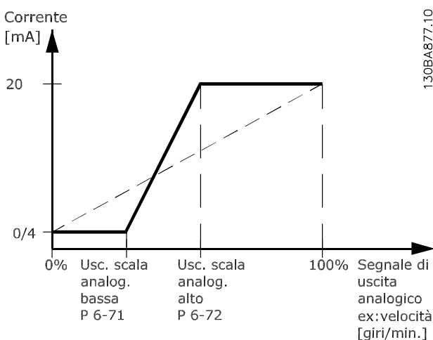
Disegno 3.45 Uscita a scala massima
