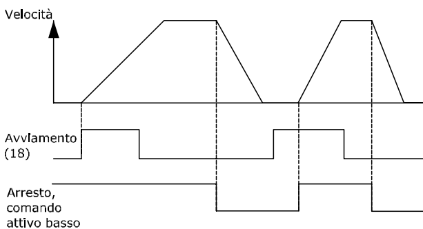
Disegno 1.7 Avviamento/arresto a impulsi
