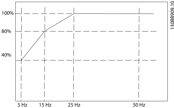
Disegno 3.18 Esempio di curva del limite termico ETR ATEX.
