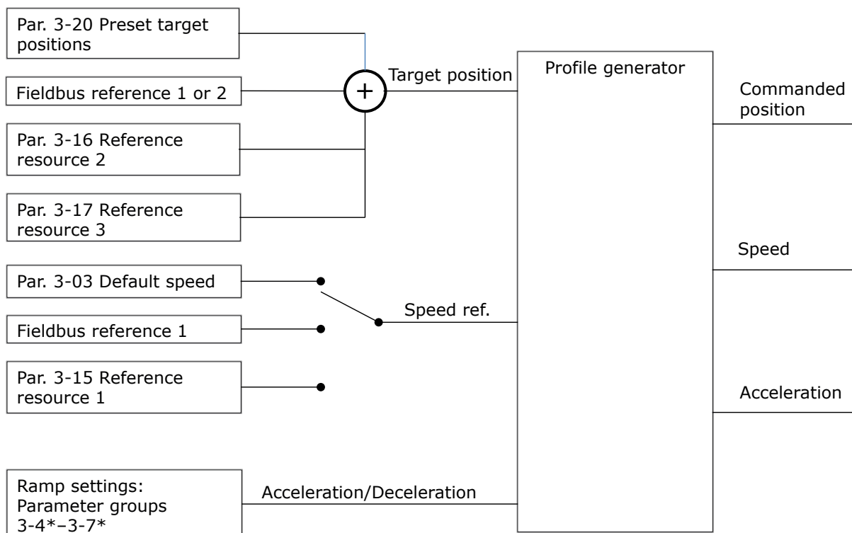
Disegno 4.1 Riferimenti di posizionamento
