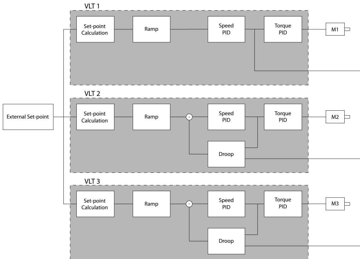
Disegno 3.47 Variazione della velocità
