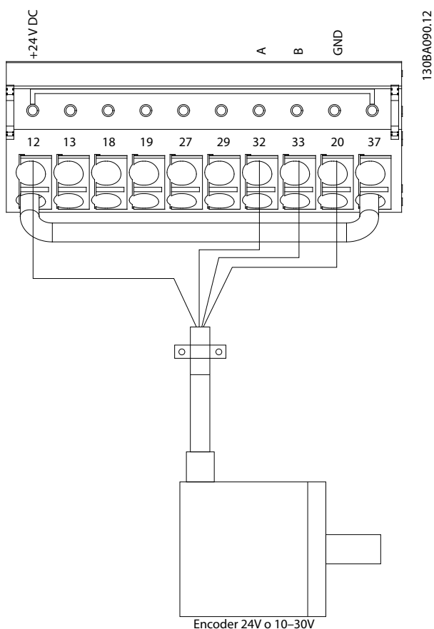
Disegno 3.40 Collegamento encoder
