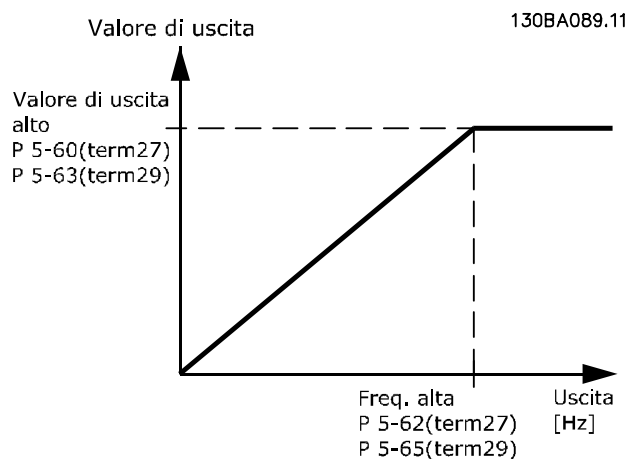
Disegno 3.39 Configurazione delle uscite a impulsi
