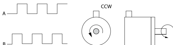
Disegno 3.41 Senso di rotazione dell'encoder
