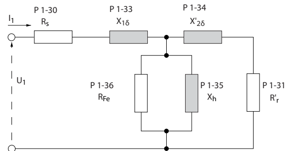
Disegno 3.6 Grafico equivalente per un motore asincrono
