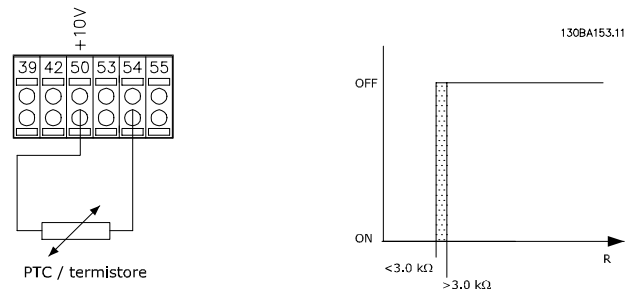
Disegno 3.14 Collegamento termistore PTC - ingresso analogico
