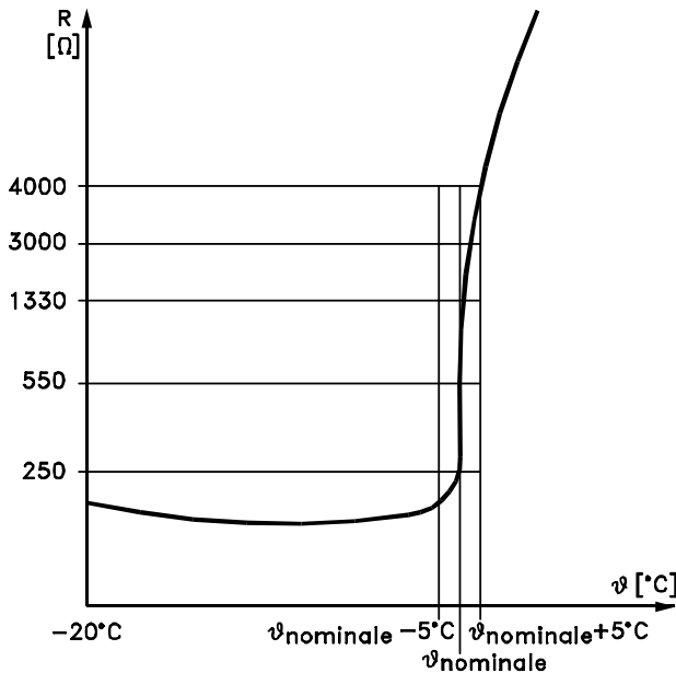
175HA183.10 Disegno 3.12 Profilo PTC
