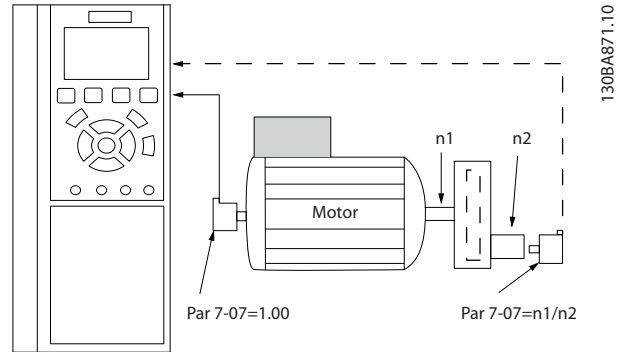
Disegno 3.49 Retroaz. vel. PID Rapp. transmiss.
