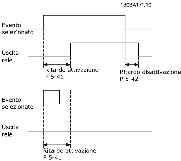
Disegno 3.36 Ritardo attiv., relè
