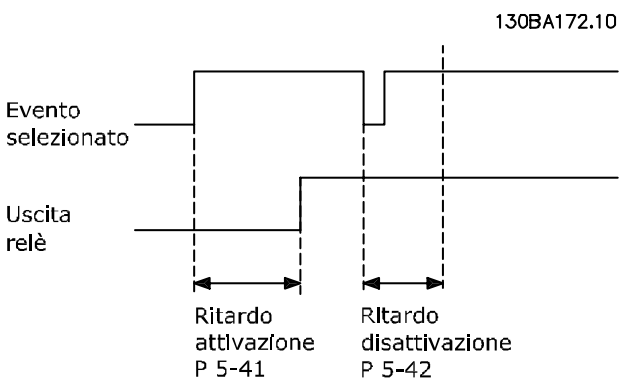
Disegno 3.37 Ritardo disatt., relè
