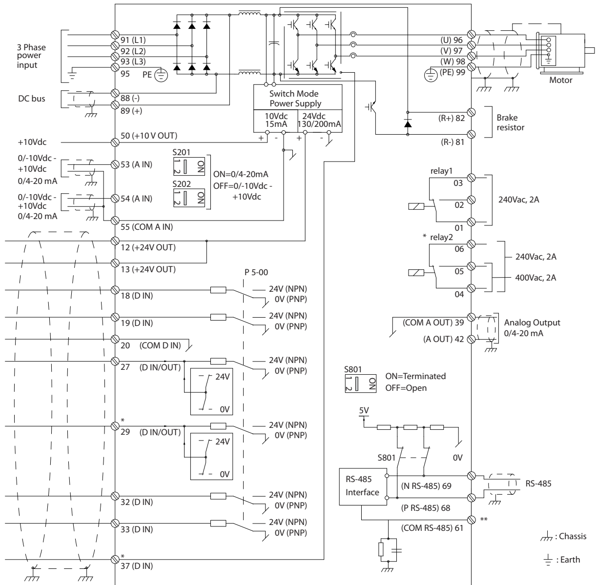
Disegno 1.2 Schema di cablaggio base
