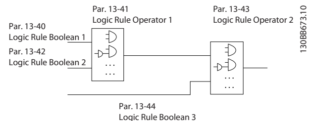
Disegno 3.56 Regole logiche
