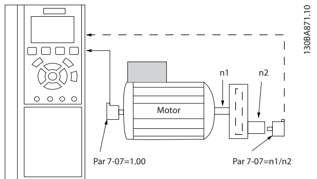
图 3.50 速度 PID 反馈传动比
