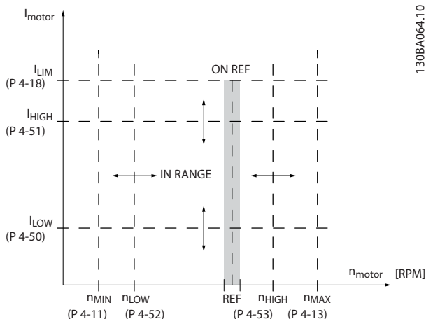
图 3.33 可调整警告
