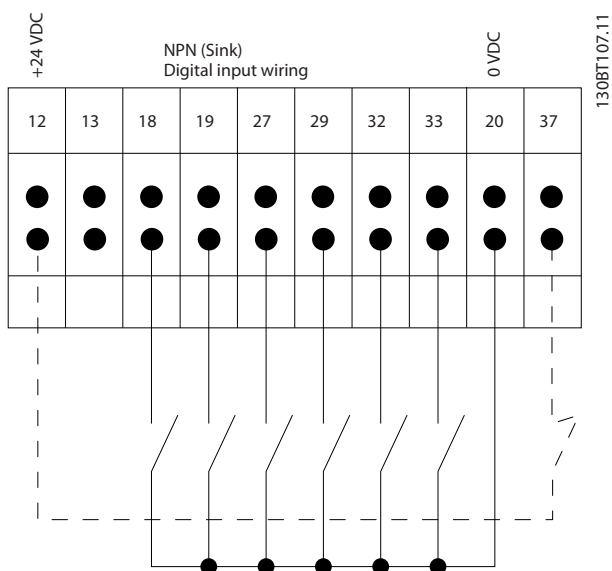
图 1.4 NPN (漏型)
