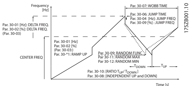
图 3.72 摆频功能
