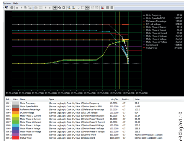
图 3.66 服务日志视图, 5 s
