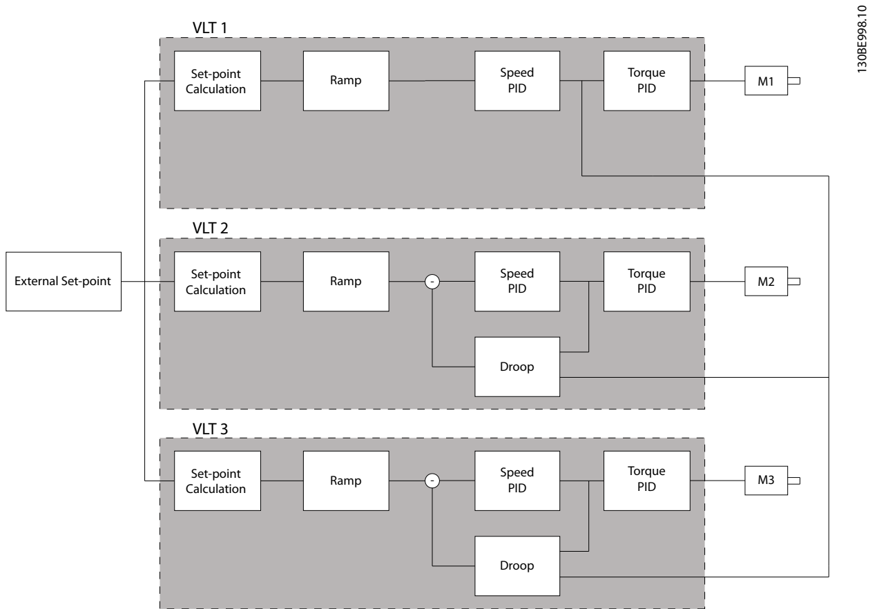
图 3.48 速度调整
