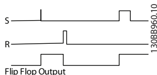
图 3.56 正反器输出
