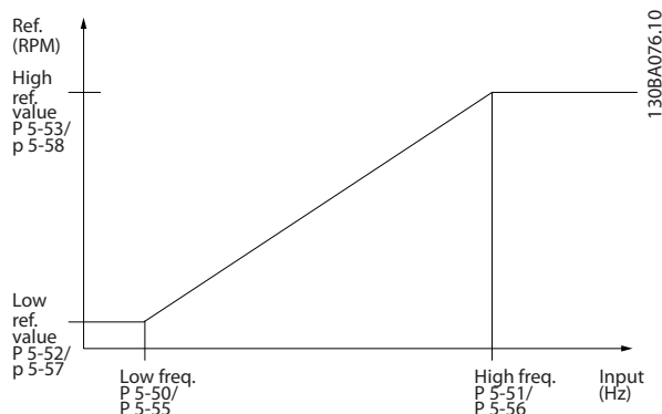
图 3.39 脉冲输入
