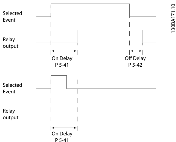
图 3.37 继电器打开延时
