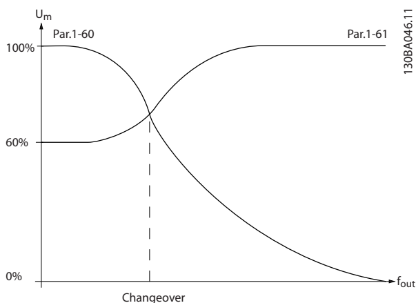
图 3.11 切换
