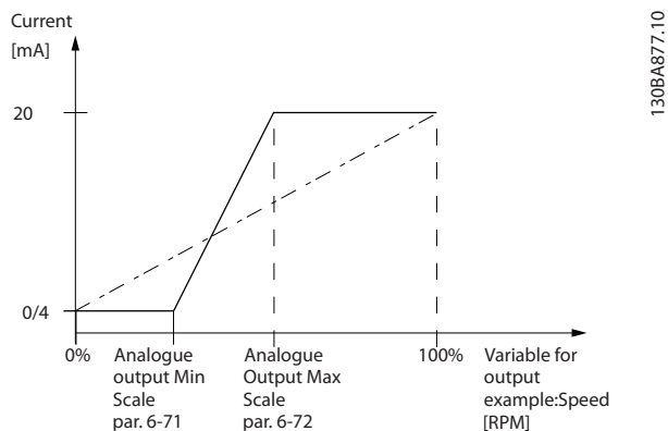
图 3.46 输出最大标定
