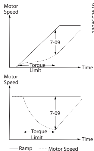
图 3.51 加减速和实际速度之间的速度误差
