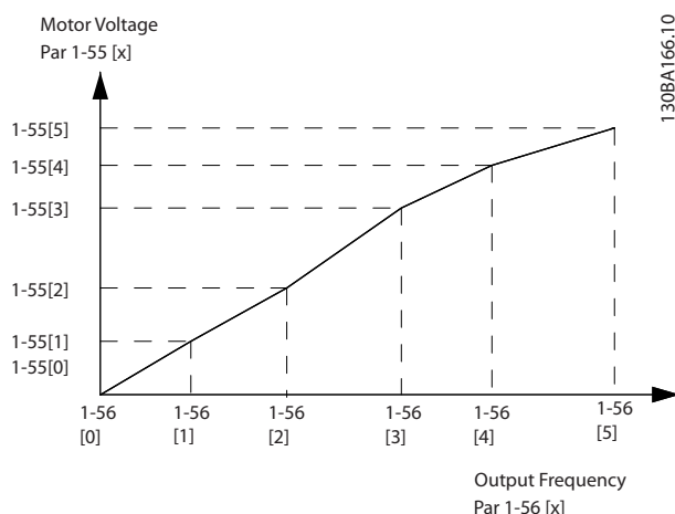
图 3.10 U/f 特性
