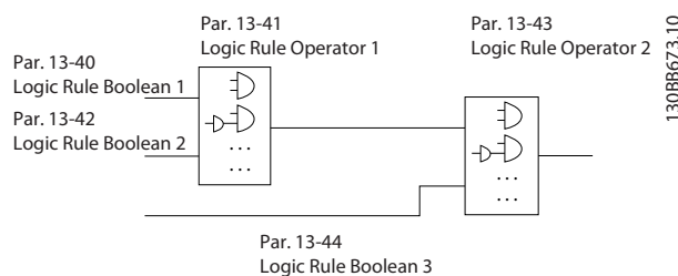
图 3. 57 逻辑规则
