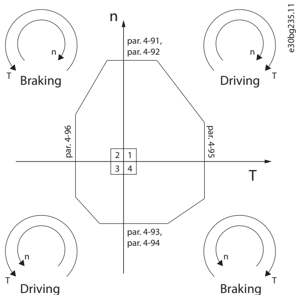
图 3.34 方向极限
