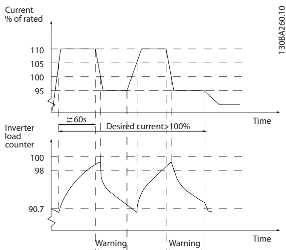
图 3.64 过载条件下的输出电流
