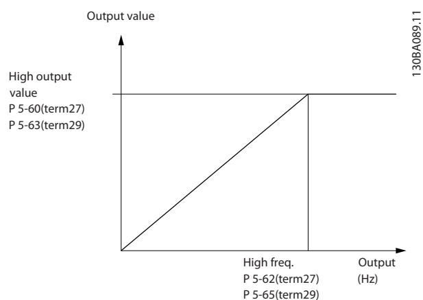
图 3.40 脉冲输出的配置
