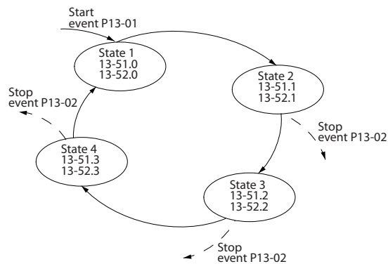
图 3.53 事件和操作
