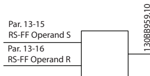
图 3.55 复位/设置触发器
