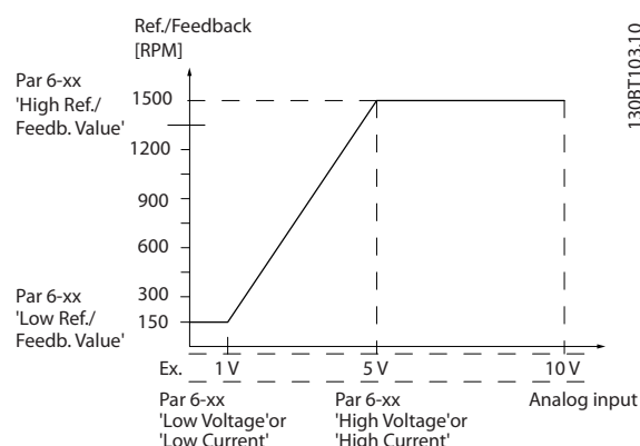
图 3.43 模拟输入 1
