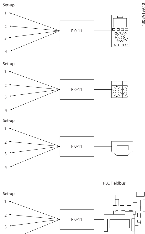
图 3.1 编辑菜单
