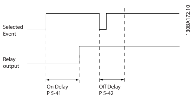
图 3.38 继电器关闭延迟
