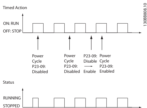
图 3.70 重新激活测试图
