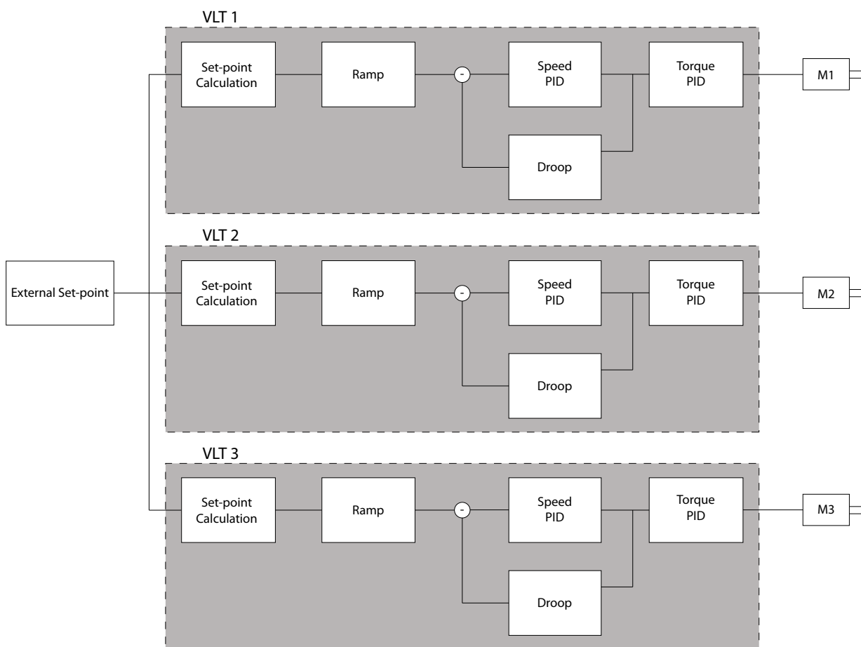
图 3.47 速度 PID 不等率
