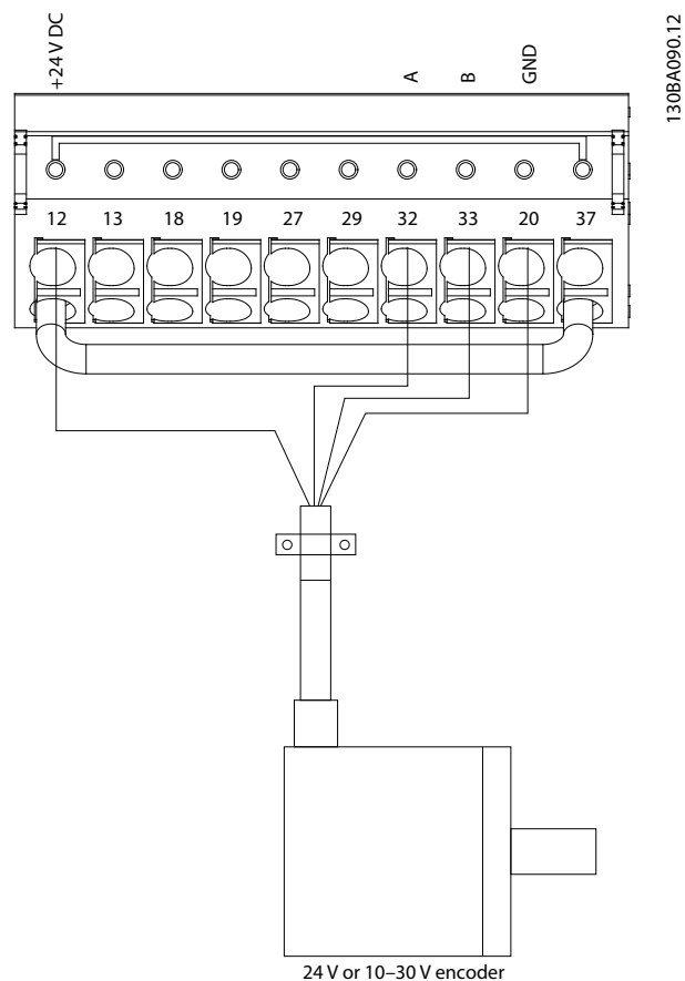
图 3.41 编码器连接
