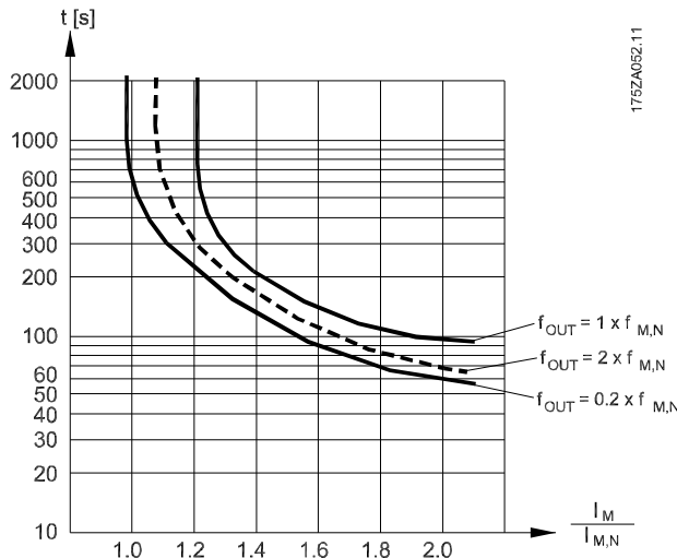
图 3.16 ETR 协议
