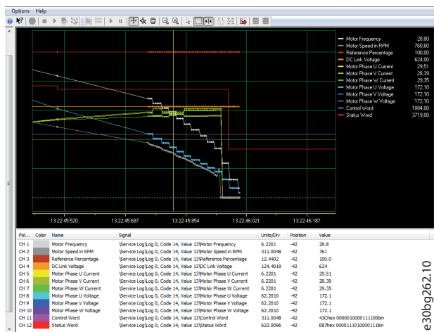
图 3.67 服务日志详细视图, 250 ms
