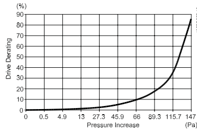
Ilustración 3.27: Bastidor D reducción de potencia vs. cambio de presión Caudal de aire del convertidor: 450 cfm (765 m3/h)
