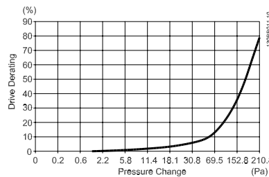
Ilustración 3.29: Bastidor E reducción de potencia vs. cambio de presión (ventilador grande), P315T5-P400T5 y P500T7-P560T7 Caudal de aire del convertidor: 850 cfm (1445 m3/h)
