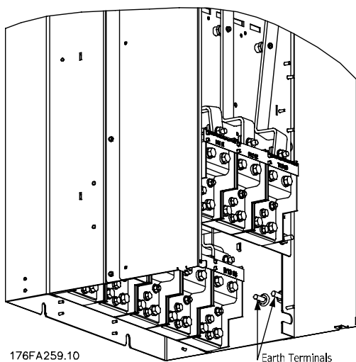
Ilustración 3.46: Posición de terminales de conexión a tierra IP00, tamaños de bastidor E
