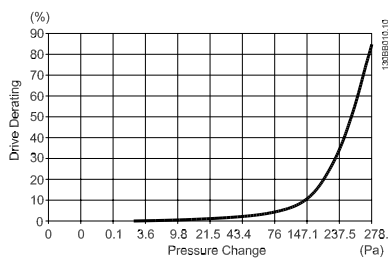
Ilustración 3.28: Bastidor E reducción de potencia vs. cambio de presión (ventilador pequeño), P250T5 y P355T7-P400T7 Caudal de aire del convertidor: 650 cfm (1105 m3/h)
