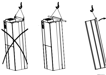
Ilustración 3.2: Método de elevación recomendado, tamaños de bastidor D y E .
