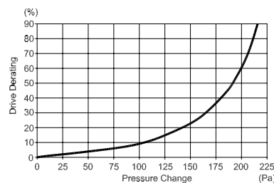
Ilustración 3.30: Bastidor F1, F2, F3, F4 reducción de potencia vs. cambio de presión Caudal de aire del convertidor: 580 cfm (985 m3/h)
