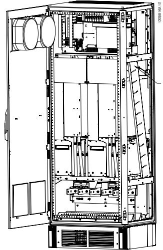
Ohjaukorkin johdotusreitti mallille F1/F3. Ohjaukorkin johdotus malleille F2/F4 käytetään samaa reittiä.
