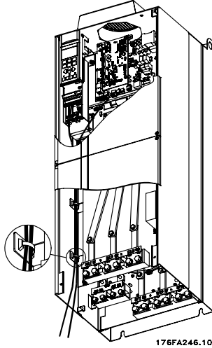
Ohjaukorkin johdotusreitti mallille D3. Ohjaukorkin johdotus malleille D1, D2, malleissa D4, E1 ja E2 käytetään samaa reittiä.
