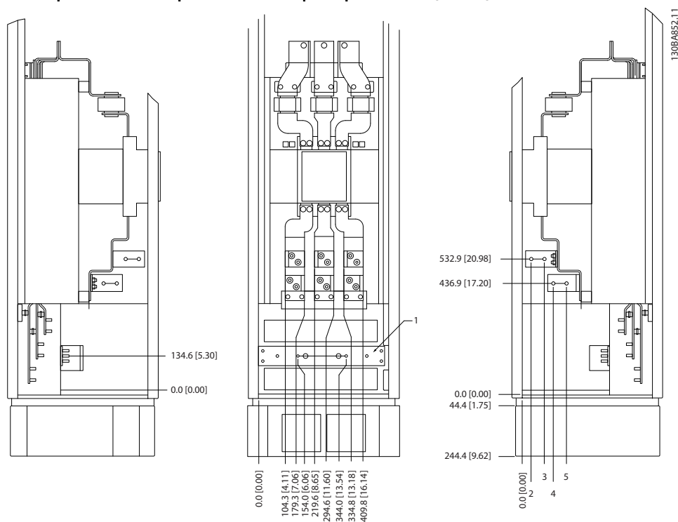
Slika 3.27 Lokacija priključaka - opcioni orman sa prekidačem/ uklopnim prekidačem (pogled sleva, spreda i zdesna). Ploča ulodnika je 42 mm ispod .0 nivoa.
