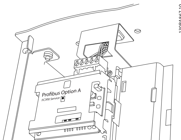
Slika 3.65 Gornji priključak komunikacionog protokola.
