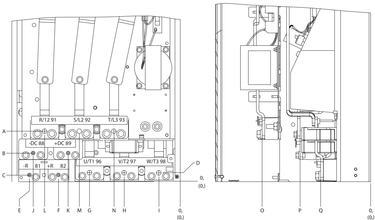
Slika 3.12 Položaj priključaka mrežnog napajanja, veličine kućišta D3 i D4
