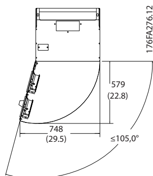
Slika 3.7 Prostor ispred kućišta tipa IP21/IP54, veličina kućišta E1.
