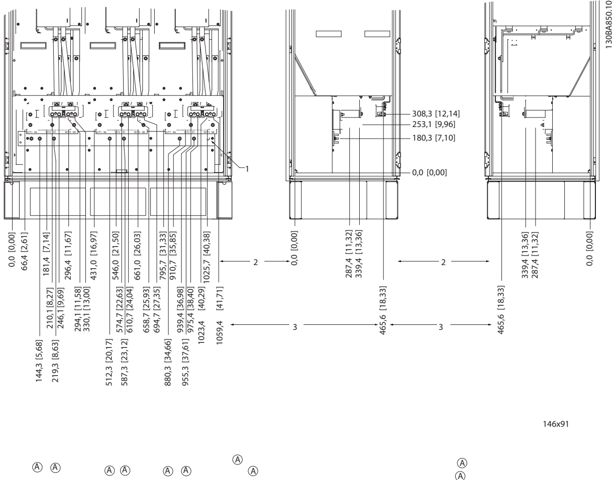
Slika 3.23 Lokacija priključaka - orman invertora - F2 i F4 (pogled sprede, sleva i zdesna). Ploča uvodnika je 42 mm ispod .0 nivoa.
