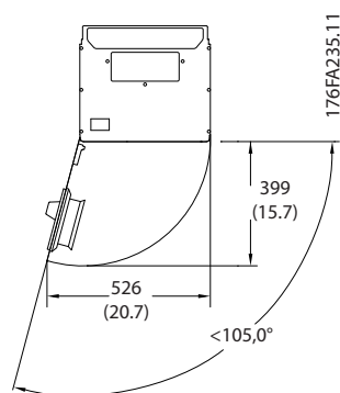
Slika 3.6 Prostor ispred kućišta tipa IP21/IP54, veličina kućišta D1 i D2 .
