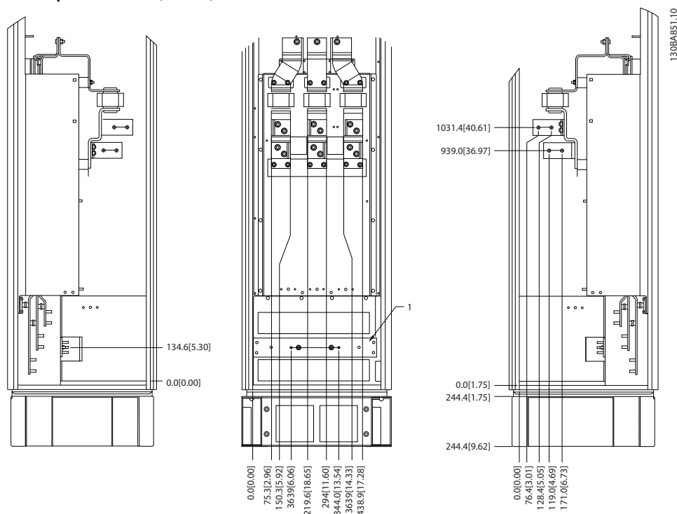
Slika 3.26 Lokacija priključaka - opcioni orman (pogled sleva, spreda i zdesna). Ploča ulodnika je 42 mm ispod .0 nivoa.
