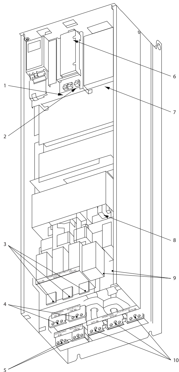
Slika 3.50 Kompakt IP 00 (kućište) sa rastavljačem, osiguračem i RFI filterom, veličina kućišta D4
