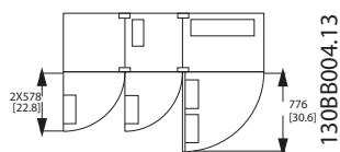
Slika 3.9 Prostor ispred kućišta tipa IP21/IP54, veličina kućišta F3
