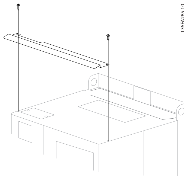
Slika 3.40 Montaža štitnika protiv okapljivanja.
