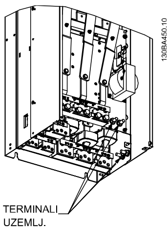
Slika 3.51 Položaj priključaka uzemljenja IP00, veličina kućišta D
