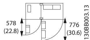
Slika 3.8 Prostor ispred tipa kućišta IP21/IP54, veličina kućišta F1
