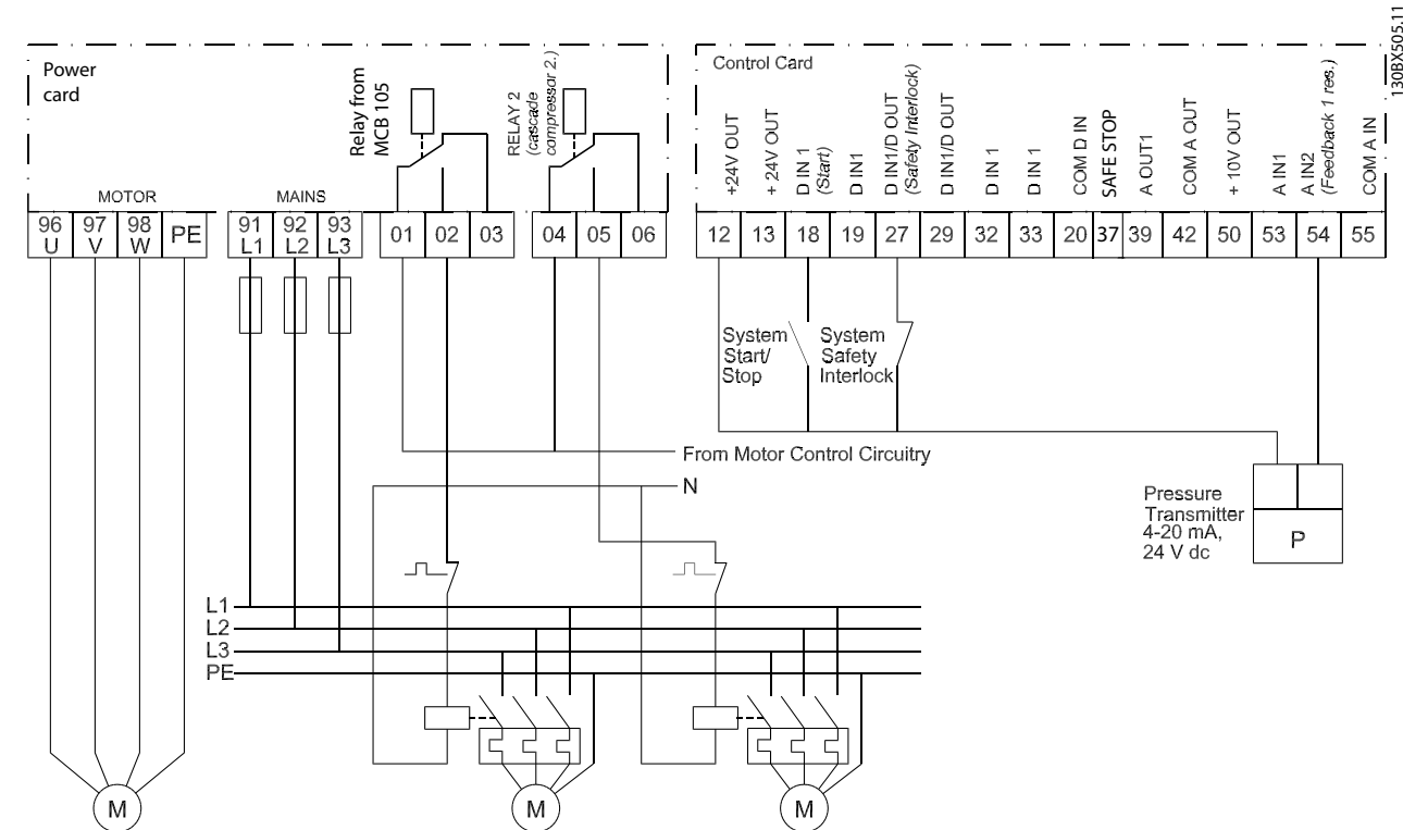
图 3.32 内置 BASIC 多泵控制器示例
