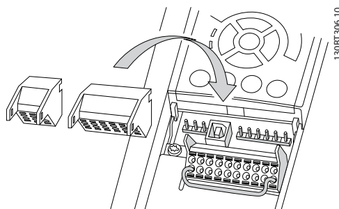
图 3.22 安装端子
