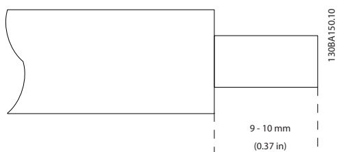
图 3.21 剥除电缆皮
