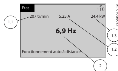
Illustration 5.3 Écran d'état II - Variables d'exploitation
