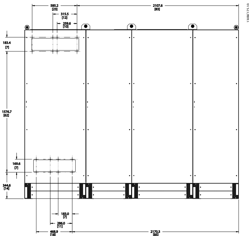
Illustration 4.9 Châssis de taille F18, vue arrière
