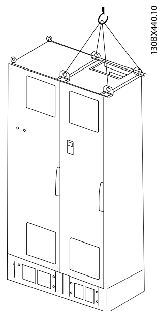
Illustration 4.4 Méthode de levage recommandée, châssis de taille F18 - section du filtre.
