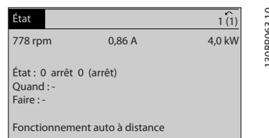
Illustration 5.4 Écran d'état III - Variables d'exploitation
