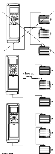
Illustration 4.41 Installations avec câbles connectés en un point commun
