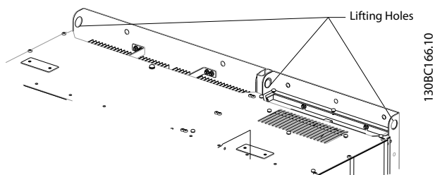
Illustration 4.2 Méthode de levage recommandée, châssis de taille D13
