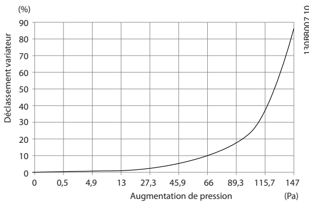
Illustration 4.21 Déclassement du châssis D en fonction du changement de pression Débit d'air du variateur : 450 cfm (765 m 3 /h)
