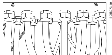
Illustration 4.25 Exemple d'installation correcte de la plaque presse-étoupe.
