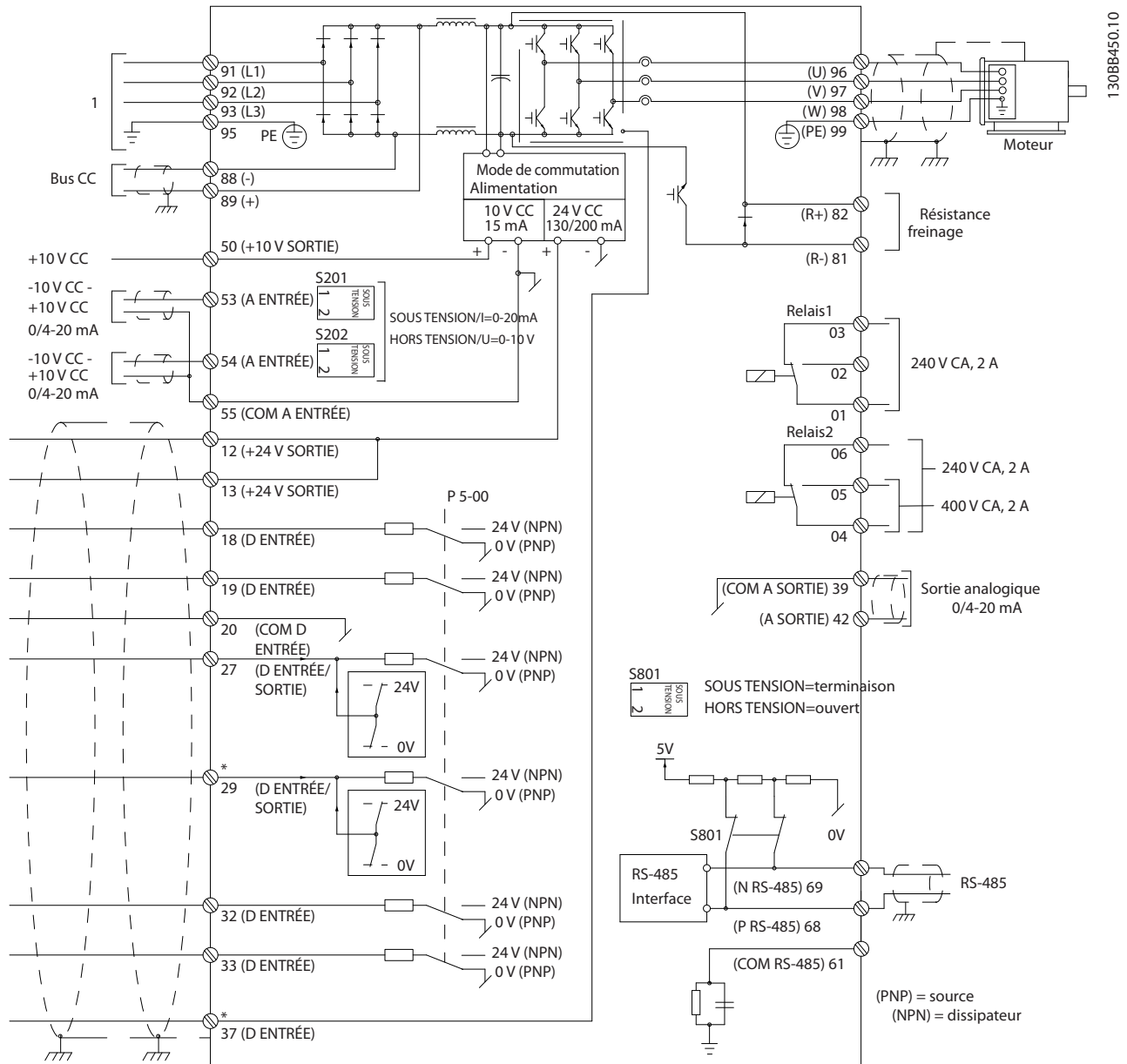
Illustration 4.40 Schéma représentant toutes les bornes sans options.
