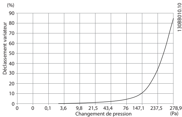
Illustration 4.22 Déclassement du châssis E en fonction du changement de pression (petit ventilateur), P315 Débit d'air du variateur : 1105 m 3 /h (650 cfm)
