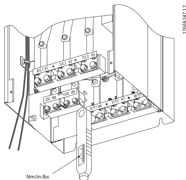
Illustration 4.37 Toujours utiliser une clé dynamométrique pour serrer les boulons.
