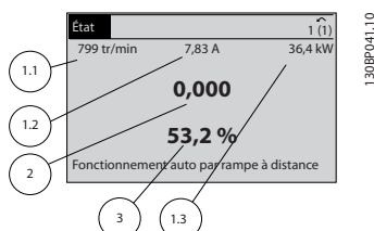
Illustration 5.2 Écran d'état I - Variables d'exploitation
