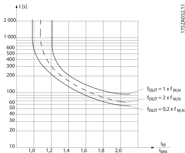
Illustration 6.3 Profil ETR
