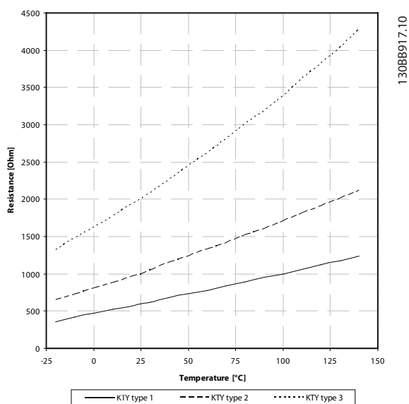
Illustration 6.2 Sélection du type KTY
