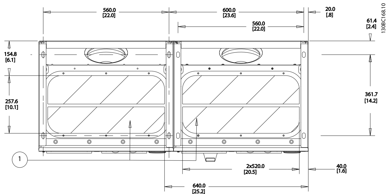
Illustration 4.27 Châssis de taille E9
