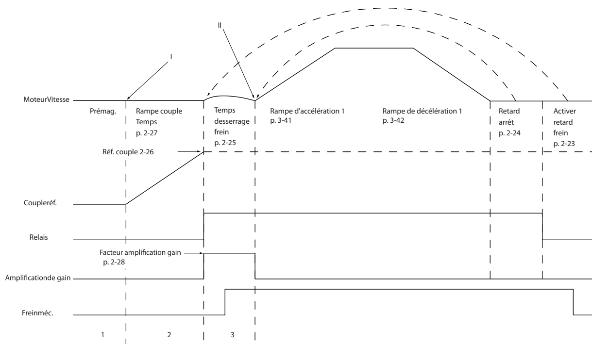
Illustration 6.4 Séquence de déclenchement du frein pour la commande de frein mécanique pour levage
