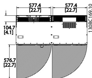
Illustration 4.11 Espace devant le type de protection IP21/IP54, châssis de taille E9.
