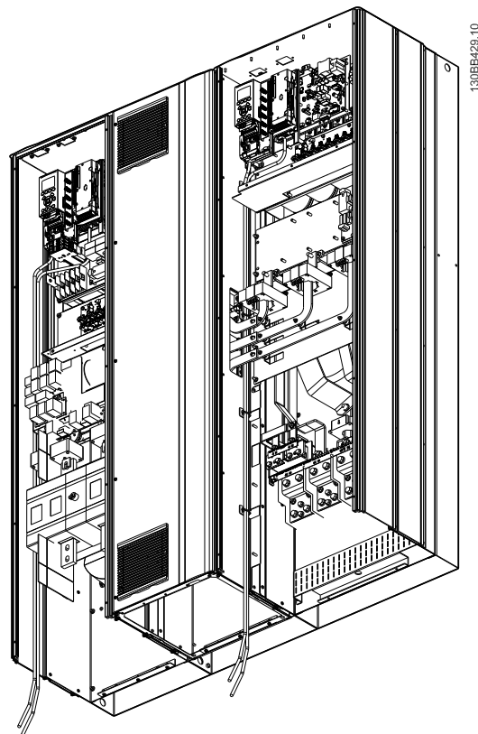
Illustration 4.39 Passage des câbles de la carte de commande pour E9
