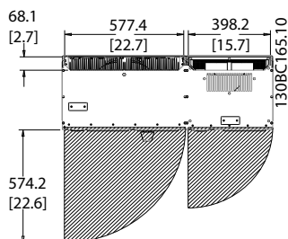
Illustration 4.10 Espace devant le type de protection IP21/IP54, châssis de taille D13.
