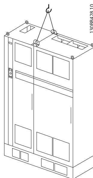
Illustration 4.5 Méthode de levage recommandée, châssis de taille F18 - section du variateur.
