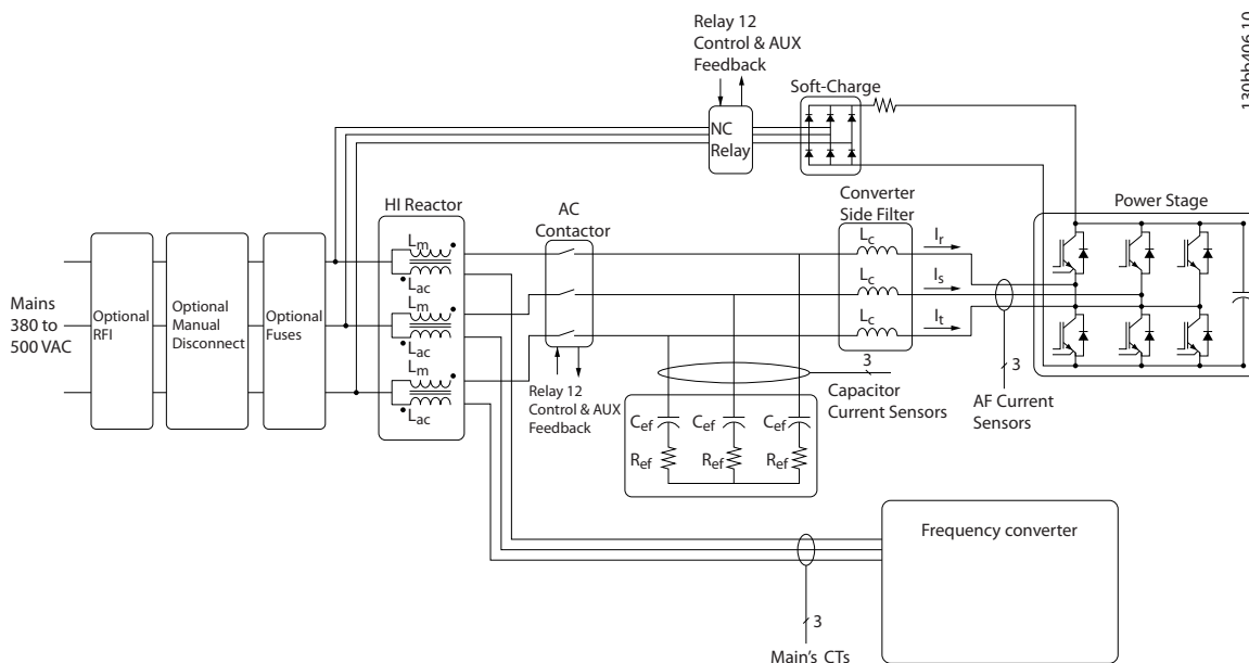
Illustration 3.1 Configuration de base d'un variateur Low Harmonic Drive
