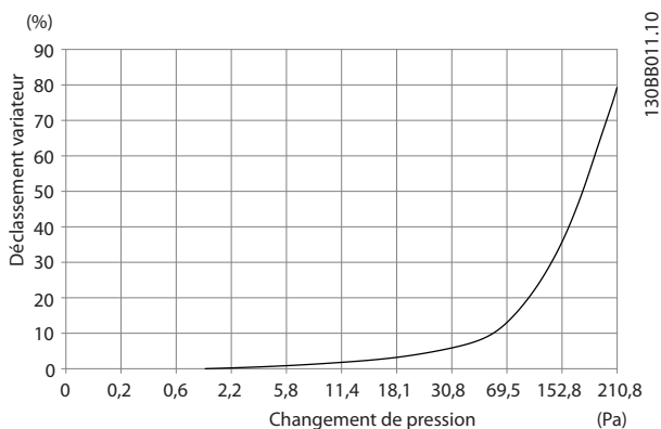
Illustration 4.23 Déclassement du châssis E en fonction du changement de pression (grand ventilateur), P355-P450 Débit d'air du variateur : 1445 m 3 /h (850 cfm)
