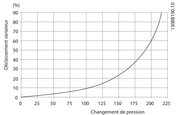
Illustration 4.24 Déclassement du châssis F en fonction du changement de pression Débit d'air du variateur : 985 m 3 /h (580 cfm)
