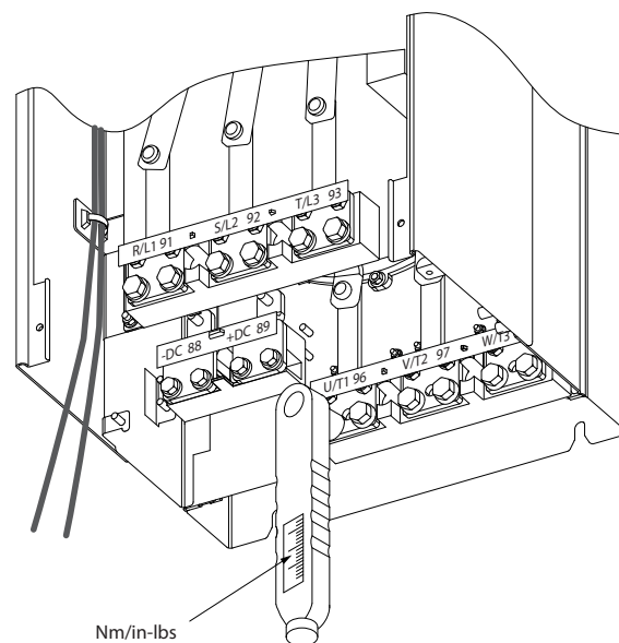
Ilustración 4.37 Utilice siempre una llave dinamométrica para apretar los pernos.
