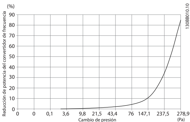
Ilustración 4.22 Reducción de potencia en bastidor E frente a cambio de presión (ventilador pequeño), P315
