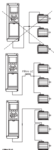
Ilustración 4.41 Instalaciones con cables conectados a un punto común
