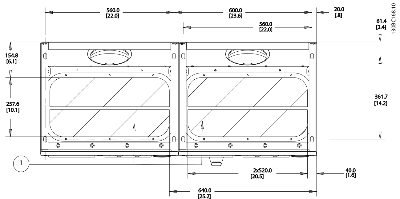
Ilustración 4.27 Tamaño del bastidor E9
