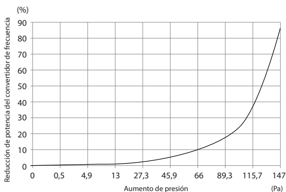
Ilustración 4.21 Reducción de potencia del bastidor D frente a cambio de presión
