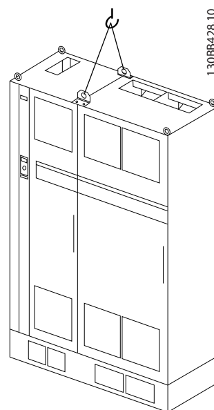
Ilustración 4.5 Método de elevación recomendado, tamaño de bastidor F18: sección del convertidor.
