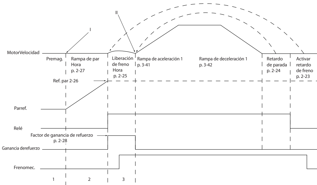
Ilustración 6.4 Secuencia de liberación de freno para control de freno mecánico para elevación
