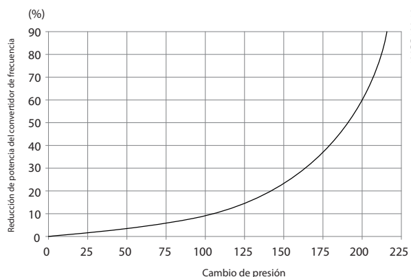
Ilustración 4.24 Reducción de potencia del bastidor F frente a cambio de presión
