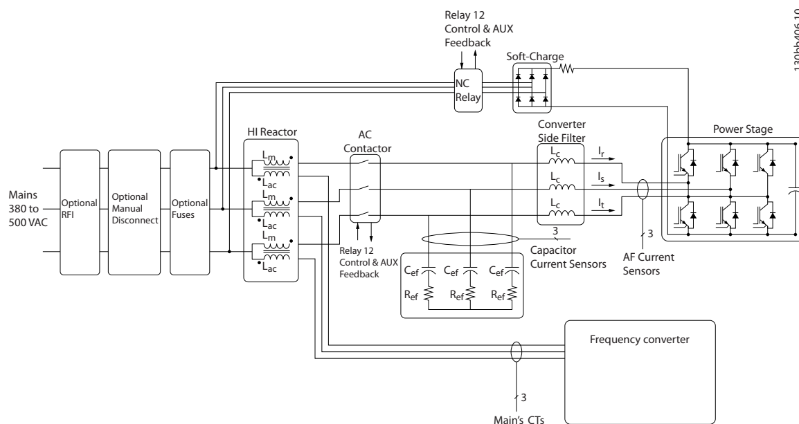
Ilustración 3.1 Disposición básica del convertidor de frecuencia de bajos armónicos
