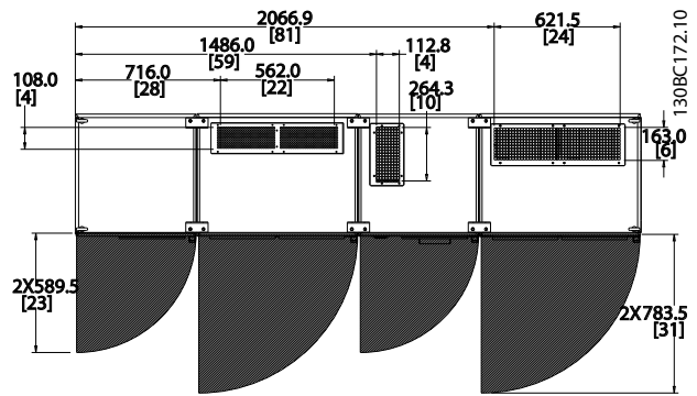
Ilustración 4.12 Espacio delante de la protección tipo IP21 / IP54 , tamaño de bastidor F18.
