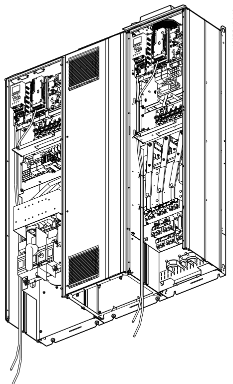
Ilustración 4.38 Trayecto del cableado de la tarjeta de control para el D13
