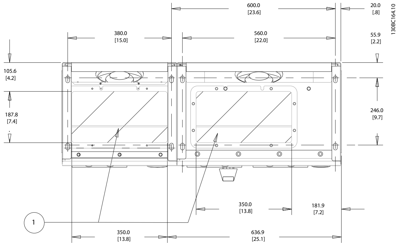
Ilustración 4.26 Tamaño del bastidor D13
