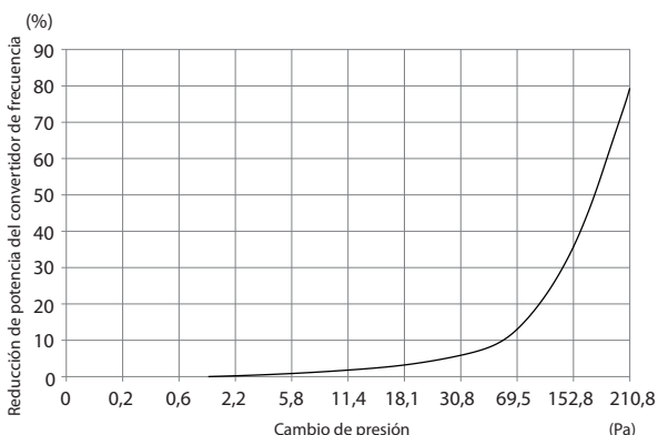
Ilustración 4.23 Reducción de potencia en bastidor E frente a cambio de presión (ventilador grande) P355-P450
