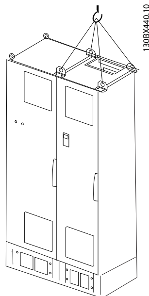
Ilustración 4.4 Método de elevación recomendado, tamaño de bastidor F18: sección de filtro.
