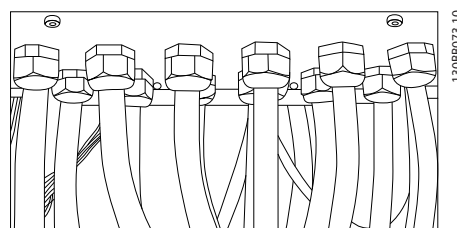
Ilustración 4.25 Ejemplo de instalación adecuada de la placa de prensacables.
