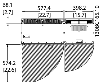
Ilustración 4.10 Espacio delante de la protección tipo IP21 / IP54, tamaño de bastidor D13.
