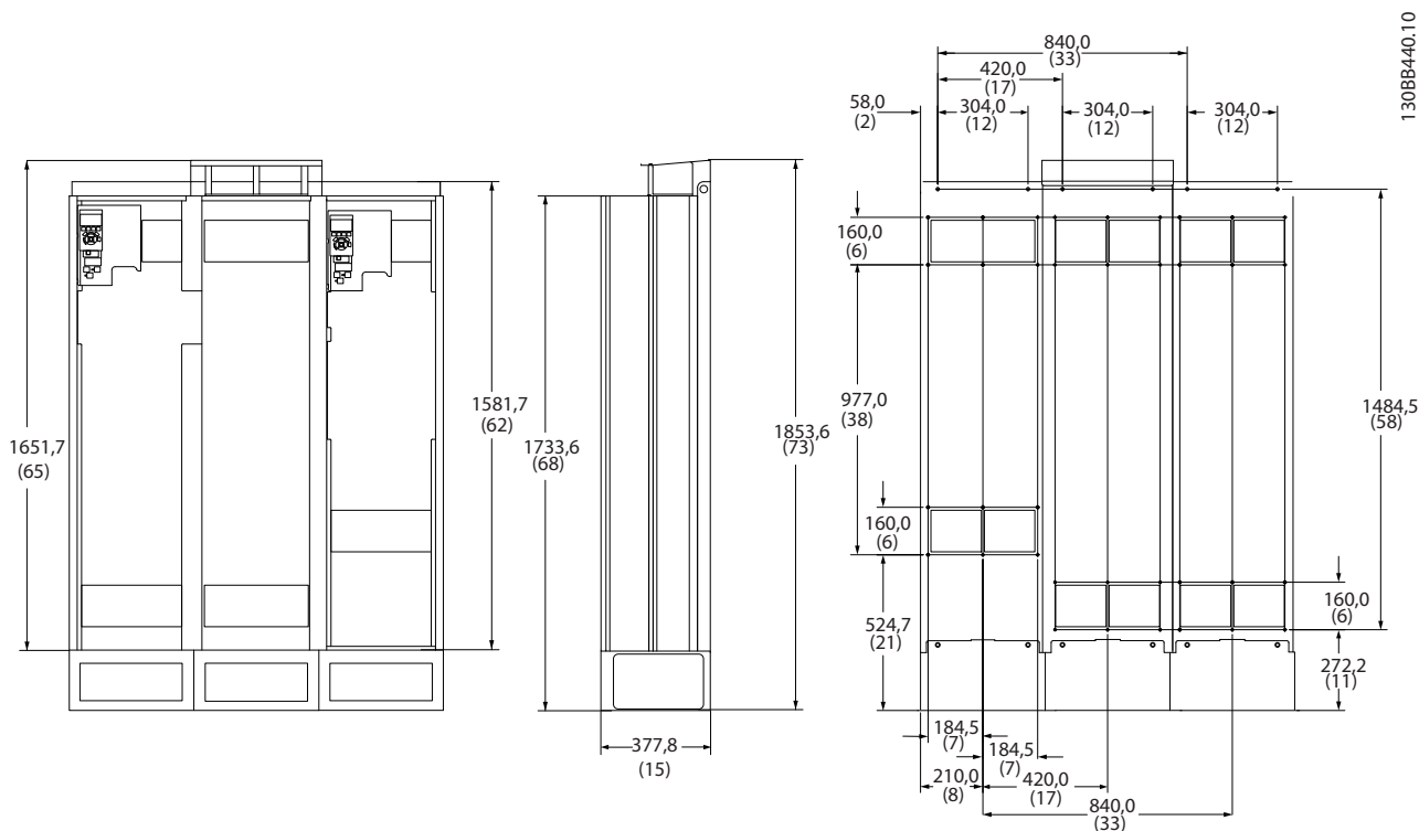
Ilustración 4.6 Tamaño del bastidor D13
