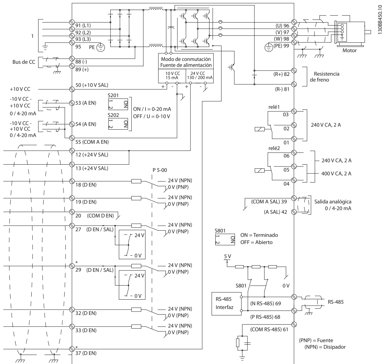
Ilustración 4.40 Diagrama que muestra todos los terminales eléctricos sin opciones.
