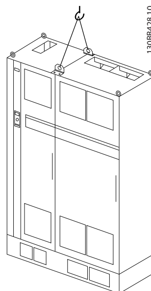
Bild 4.5 Rekommenderad lyftmetod, kapsling F18 - frekvensomformaravsnitt.
