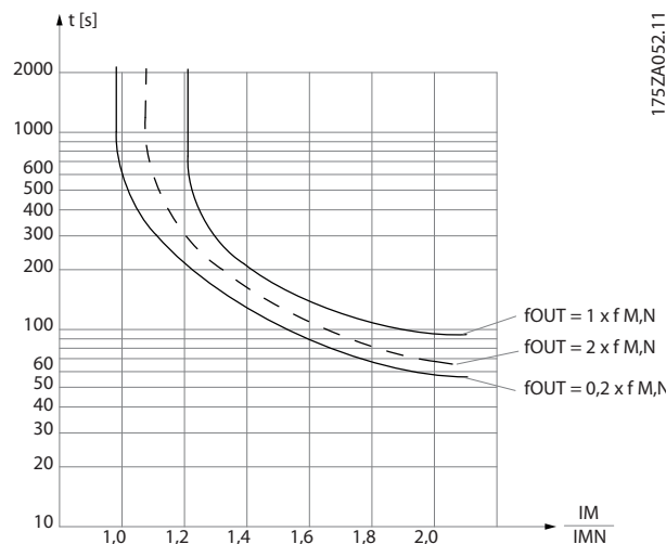
Bild 6.3 ETR-profil
