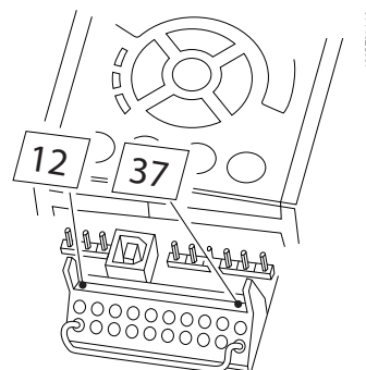
Bild 2.1 Bygel mellan plint 37 och 24 V DC
