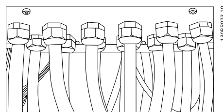
Bild 4.25 Exempel på korrekt installation av boxplåten.
