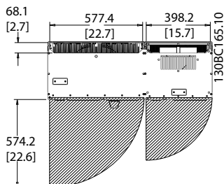
Bild 4.10 Utrymme framför IP21/IP54-kapslingstyp, kapslingsstorlek D13.
