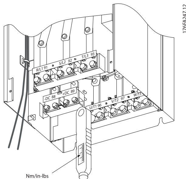
Bild 4.37 Använd alltid en momentnyckel för att dra åt bultarna.
