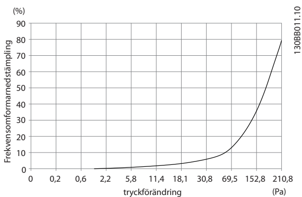
Bild 4.23 E-kapsling, nedstämpling vs. Tryckförändring (stor fläkt), P355-P450
