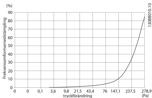
Bild 4.22 E-kapsling, nedstämpling vs. Tryckförändring (liten fläkt), P315
