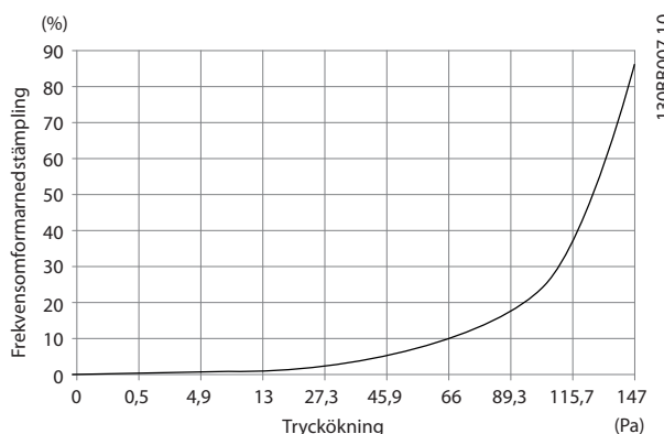
Bild 4.21 D-kapsling, nedstämpling vs. tryckförändring Frekvensomformarens luftflöde: 450 cfm (765 m 3 /h)
