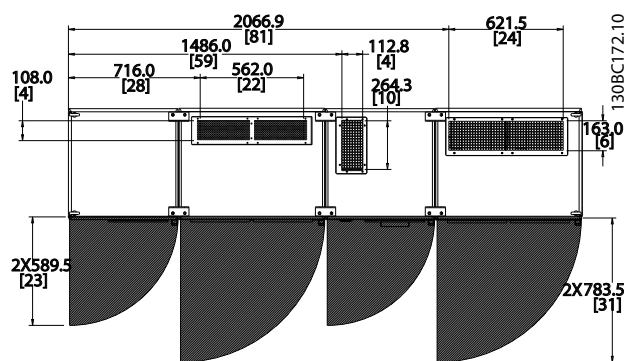
Bild 4.12 Utrymme framför IP21/IP54-kapslingstyp, kapslingsstorlek F18.
