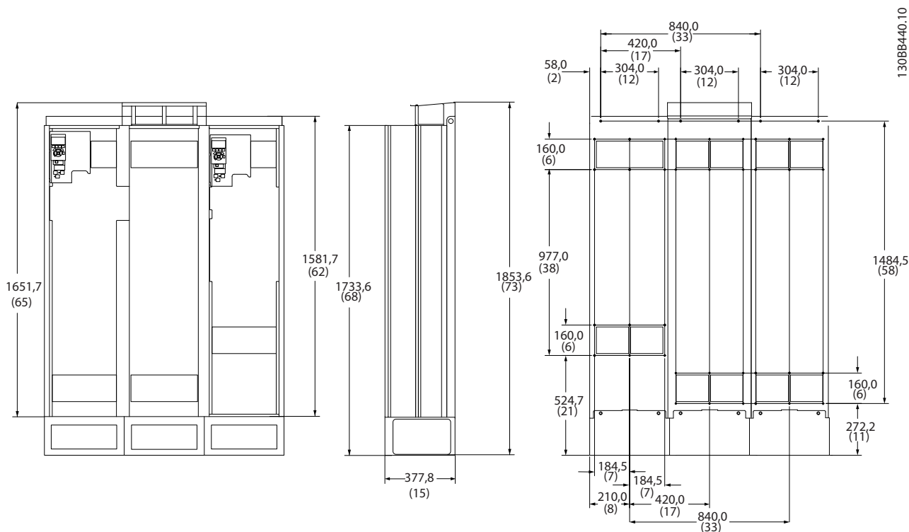
Bild 4.6 Kapsling D13
