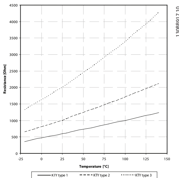
Bild 6.2 Val av KTY-typ
