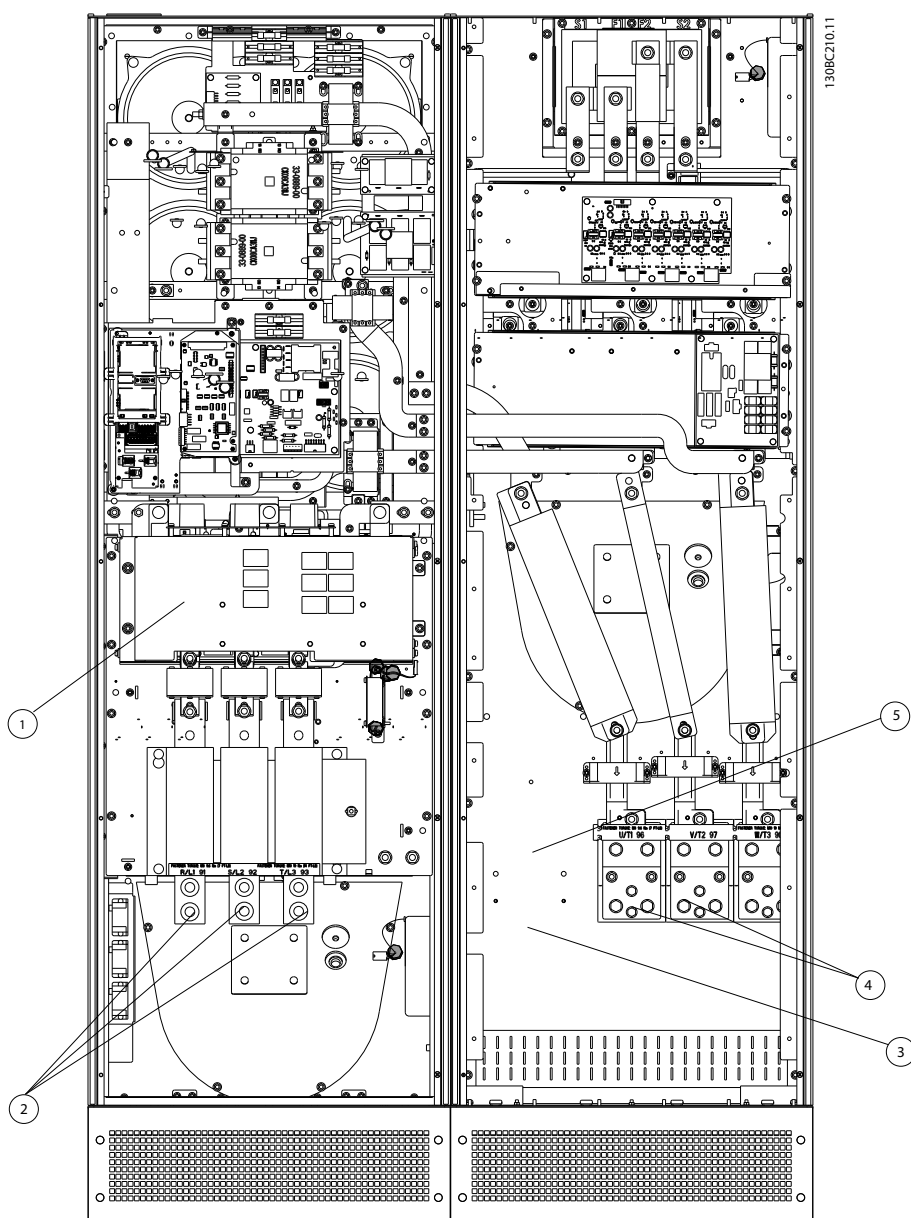
Bild 4.32 Kapsling E9
