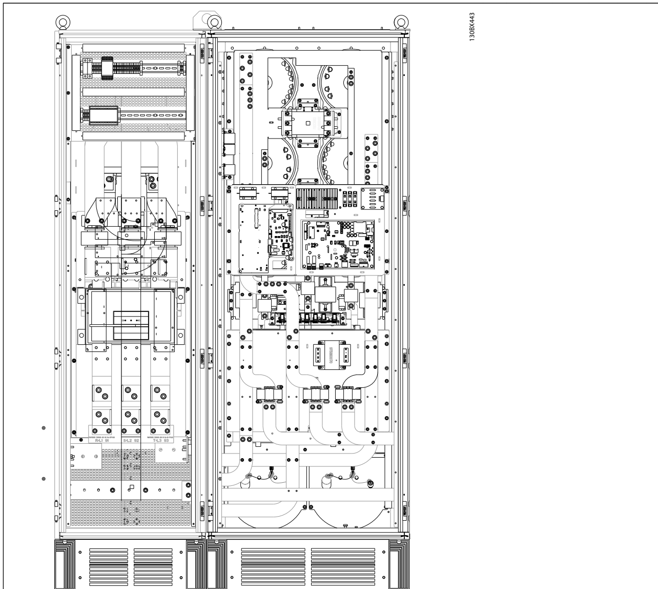
Bild 4.34 Aktivt filter, kapsling F18
