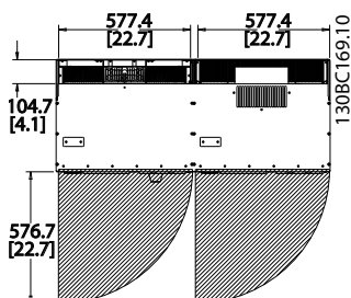
Bild 4.11 Utrymme framför IP21/IP54-kapslingstyp, kapslingsstorlek E9.
