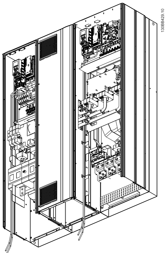
Bild 4.39 Kabeldragning för styrkort för E9
