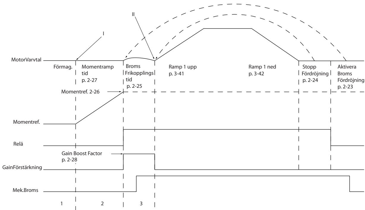
Bild 6.4 Bromsfrikopplingssekvens för styrning av mekanisk broms i lyfttillämpningar
