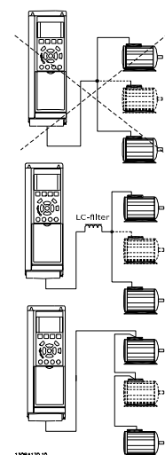
Bild 4.41 Installationer med kablar anslutna i en gemensam koppling
