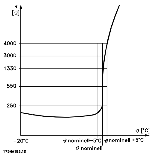
Bild 6.1 PTC-profil
