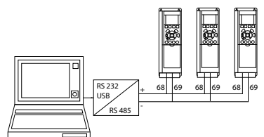
Bild 5.8 Anslutningsexempel.
