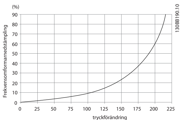
Bild 4.24 F-kapsling nedstämpling vs. tryckförändring
