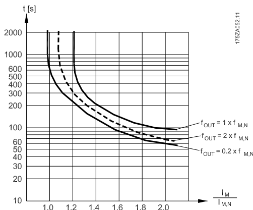
그림 6.3 ETR 프로파일
