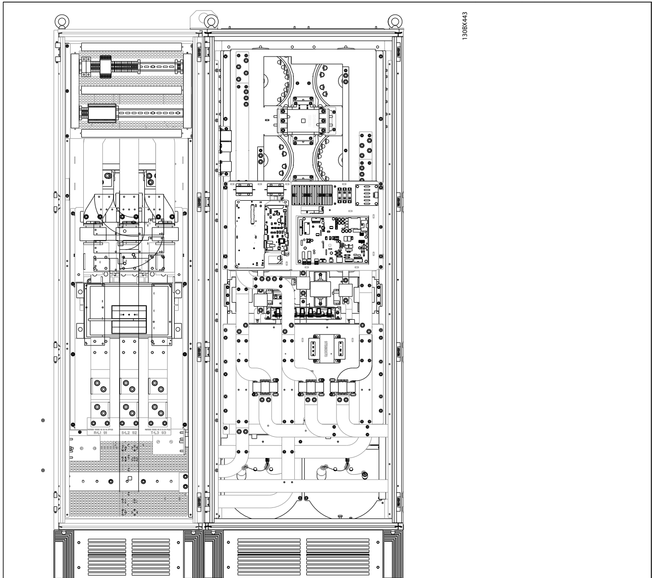
그림 4.34 Active Filter, 프레임 용량 F18
