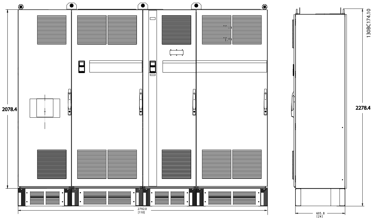
그림 4.8 프레임 용량 F18, 전면 및 측면 보기
