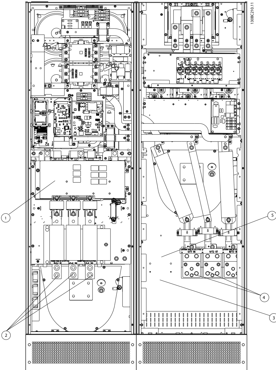
그림 4.32 프레임 용량 E9
