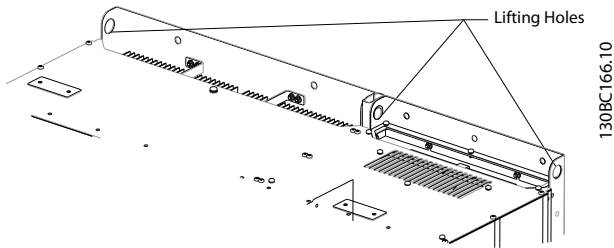
그림 4.2 들어 올리는 방법(권장), 프레임 용량 D13
