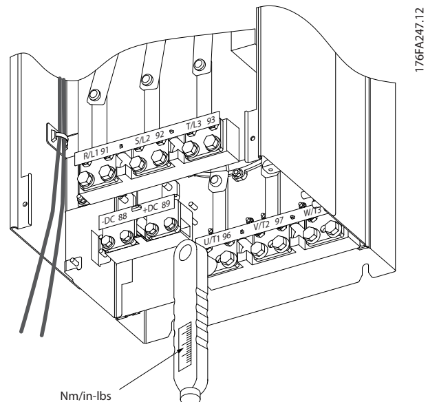
그림 4.37 볼트를 조일 때는 반드시 토크 측정용 렌치를 사용하십시오.
