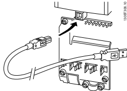
그림 5.9 제어 케이블 연결은 4.8.1 전기적인 설치, 제어 케이블 을 참조하십시오.
