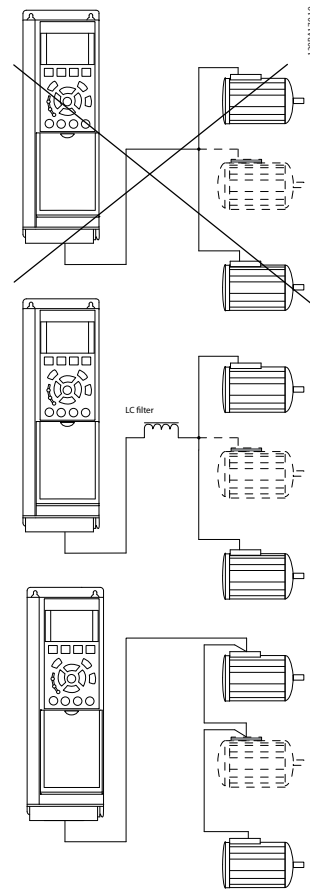
그림 4.41 공통 조인트에 연결된 케이블을 사용하여 설치한 경우
