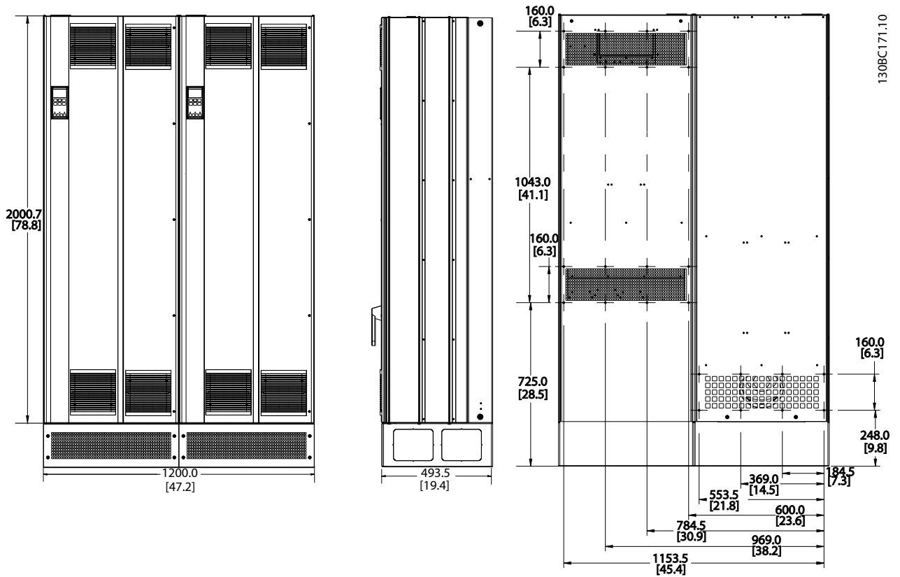
그림 4.7 프레임 용량 E9
