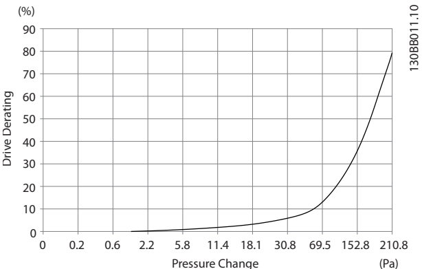
그림 4.23 E 프레임 용량 감소와 압력 변화 간 비교(대형 팬), P355-P450 인버터 통풍량: 850 cfm (1445 m 3 /h)
