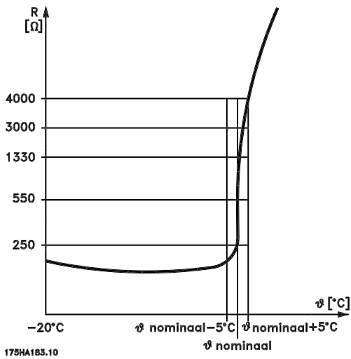
그림 6.1 PTC 프로파일
