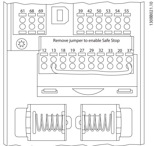
그림 7.1 제어카드 단자
