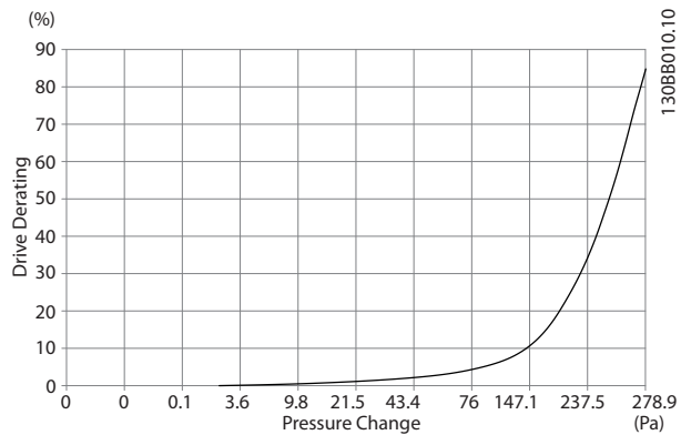
그림 4.22 E 프레임 용량 감소와 압력 변화 간 비교(소형 팬), P315 인버터 통풍량: 650 cfm (1105 m 3 /h)
