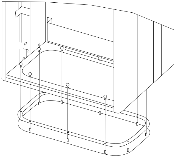
그림 4.28 하단 플레이트 장착, 프레임 용량 E9
