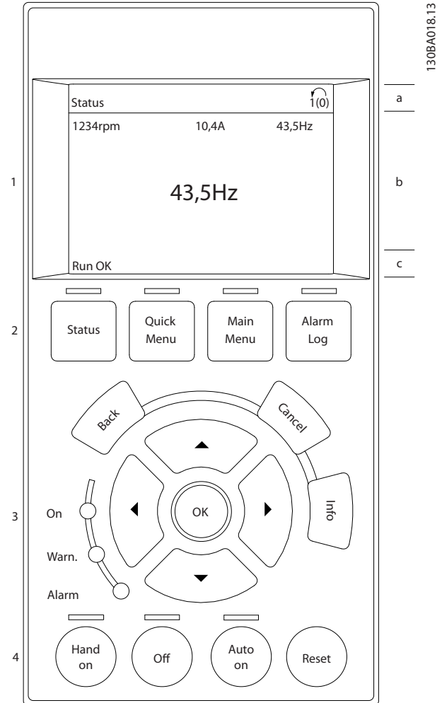
그림 5.1 LCP
