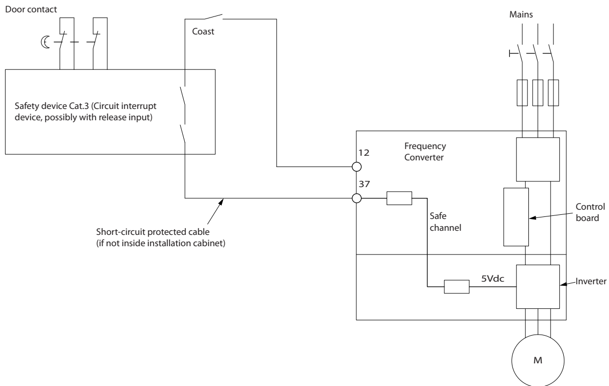
그림 2.2 안전 부문 3(EN 954-1)에 의거, 정지 부문 0(EN 60204-1)을 만족시키기 위한 설비의 필수 요소 그림.
