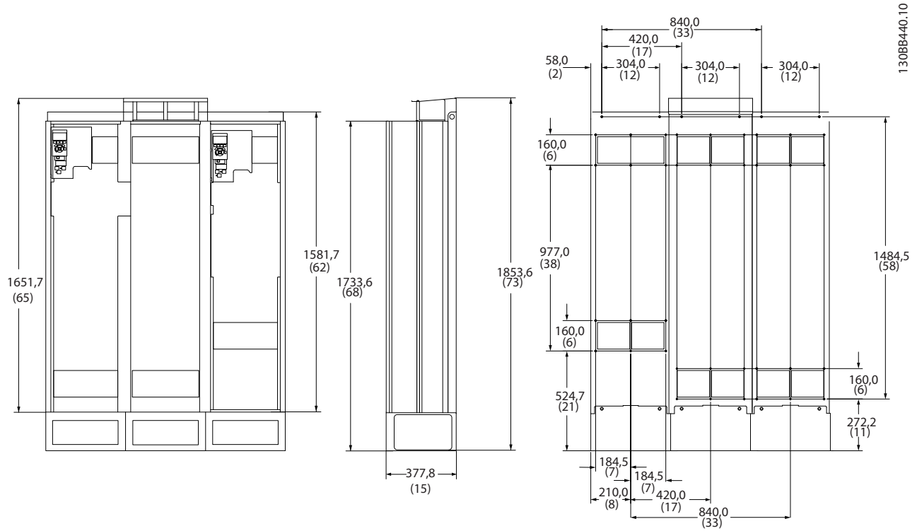
그림 4.6 프레임 용량 D13
