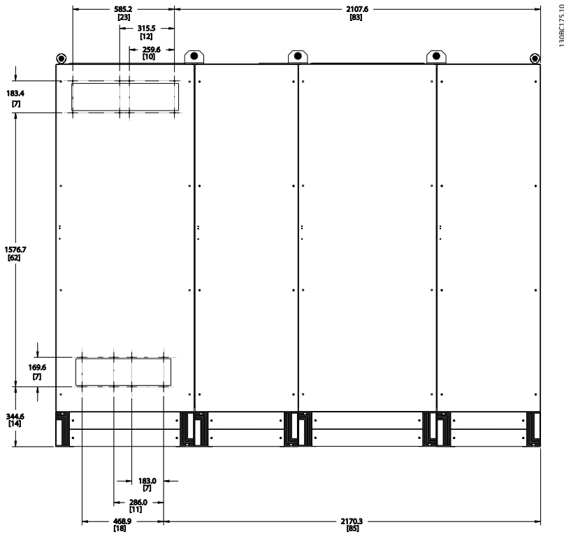
그림 4.9 프레임 용량 F18, 뒷면 보기
