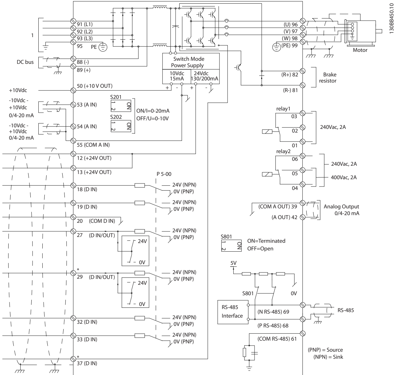
그림 4.40 옵션을 제외한 모든 전기 단자를 나타내는 다이어그램.
