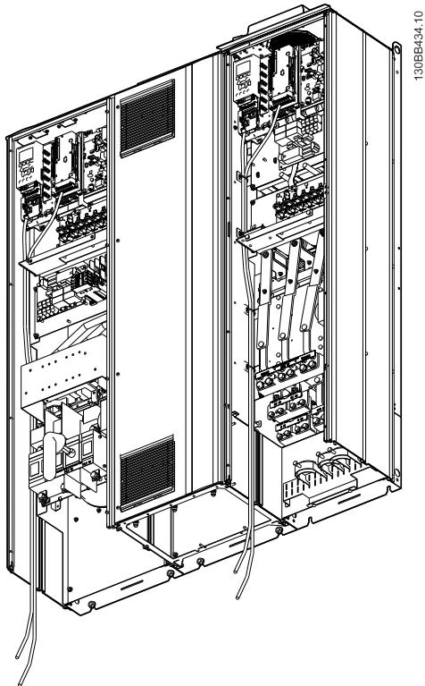
그림 4.38 D13의 제어 카드 배선 경로
