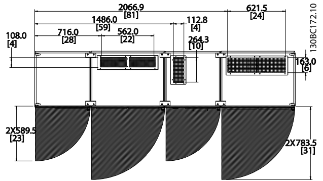
그림 4.12 IP21/IP54 외함 유형, 프레임 용량 F18 전면의 여유 공간.
