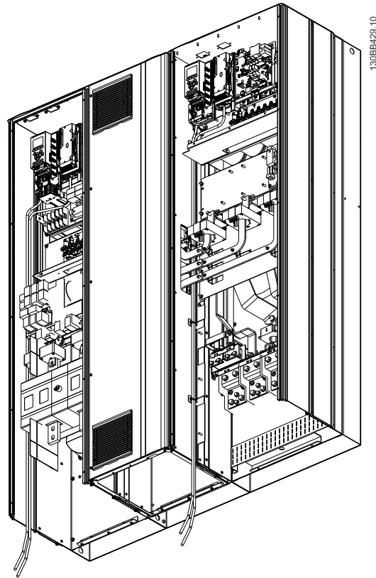
그림 4.39 E9의 제어 카드 배선 경로
