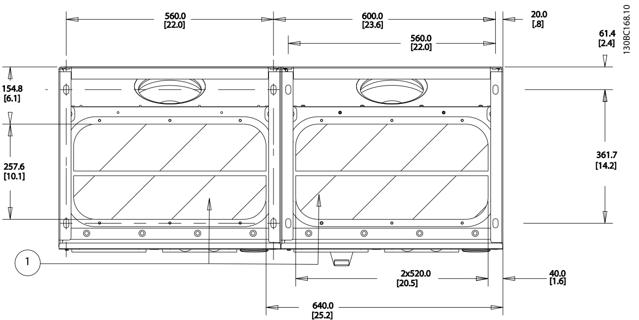
그림 4.27 프레임 용량 E9
