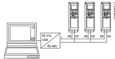
그림 5.8 연결 예.
