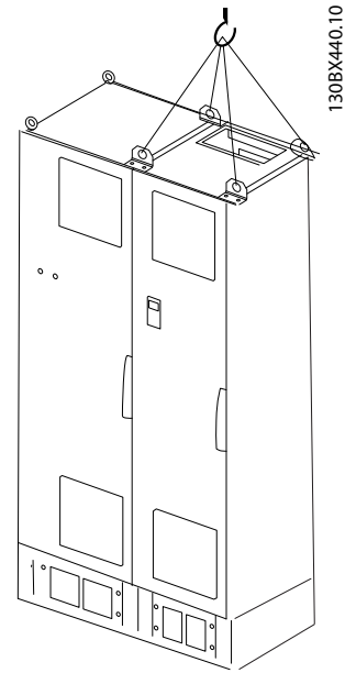
그림 4.4 들어 올리는 방법(권장), 프레임 용량 F18 - 필터부
