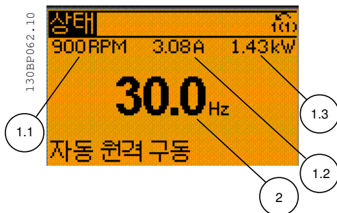
그림 5.3 상태 표시 II - 운전 변수
