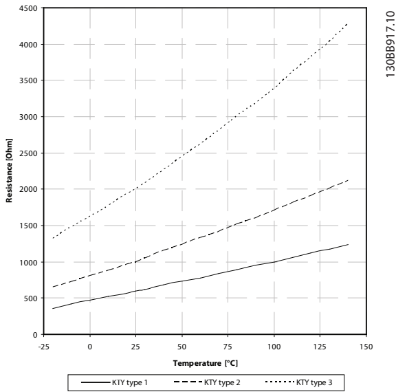
그림 6.2 KTY 유형 선택
