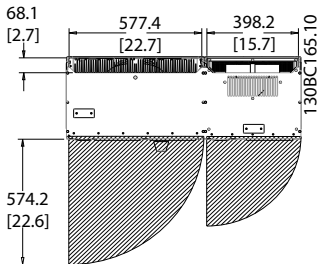
그림 4.10 IP21/IP54 외함 유형, 프레임 용량 D13 전면의 여유 공간.
