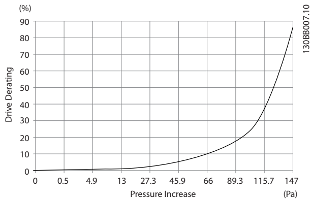
그림 4.21 D 프레임 용량 감소와 압력 변화 간 비교 인버터 통풍량: 450 cfm (765 m 3 /h)
