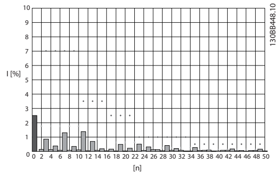
그림 3.2 인버터 주전원 단자에서의 일반 고조파 주파수 스펙트럼 및 THD 값
