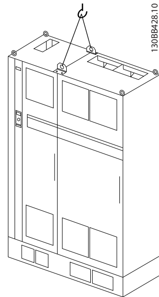
그림 4.5 들어 올리는 방법(권장), 프레임 용량 F18 - 인버터부
