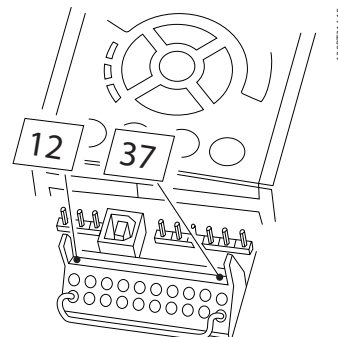
그림 2.1 단자 37 과 24V DC 간의 브리지 점퍼
