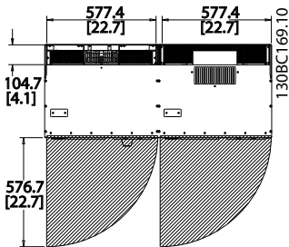
그림 4.11 IP21/IP54 외함 유형, 프레임 용량 E9 전면의 여유 공간.
