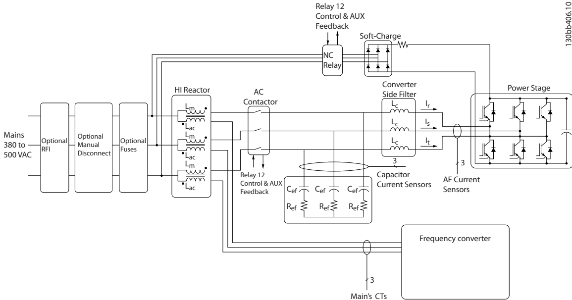
그림 3.1 최소 고조파 인버터를 위한 기본 설계
