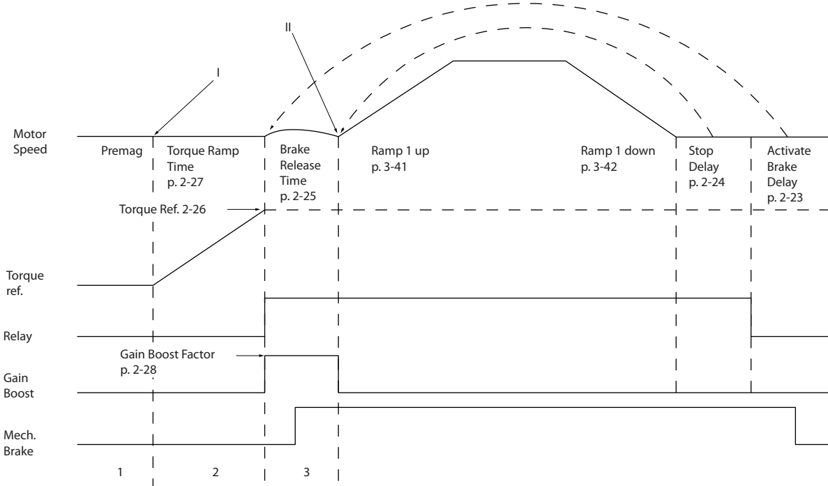
그림 6.4 호이스트 기계식 제동장치 제어를 위한 제동 해제 시퀀스
