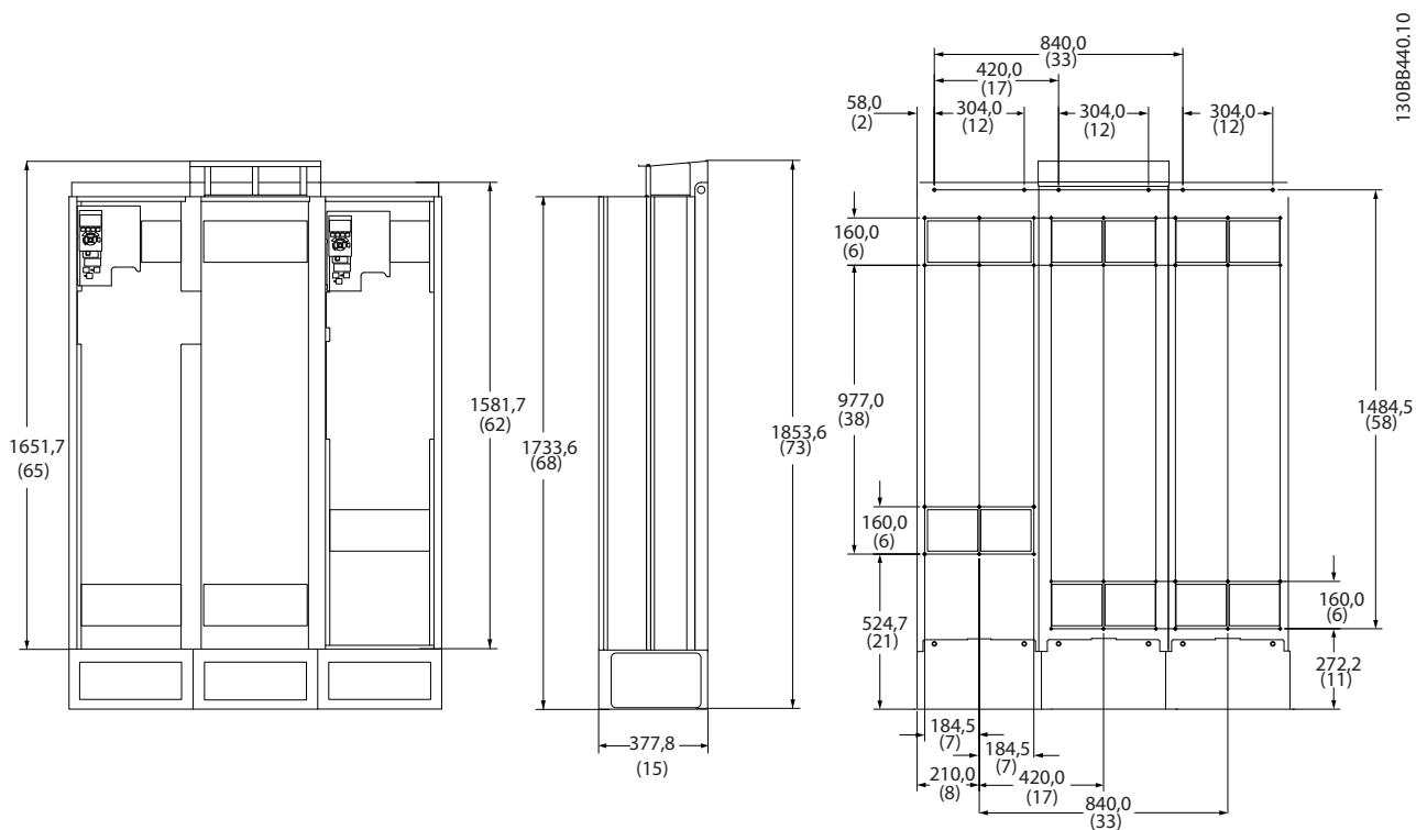
圖 4.6 機架大小 D13
