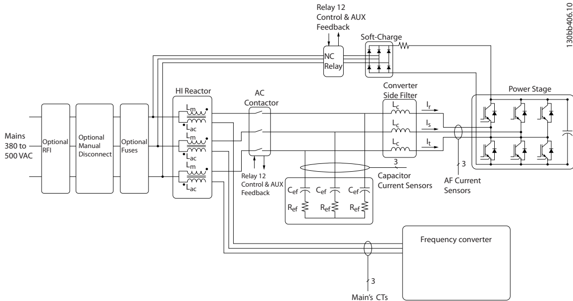
圖 3.1 低諧波變頻器的基本配置
