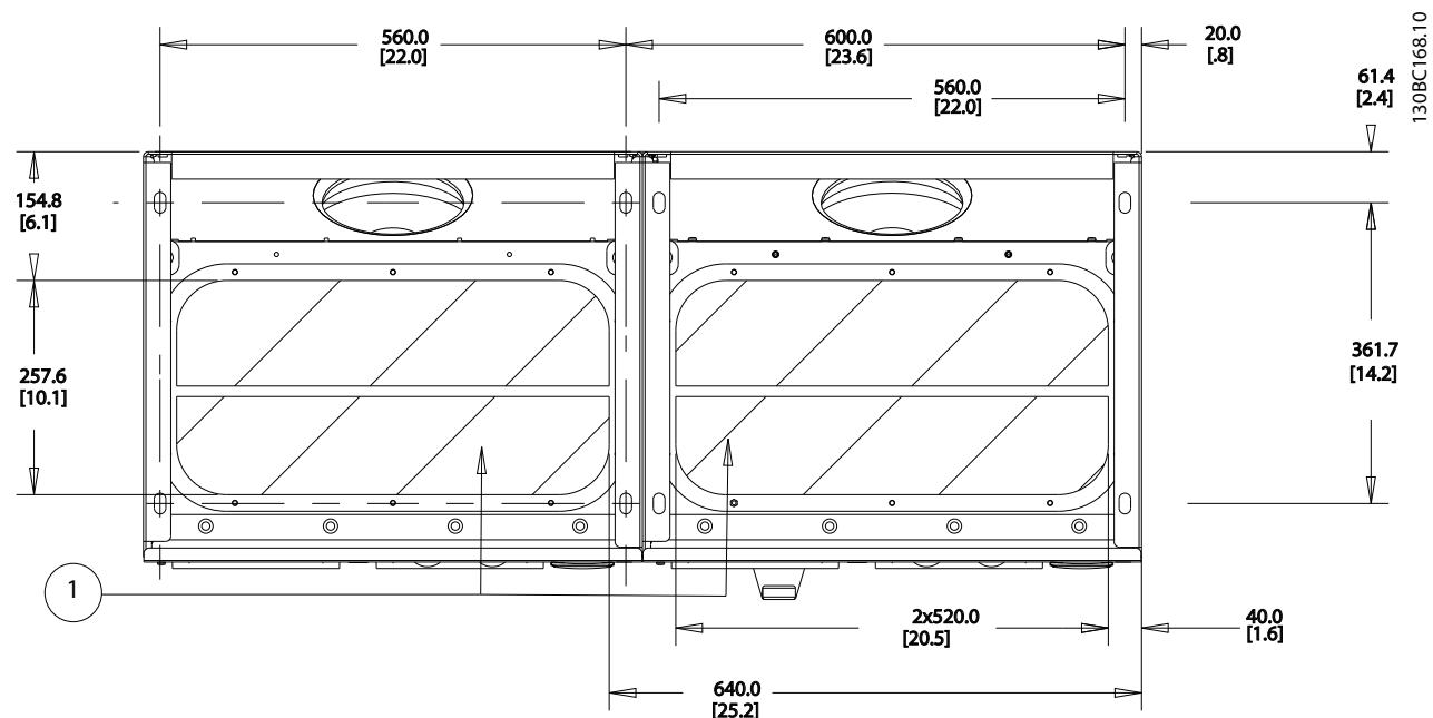
圖 4.27 機架大小 E9
