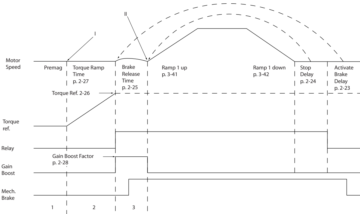
圖 6.4 起重機械煞車控制的煞車釋放程序
