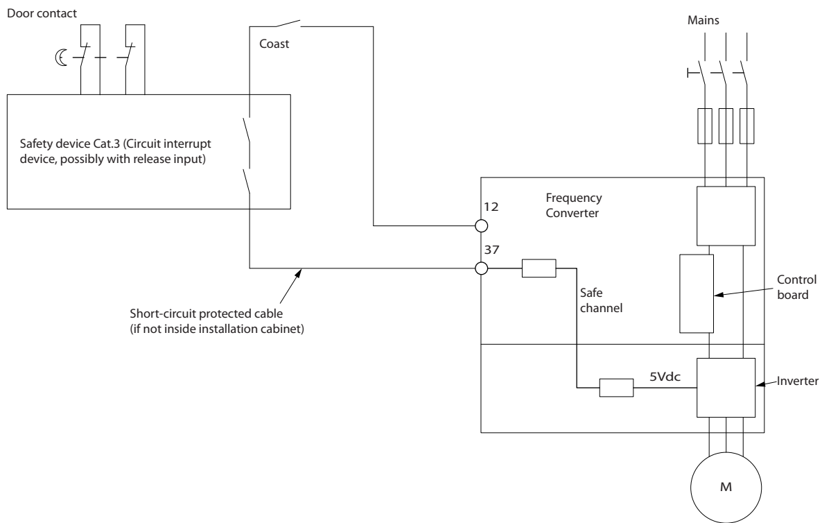
圖 2.2 符合 安全類別 3 (EN 954-1) 的停止類別 0 (EN 60204-1) 的安裝所需的基本配置之圖解。
