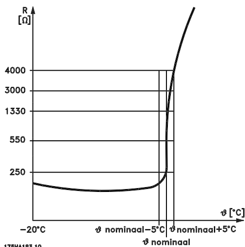
圖 6.1 PTC 描述檔
