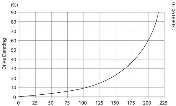
圖 4.24 F 機架隨著 壓力變化降低額定值 變頻器空氣流量: 580 cfm (985 m 3 /h)
