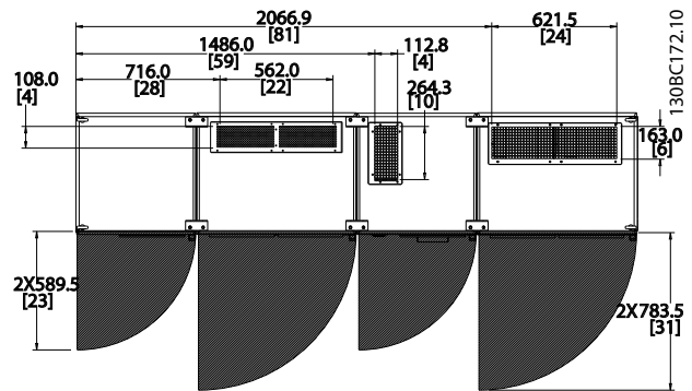
圖 4.12 IP21/IP54 外殼類型, 機架大小 F18 的前方空間。
