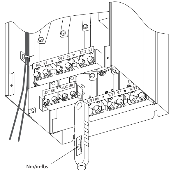
圖 4.37 務必使用扭力扳手將螺栓扭緊。
