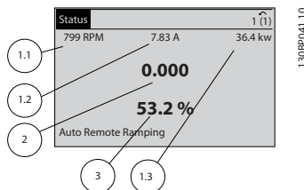
圖 5.2 狀態顯示 I - 操作變數
