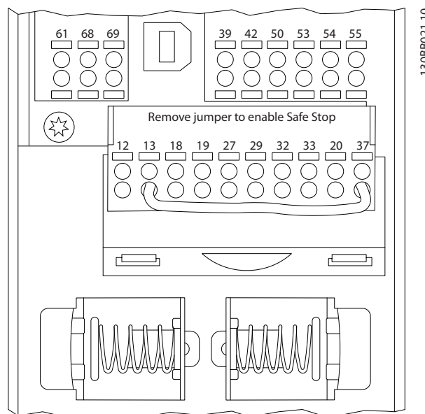
圖 7.1 控制卡端子
