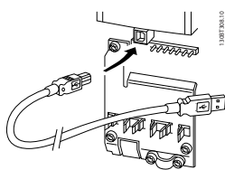
圖 5.9 有關控制電纜的連接，請參閱 4.8.1 電氣安裝，控制電纜線。
