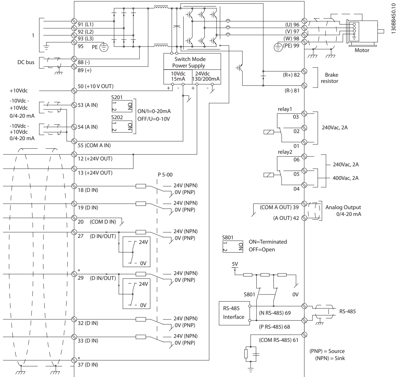
圖 4.40 顯示所有不含選項的電氣端子的圖表。
