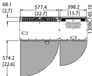
圖 4.10 IP21/IP54 外殼類型, 機架大小 D13 的前方空間。
