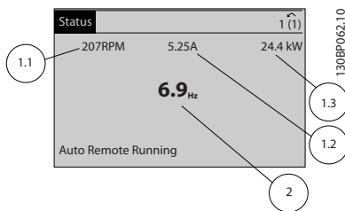
圖 5.3 狀態顯示 II - 操作變數
