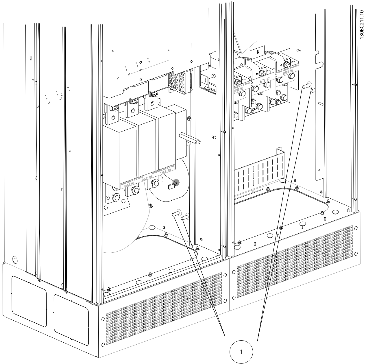
圖 4.33 地線端子位置
