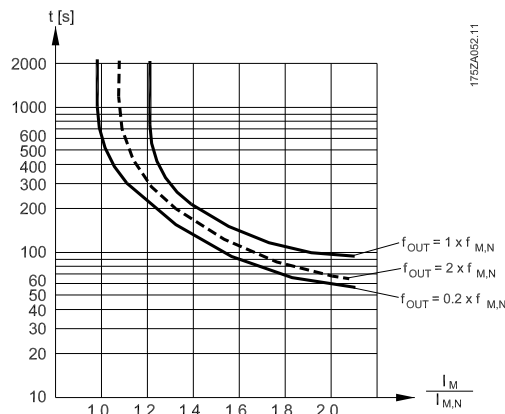
圖 6.3 ETR 描述檔
