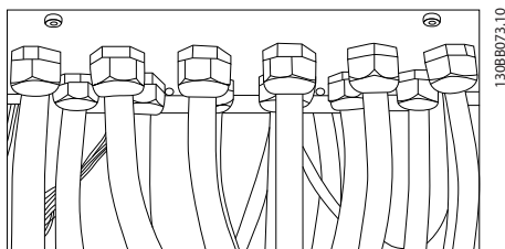
圖 4.25 纜線固定頭板正確安裝的範例。
