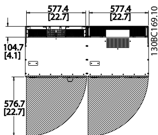
圖 4.11 IP21/IP54 外殼類型, 機架大小 E9 的前方空間。
