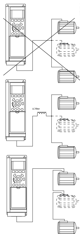
圖 4.41 電纜線連接至共同接合處的安裝例
