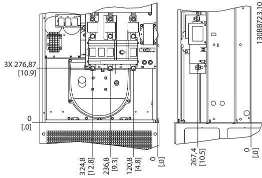
圖 4.13 端子位置 - 主電源電纜線
