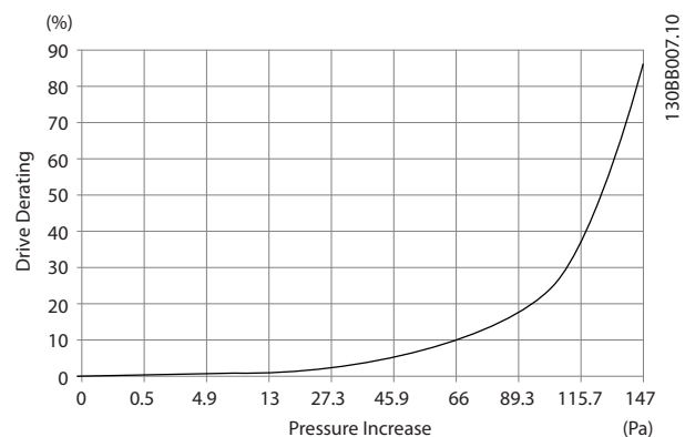
圖 4.21 D 機架隨著 壓力變化降低額定值 變頻器空氣流量：450 cfm (765 m 3 /h)
