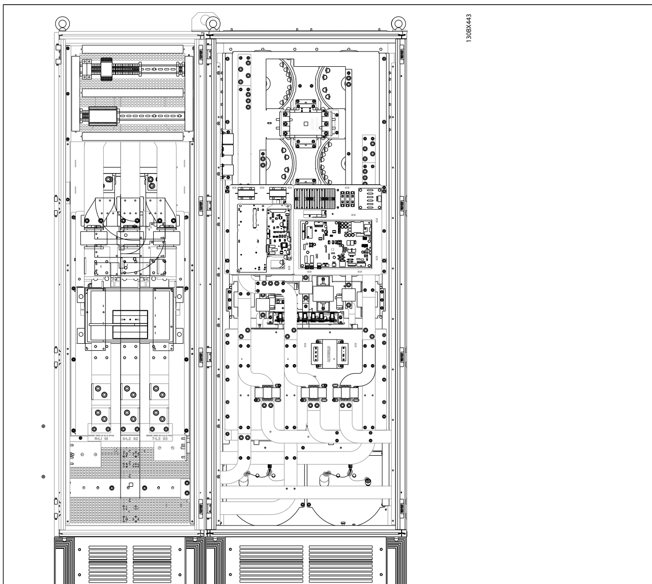
圖 4.34 主動型濾波器，機架大小 F18
