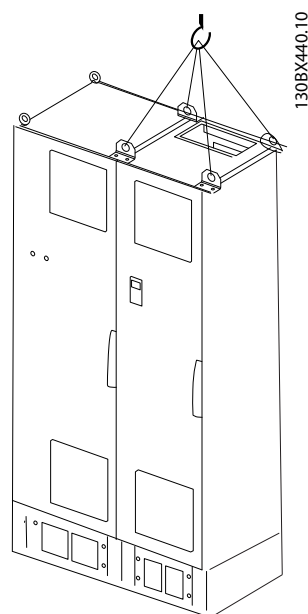
圖 4.4 建議的吊掛方式，機架大小 F18 - 濾波器部分。
