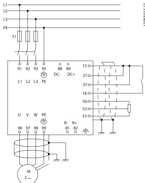
圖 4.1 本圖顯示基本的安裝，包括：主電源、馬達、啟動/停機鍵和用於速度調整的電位器。
