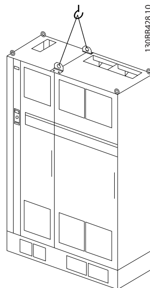
圖 4.5 建議的吊掛方式，機架大小 F18 - 變頻器部分。
