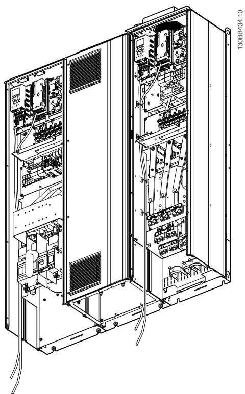
圖 4.38 D13 控制卡線路的路線
