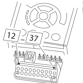
圖 2.1 端子 37 和 24 V 直流之間的橋接器跳線
