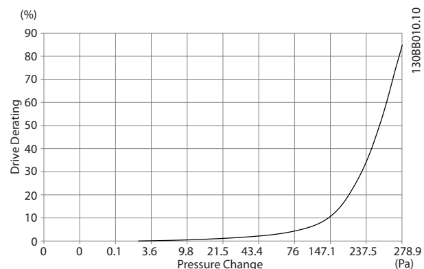
圖 4.22 E 機架隨著 壓力變化降低額定值（小風扇），P315 變頻器空氣流量：650 cfm (1105 m 3 /h)
