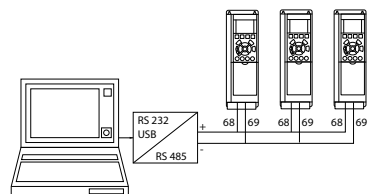
圖 5.8 連接範例。
