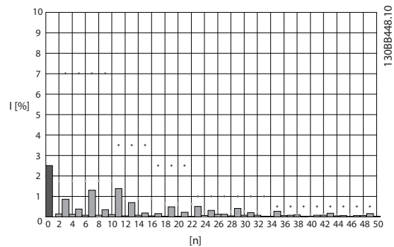
圖 3.2 在變頻器主電源端子的典型諧波變頻器頻譜與 THD 值 n = 諧波級數 ◇.....IEEE519 對個別諧波級數的限制 ( I_{sc}/I_l > 20 )
