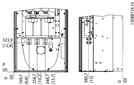
圖 4.14 端子位置 E9 - 變頻器
