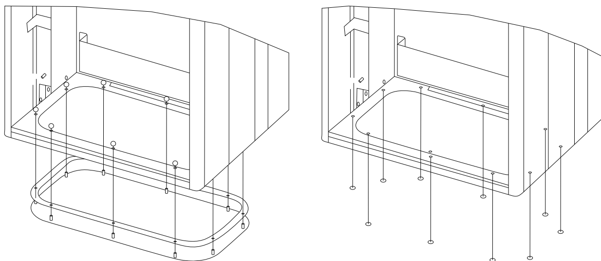
圖 4.28 底板的安裝，機架大小 E9
