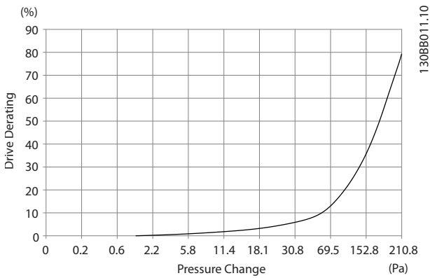
圖 4.23 E 機架隨著 壓力變化降低額定值 (大風扇), P355-P450 變頻器空氣流量: 850 cfm (1445 m 3 /h)
