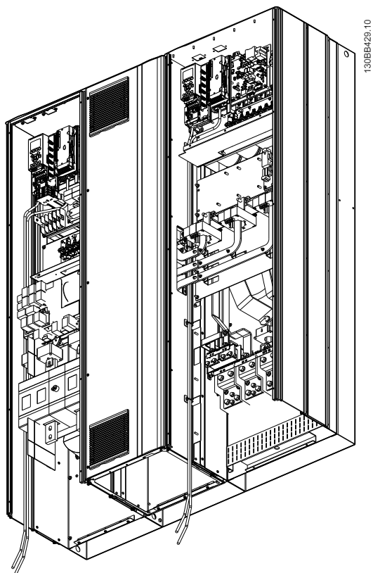
圖 4.39 E9 控制卡線路的路線
