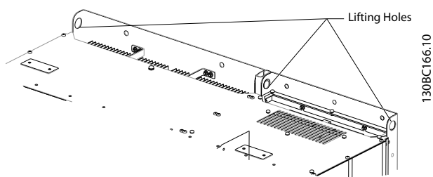
圖 4.2 建議的吊掛方式，機架大小 D13
