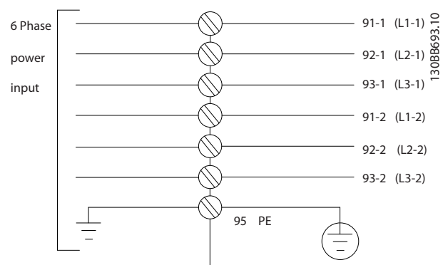
Illustration 3.32 Strømkabeltilslutninger
