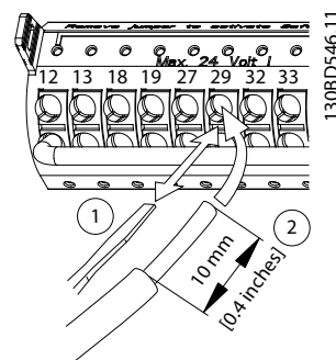
Illustration 3.49 Tilslutning af styreledninger
