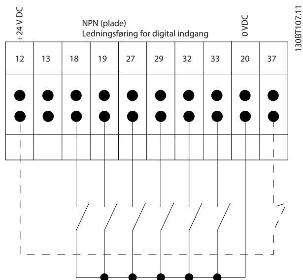
Illustration 3.53 NPN (plade)
