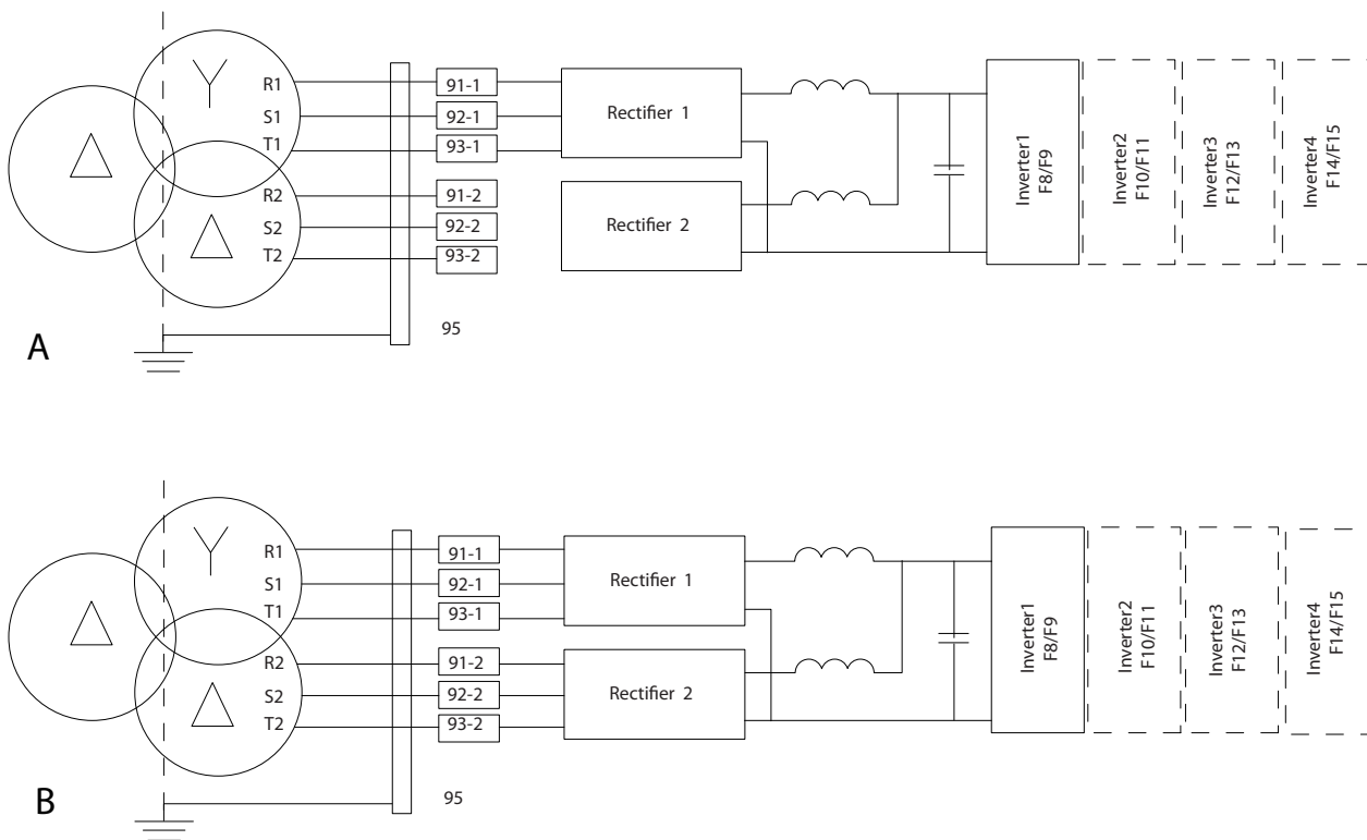
Disegno 3.33 A) Collegamento provvisorio a 6 impulsi 1) B) Collegamento a 12 impulsi
