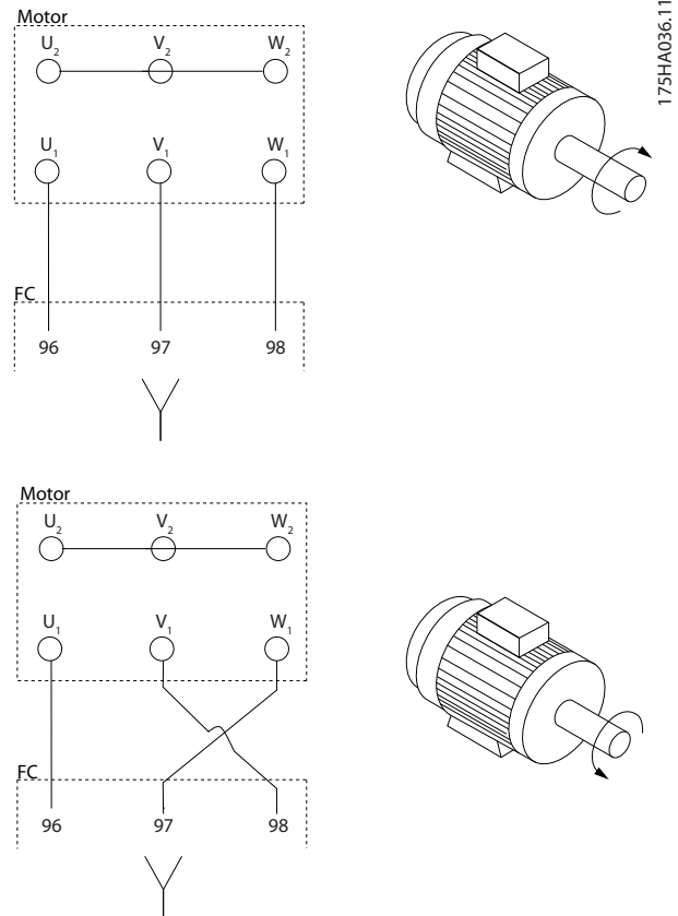
Disegno 3.45 Cablaggio per la rotazione oraria e antioraria del motore
