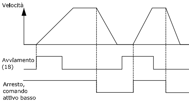
Disegno 3.57 Avviamento/arresto a impulsi cablaggio
