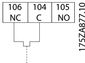
그림 3.47 제동 저항 온도 스위치
