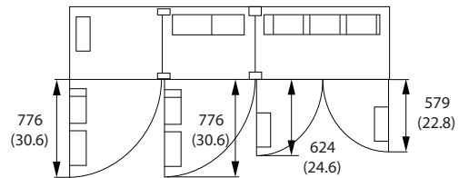
그림 3.10 외함 용량 F13 전면의 여유 공간
