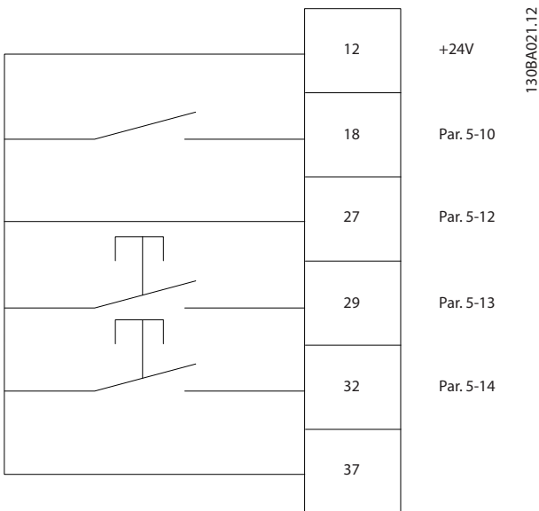
그림 3.58 가속/감속
