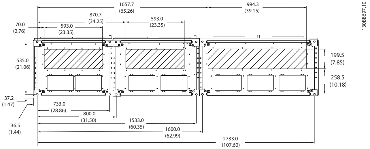
그림 3.29 F13, 주파수 변환기 하단에서 본 케이블 입구
