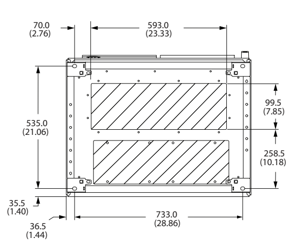
그림 3.24 F8, 주파수 변환기 하단에서 본 케이블 입구
