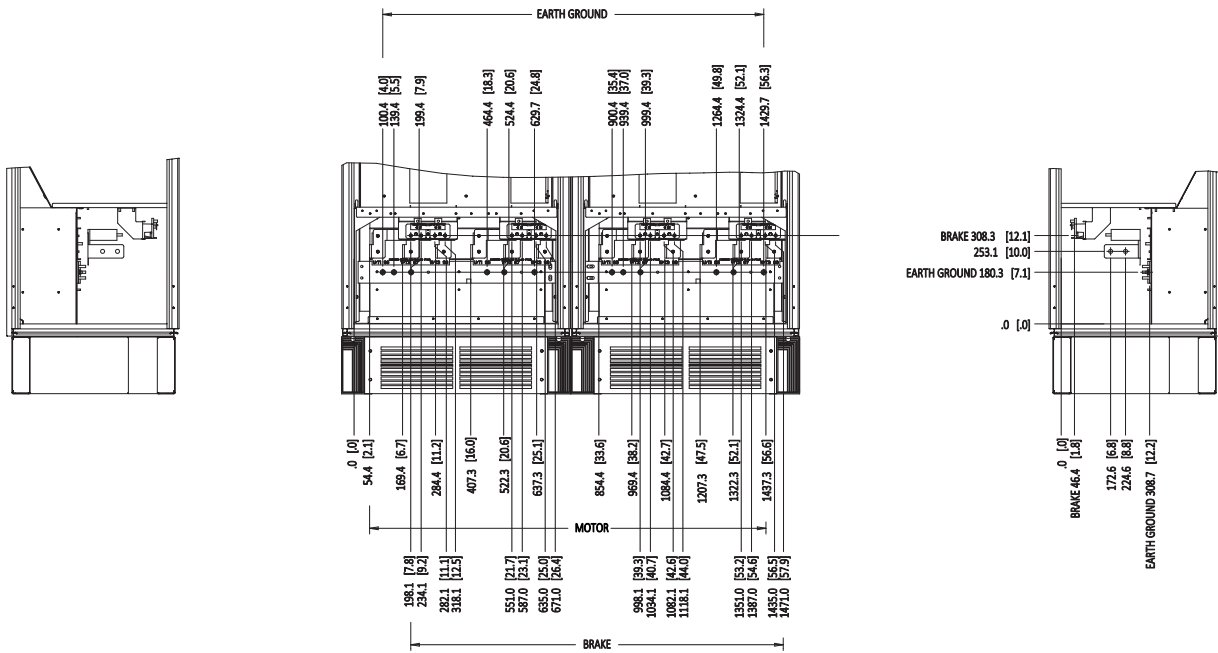
그림 3.16 단자 위치 - 왼쪽, 전면 및 오른쪽 보기. 브레이크 플레이트는 0.0 레벨보다 42 mm (1.65인치) 아래에 있습니다.
