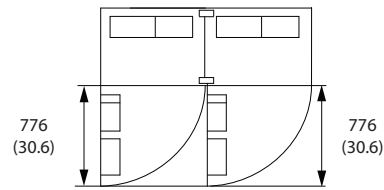
그림 3.7 외함 용량 F10 전면의 여유 공간
