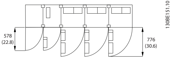
그림 3.12 외함 용량 F15 전면의 여유 공간
