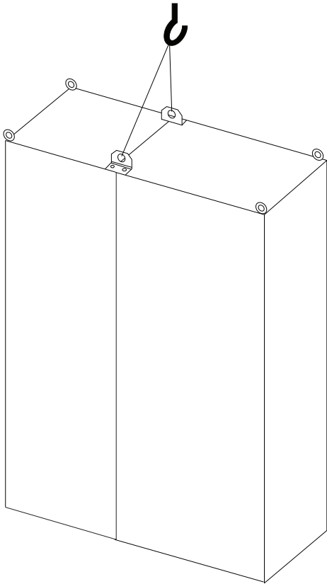
그림 3.2 들어 올리는 방법(권장), 외함 용량 F9/F10.
