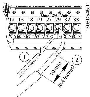
그림 3.49 제어 와이어 연결
