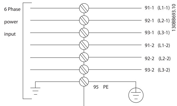
그림 3.32 전원 케이블 연결
