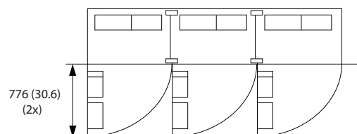
그림 3.11 외함 용량 F14 전면의 여유 공간
