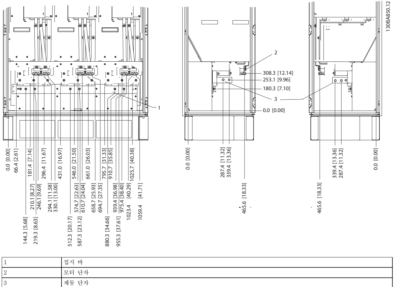
그림 3.15 단자 위치 - 왼쪽, 전면 및 오른쪽 보기. 글랜드 플레이트는 0.0 레벨보다 42 mm (1.65인치) 아래에 있습니다.
