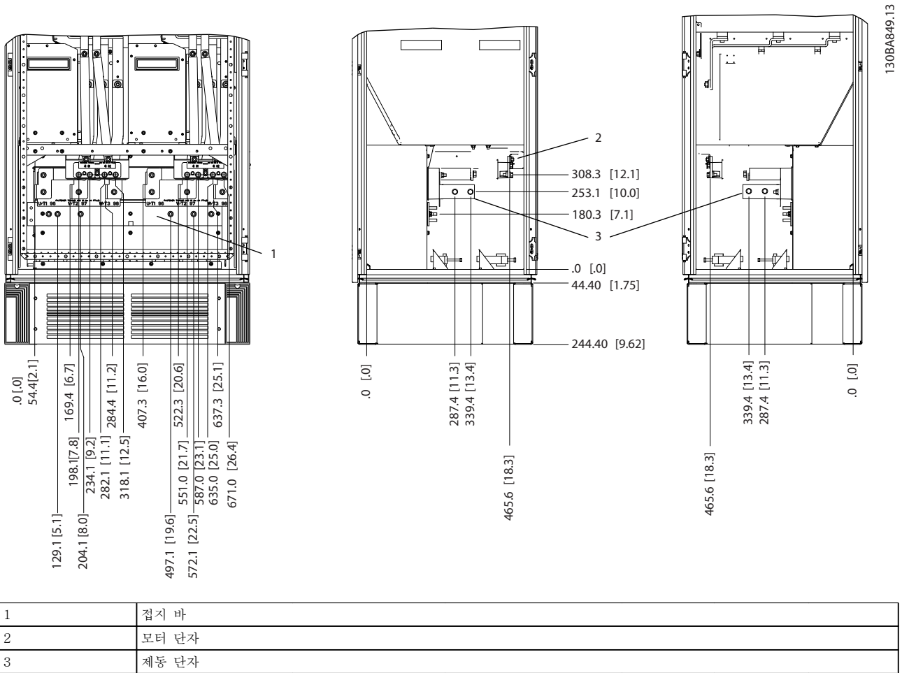
그림 3.14 단자 위치 - 왼쪽, 전면 및 오른쪽 보기. 글랜드 플레이트는 0.0 레벨보다 42 mm (1.65인치) 아래에 있습니다.
