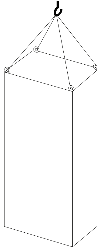
그림 3.1 들어 올리는 방법(권장), 외함 용량 H8.
