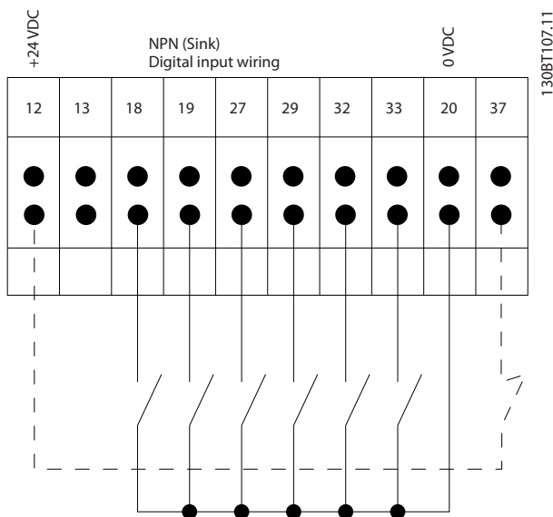
그림 3.53 NPN (싱크)
