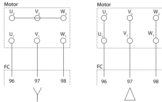
그림 3.34 스타 연결형 및 델타 연결형 연결 방법
