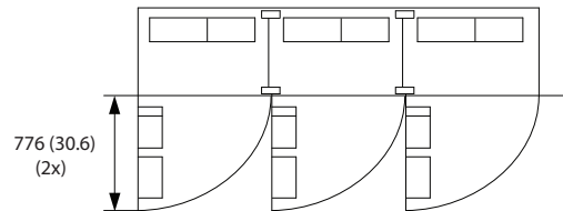
그림 3.8 외함 용량 F11 전면의 여유 공간
