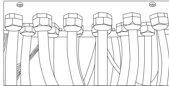
그림 3.23 글랜드 플레이트의 올바른 설치 예
