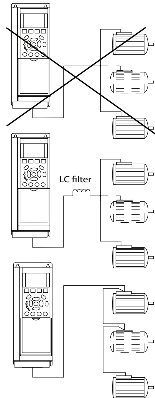
그림 3.61 병렬 모터 연결
