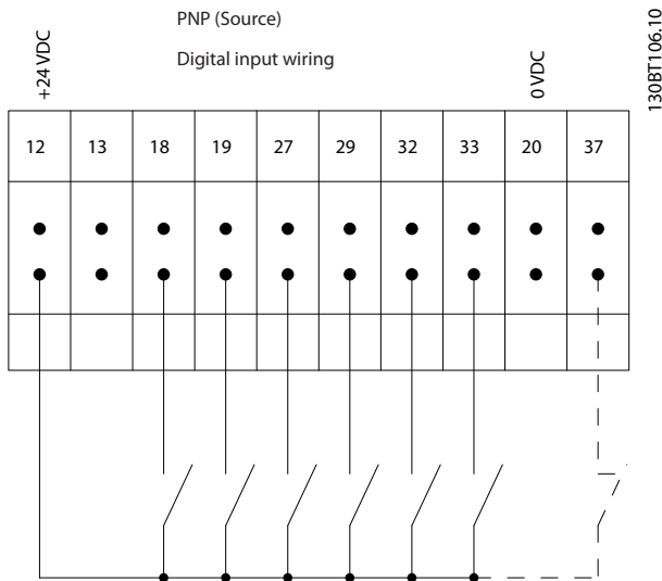
그림 3.52 PNP (소스)
