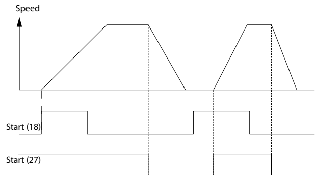
그림 3.57 배선 펄스 기동/정지
