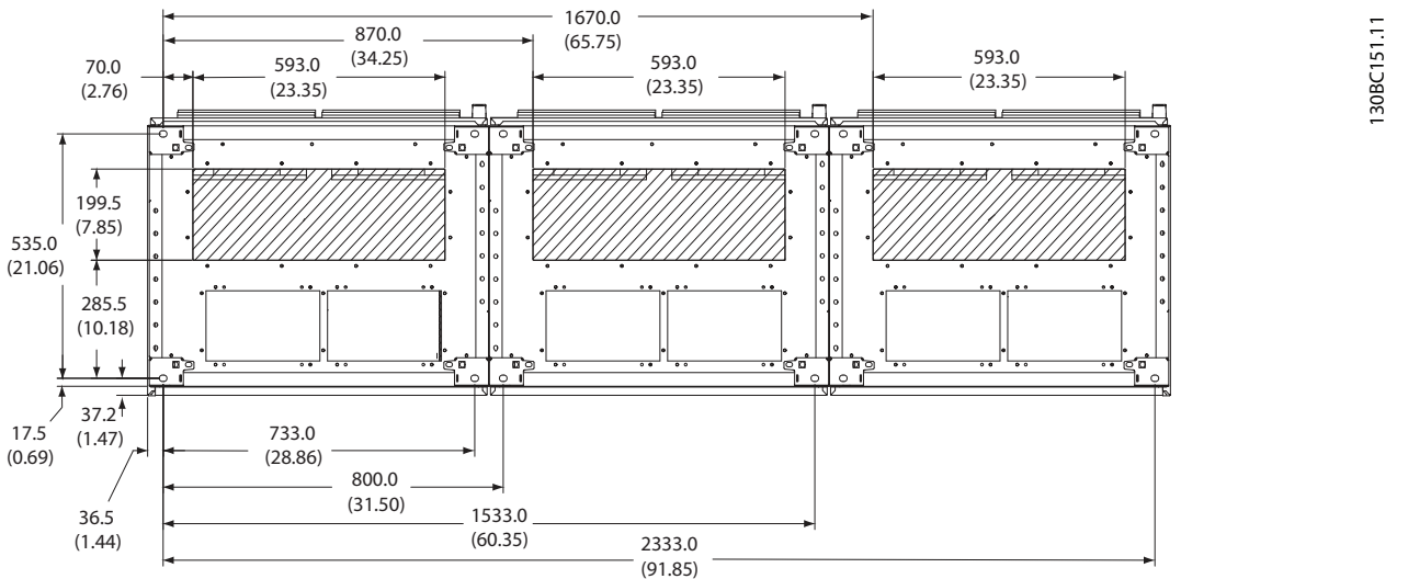
그림 3.30 F14, 주파수 변환기 하단에서 본 케이블 입구
