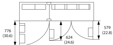
그림 3.9 외함 용량 F12 전면의 여유 공간
