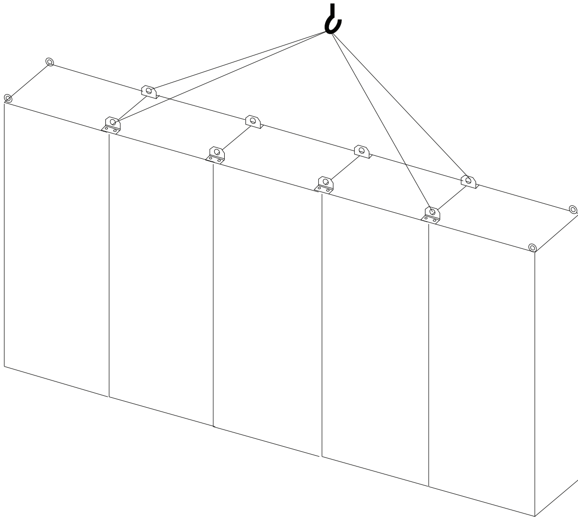
그림 3.4 들어 올리는 방법(권장), 외함 용량 F15
