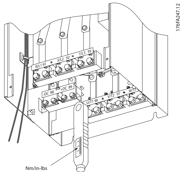
그림 3.44 조임 강도
