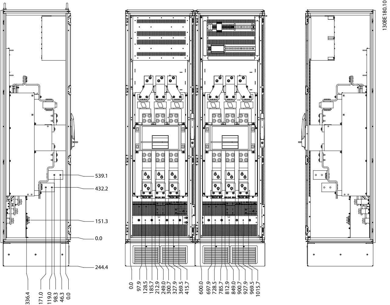
그림 3.21 단자 위치 - 왼쪽, 전면 및 오른쪽 보기
