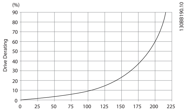
그림 3.22 외함 용량 F, 용량 감소와 압력 변화(Pa) 간 비교 인버터 통풍량: 985 m³/h (580 cfm)
