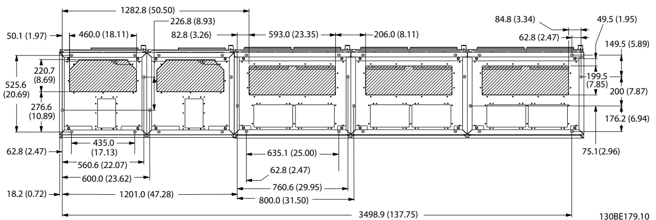
그림 3.31 F15, 주파수 변환기 하단에서 본 케이블 입구
