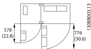
그림 3.6 외함 용량 F9 전면의 여유 공간
