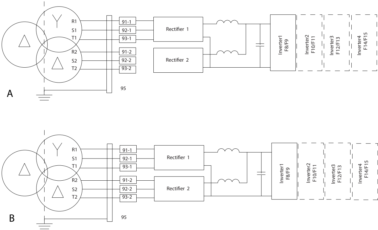
그림 3.33 A) 일시적인 6펄스 연결 1)
