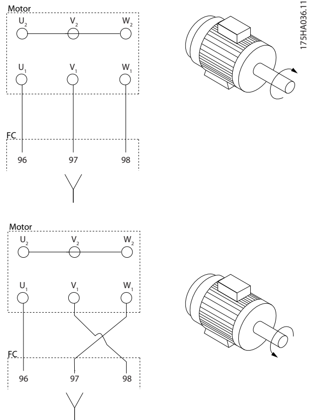
그림 3.45 시계방향 및 반시계방향의 모터 회전 배선
