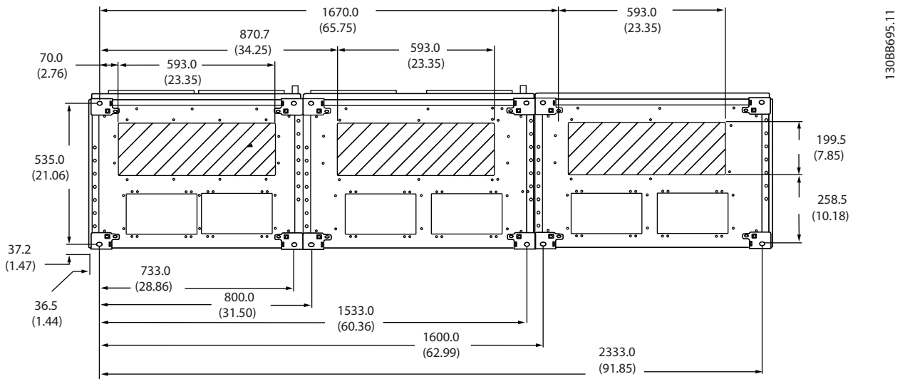
그림 3.27 F11, 주파수 변환기 하단에서 본 케이블 입구
