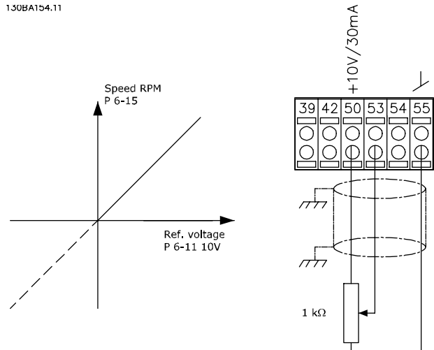
그림 3.59 가변 저항 지령
