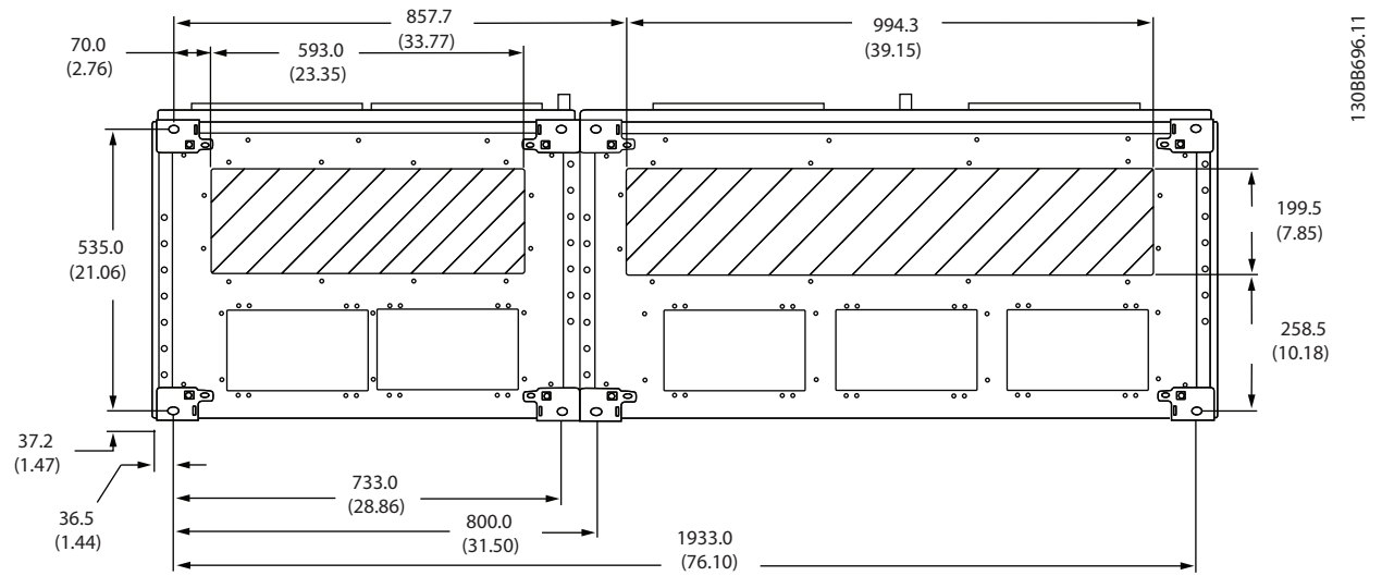
그림 3.28 F12, 주파수 변환기 하단에서 본 케이블 입구
