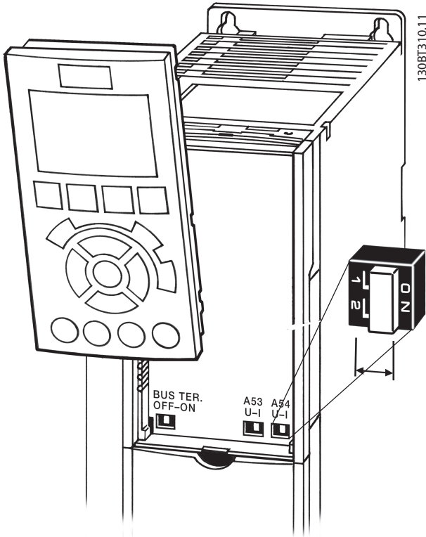
그림 3.55 스위치 위치
