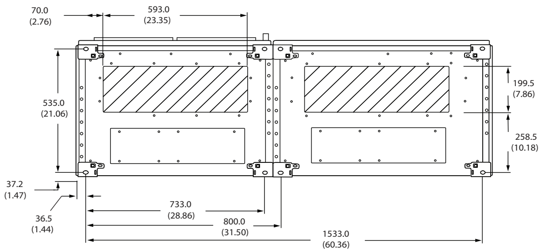
그림 3.26 F10, 주파수 변환기 하단에서 본 케이블 입구
