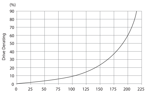
图 3.22 机箱规格 F，降容与压力变化的关系 (Pa) 变频器气流：985 m 3 /h (580 cfm)
