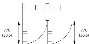
图 3.7 F10 机箱规格前方的空间
