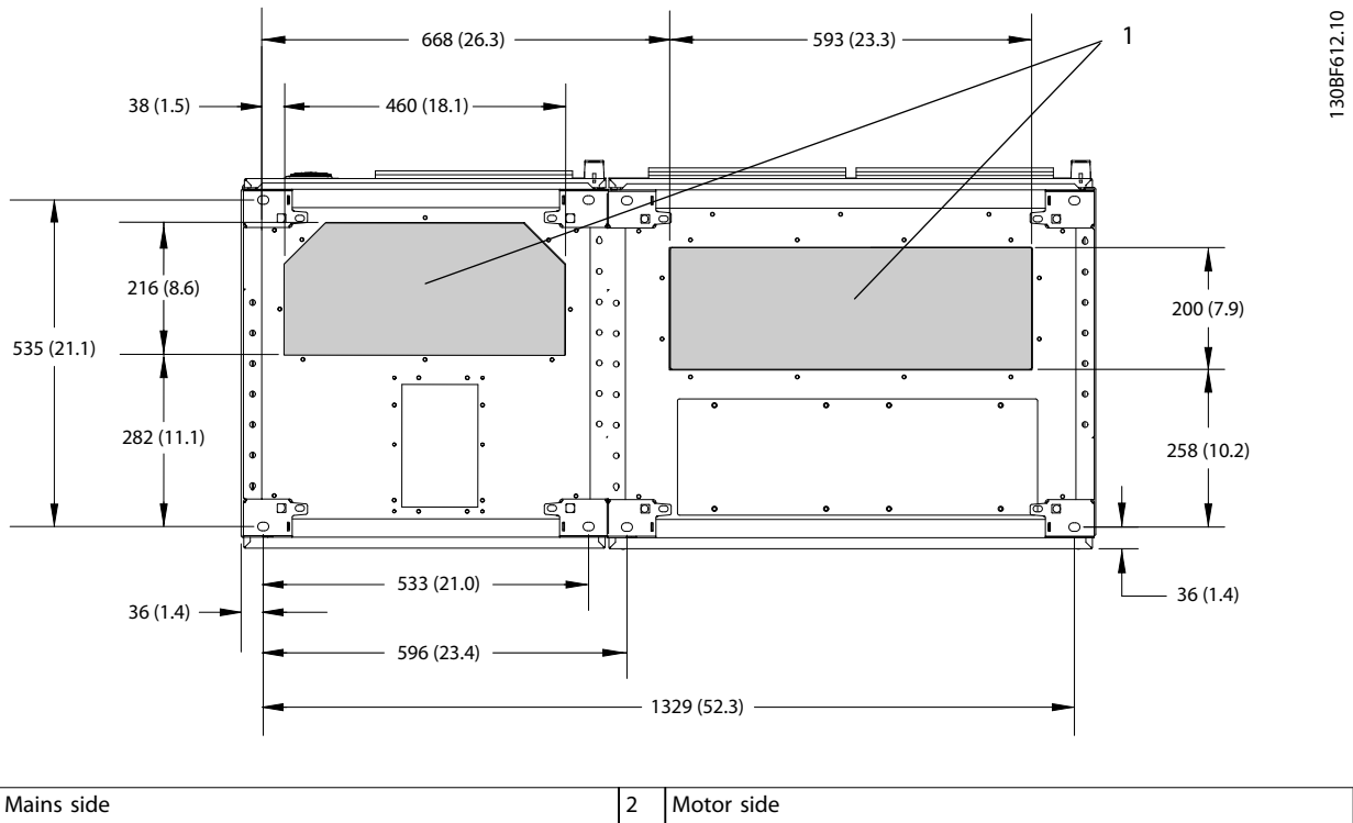
Figure 8.20 Gland Plate Dimensions for F1
