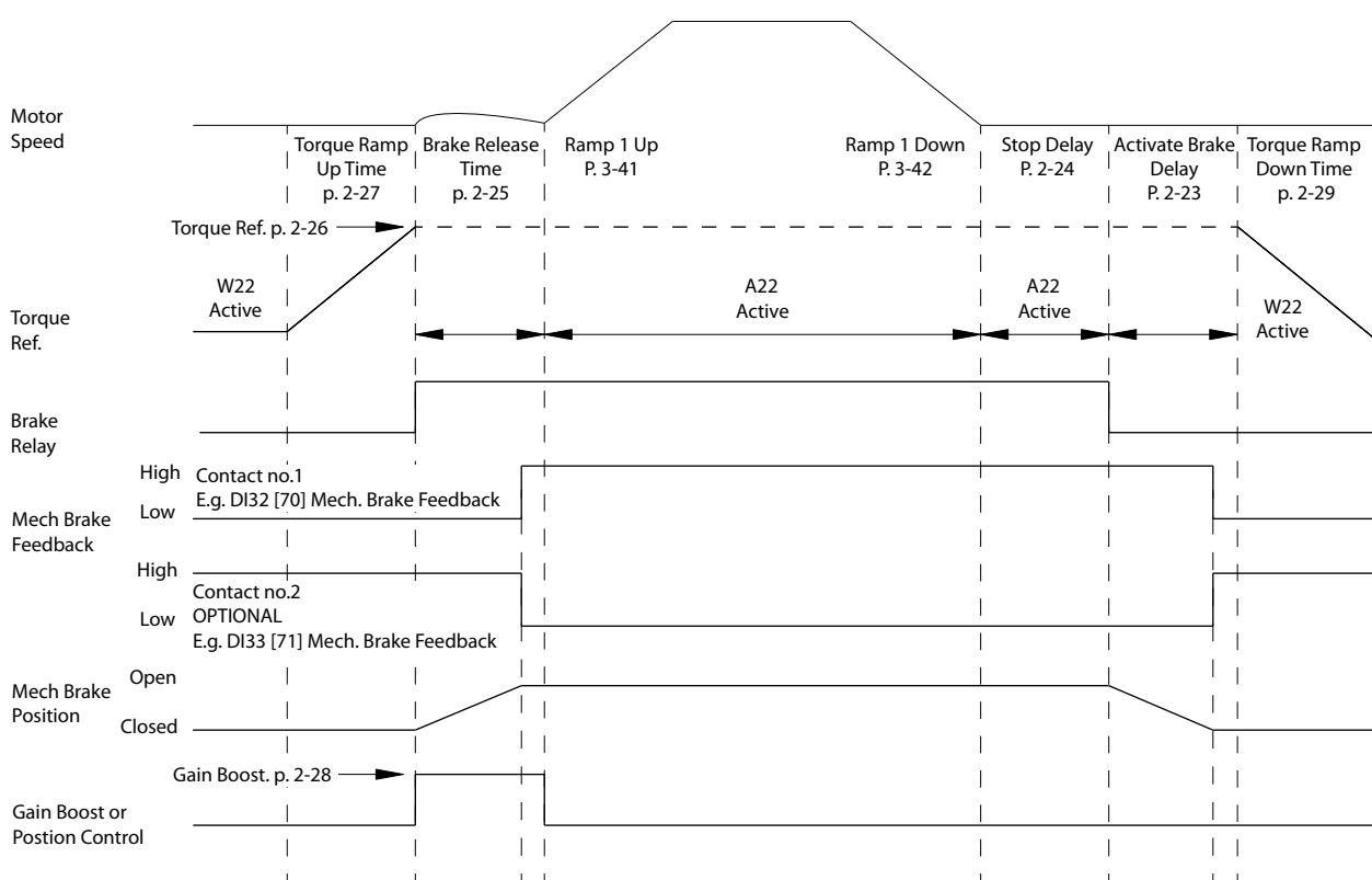
图 5.8 起重机械制动控制的抱闸释放过程
