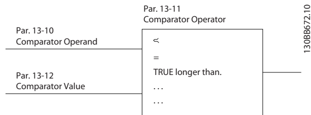
图 5.5 比较器
