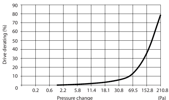
图 9.6 以下机箱随压力变化发生的降容：E1 - E2 机箱 380 - 500 V 型号：P315 - P400 和 525 - 690 V 型号：P500 - P560。气流：850 cfm (1445 m 3 /h)
