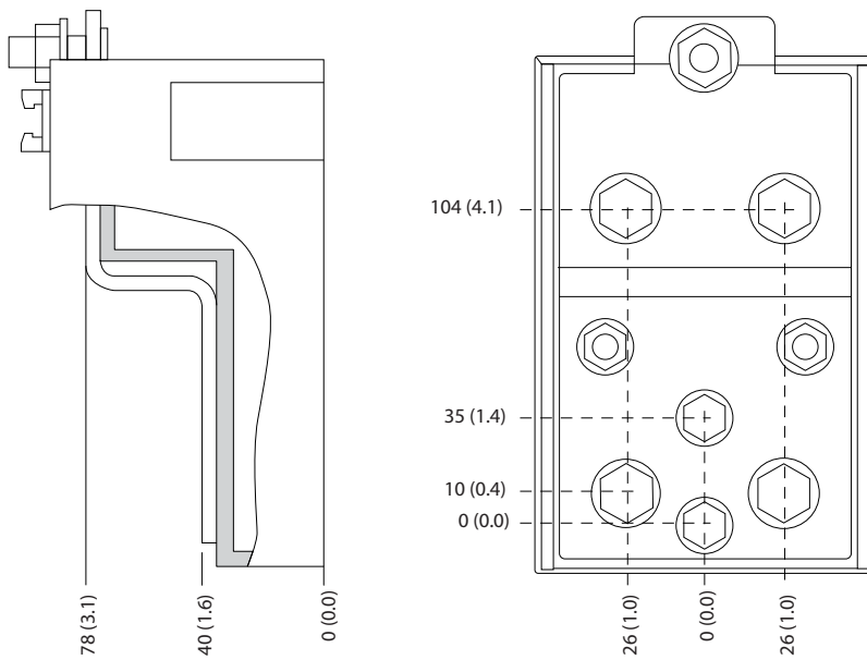
图 8.3 E1/E2 的详细端子尺寸
