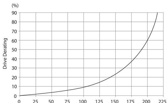
图 9.7 以下机箱随压力变化发生的降容：F1 - F4 机箱。气流：580 cfm (985 m 3 /h)
