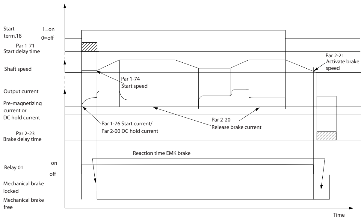
图 5.7 开环中的机械制动控制
