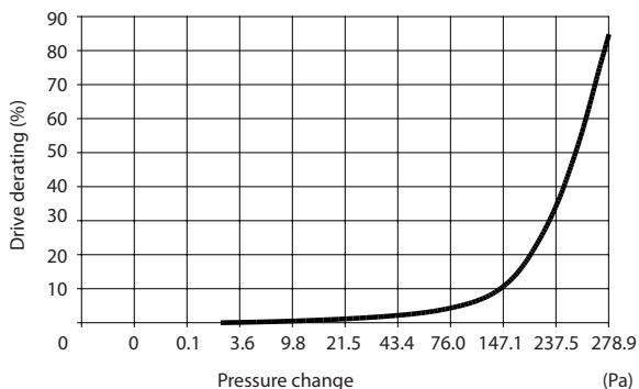
图 9.5 以下机箱随压力变化发生的降容：E1 - E2 机箱 380 - 500 V 型号：P250 和 525 - 690 V 型号：P355 - P400。气流：650 cfm (1105 m 3 /h)
