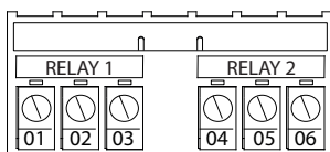
图 10.13 继电器 1 和继电器 2 端子
