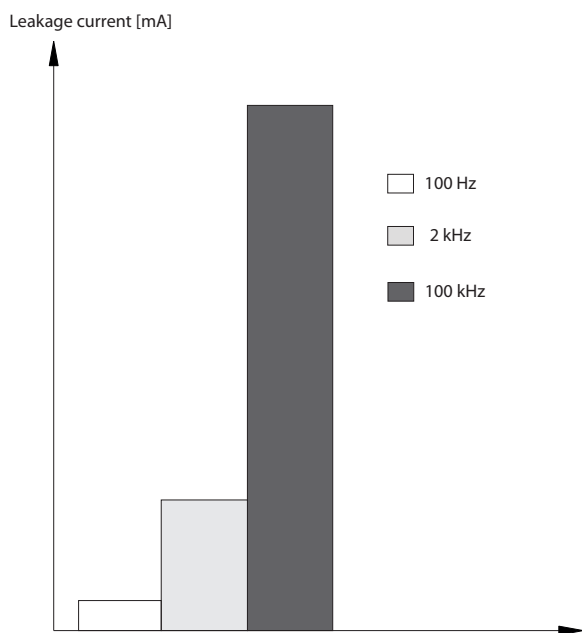
图 10.25 RCD 截止频率对漏电流的影响
