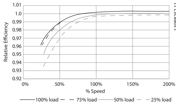
图 10.26 典型效率曲线
