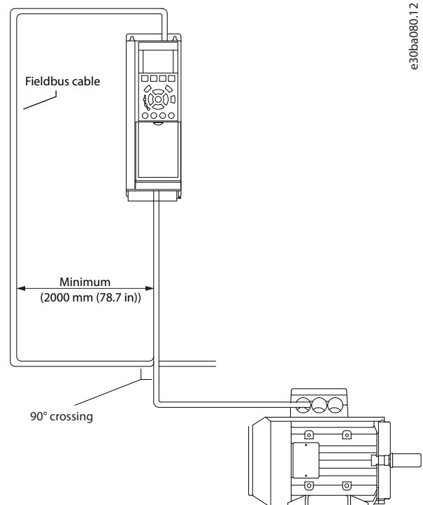
Рисунок 14.4 Обеспечение ЭМС
