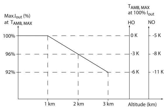
Рисунок 9.8 Снижение выходного тока в зависимости от высоты над уровнем моря при температуре окружающей среды T_{AMB,MAX}
