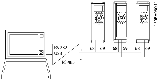
Рисунок 14.2 Параллельные соединения
