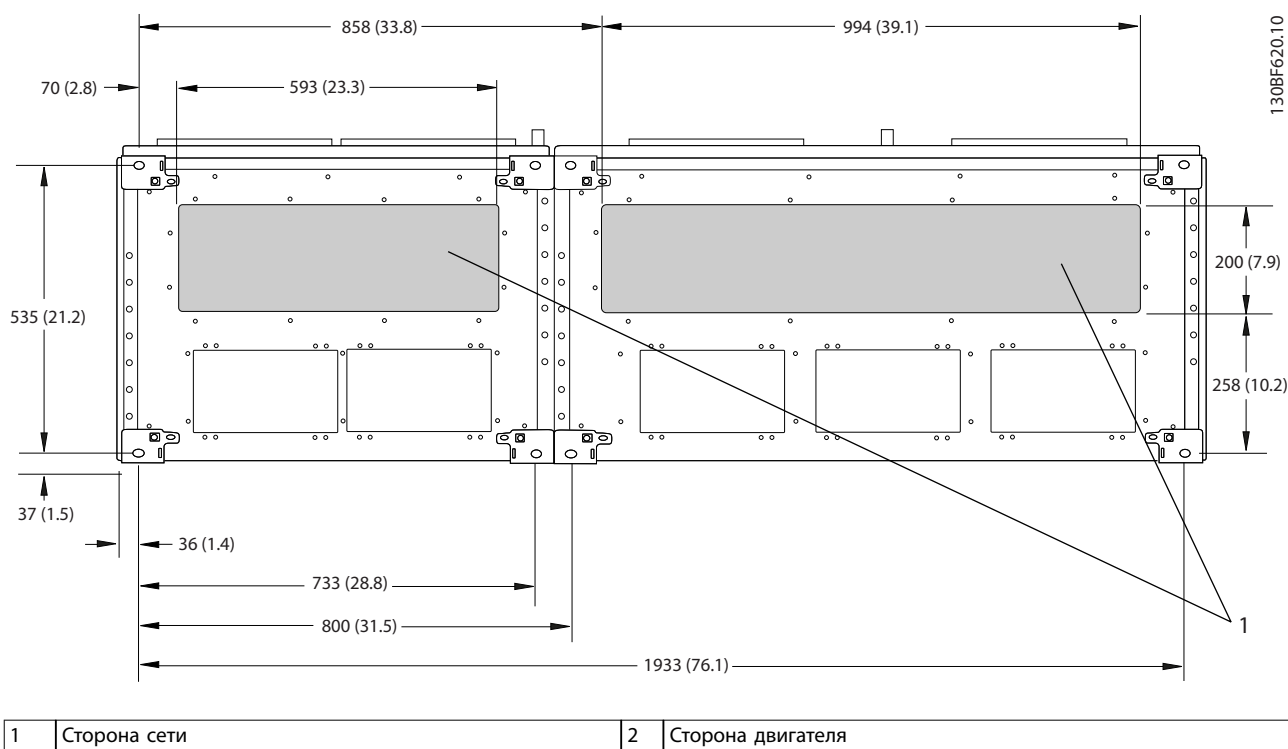
Рисунок 8.81 Размеры панели уплотнений для F12
