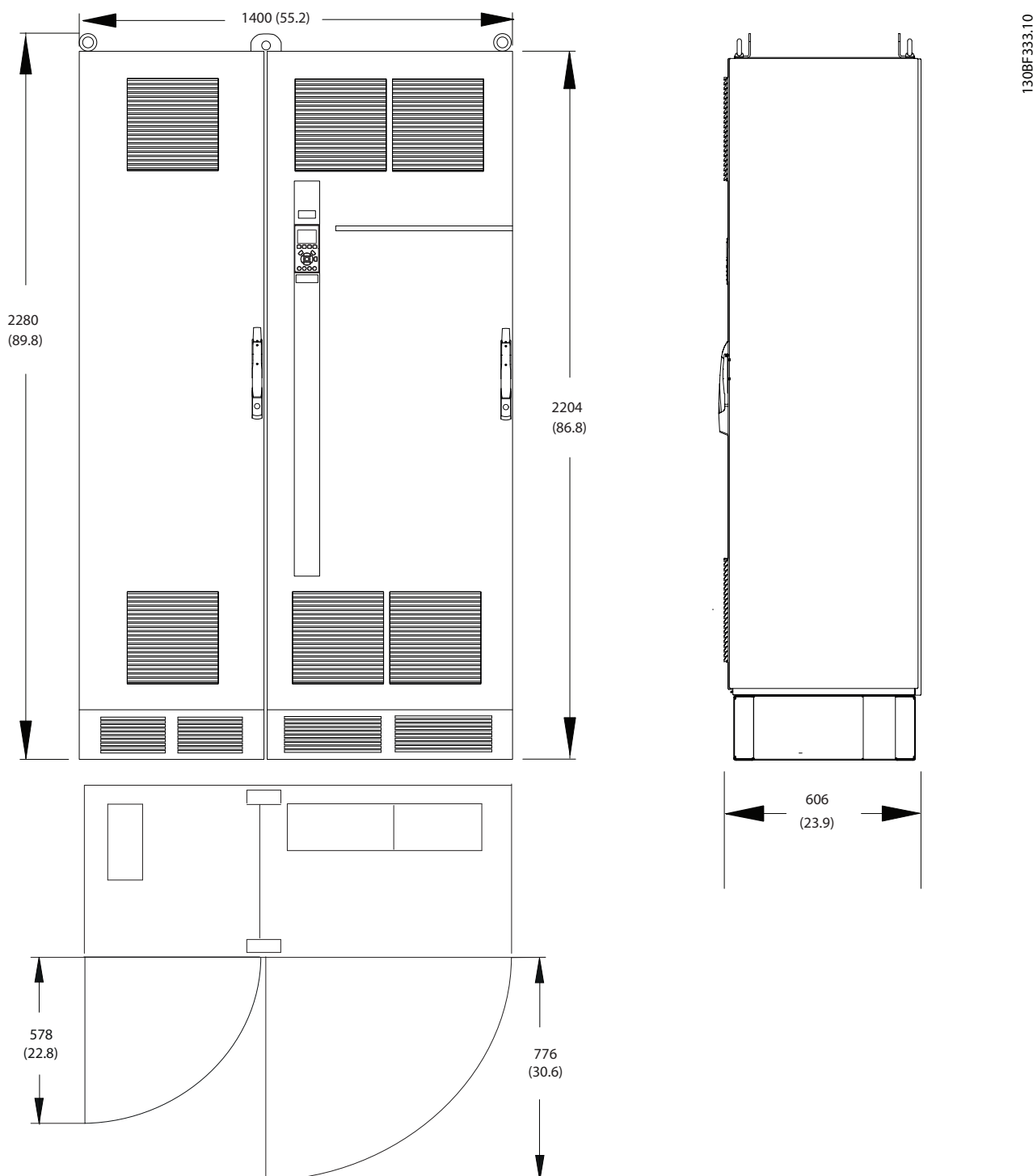
Рисунок 8.60 Размеры зазоров спереди, сбоку и пространство для открытия дверей для F9
