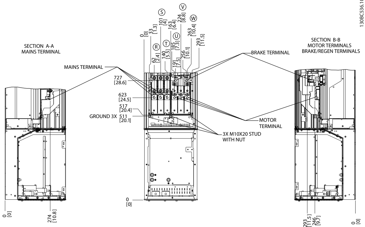
圖 2.14 端子位置，含煞車選項的 D5h
