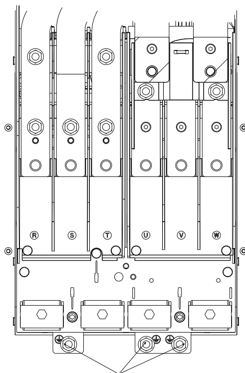
圖 2.5 IP20 (底架) 外殼的接地點
