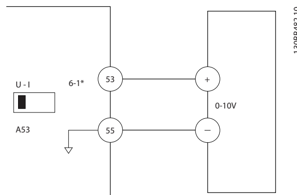
圖 5.10 提供 0-10V 控制信號之外部裝置的線路範例
