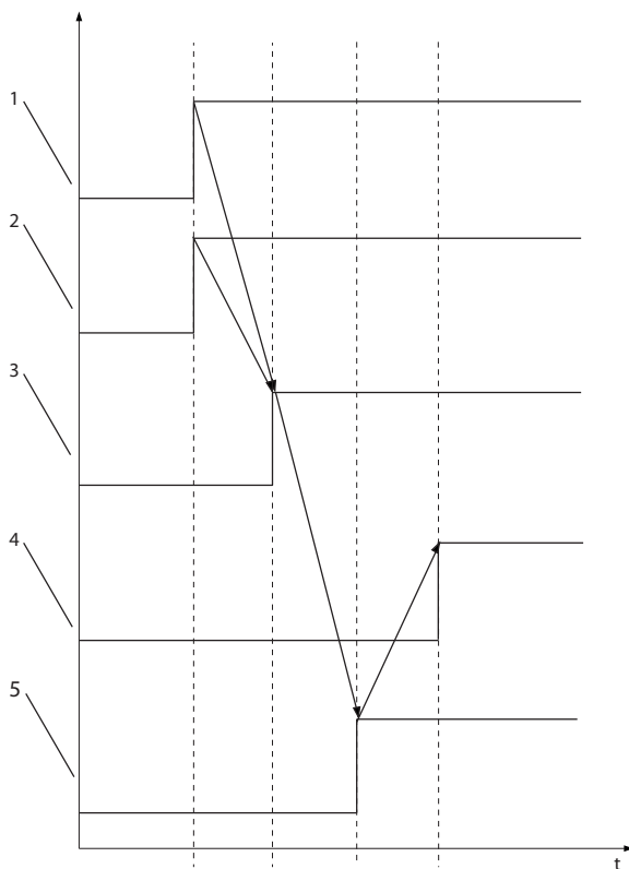
Abbildung 11.8 19-86 Enable Simple Control=[1] (Einfache Steuerung aktivieren=[1])
