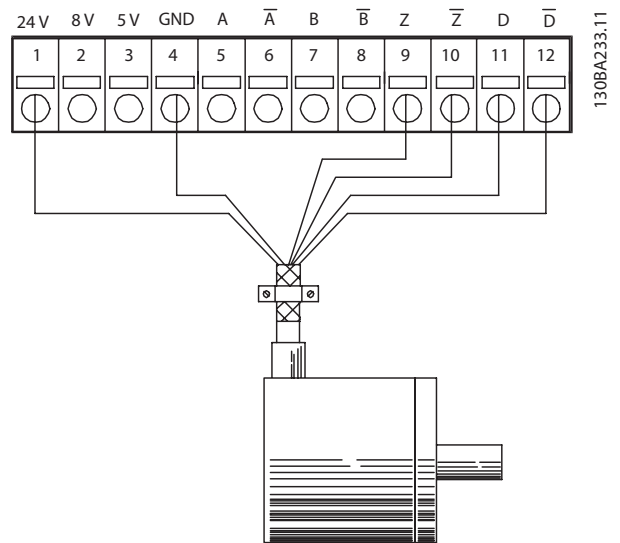
Abbildung 9.6 24-V-Inkrementalgeber (SSI), versorgt über eine externe Stromquelle
