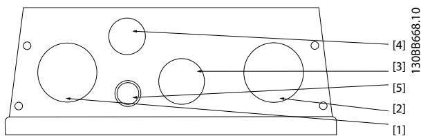
Abbildung 4.6 B1 (IP55) Geschraubte Kabeleinführungsöffnungen
