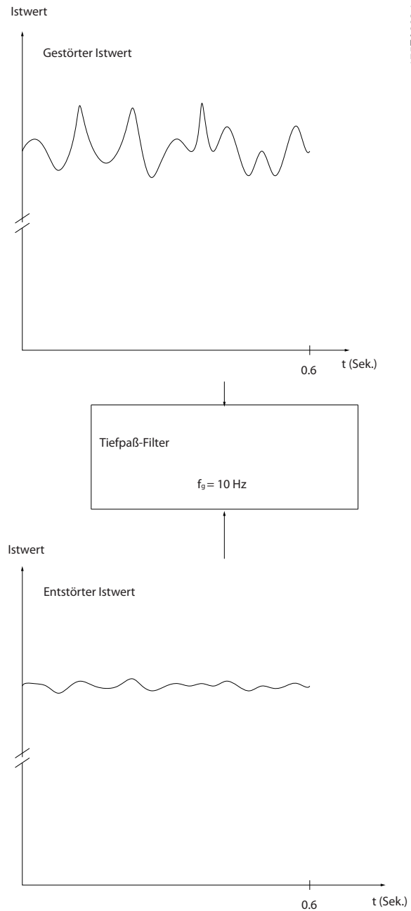
Abbildung 11.3 Istwert-Filterung durch Tiefpassfilter
