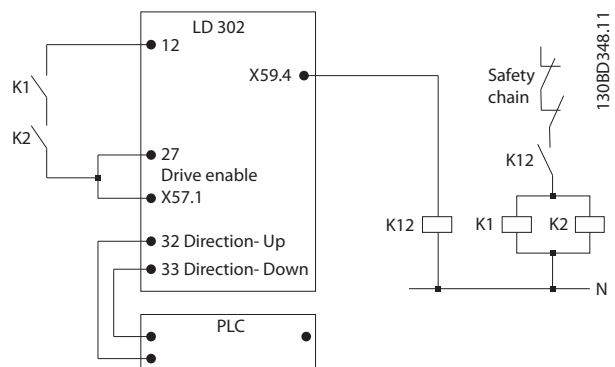
Abbildung 11.7 19-86 Enable Simple Control=[1] (Einfache Steuerung aktivieren=[1])
