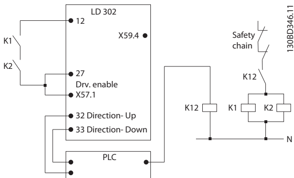
Abbildung 11.5 19-86 Enable Simple Control=[0] (Einfache Steuerung aktivieren=[0])
