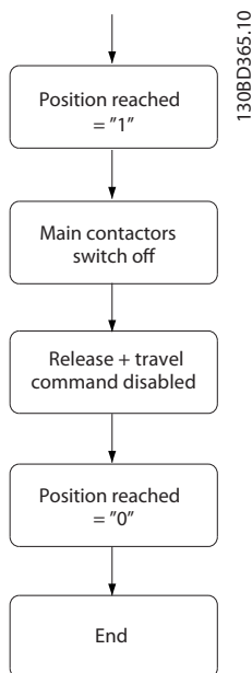
Abbildung 9.2 Hauptschütze Strom aus
