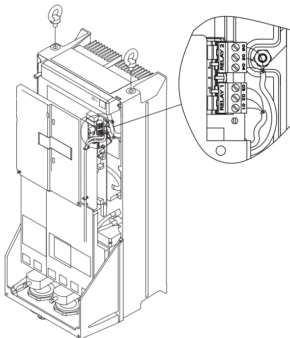
Abbildung 4.26 Klemmen für Relaisanschluss (Gehäusetypen C1 und C2)
