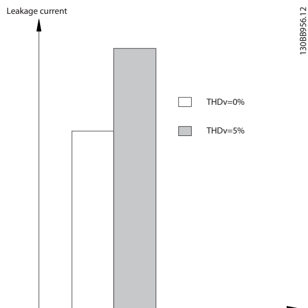
Abbildung 4.12 Die Netzverzerrung beeinflusst den Ableitstrom
