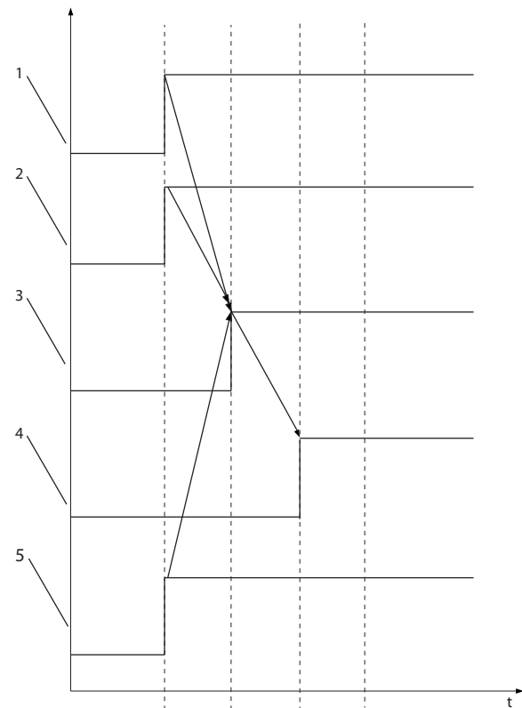
Abbildung 11.6 19-86 Enable Simple Control=[0] (Einfache Steuerung aktivieren=[0])
