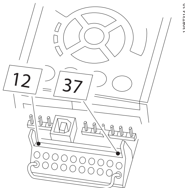
Abbildung 4.32 Drahtbrücke zwischen Klemme 37 und 12, 24 V DC.
