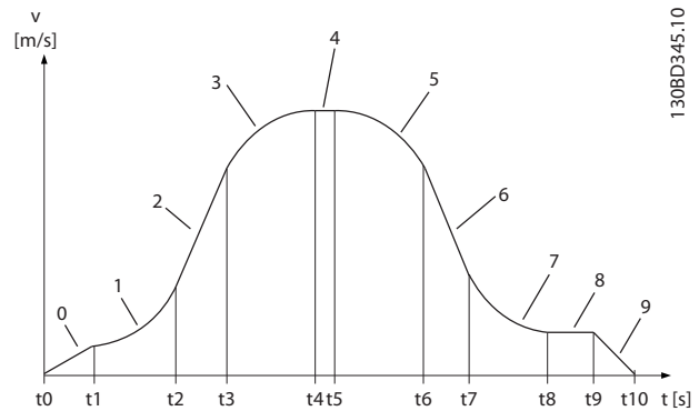
Abbildung 11.1 Rampenparameter für Beschleunigung, Verzögerung und Ruck
