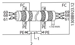
Abbildung 4.31 Kabel mit verdrehten Aderpaaren
