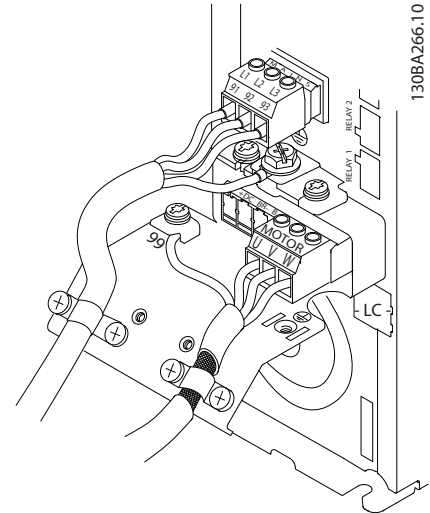
Abbildung 4.15 Erdung mit abgeschirmtem Kabel
