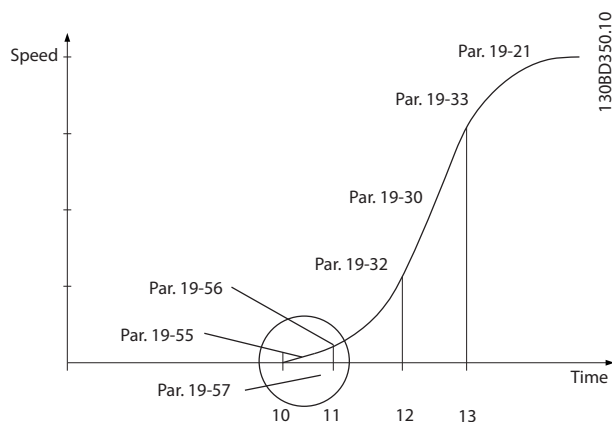
Abbildung 11.4 Lineare Startzeit
