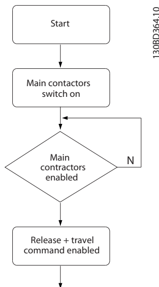
Abbildung 9.1 Hauptschütze Strom ein
