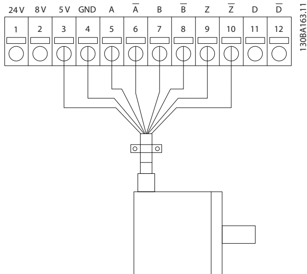
Abbildung 9.4 5 V Inkrementalgeber (RS-422), versorgt über MCO 361
