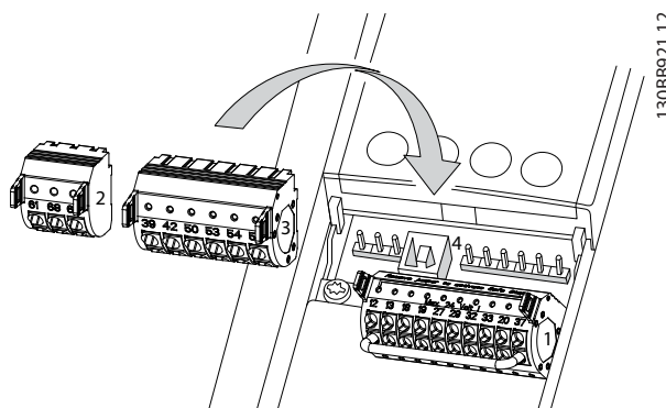
Abbildung 4.22 Anordnung der Steuerklemmen
