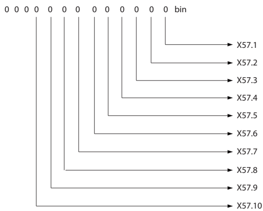
Abbildung 5.8 LCP-Display, Statusklemme X.57
