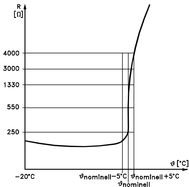
Abbildung 10.2 Thermistoreingang
