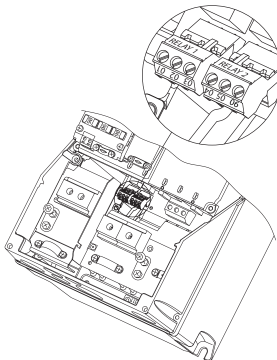
Abbildung 4.25 Klemmen für Relaisanschluss (Gehäusetypen A5, B1 und B2)
