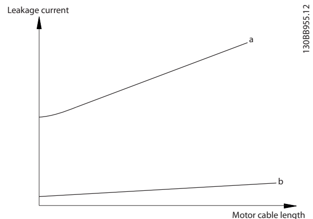
Abbildung 4.11 Einfluss von Kabellänge und Leistungsgröße auf Ableitstrom. Pa > Pb.
