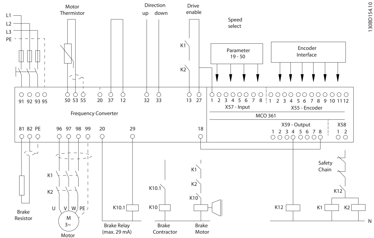
Abbildung 4.17 Anschlussdiagramm mit Schützen
