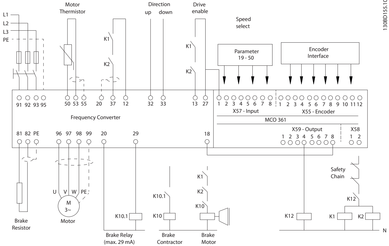
Abbildung 4.18 Anschlussdiagramm ohne Schütze
