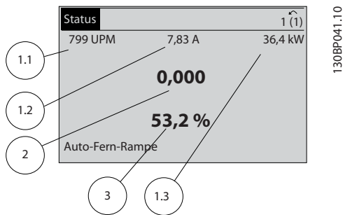
Abbildung 5.2 Beispiel mit allen Displayzeilen
