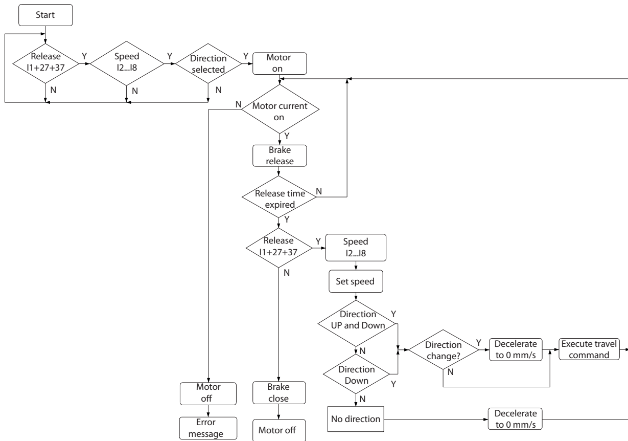
Abbildung 6.1 Startsequenz der Aufzugssteuerung
