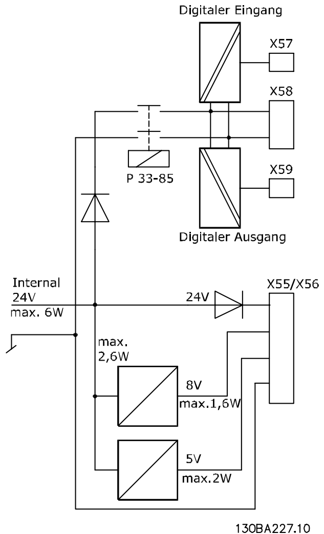
Abbildung 12.3 Anschlussplan – Versorgungsspannung
