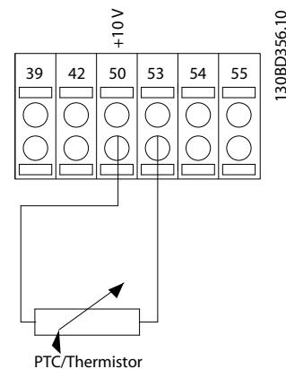
Abbildung 10.1 Motorthermistor
