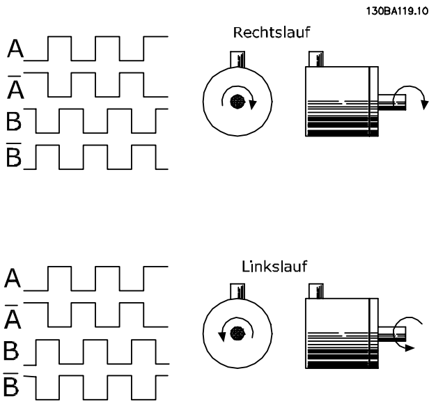
Abbildung 9.3 Drehgeberichtung
