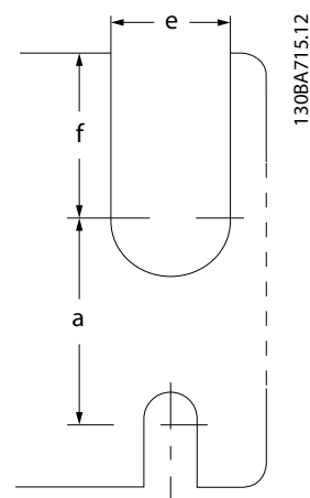
Abbildung 12.2 Obere und untere Befestigungsbohrungen (nur B4)
