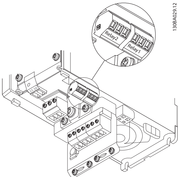
Abbildung 4.24 Klemmen für Relaisanschluss (Gehäusetypen A1, A2 und A3)
