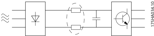
Abbildung 4.10 Zwischenkreisdrosseln
