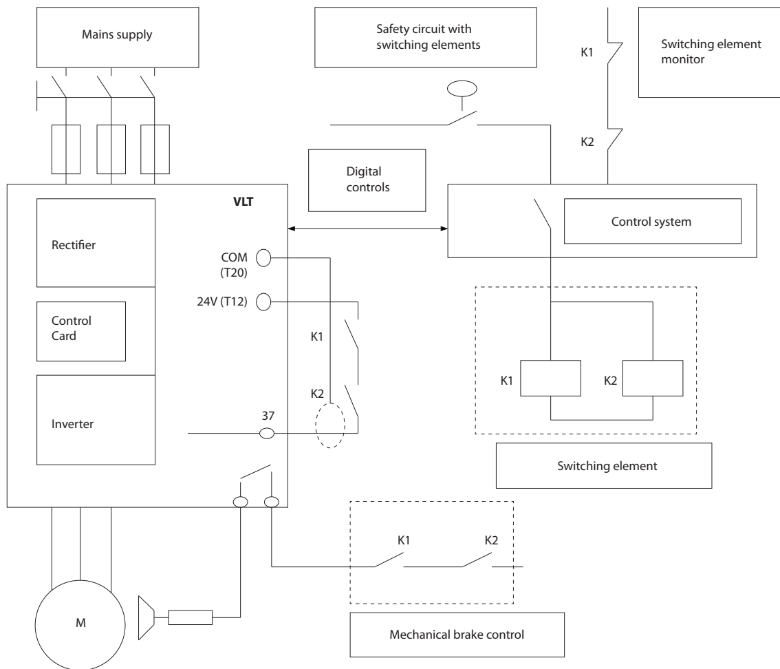
Abbildung 4.33 Verdrahtung in Aufzugsanwendungen
