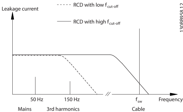
Abbildung 4.13 Hauptbeitragsfaktoren zum Ableitstrom
