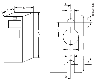
Abbildung 12.1 Bohrungen oben und unten
