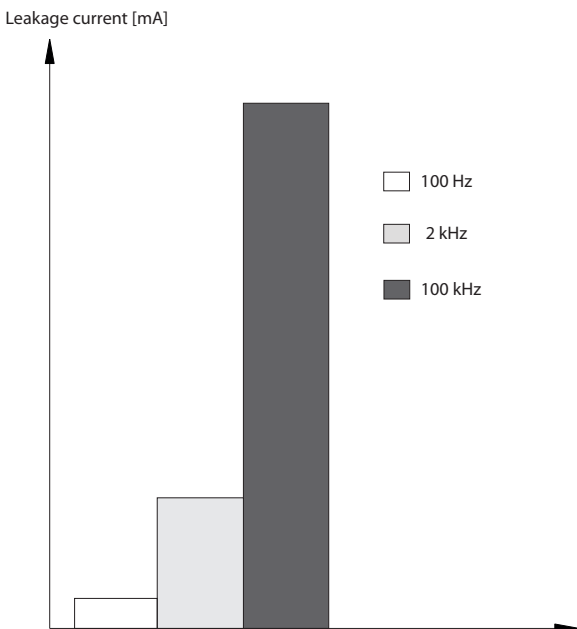
Abbildung 4.14 Einfluss der Trennfrequenz des Fehlerstromschutzschalters
