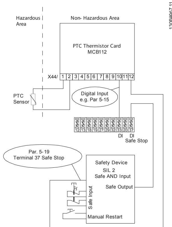
图 3.3 组合应用安全转矩关断与 MCB 112
