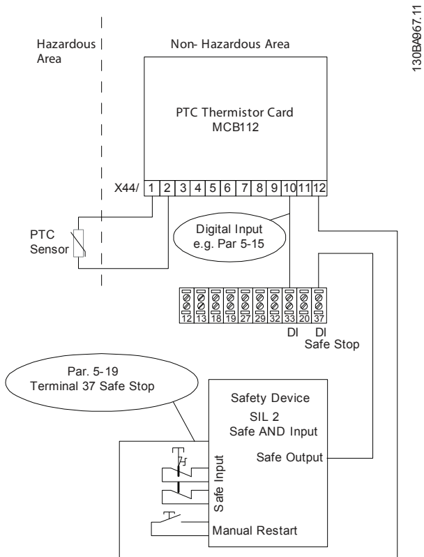
그림 3.3 STO 어플리케이션과 MCB 112 어플리케이션을 함께 사용하는 경우
