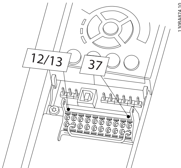
그림 3.1 단자 12/13(24V)과 37 간의 점퍼
