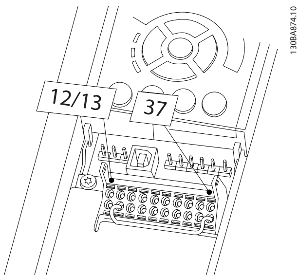
Ilustracja 3.1 Zworka pomiędzy zaciskami 12/13 (24 V) i 37
