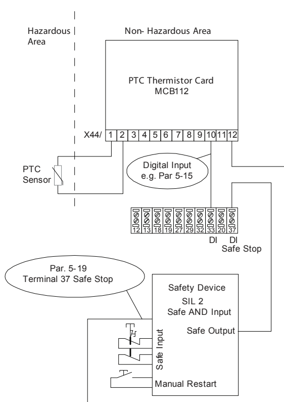
Ilustracja 3.3 Połączenie aplikacji bezpiecznego wyłączenia momentu z kartą MCB 112
