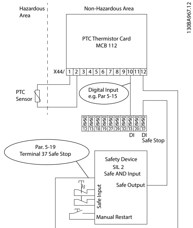
Illustration 3.4 Kombinationen af STO-applikationen og en MCB 112-applikation
