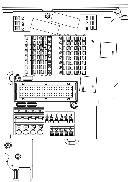
Illustration 3.2 Forbindelse mellem klemmerne 13 (24 V) og 37 (FCD 302)
