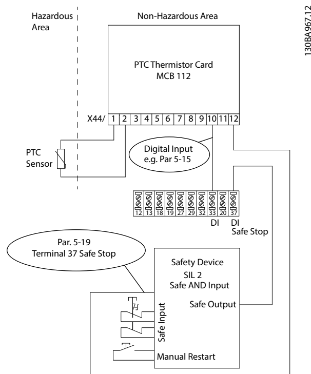
Kuva 3.4 STO-sovelluksen ja MCB 112 -sovelluksen yhdistelmä
