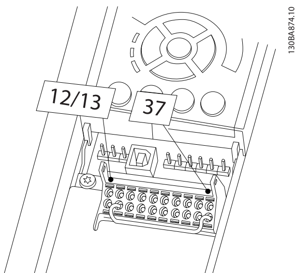
Kuva 3.1 Hyppyjohdin liitinten 12/13 (24 V) ja 37 välissä (kaikki taajuusmuuttajat paitsi FCD 302)
