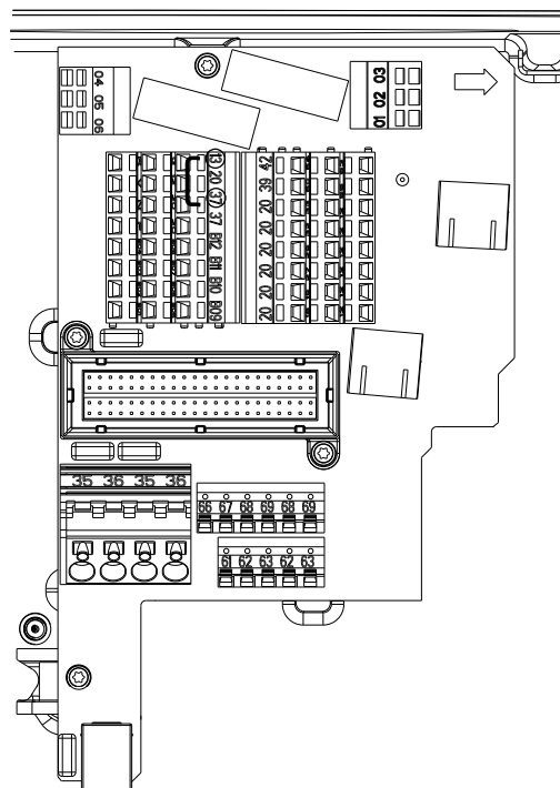
Kuva 3.2 Hyppyjohdin liitinten 13 (24 V) ja 37 (FCD 302) välissä
