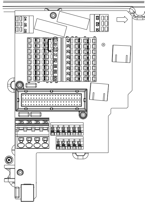
그림 3.2 단자 12/13 (24 V)과 37 간의 점퍼(FCD 302)
