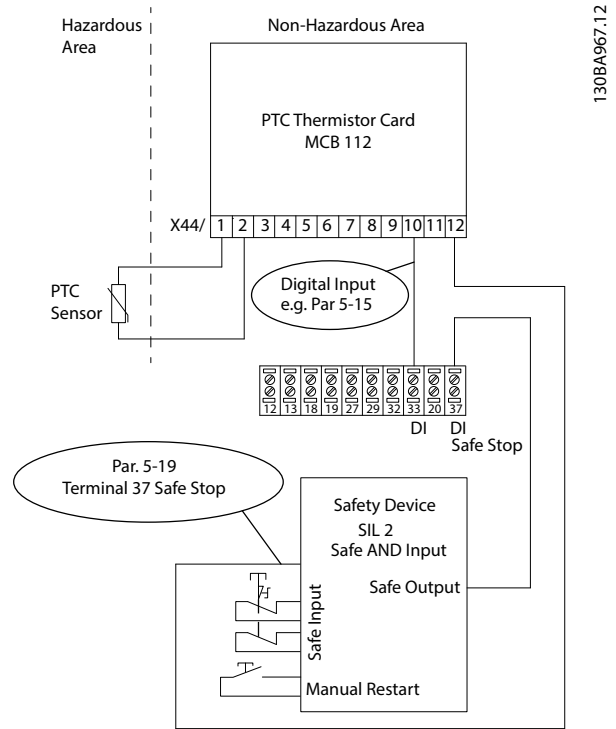
그림 3.4 STO 어플리케이션과 MCB 112 어플리케이션을 함께 사용하는 경우
