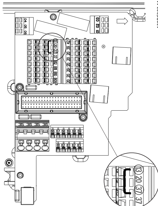
Bild 3.2 Bygel mellan plint 13 (24 V) och 37 (FCD 302)
