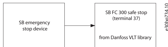
Bild 5.2 Säkerhetsrelaterat blockdiagram
