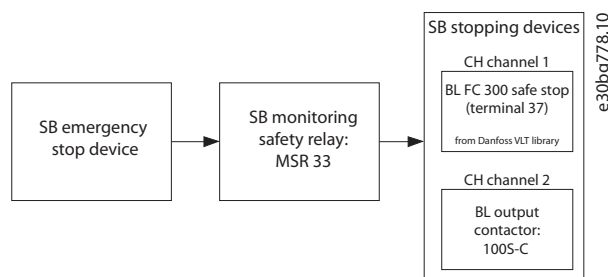
Bild 5.6 Säkerhetsrelaterat blockdiagram
