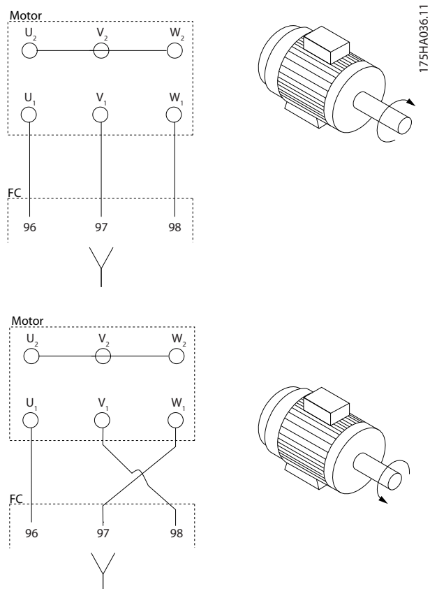
图 5.7 更改电动机旋转情况
