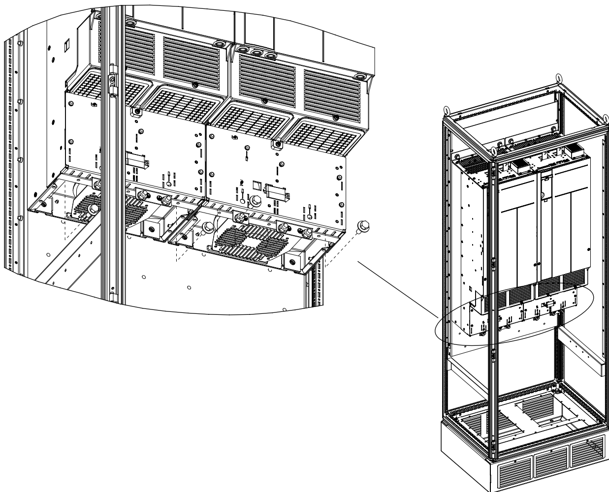
图 4.6 安装底部安装螺栓
