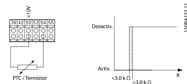
图 5.4 PTC 热敏电阻连接 - 带有 10 V 电源的模拟输入
