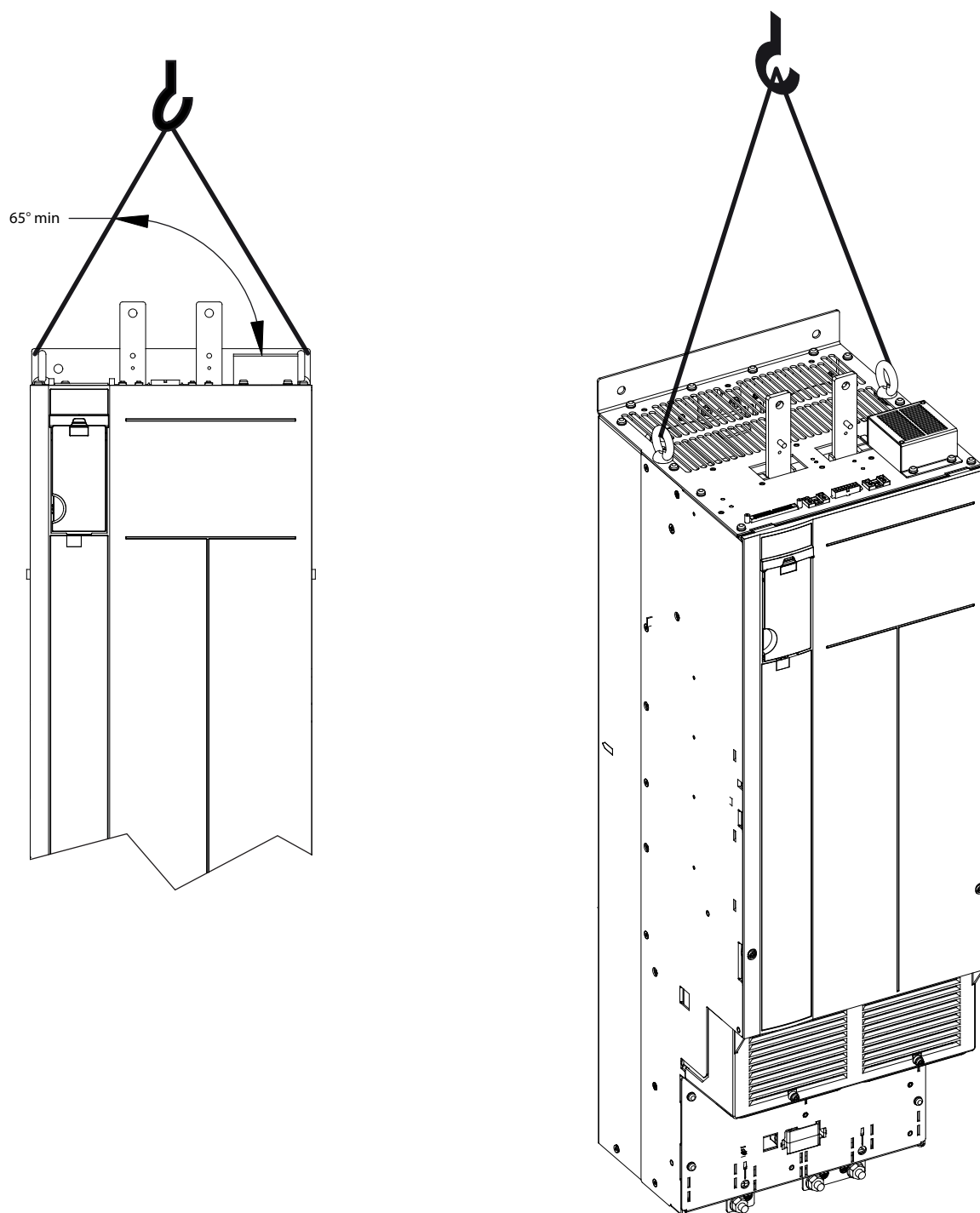
图 4.3 起吊变频器模块
