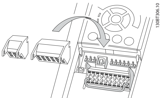
图 5.10 取下控制端子
