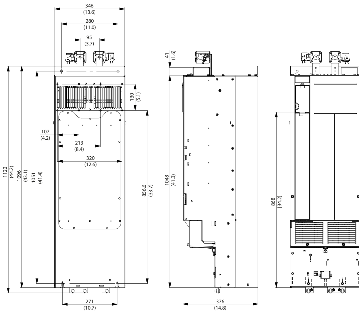
图 7.2 VLT® Parallel Drive Modules 安装尺寸
