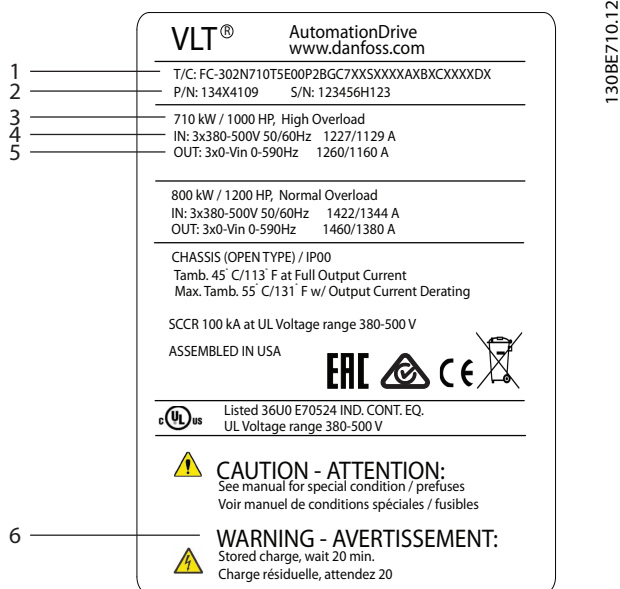
图 4.2 变频器模块铭牌（示例）
