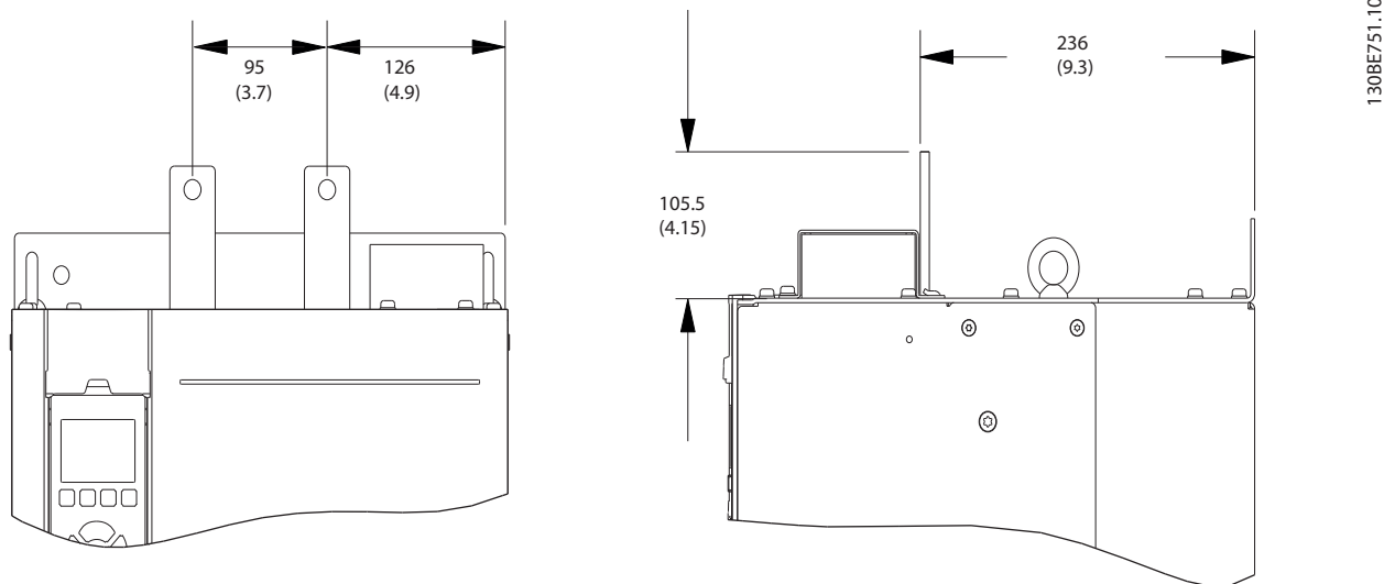
图 7.5 直流母线尺寸（正视图和侧视图）
