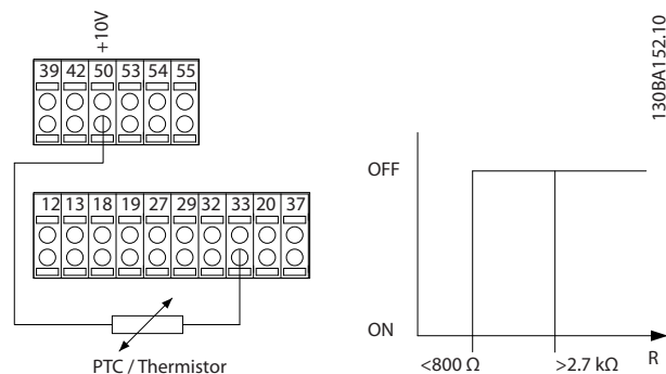
图 5.3 PTC 热敏电阻连接 - 带有 10 V 电源的数字输入
