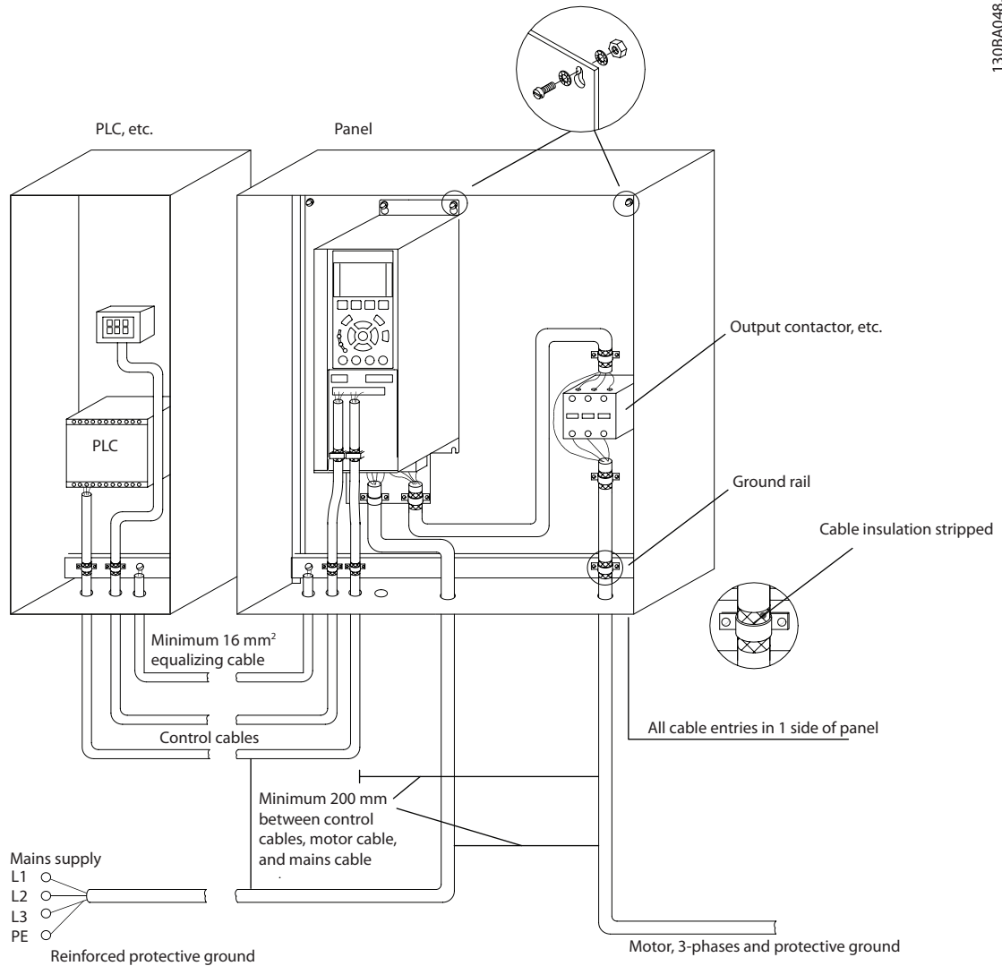
图 5.13 在机柜中对变频器执行符合 EMC 规范的电气安装
