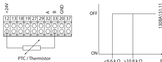
图 5.5 PTC 热敏电阻连接 - 带有 24 V 电源的数字输入
