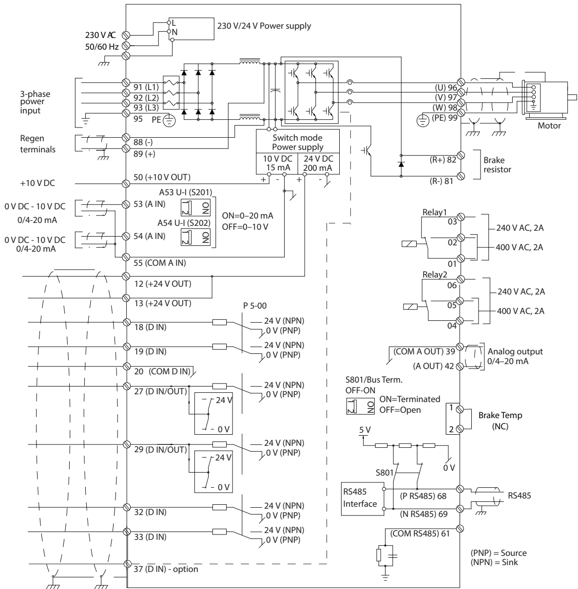
图 5.1 接线图
