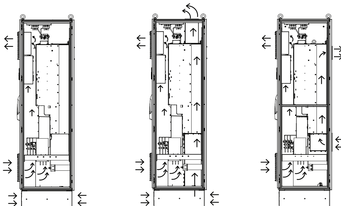
图 4.4 气流：标准单元（左）、底部/顶冷却套件（中）以及背部冷却套件（右）
