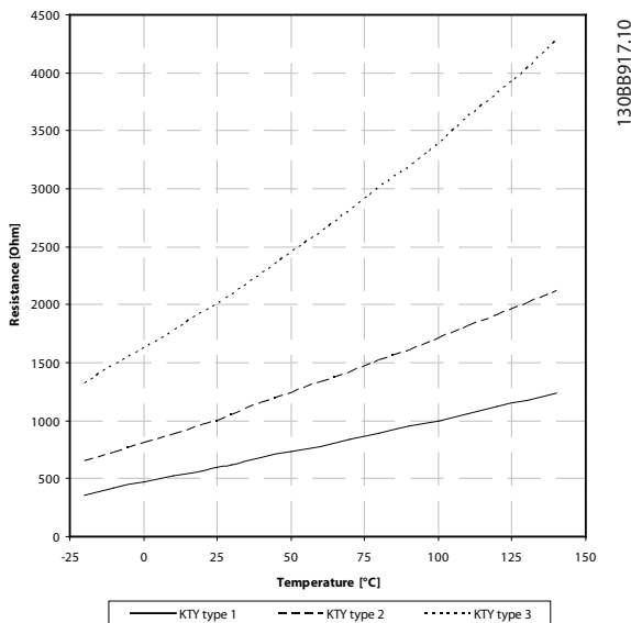
图 5.6 KTY 类型选择
