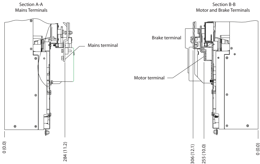
图 7.4 变频器模块端子尺寸（侧视图）
