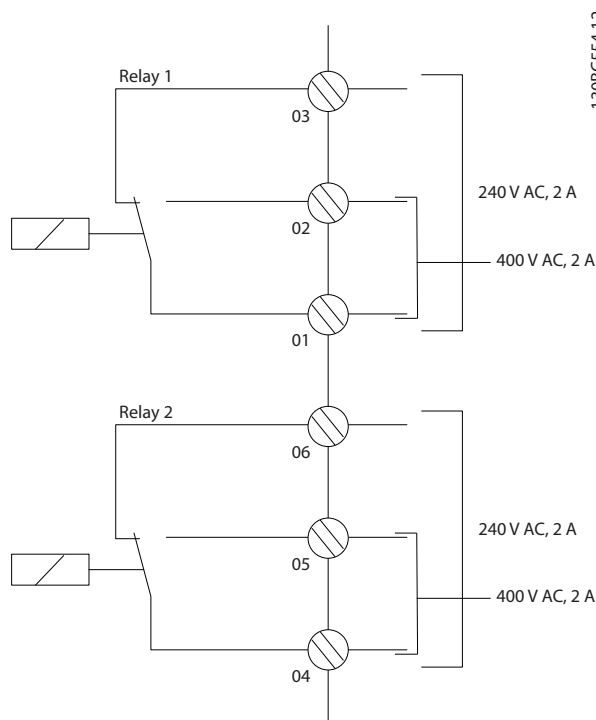
图 5.12 其他继电器输出
