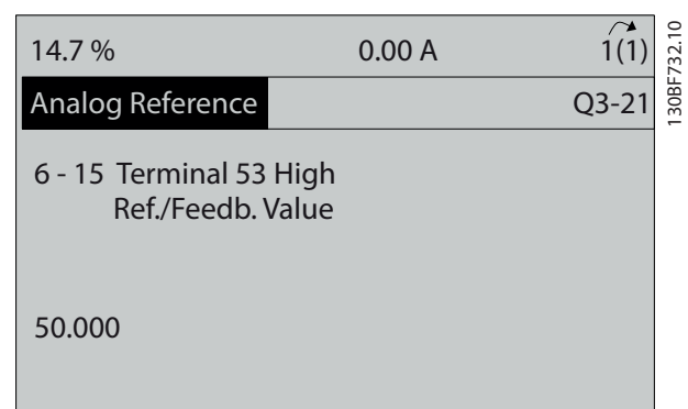
Illustration 6.11 Paramètre 6-15 Val.ret./Réf.haut.born.53
