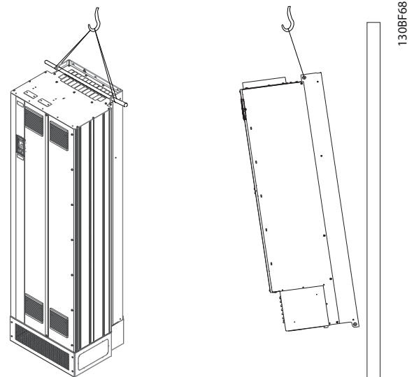
그림 4.2 들어 올리는 방법(권장)
