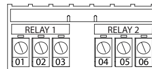
그림 5.19 릴레이 1 및 릴레이 2 단자
