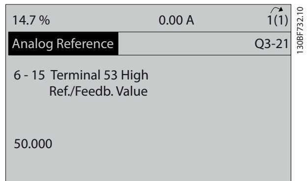
그림 6.11 파라미터 6-15 단자 53 최고 지령/피드백 값
