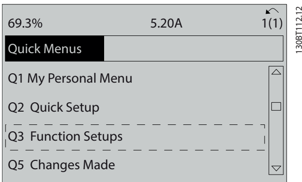
그림 6.3 Q3 기능 셋업
