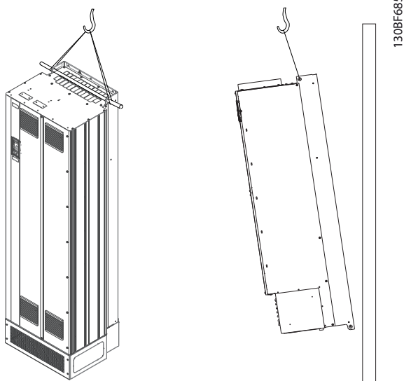
Illustration 4.2 Méthode de levage recommandée
