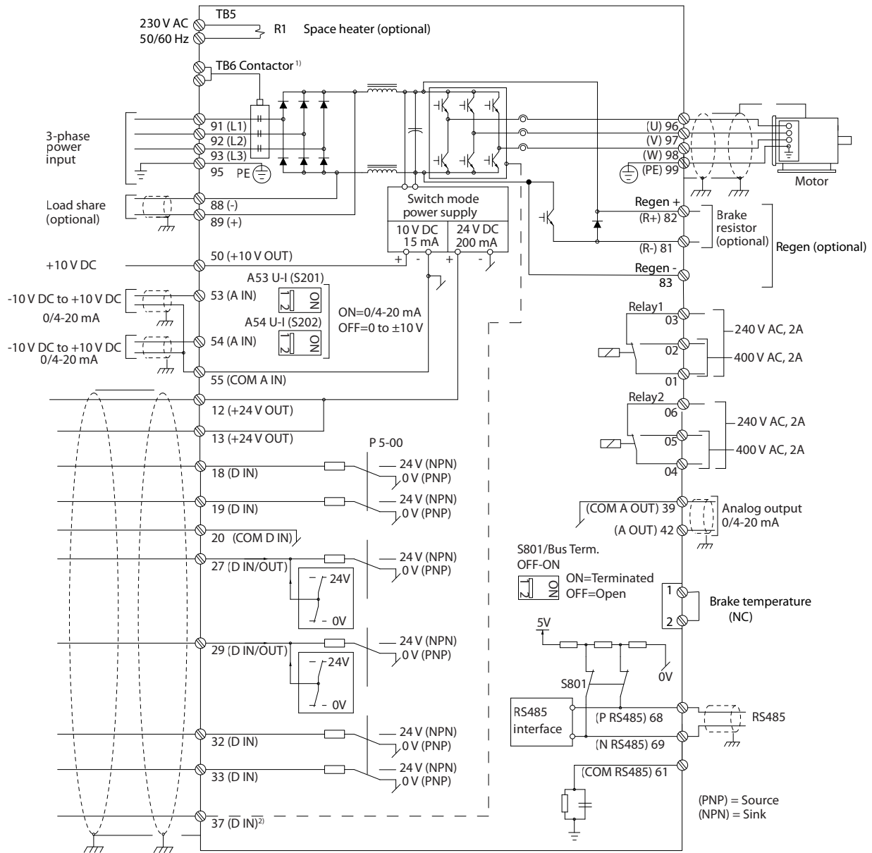
Kuva 5.2 Peruskytkennän kaavio
