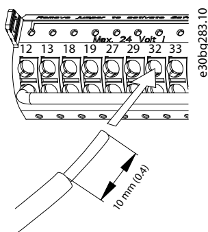
图 5.19 连接硬质控制线缆
