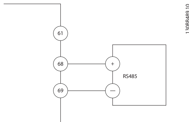
图 5.21 串行通讯接线图
