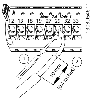
图 5.20 连接软质控制线缆
