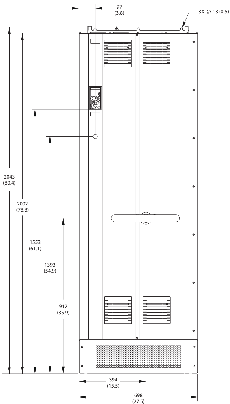
图 9.6 E2h 的正视图
