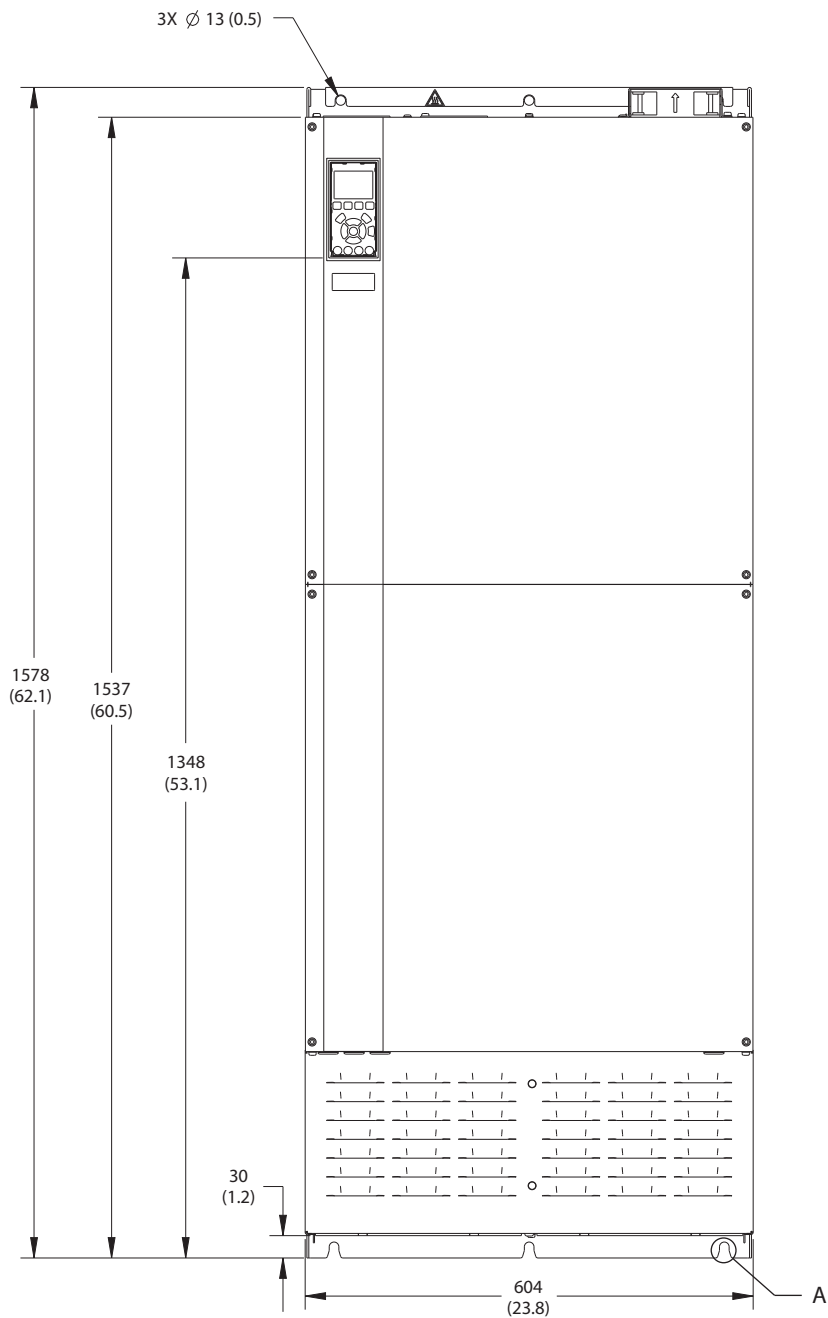
图 9.14 E4h 的正视图
