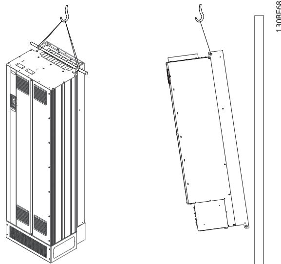
Илюстрация 4.2 Препоръчителен метод на повдигане
