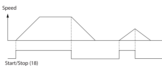
Илюстрация 7.2 Команда пуск/спиране със Safe Torque Off
