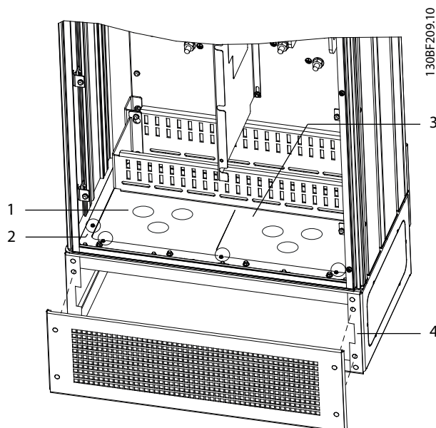
Илюстрация 4.5 Монтажни точки за фиксиране на корпуса към подставката
