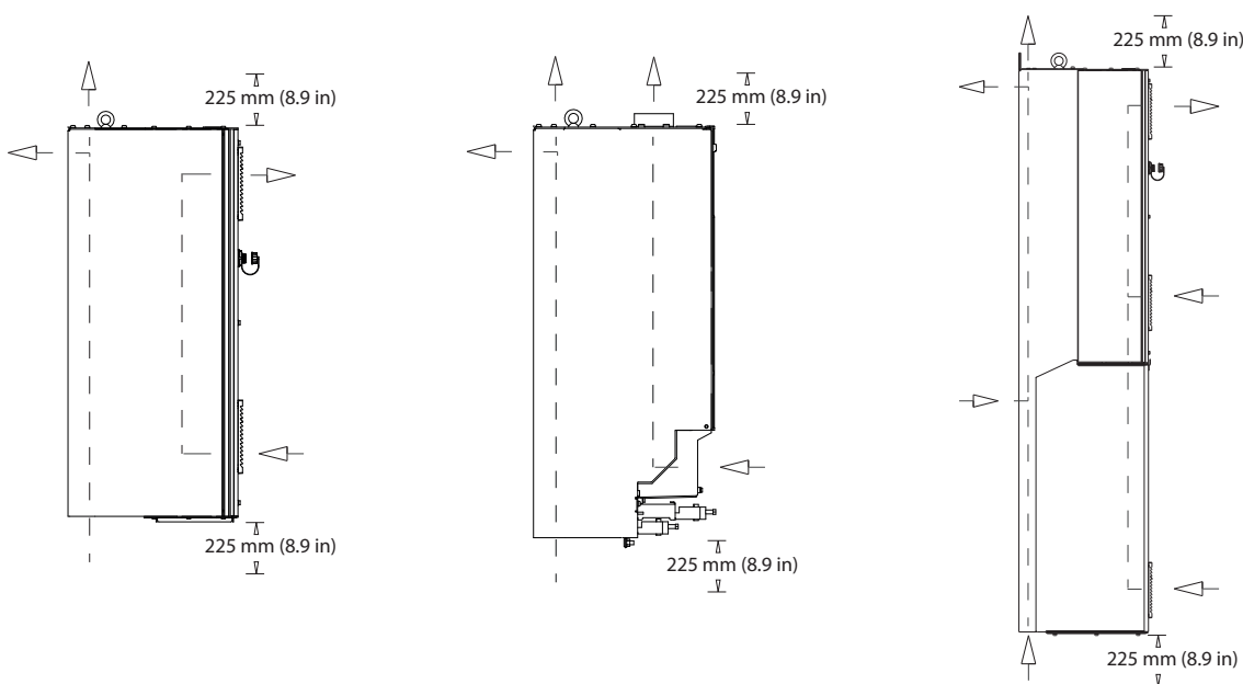
Ilustración 5.10 Configuración estándar del flujo de aire para alojamientos D1h/D2h (izquierda), D3h/D4h (centro) y D5h-D8h (derecha).
