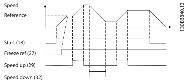
Ilustración 12.4 Aceleración/desaceleración
