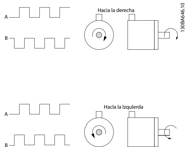
Ilustración 12.6 Determinar la dirección del encoder
