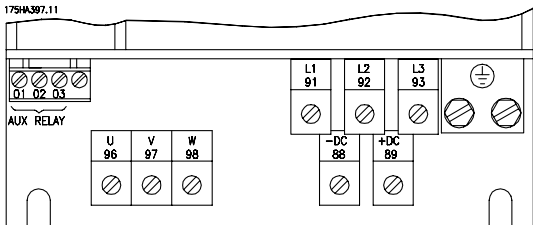
IP 20 VLT 7016-7072, 380-460 V
