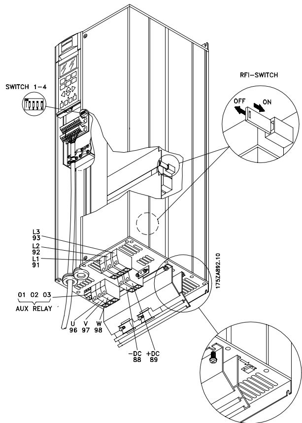
紧凑型 IP 20 VLT 7016-7072, 380-460 V
