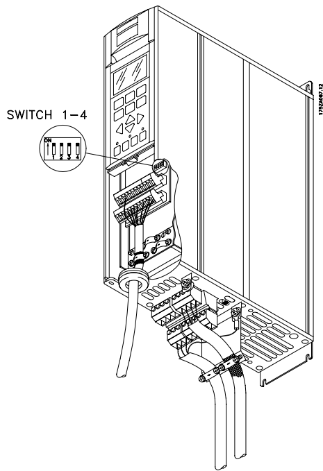
书本型 IP 20 VLT 7002-7011, 380-460 V
