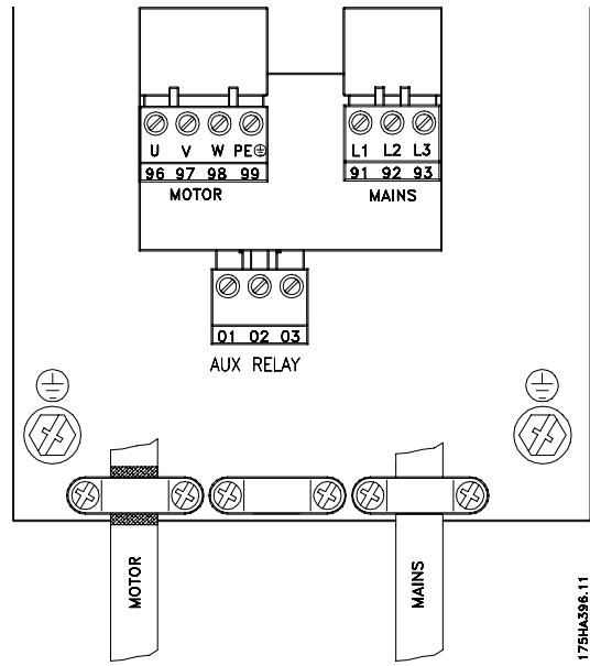
紧凑型 IP 20 VLT 7002-7011, 380-460 V
