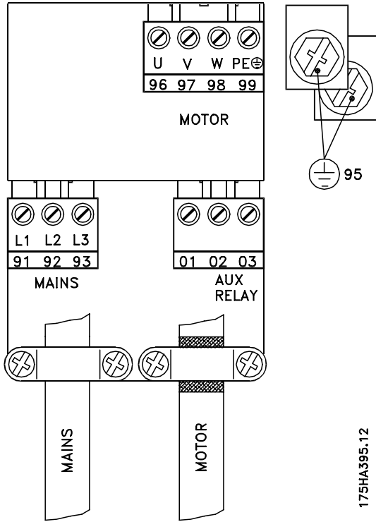
书本型 IP 20 VLT 7002-7011, 380-460 V
