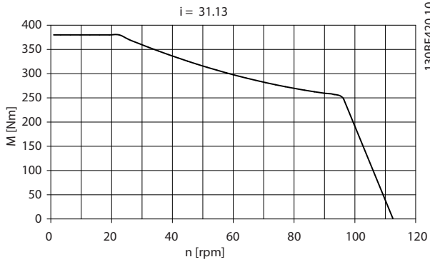
Afbeelding 8.2 Verhouding i = 31,13
