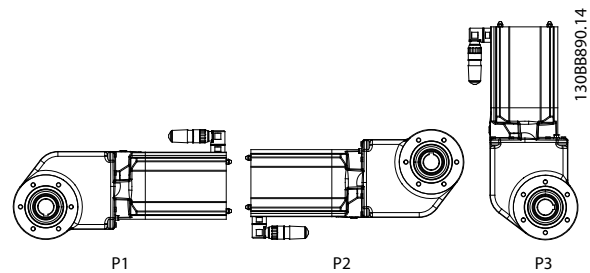
Afbeelding 6.2 Montageposities
