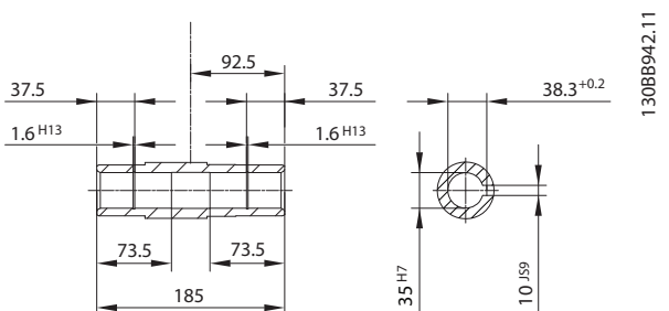
Afbeelding 8.7 Staal/roestvrij staal 35
