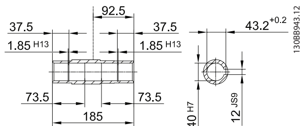
Afbeelding 8.8 Staal/roestvrij staal 40
