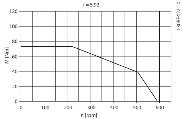
Afbeelding 8.4 Verhouding i = 5,92
