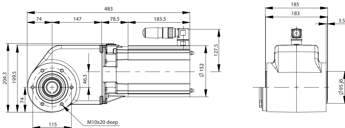
Afbeelding 8.10 OneGearDrive Hygienic
