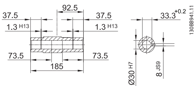
Afbeelding 8.6 Staal/roestvrij staal 30
