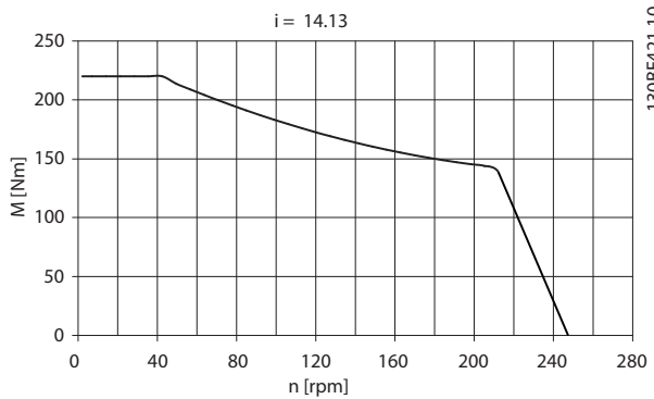
Afbeelding 8.3 Verhouding i = 14,13
