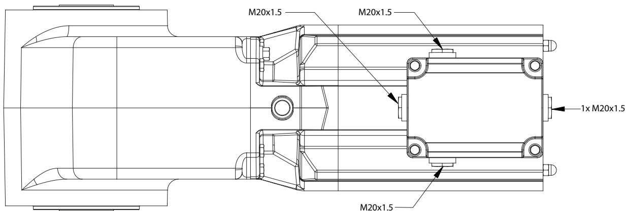
Afbeelding 4.2 Schroeven aansluitkast
