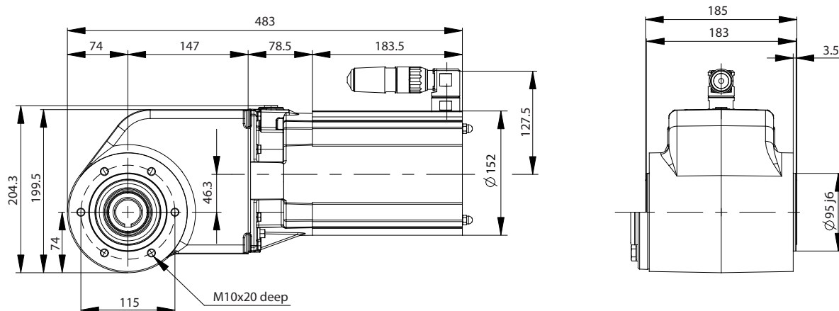
Ilustração 8.10 OneGearDrive™ Hygienic
