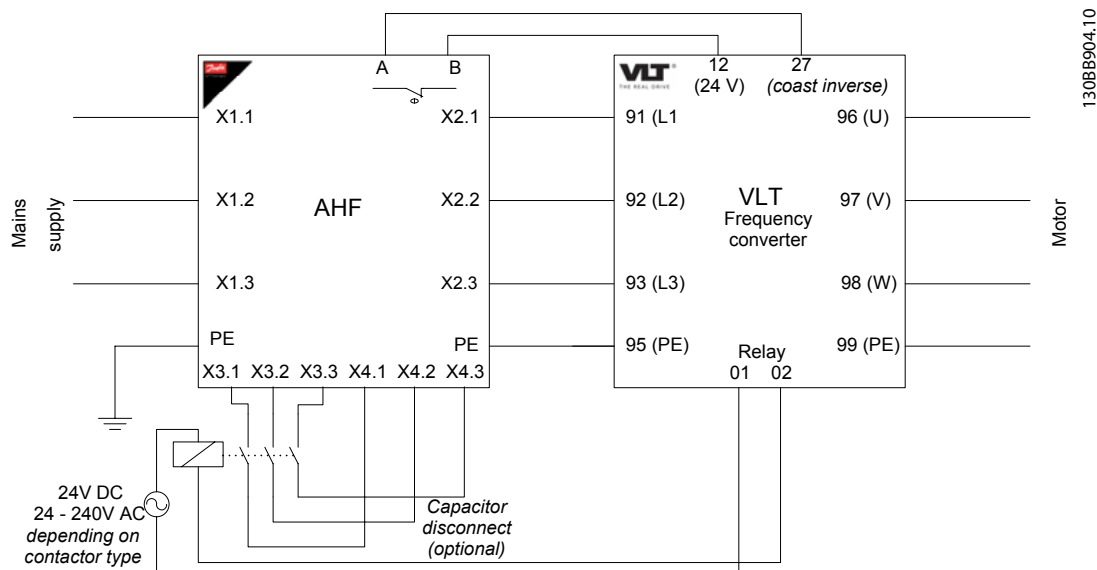
Рисунок 4.13 Схема подключения
