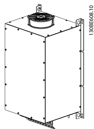
Рисунок 4.6 Конфигурация вентилятора, внешний вентилятор 1
