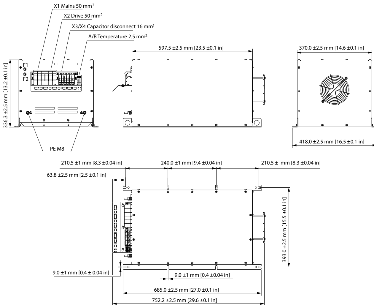
Рисунок 7.33 IP20 X5, внешний вентилятор 1
