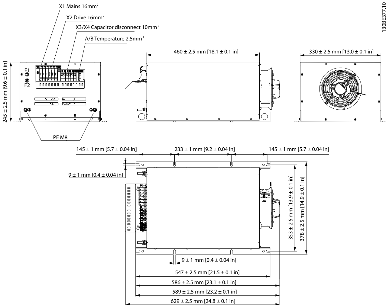
Рисунок 7.19 IP20 X3, внешний вентилятор 2
