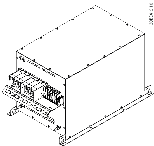
Рисунок 7.44 IP20 X6, внешний вентилятор 2, 3D-вид
