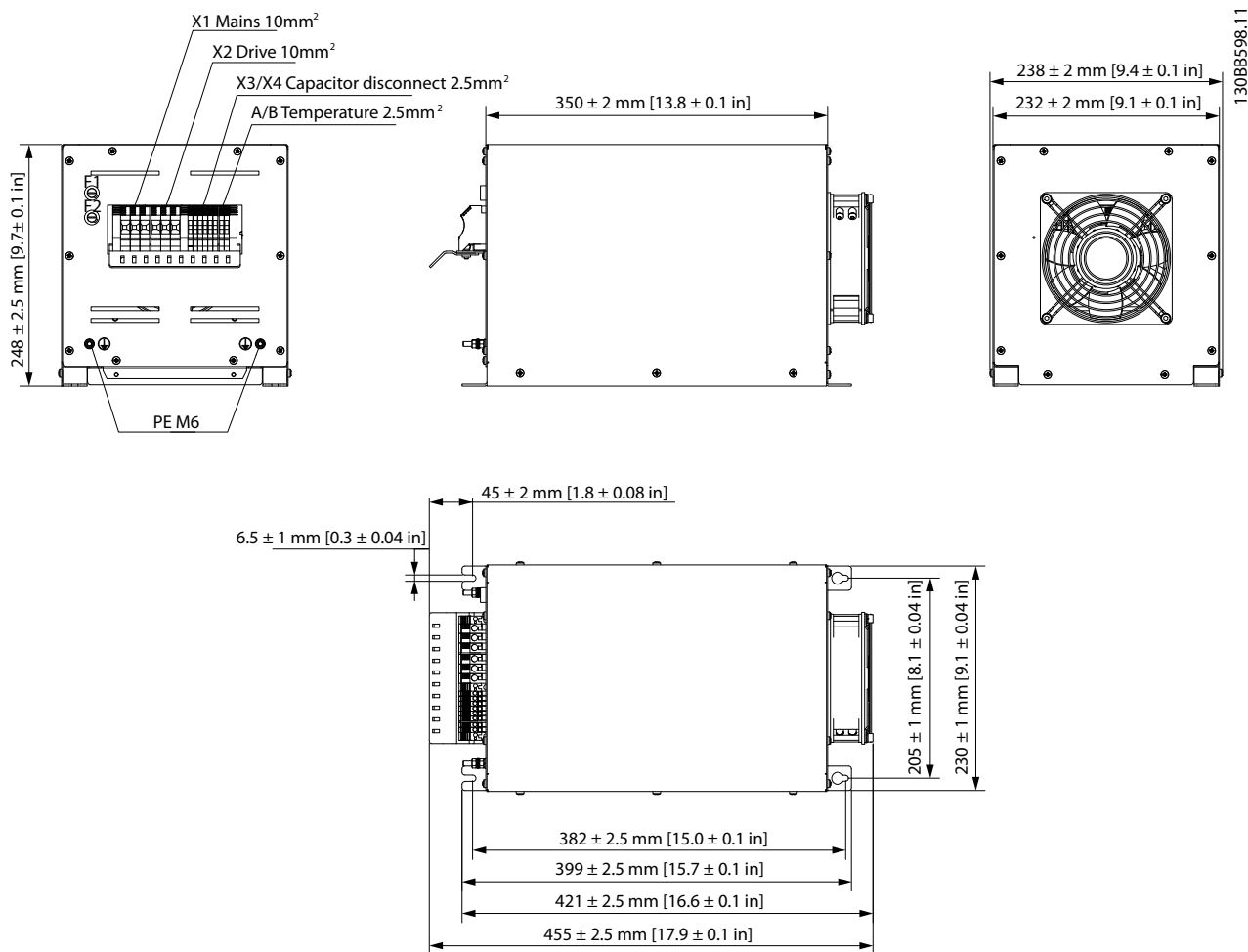
Рисунок 7.11 IP20 X2, внешний вентилятор 1
