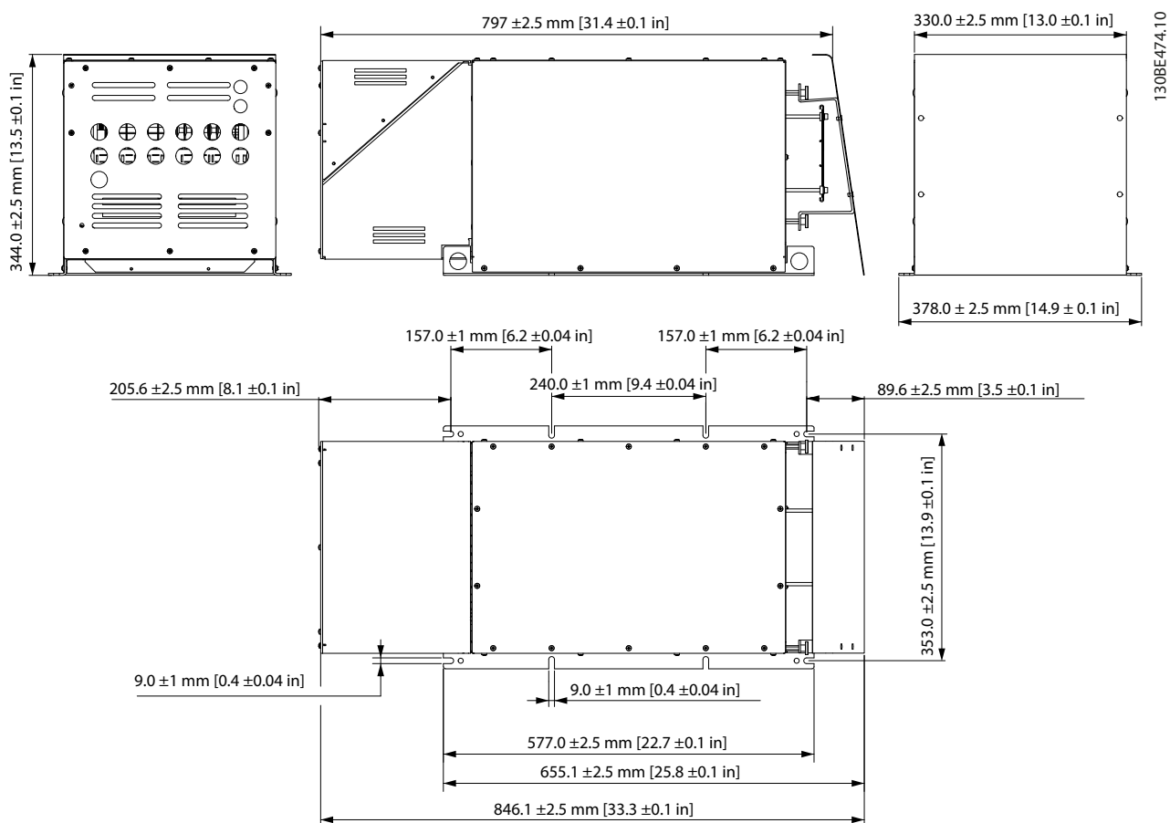
Рисунок 7.81 IP21 X4, внешний вентилятор 1
