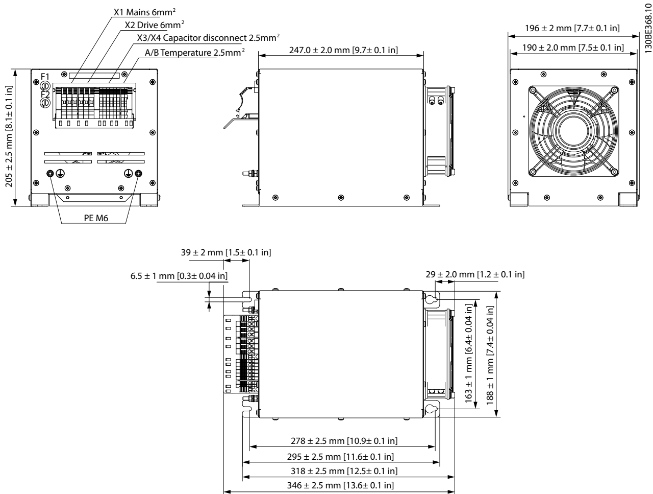
Рисунок 7.7 IP20 X1, внешний вентилятор 1
