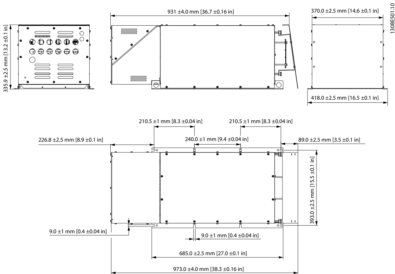
Рисунок 7.89 IP21 X5, внешний вентилятор 1
