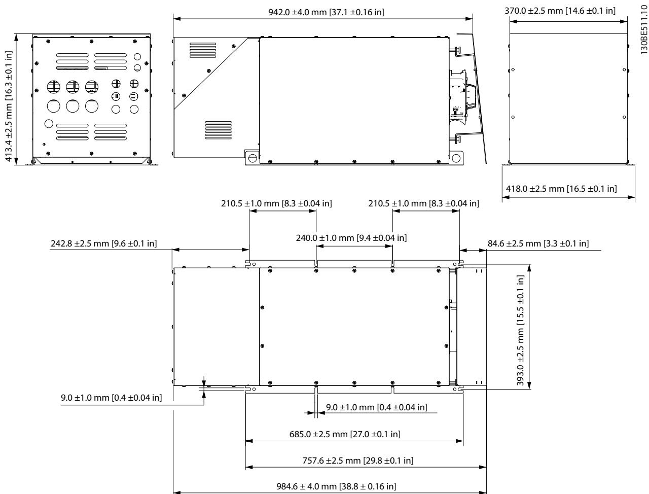
Рисунок 7.99 IP21 X6, внешний вентилятор 2
