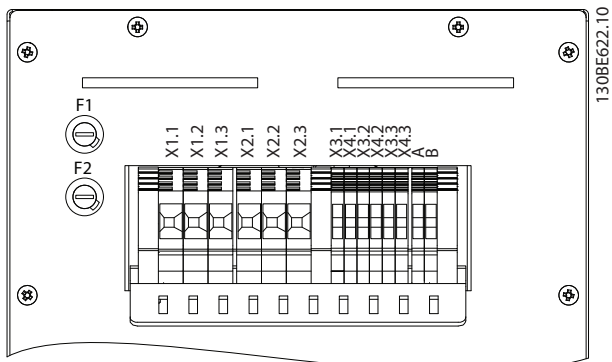
Рисунок 7.3 Обозначения клемм, IP20/IP21 X5–X6
