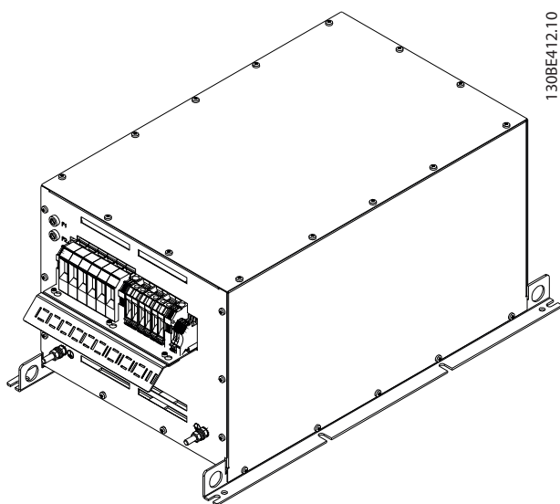
Рисунок 7.34 IP20 X5, внешний вентилятор 1, 3D-вид
