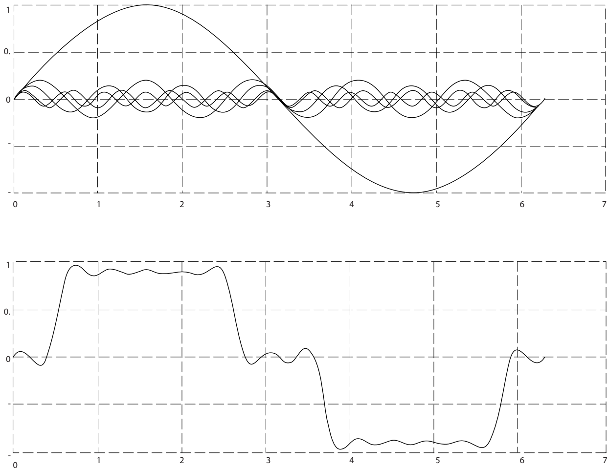
Рисунок 2.3 Синусоидальные колебания
