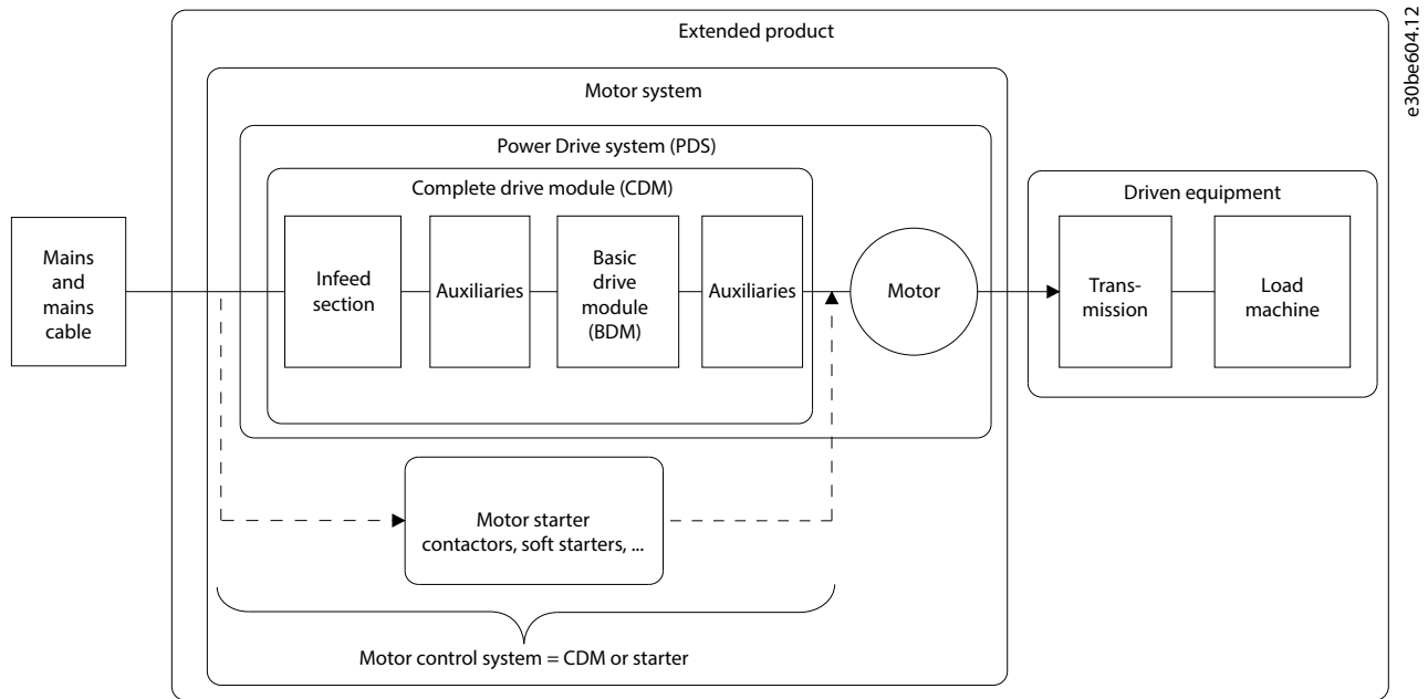
Рисунок 3.9 Система силового привода (PDS) и комплектный модуль привода (CDM)
