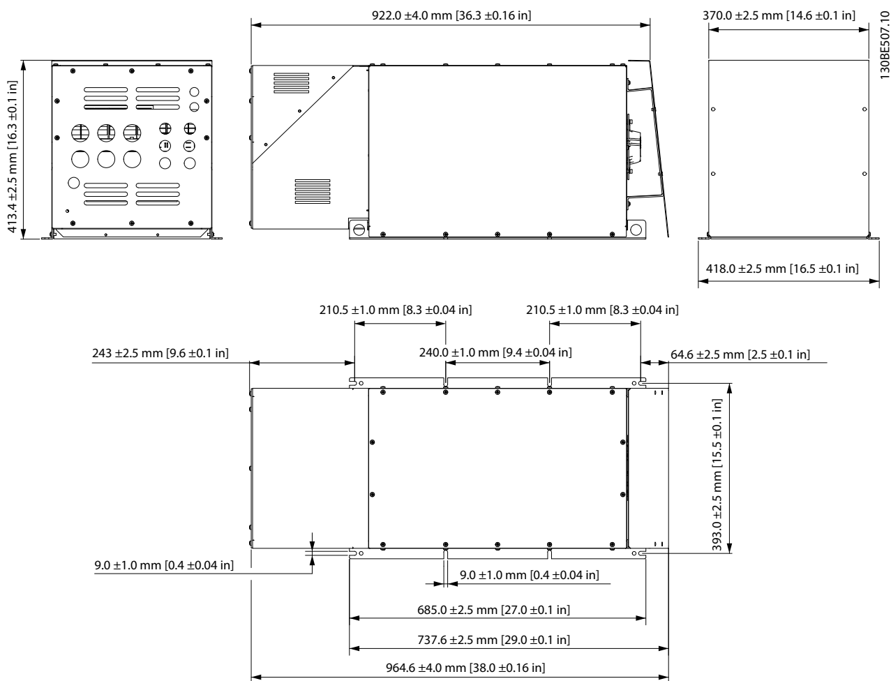
Рисунок 7.95 IP21 X6, внутренний вентилятор 2
