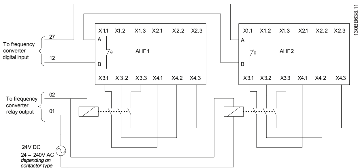
Рисунок 4.14 Параллельное использование ANF в сочетании с разъединителем конденсаторов
