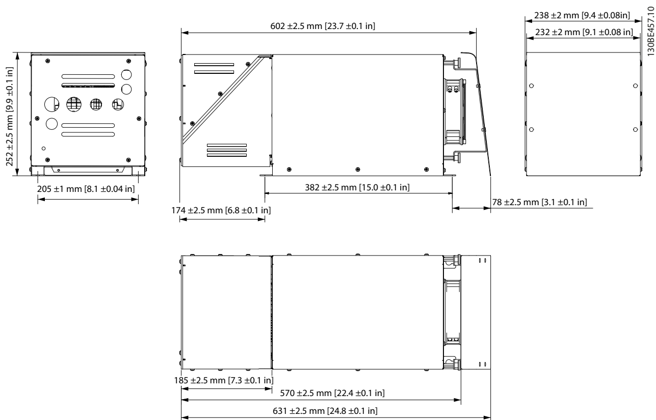
Рисунок 7.67 IP21 X2, внешний вентилятор 1
