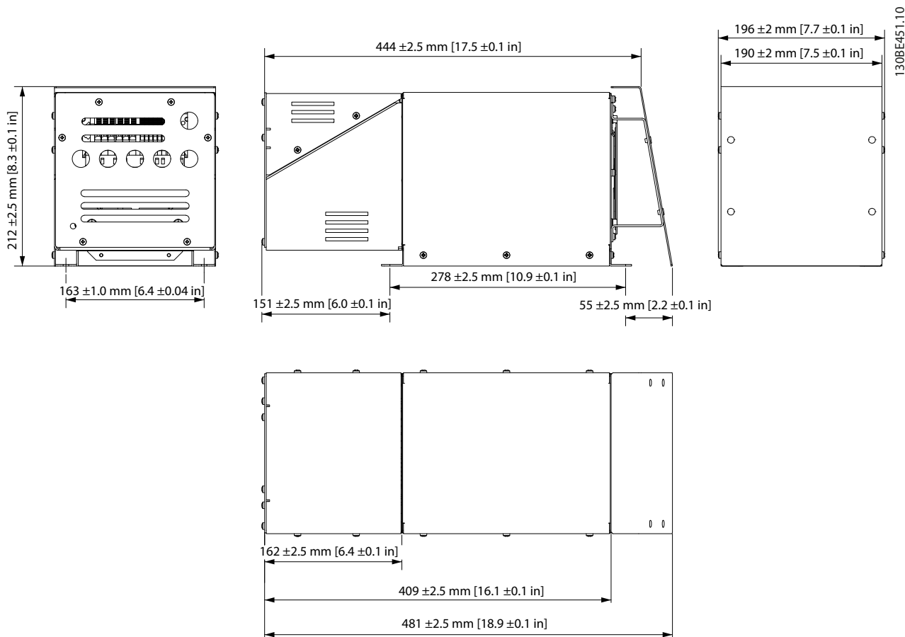
Рисунок 7.61 IP21 X1, внутренний вентилятор 1
