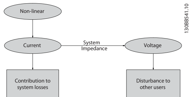
Рисунок 2.5 Негативное влияние гармоник
