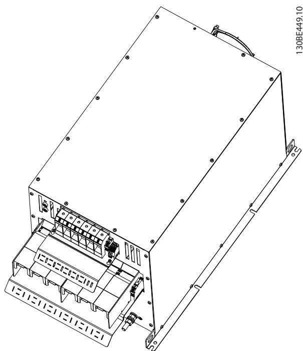
Рисунок 7.58 IP20 X8, внешний вентилятор 1, 3D-вид
