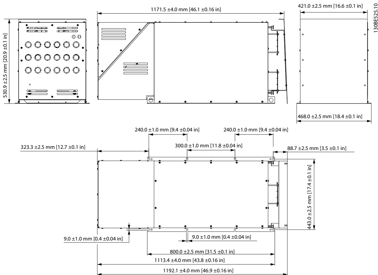
Рисунок 7.113 X8 IP21, внешний вентилятор 1
