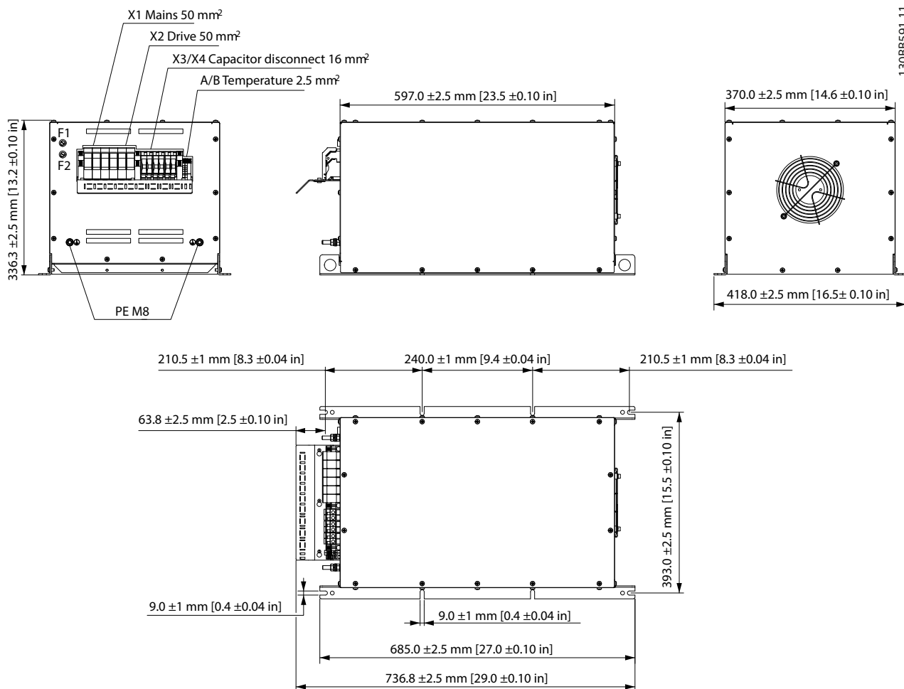
Рисунок 7.29 IP20 X5, внутренний вентилятор 1
