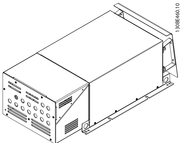
Рисунок 7.70 IP21 X3, внутренний вентилятор 1, 3D-вид
