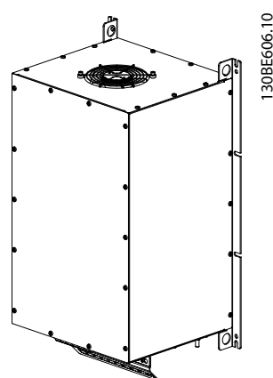
Рисунок 4.4 Конфигурация вентилятора, внутренний вентилятор 1
