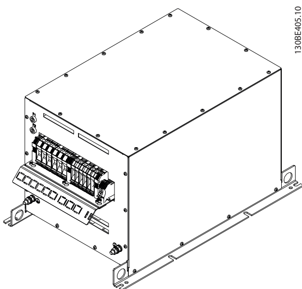
Рисунок 7.28 IP20 X4, внешний вентилятор 2, 3D-вид
