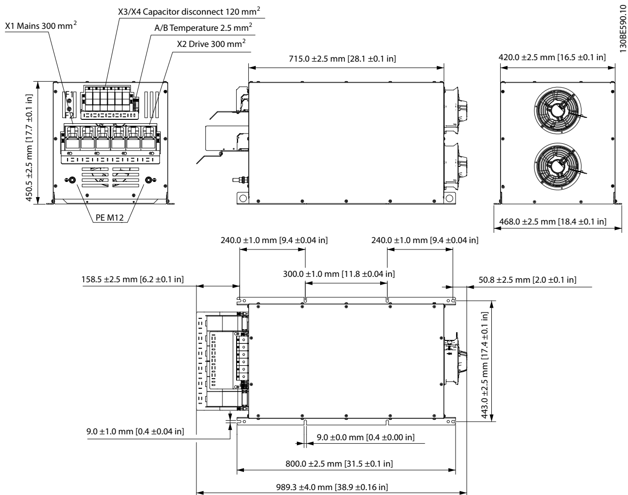
Рисунок 7.51 IP20 X7, внешний вентилятор 2
