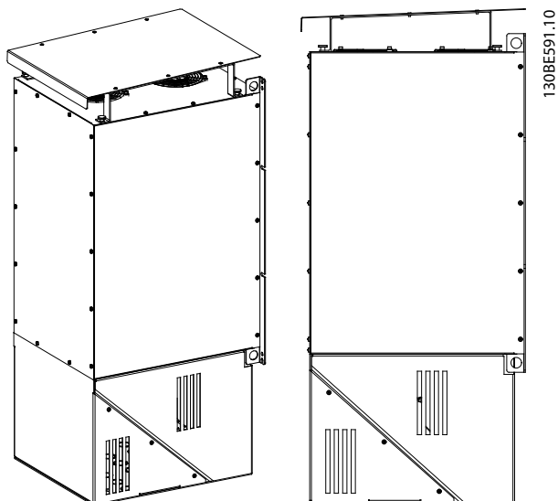
Рисунок 5.1 Комплект IP21/NEMA 1, внутренний вентилятор 1
