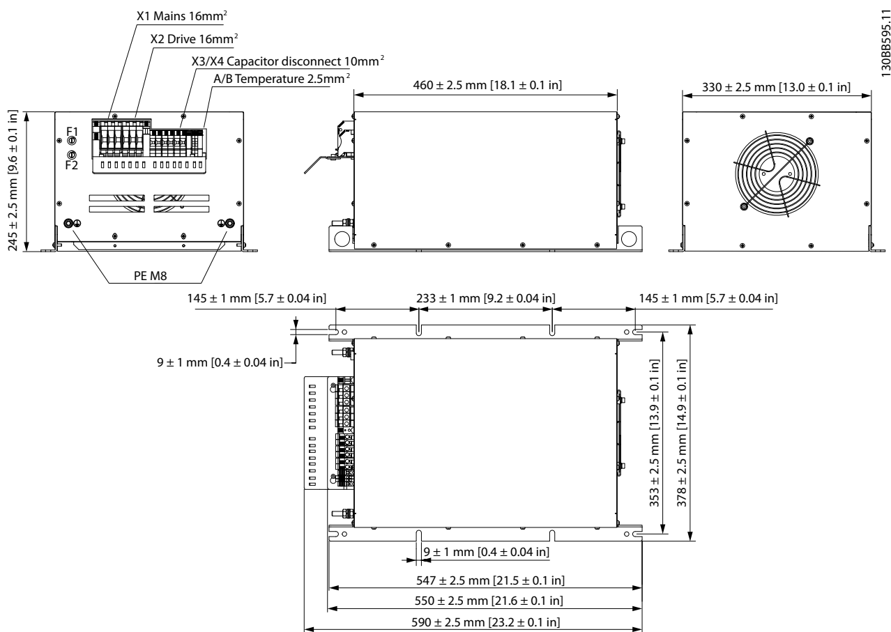
Рисунок 7.13 IP20 X3, внутренний вентилятор 1
