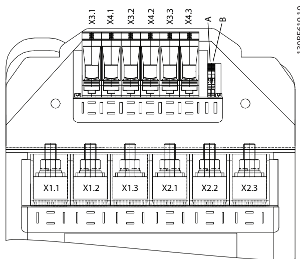
Рисунок 7.119 Обозначения клемм, IP00 X7–X8
