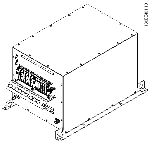
Рисунок 7.22 IP20 X4, внутренний вентилятор 1, 3D-вид
