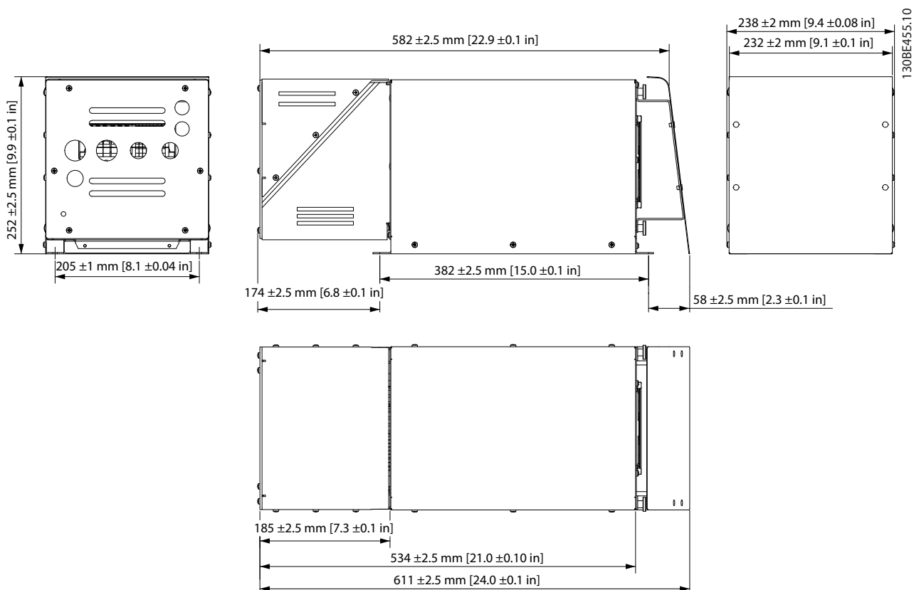
Рисунок 7.65 IP21 X2, внутренний вентилятор 1
