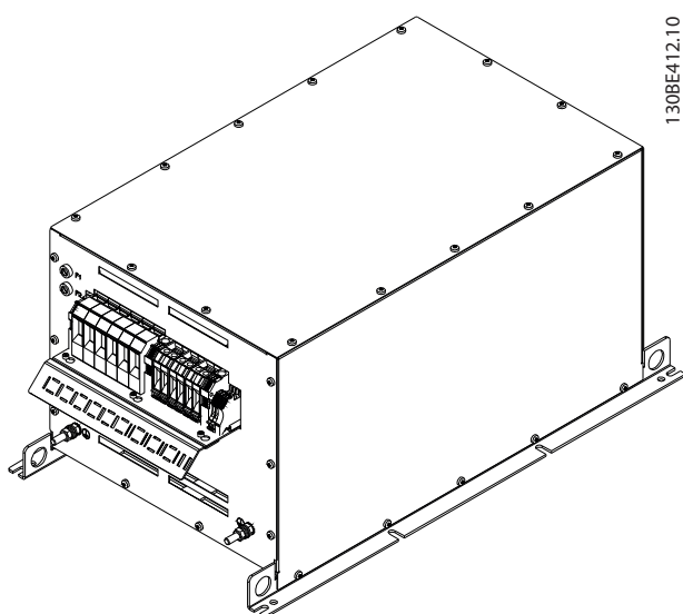
Рисунок 7.36 IP20 X5, внешний вентилятор 2, 3D-вид
