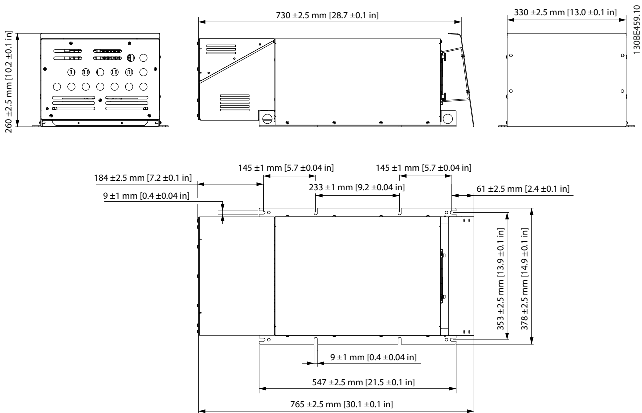
Рисунок 7.69 IP21 X3, внутренний вентилятор 1
