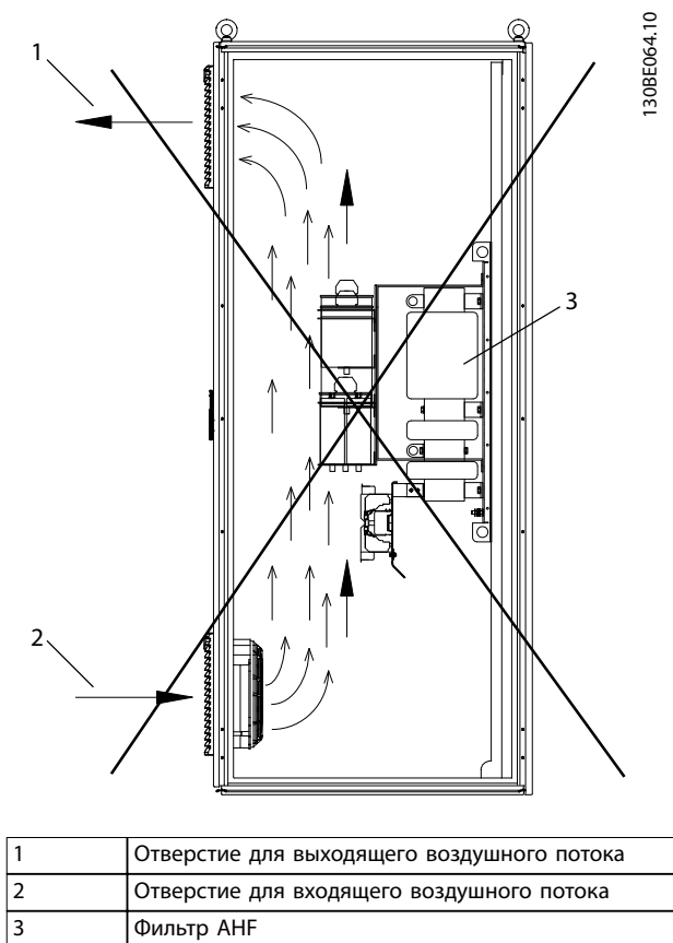
Рисунок 4.9 Неправильная установка — воздух идет в обход фильтра — вид сбоку
