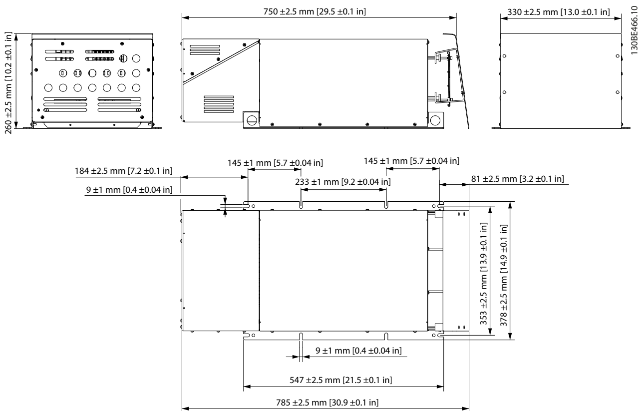
Рисунок 7.73 IP21 X3, внешний вентилятор 1
