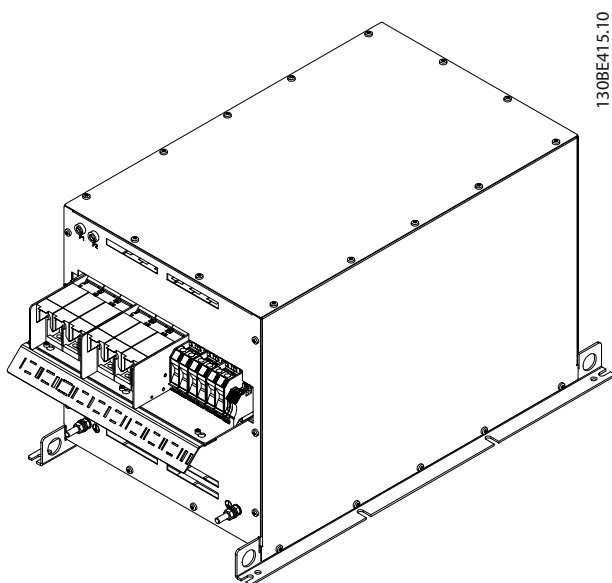
Рисунок 7.40 IP20 X6, внутренний вентилятор 2, 3D-вид
