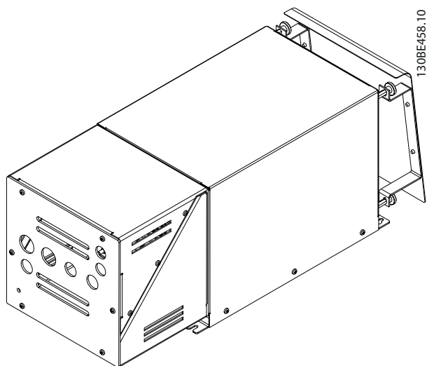
Рисунок 7.68 IP21 X2, внешний вентилятор 1, 3D-вид
