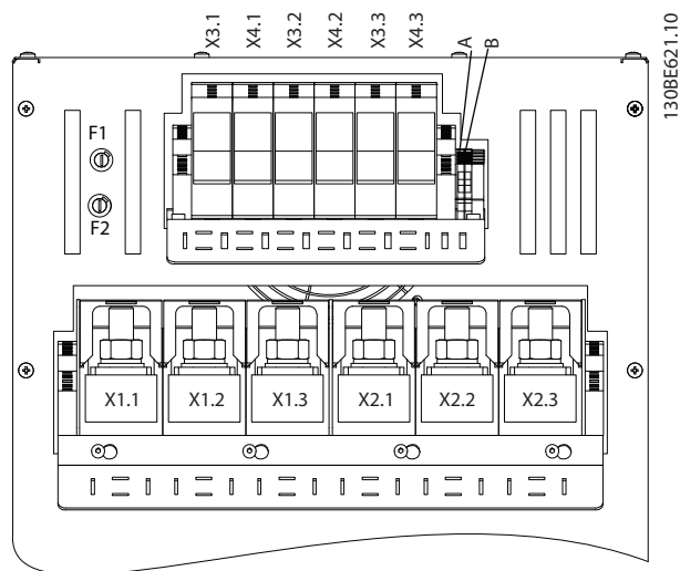
Рисунок 7.4 Обозначения клемм, IP20/IP21 X7–X8
