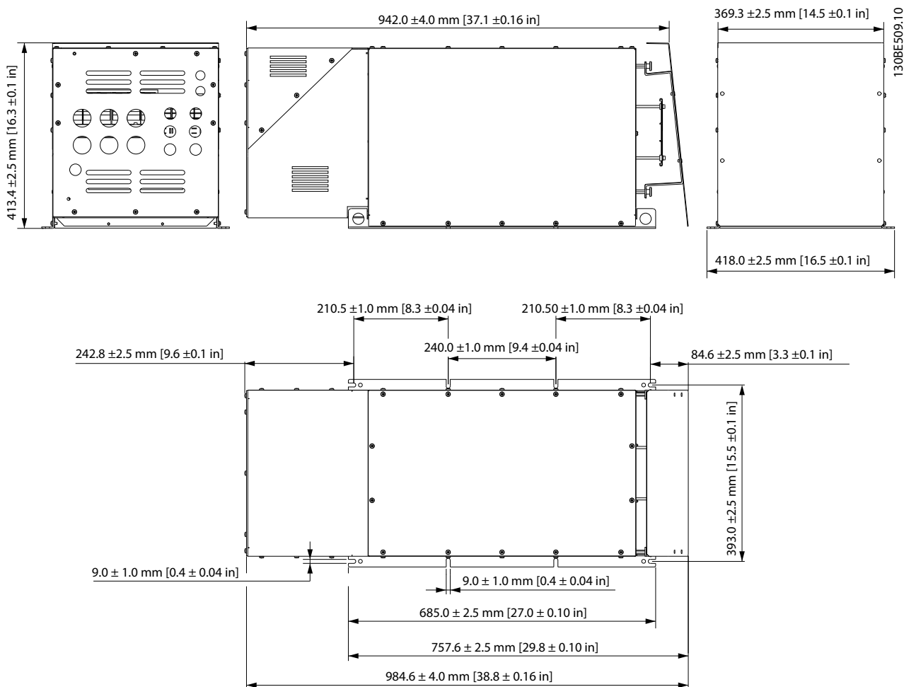
Рисунок 7.97 IP21 X6, внешний вентилятор 1
