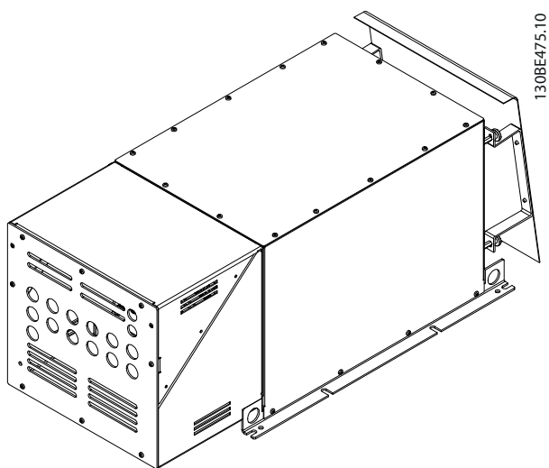
Рисунок 7.82 IP21 X4, внешний вентилятор 1, 3D-вид
