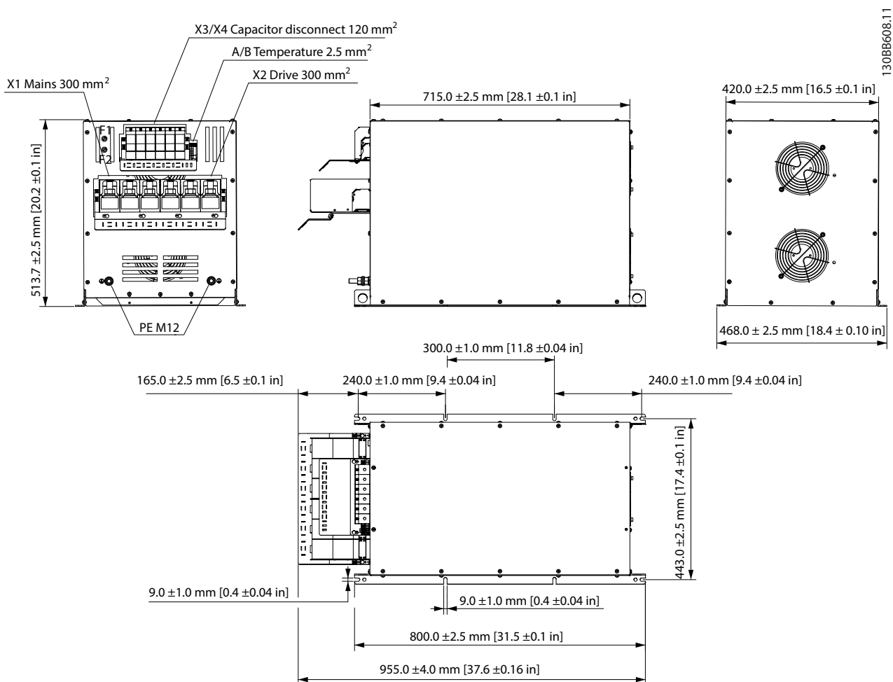
Рисунок 7.53 IP20 X8, внутренний вентилятор 1
