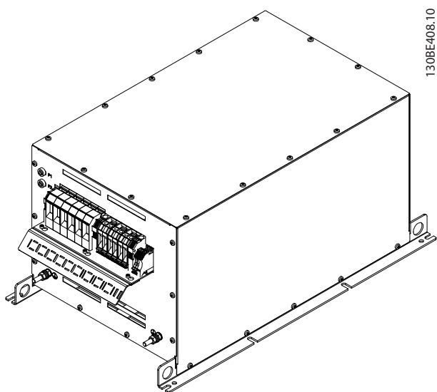
Рисунок 7.30 IP20 X5, внутренний вентилятор 1, 3D-вид
