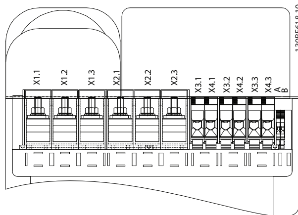
Рисунок 7.118 Обозначения клемм, IP00 X5–X6
