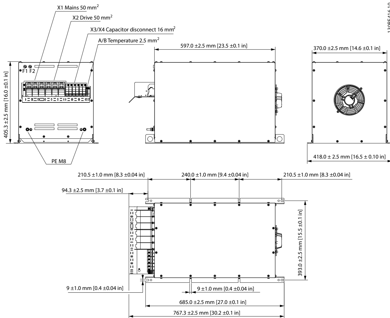
Рисунок 7.39 IP20 X6, внутренний вентилятор 2
