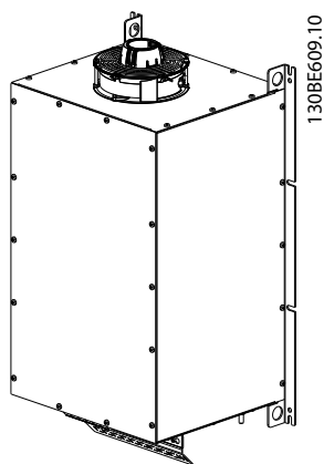
Рисунок 4.7 Конфигурация вентилятора, внешний вентилятор 2
