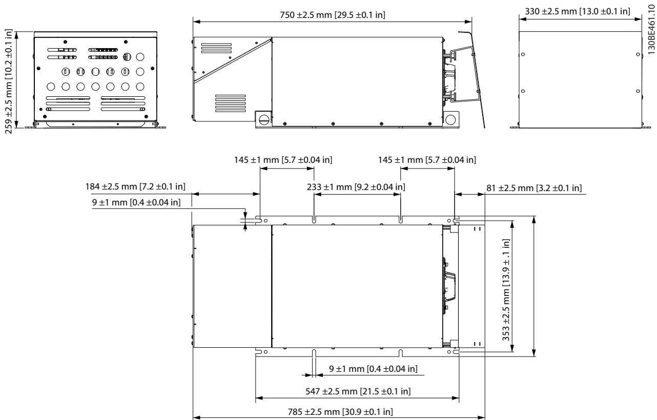
Рисунок 7.71 IP21 X3, внутренний вентилятор 2
