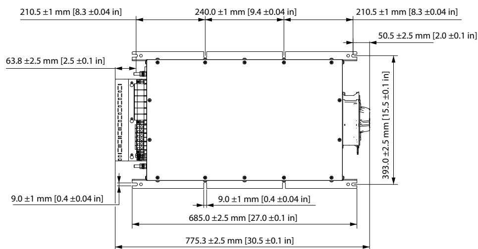
Рисунок 7.35 IP20 X5, внешний вентилятор 2
