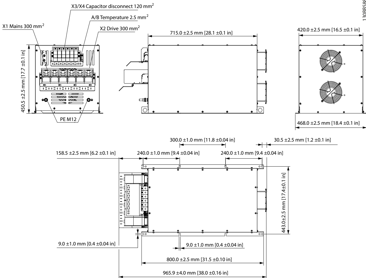
Рисунок 7.49 IP20 X7, внешний вентилятор 1
