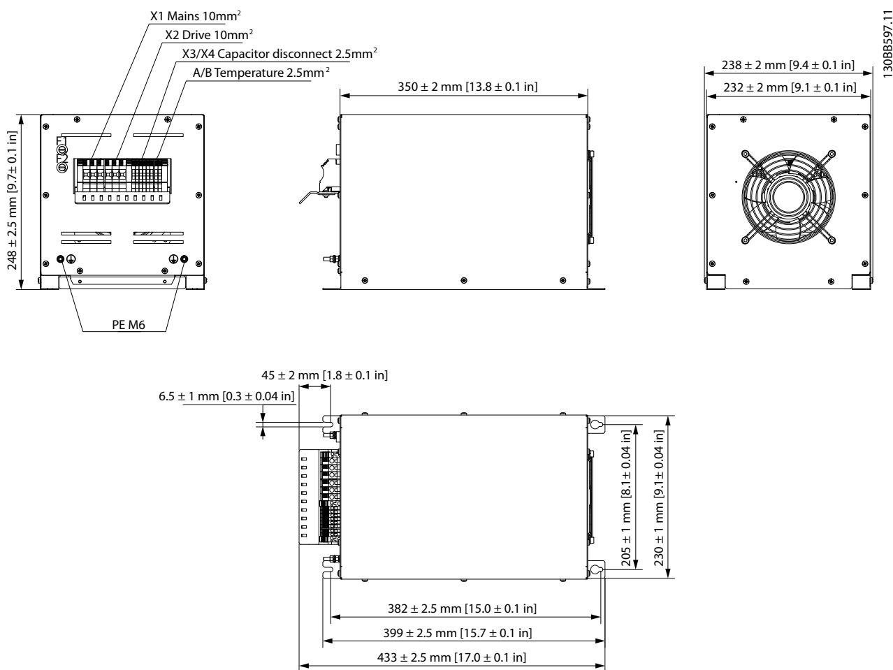
Рисунок 7.9 IP20 X2, внутренний вентилятор 1
