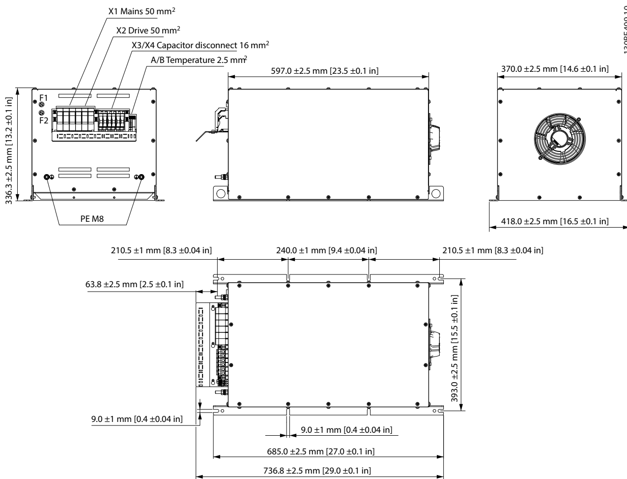
Рисунок 7.31 IP20 X5, внутренний вентилятор 2
