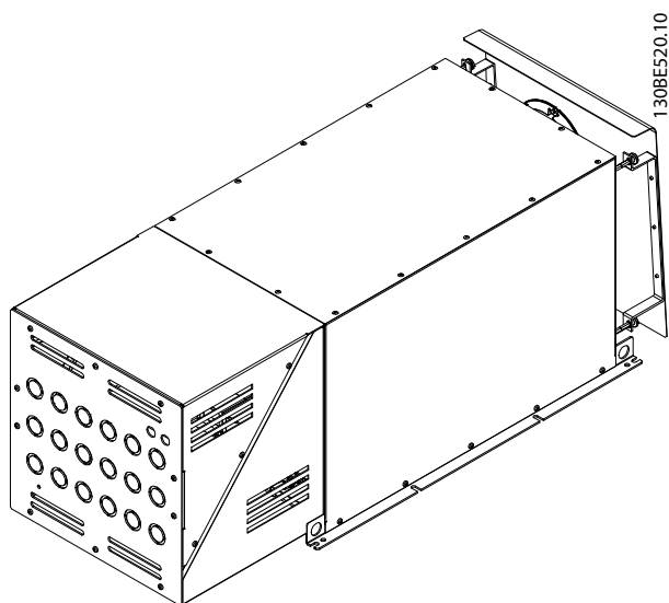
Рисунок 7.110 X8 IP21, внутренний вентилятор 1, 3D-вид
