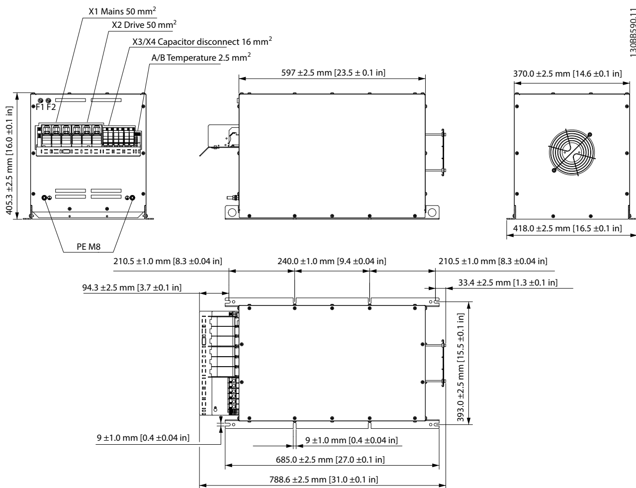
Рисунок 7.41 IP20 X6, внешний вентилятор 1
