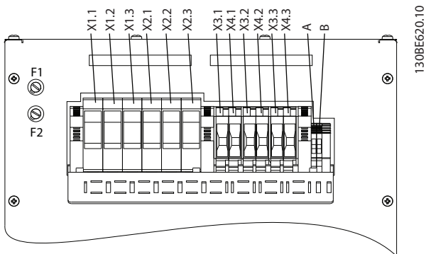
Рисунок 7.2 Обозначения клемм, IP20/IP21 X1–X4
