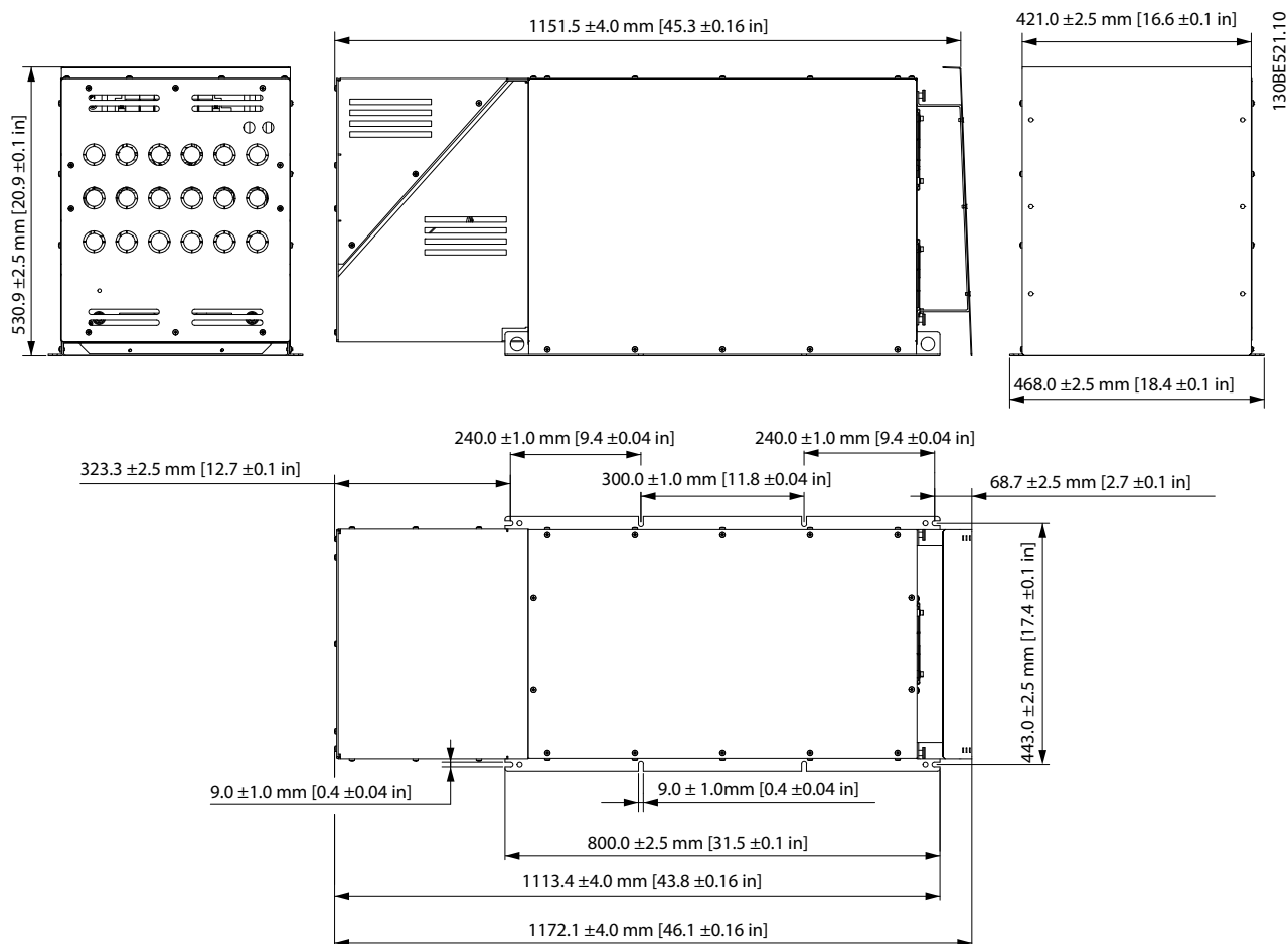
Рисунок 7.109 X8 IP21, внутренний вентилятор 1
