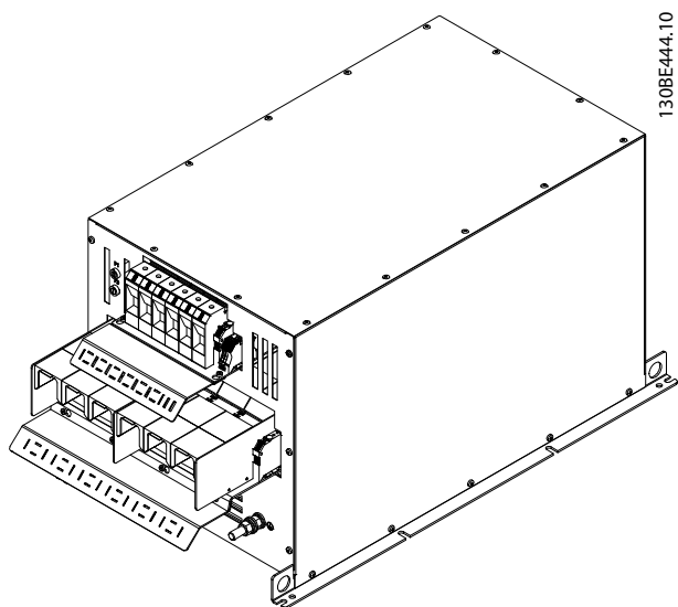
Рисунок 7.48 IP20 X7, внутренний вентилятор 2, 3D-вид
