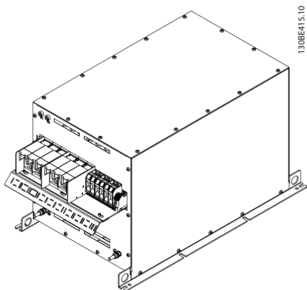
Рисунок 7.38 IP20 X6, внутренний вентилятор 1, 3D-вид
