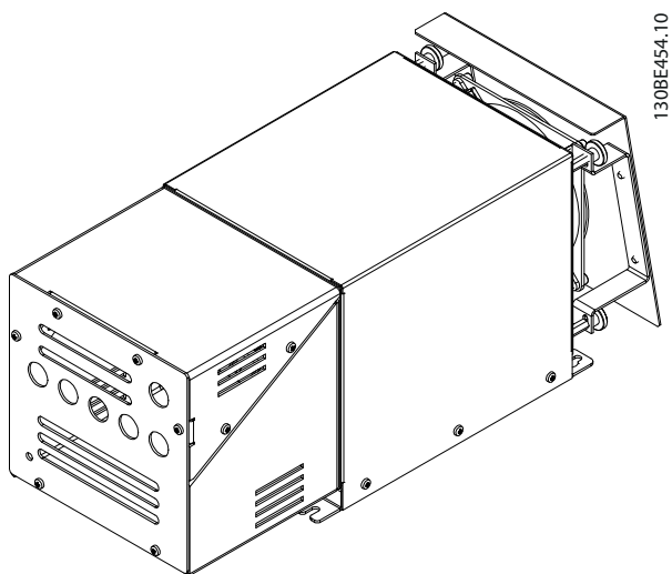
Рисунок 7.64 IP21 X1, внешний вентилятор 1, 3D-вид
