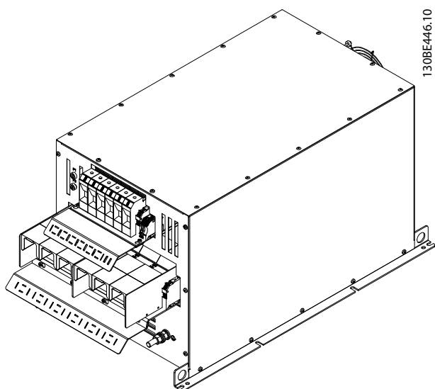
Рисунок 7.52 IP20 X7, внешний вентилятор 2, 3D-вид
