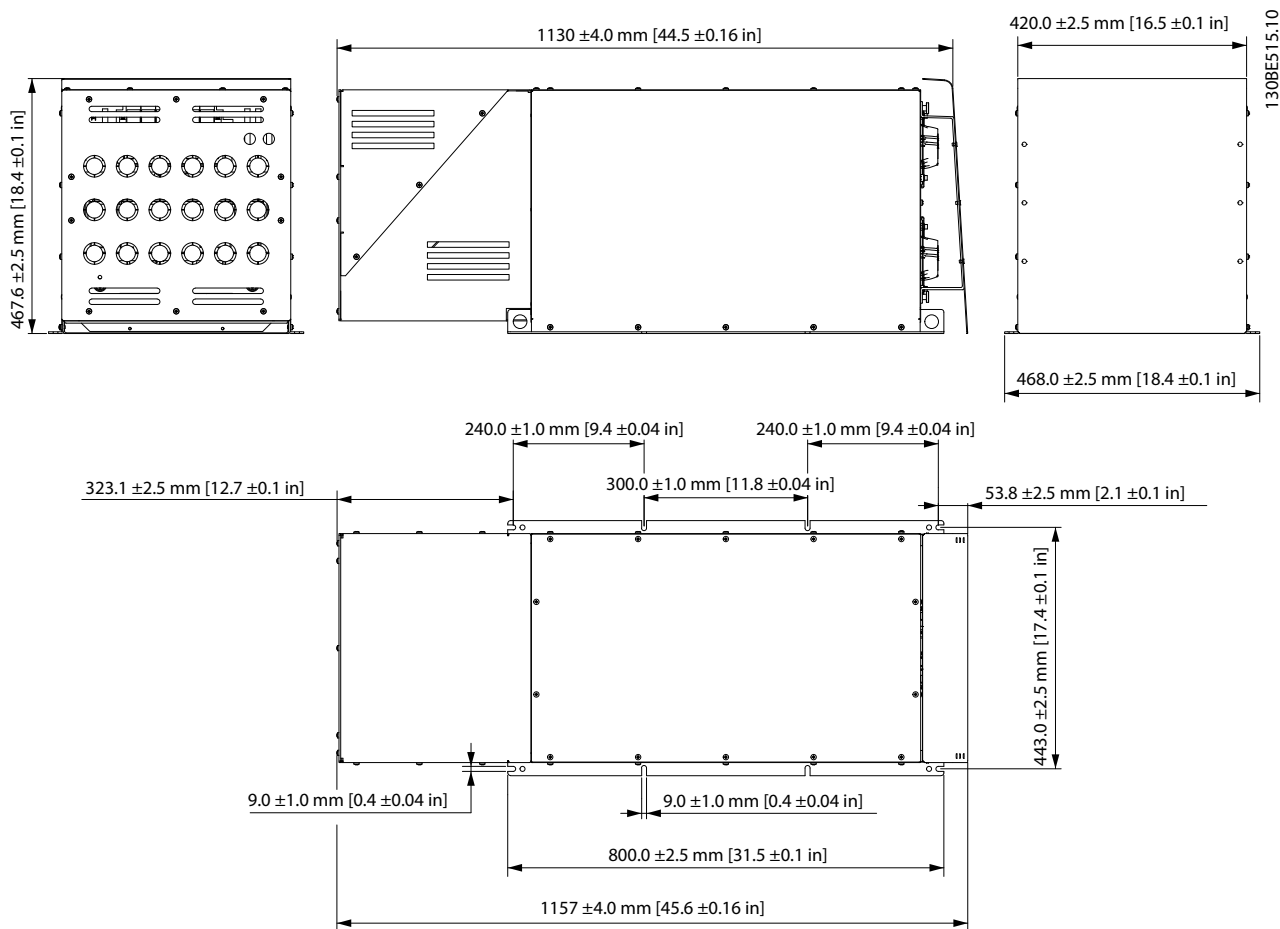
Рисунок 7.103 X7 IP21, внутренний вентилятор 2
