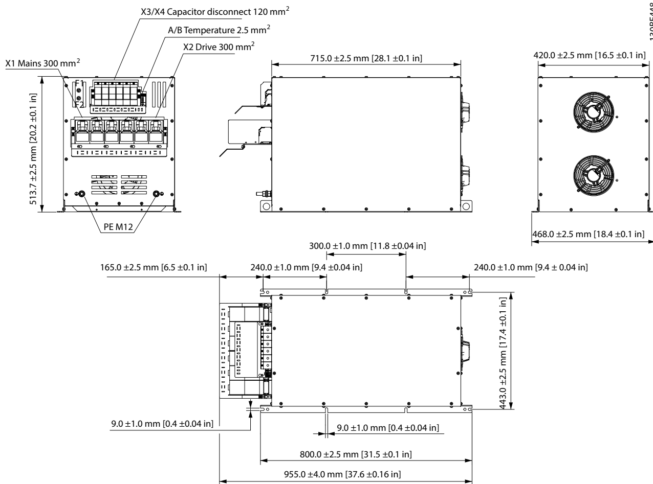
Рисунок 7.55 IP20 X8, внутренний вентилятор 2
