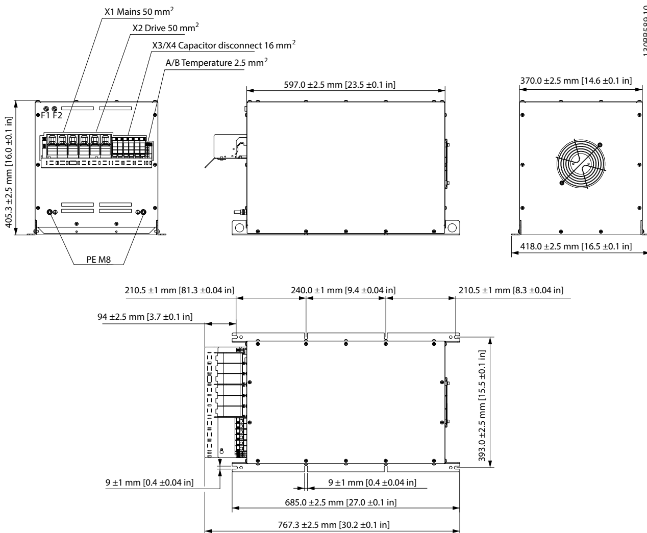
Рисунок 7.37 IP20 X6, внутренний вентилятор 1
