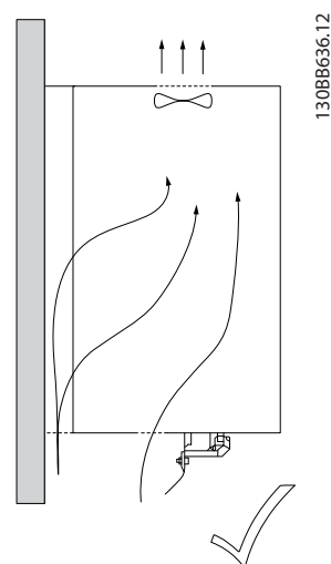
Рисунок 4.1 Правильный воздушный поток без задней панели
