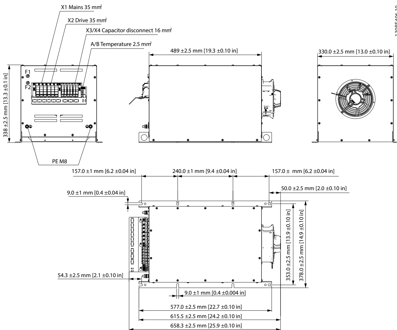
Рисунок 7.27 IP20 X4, внешний вентилятор 2
