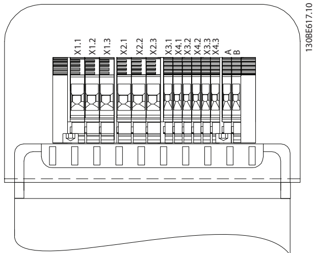
Рисунок 7.117 Обозначения клемм, IP00 X1–X4
