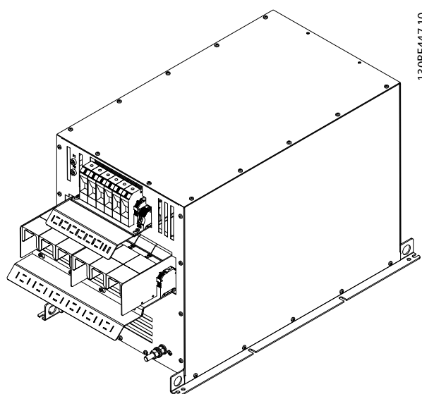
Рисунок 7.56 IP20 X8, внутренний вентилятор 2, 3D-вид
