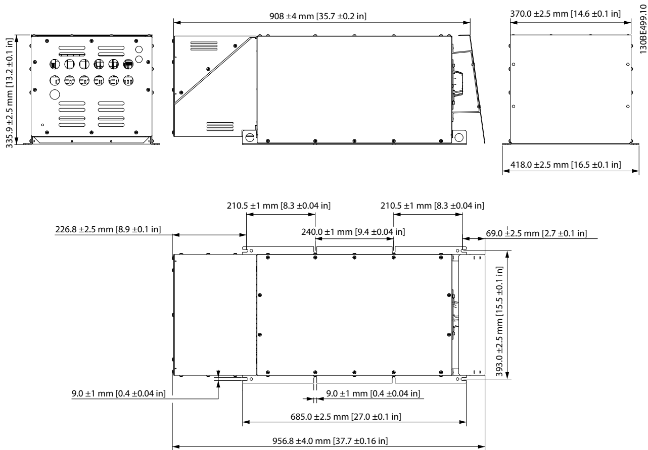
Рисунок 7.87 IP21 X5, внутренний вентилятор 2
