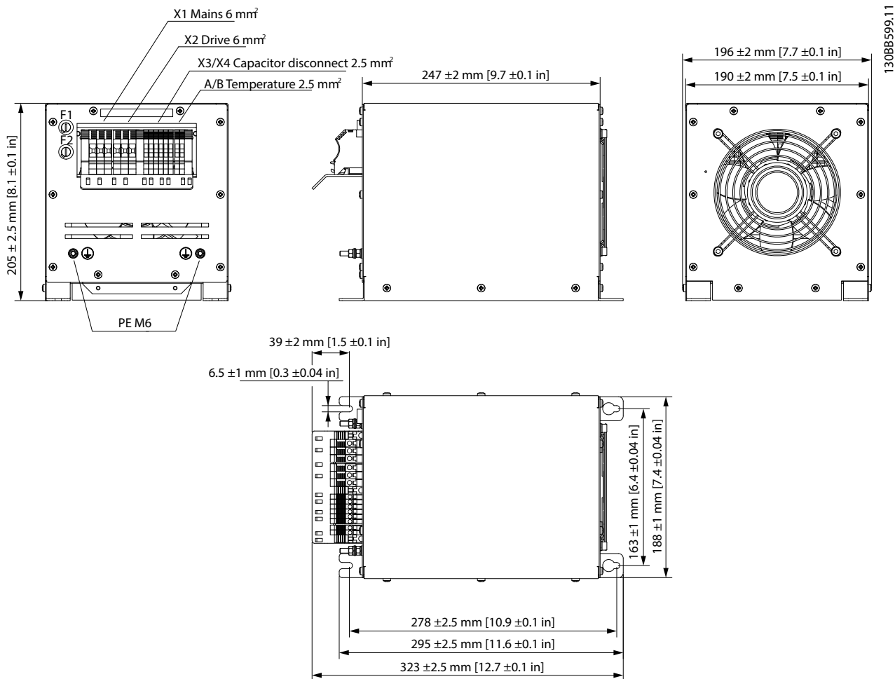
Рисунок 7.5 IP20 X1, внутренний вентилятор 1
