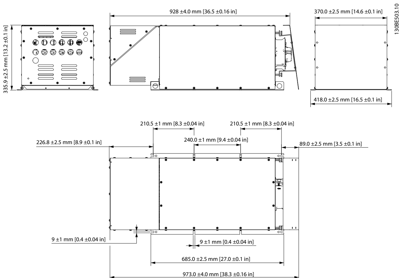
Рисунок 7.91 IP21 X5, внешний вентилятор 2
