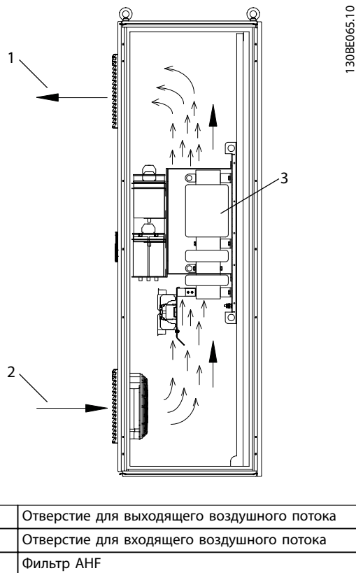
Рисунок 4.10 Правильная установка в узких шкафах — воздушный поток проходит через фильтр
