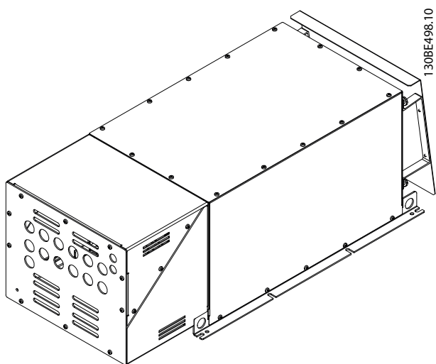
Рисунок 7.86 IP21 X5, внутренний вентилятор 1, 3D-вид
