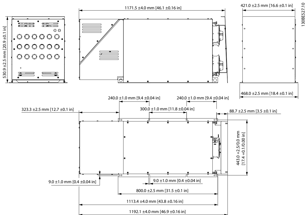
Рисунок 7.115 X8 IP21, внешний вентилятор 2
