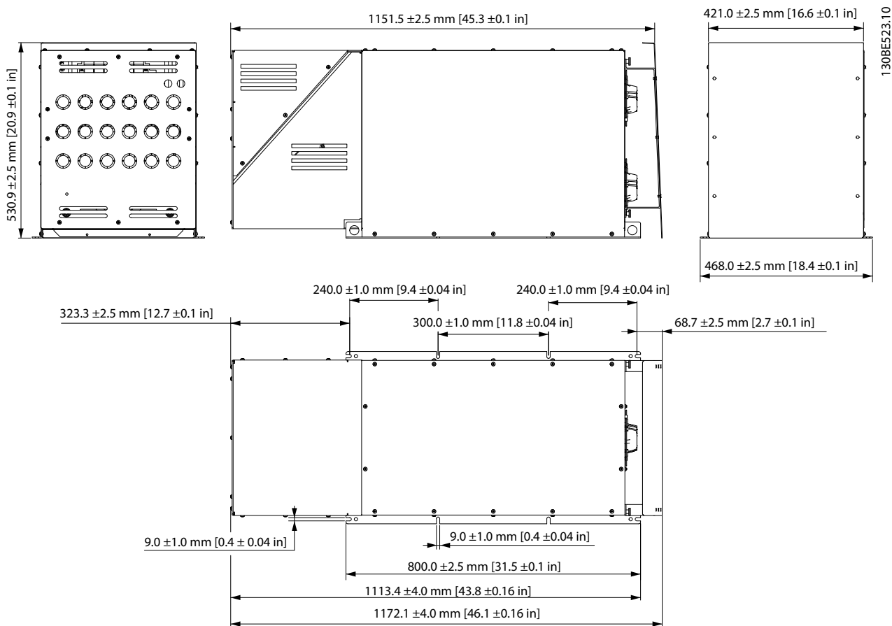
Рисунок 7.111 X8 IP21, внутренний вентилятор 2
