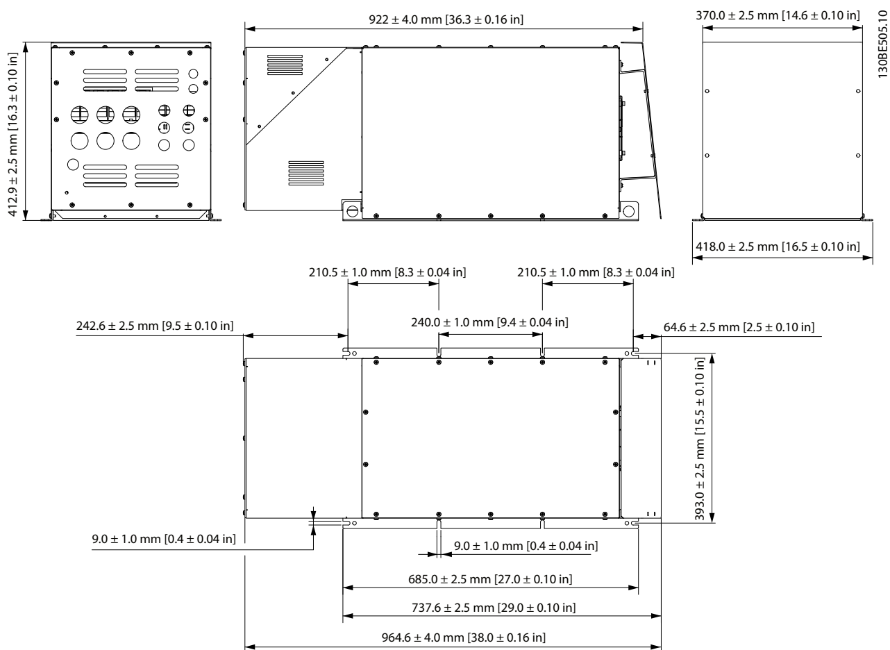
Рисунок 7.93 IP21 X6, внутренний вентилятор 1
