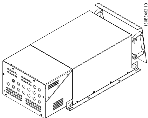
Рисунок 7.72 IP21 X3, внутренний вентилятор 2, 3D-вид
