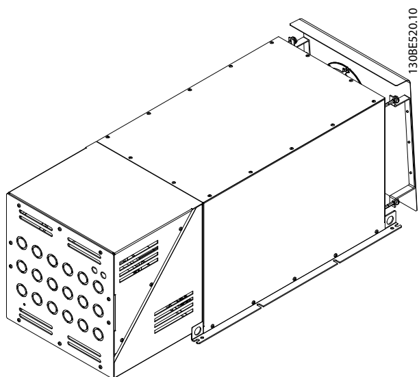
Рисунок 7.112 X8 IP21, внутренний вентилятор 2, 3D-вид
