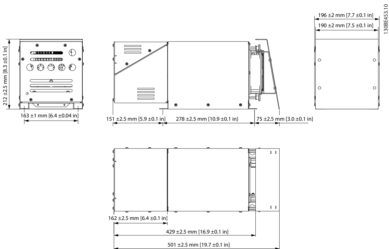
Рисунок 7.63 IP21 X1, внешний вентилятор 1
