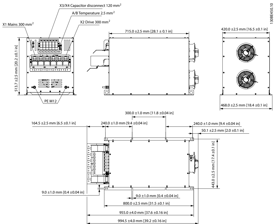
Рисунок 7.59 IP20 X8, внешний вентилятор 2
