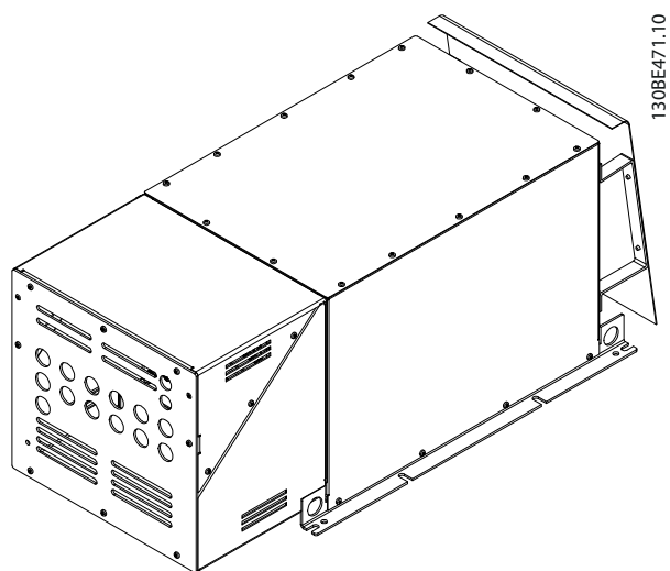
Рисунок 7.78 IP21 X4, внутренний вентилятор 1, 3D-вид
