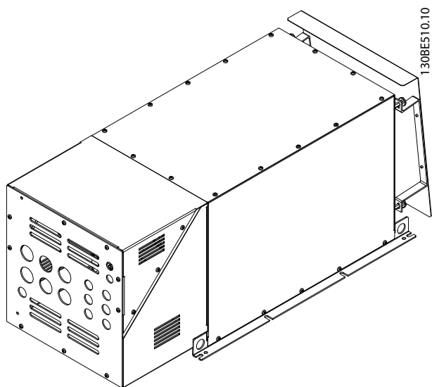
Рисунок 7.98 IP21 X6, внешний вентилятор 1, 3D-вид
