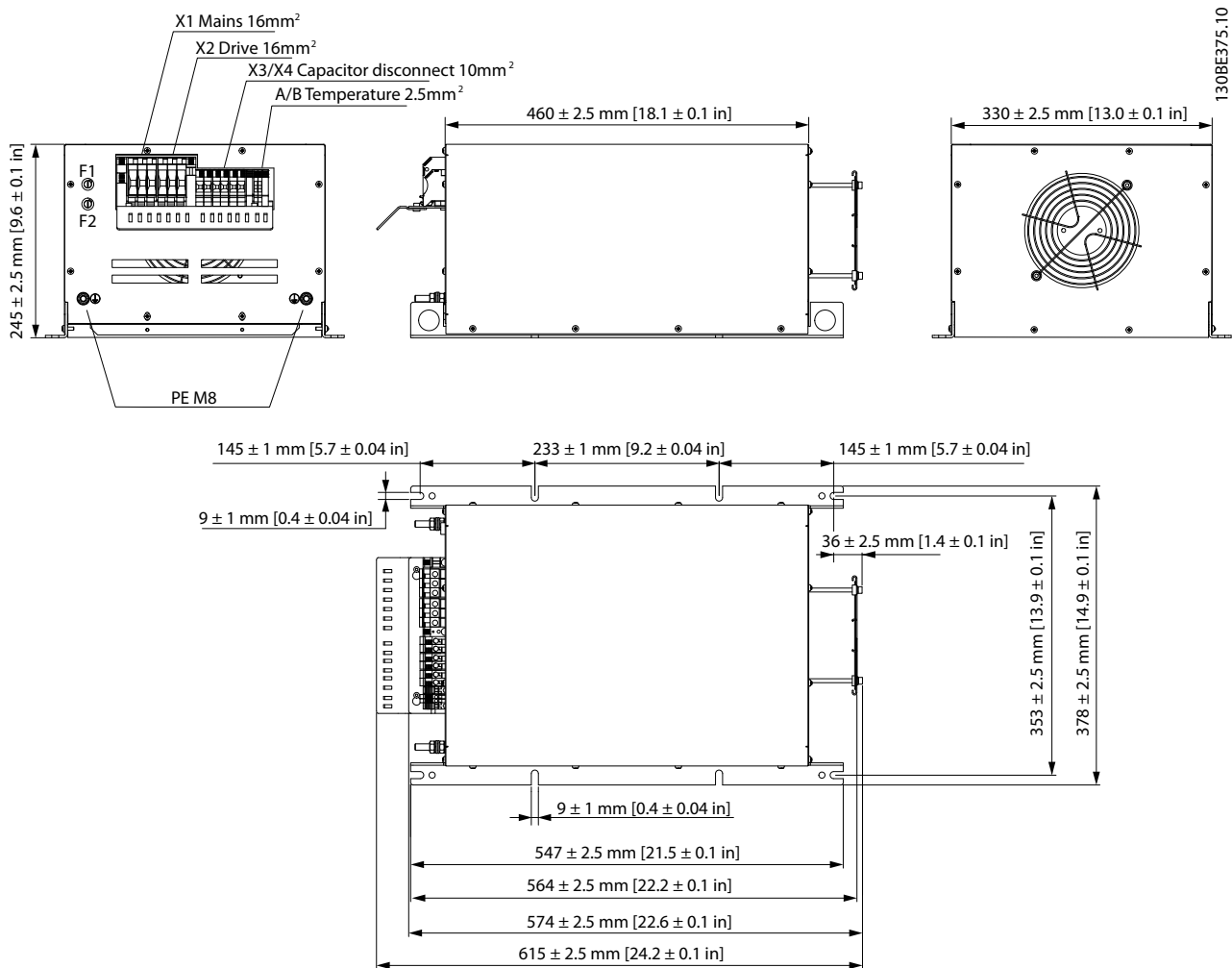
Рисунок 7.17 IP20 X3, внешний вентилятор 1
