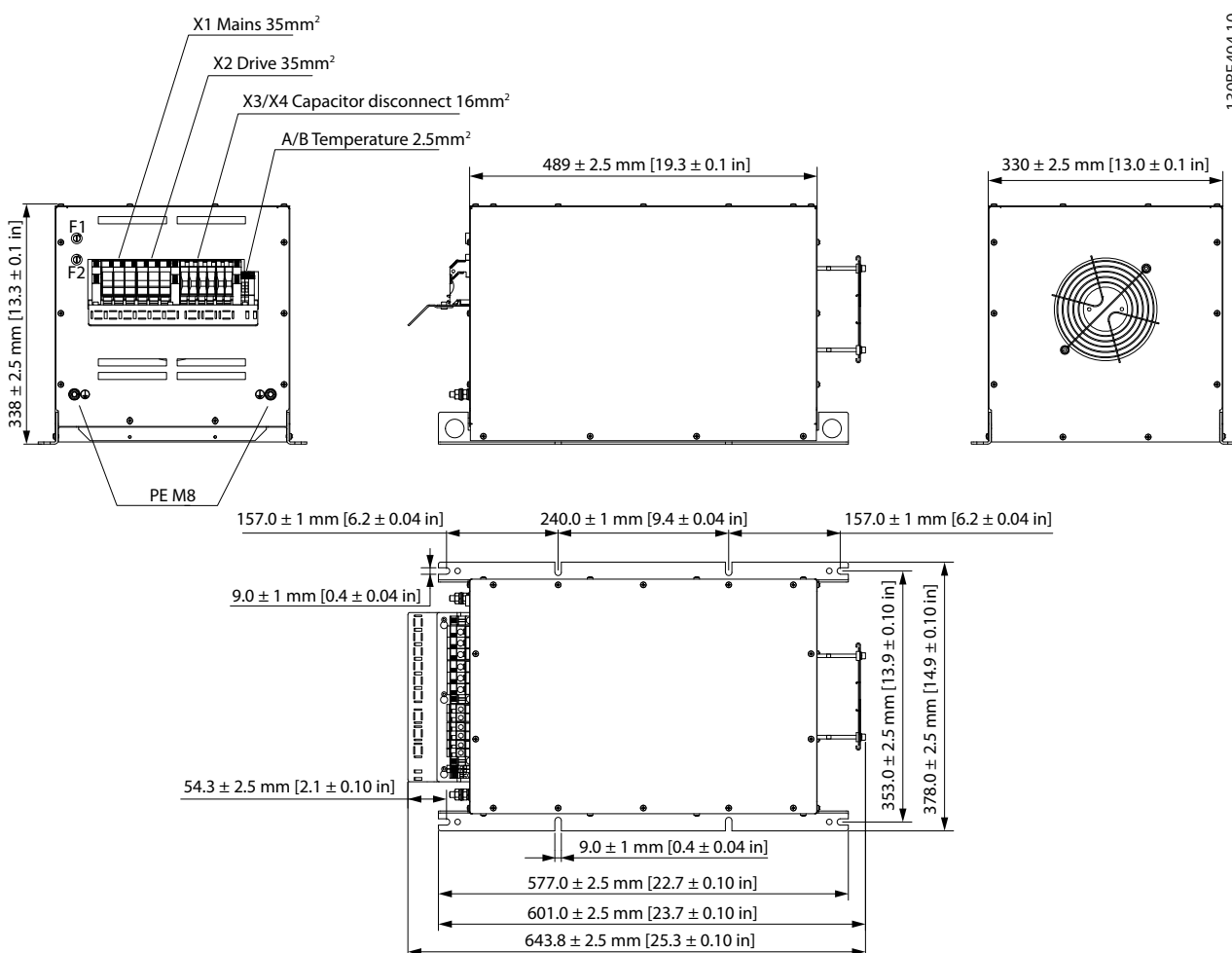
Рисунок 7.25 IP20 X4, внешний вентилятор 1
