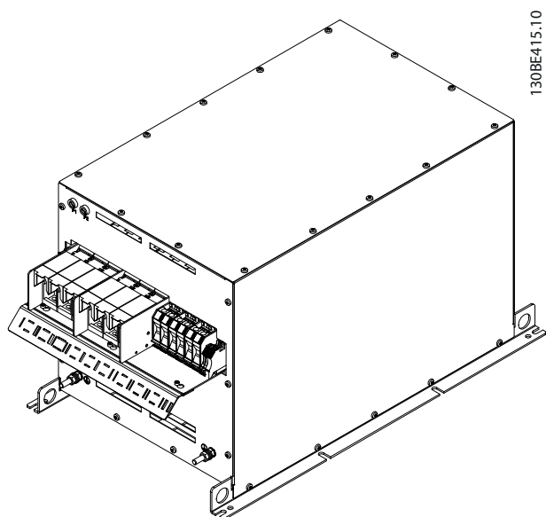
Рисунок 7.42 IP20 X6, внешний вентилятор 1, 3D-вид
