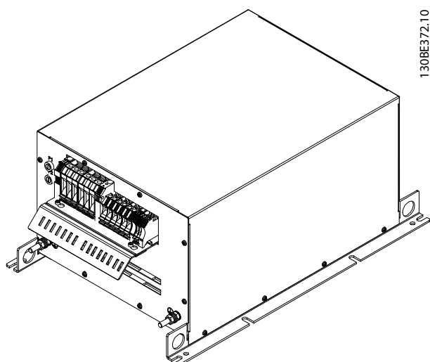
Рисунок 7.16 IP20 X3, внутренний вентилятор 2, 3D-вид
