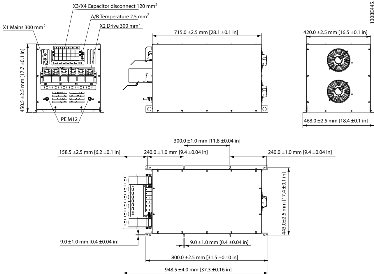
Рисунок 7.47 IP20 X7, внутренний вентилятор 2
