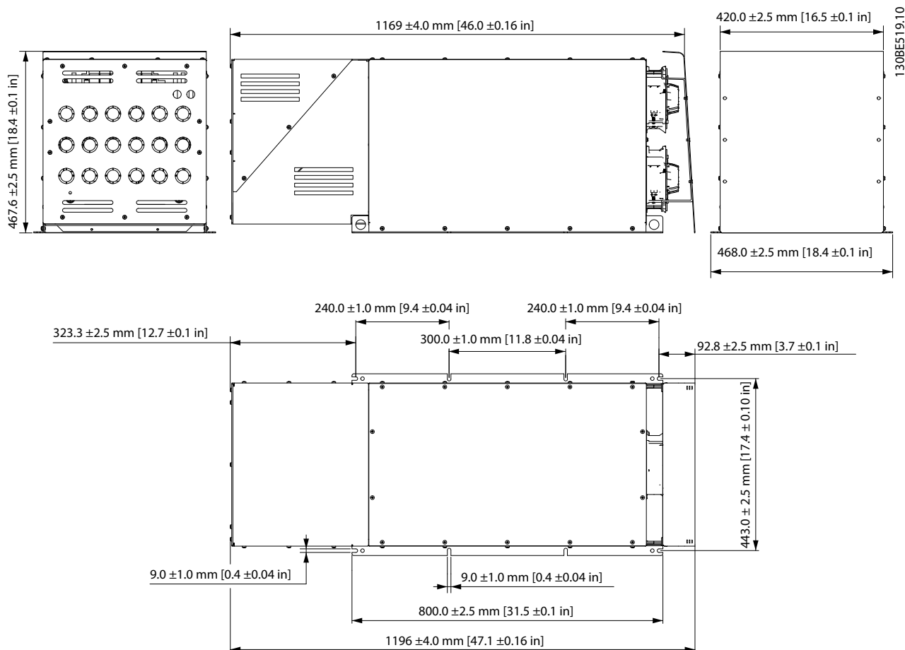
Рисунок 7.107 X7 IP21, внешний вентилятор 2
