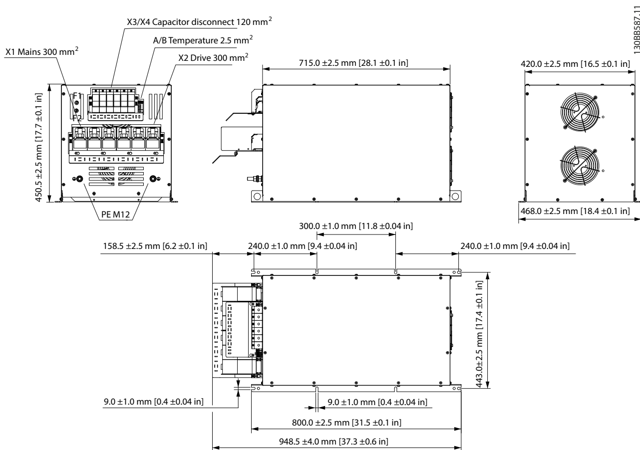
Рисунок 7.45 IP20 X7, внутренний вентилятор 1
