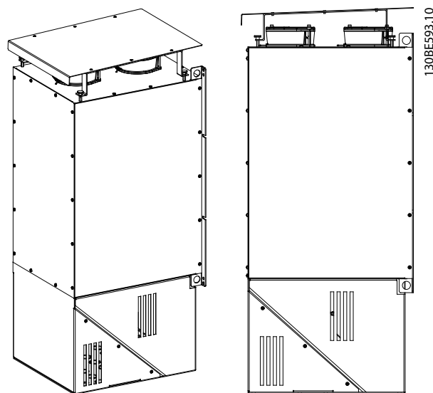
Рисунок 5.3 Комплект IP21/NEMA 1, внешний вентилятор 1
