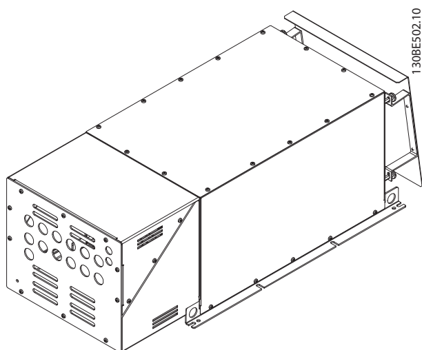
Рисунок 7.92 IP21 X5, внешний вентилятор 2, 3D-вид
