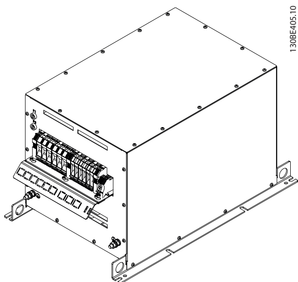
Рисунок 7.26 IP20 X4, внешний вентилятор 1, 3D-вид
