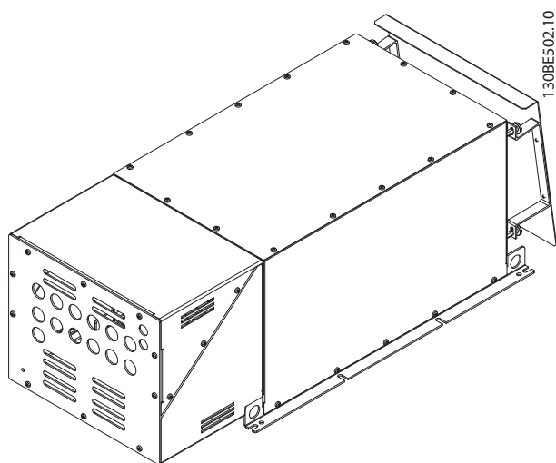
Рисунок 7.90 IP21 X5, внешний вентилятор 1, 3D-вид
