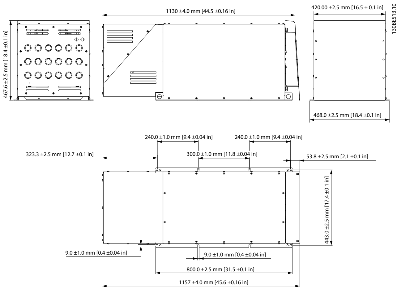
Рисунок 7.101 X7 IP21, внутренний вентилятор 1
