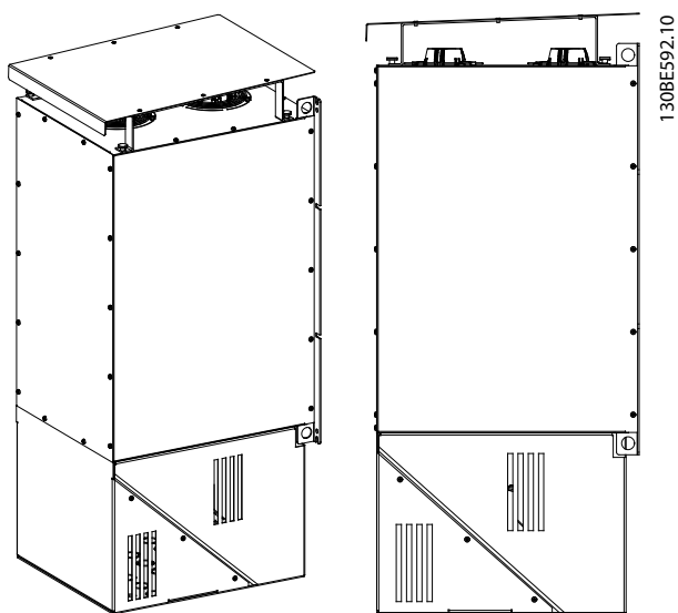
Рисунок 5.2 Комплект IP21/NEMA 1, внутренний вентилятор 2
