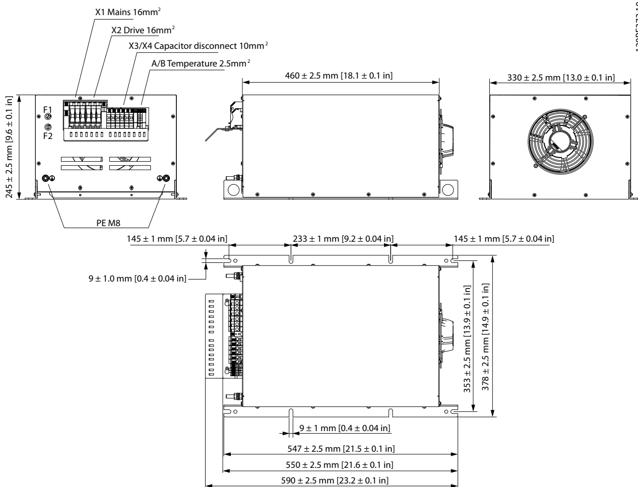
Рисунок 7.15 IP20 X3, внутренний вентилятор 2
