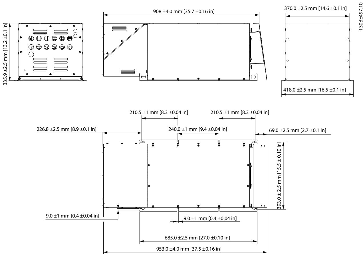
Рисунок 7.85 IP21 X5, внутренний вентилятор 1
