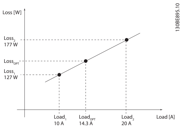
Рисунок 3.13 Определение потери мощности посредством 2-мерной интерполяции
