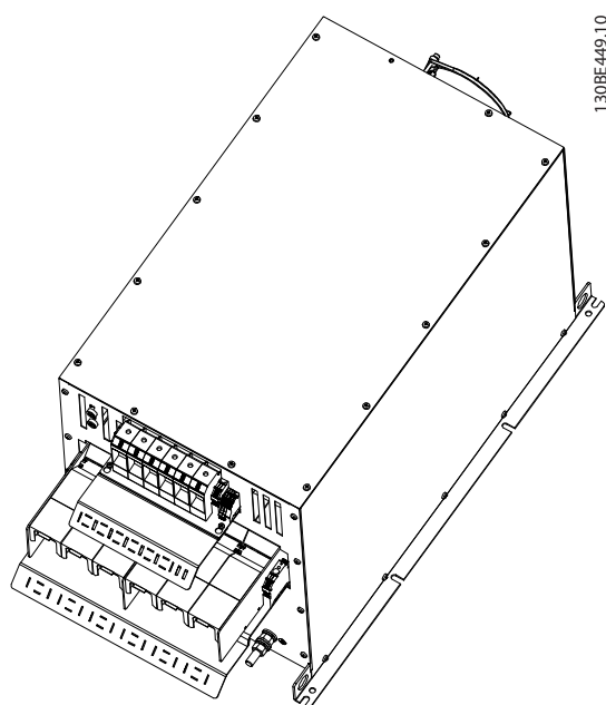
Рисунок 7.60 IP20 X8, внешний вентилятор 2, 3D-вид
