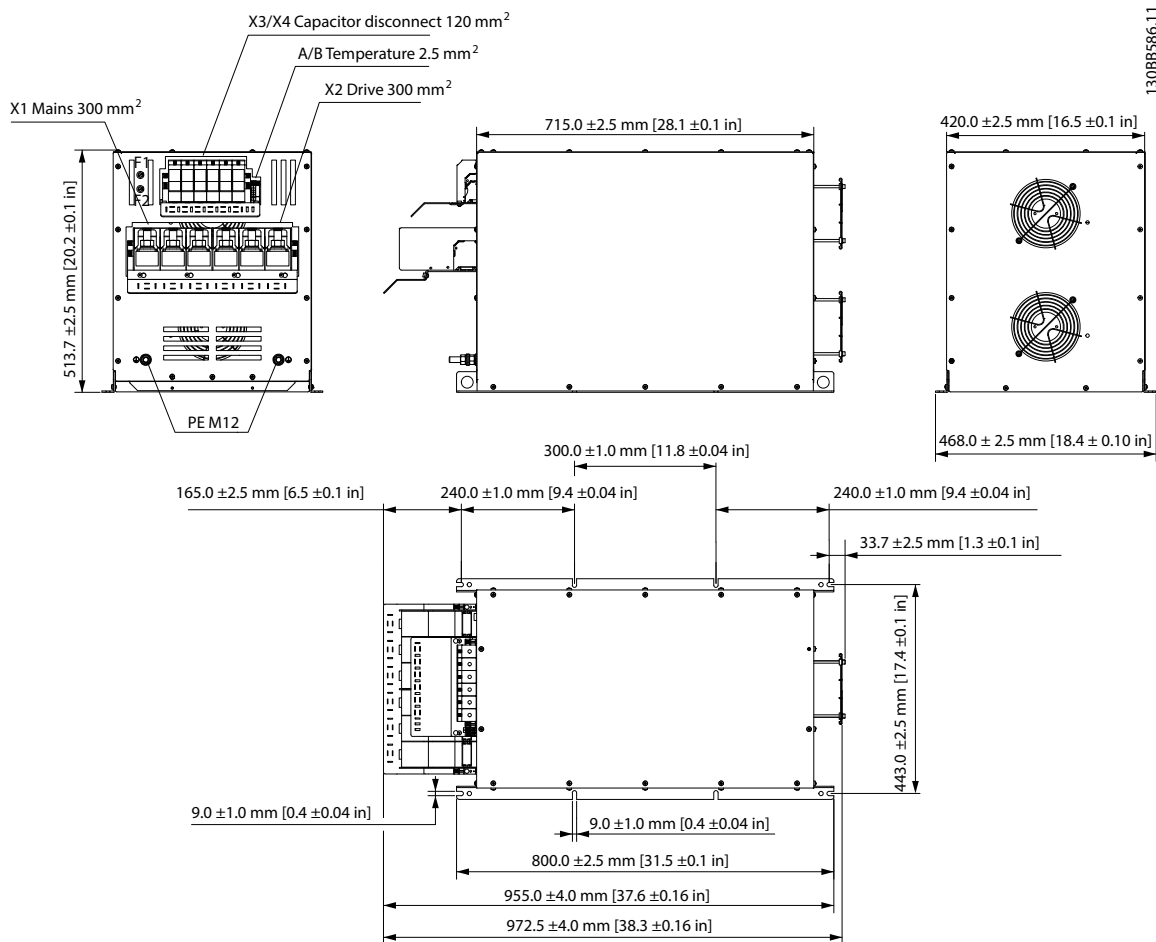
Рисунок 7.57 IP20 X8, внешний вентилятор 1
