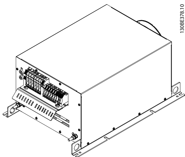
Рисунок 7.20 IP20 X3, внешний вентилятор 2, 3D-вид
