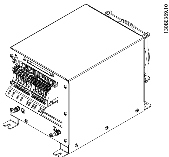
Рисунок 7.8 IP20 X1, внешний вентилятор 1, 3D-вид
