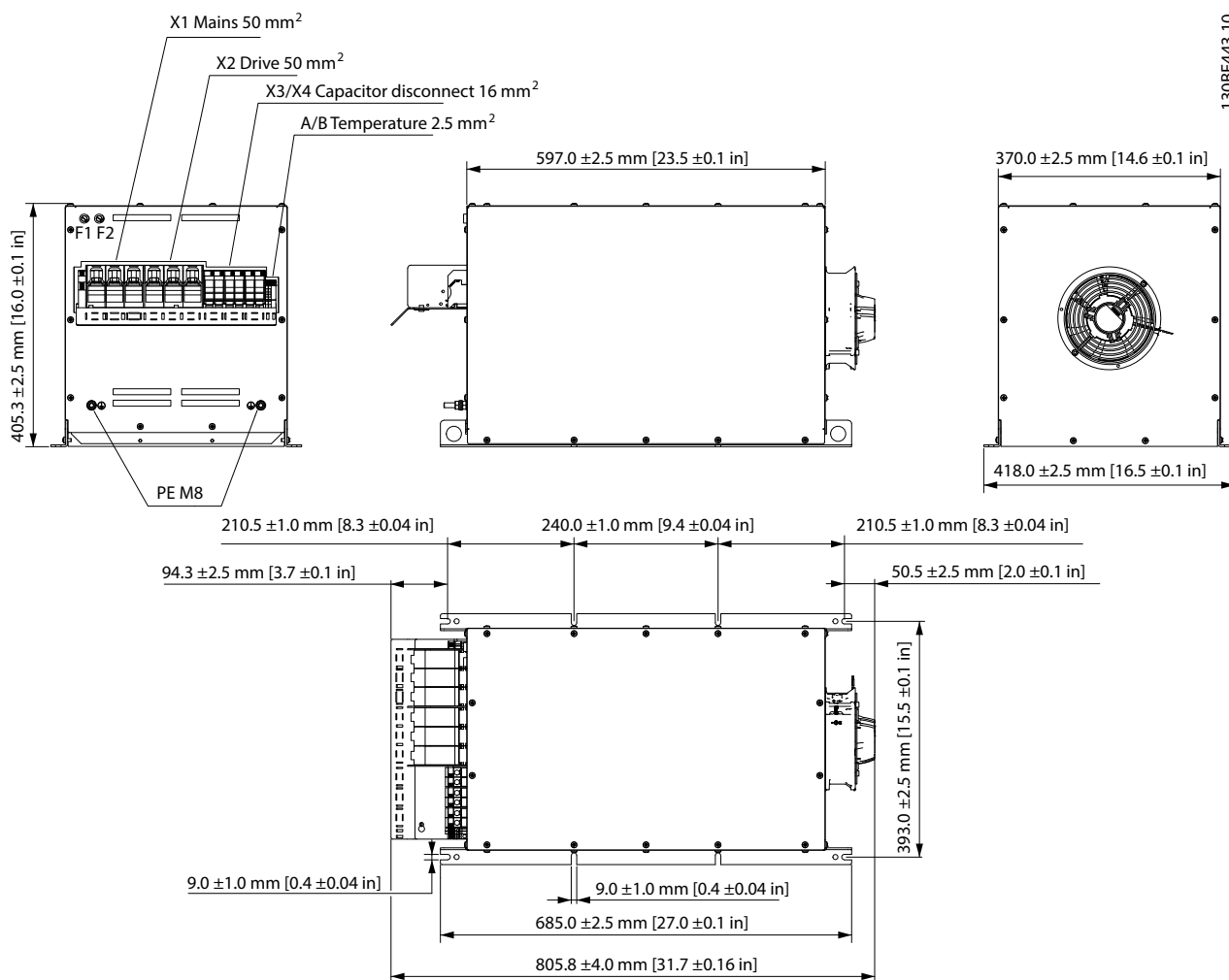
Рисунок 7.43 IP20 X6, внешний вентилятор 2
