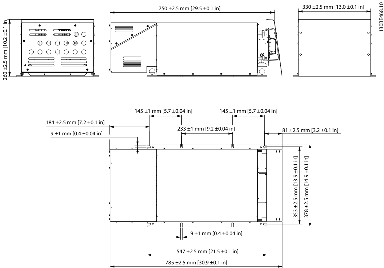
Рисунок 7.75 IP21 X3, внешний вентилятор 2
