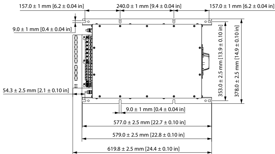
Рисунок 7.23 IP20 X4, внутренний вентилятор 2
