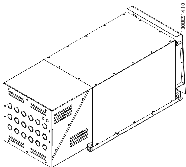
Рисунок 7.104 X7 IP21, внутренний вентилятор 2, 3D-вид
