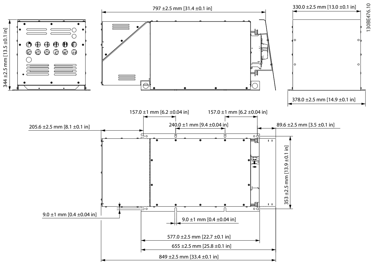
Рисунок 7.83 IP21 X4, внешний вентилятор 2
