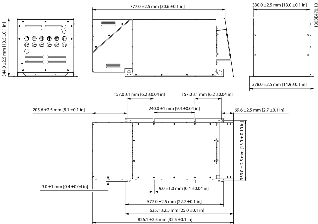
Рисунок 7.77 IP21 X4, внутренний вентилятор 1
