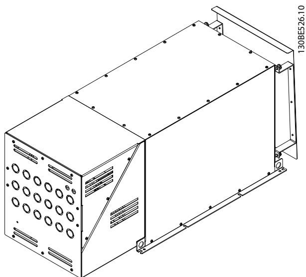
Рисунок 7.114 X8 IP21, внешний вентилятор 1, 3D-вид
