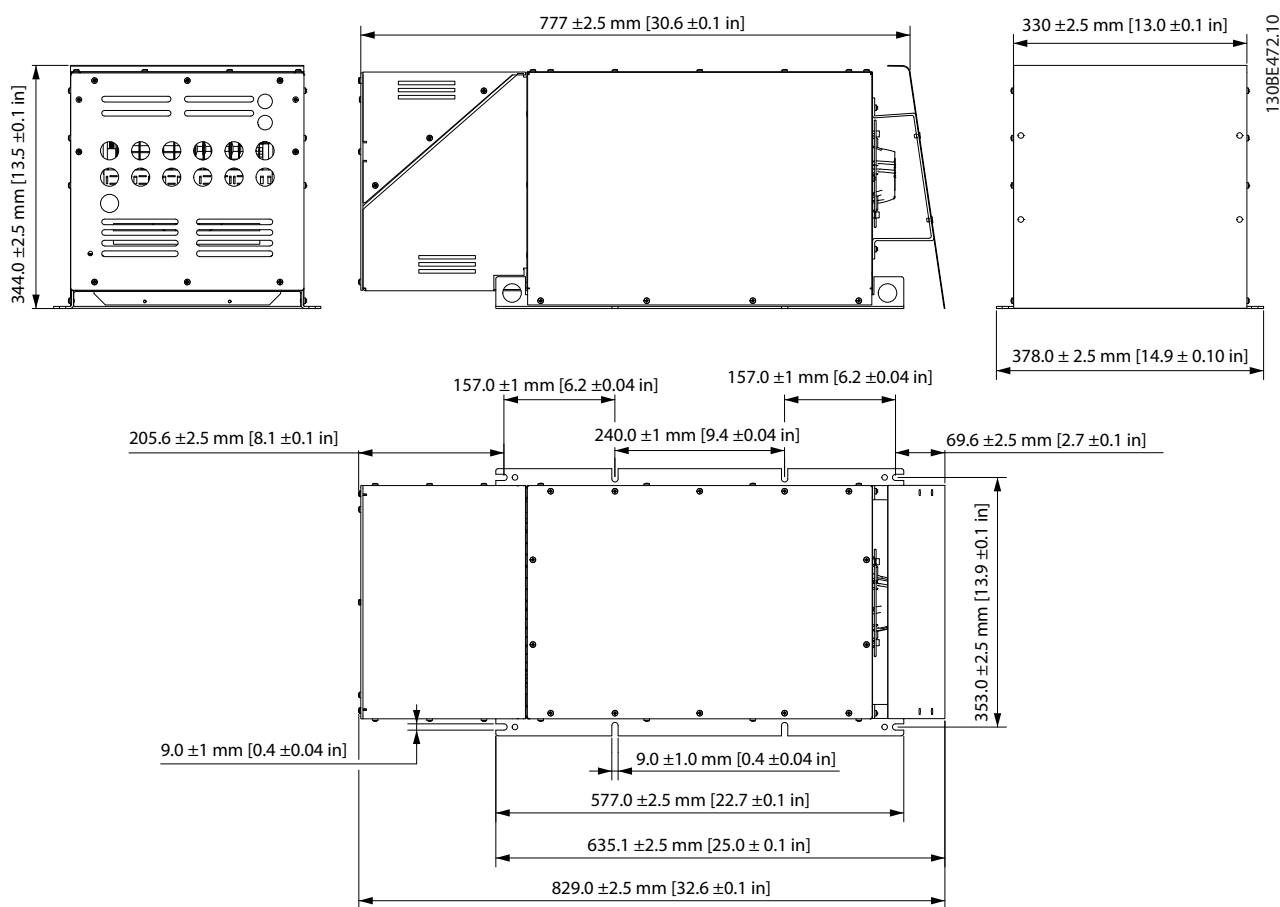
Рисунок 7.79 IP21 X4, внутренний вентилятор 2
